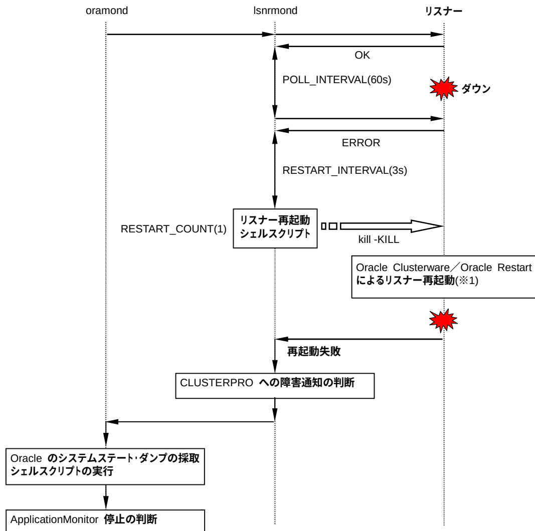
図 4-13 リスナー監視エラー時の動作 (Oracle Clusterware／Oracle Restart によってリスナーが再起動されなかった場合)
