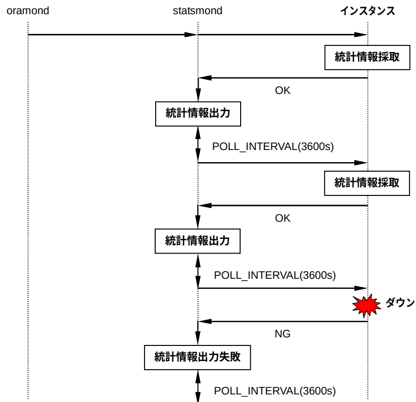
図 4-28 統計情報採取時の動作
