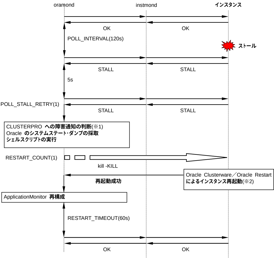
図 4-6 Oracle バックグラウンドプロセスのストール時の動作
