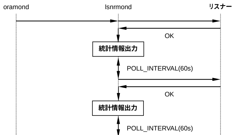
図 4-9 リスナー監視時の動作
