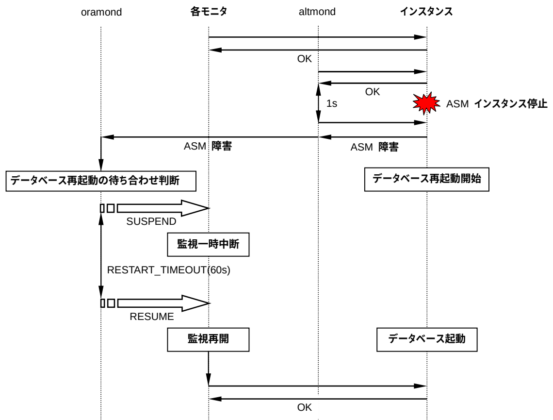
図 4-31 ASM インスタンス停止に伴うデータベースの再起動時の監視動作
