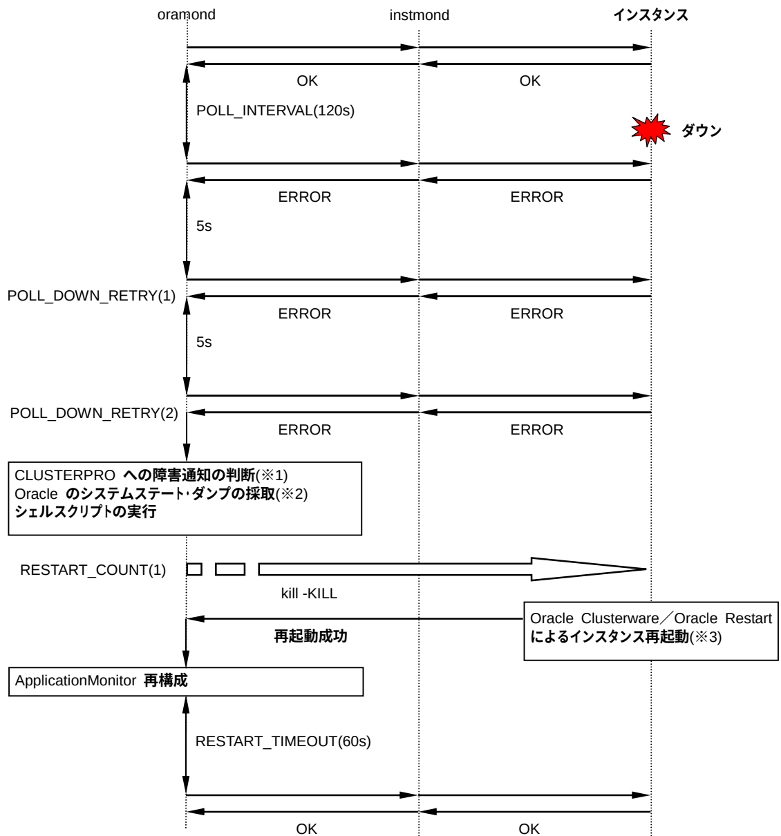
図 4-4 インスタンス監視エラー時の動作 (Oracle Clusterware／Oracle Restart によってインスタンスが再起動された場合)
