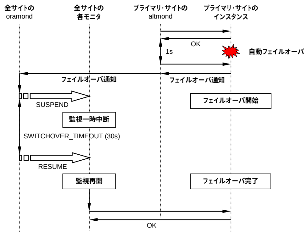
図 4-30 Oracle Data Guard Broker による自動フェイルオーバー時の監視動作
