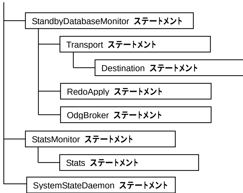
図 3-1 ステートメントの階層
