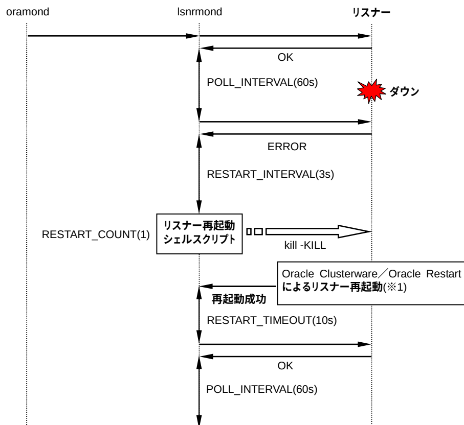
図 4-12 リスナー監視エラー時の動作 (Oracle Clusterware／Oracle Restart によってリスナーが再起動された場合)
