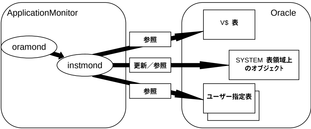
図 4-2 インスタンス監視モニタの概要
