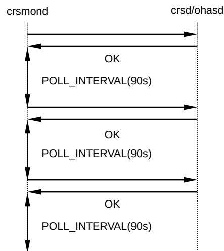
図 4-32 Oracle Clusterware／Oracle Restart 監視時の動作
