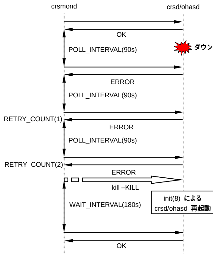
図 4-34 crsd/ohasd 監視エラー時の動作 (init(8) によって crsd/ohasd が再起動された場合)
