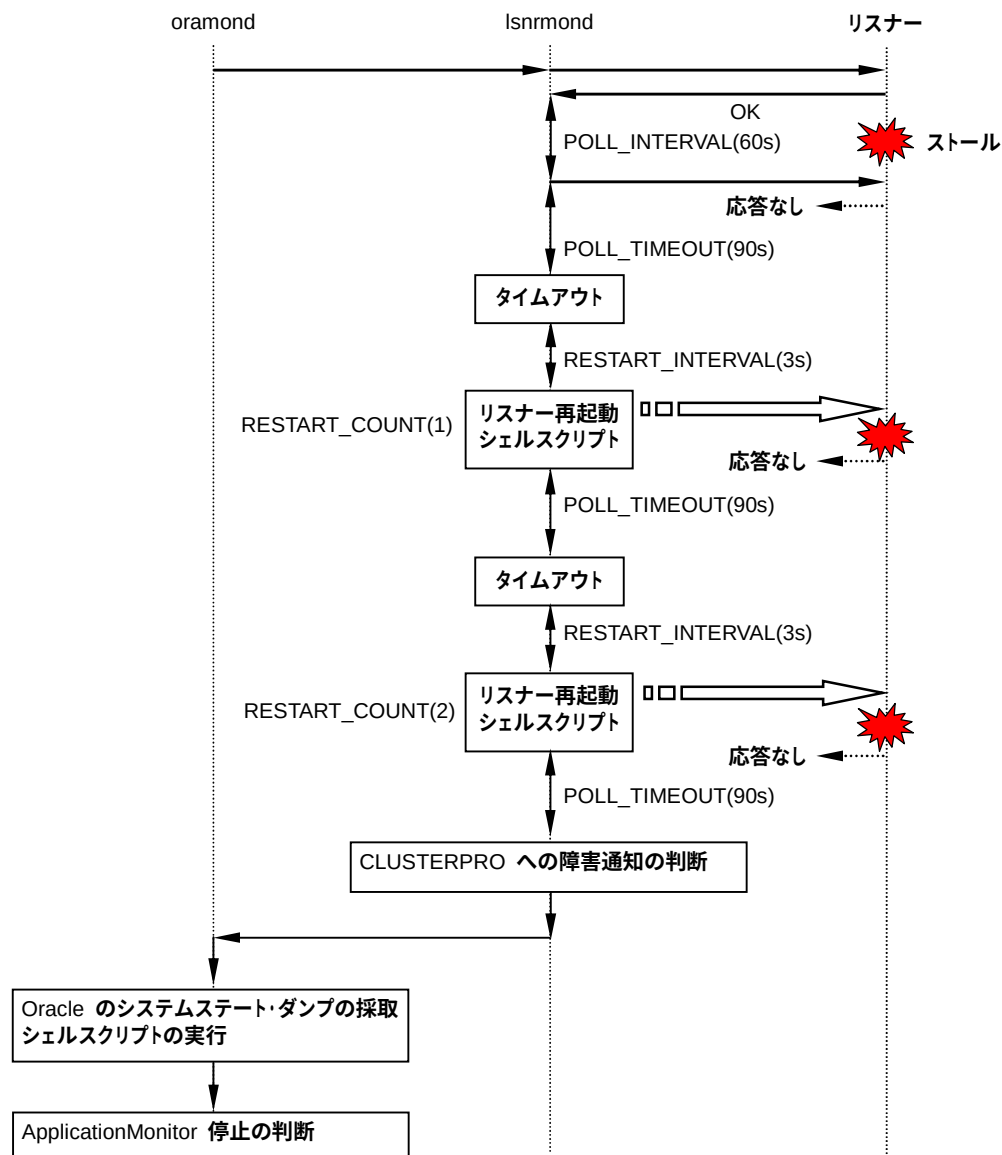
図 4-14 リスナー監視タイムアウト時の動作 (ApplicationMonitor によるリスナー再起動が失敗した場合)
