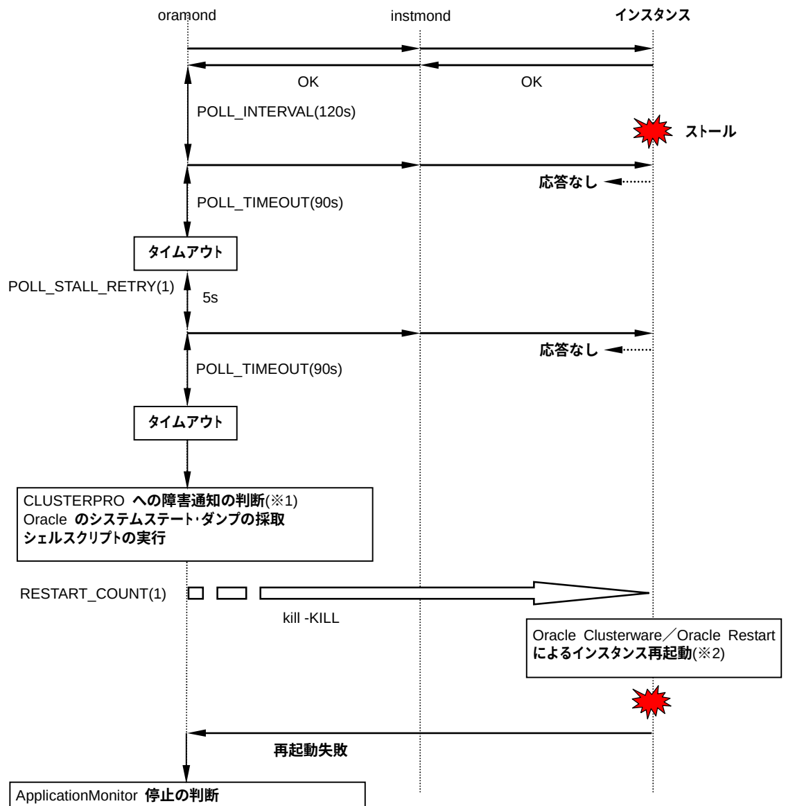
図 4-7 インスタンス監視タイムアウト時の動作
