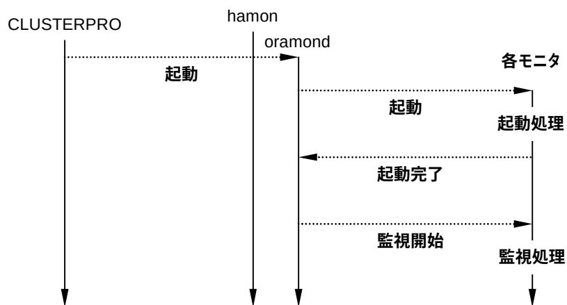
図 4-1 各モニタ起動時の動作
