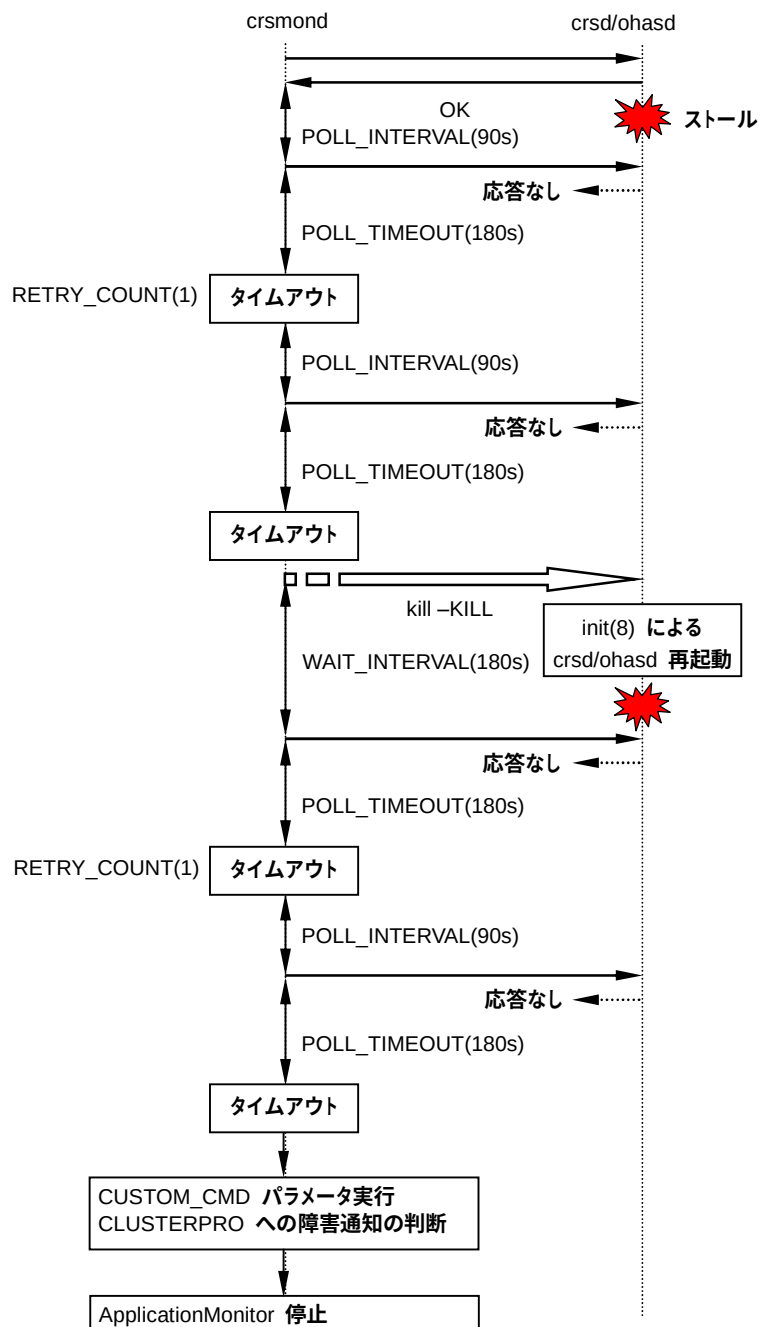
図 4-36 crsd/ohasd 監視タイムアウト時の動作
