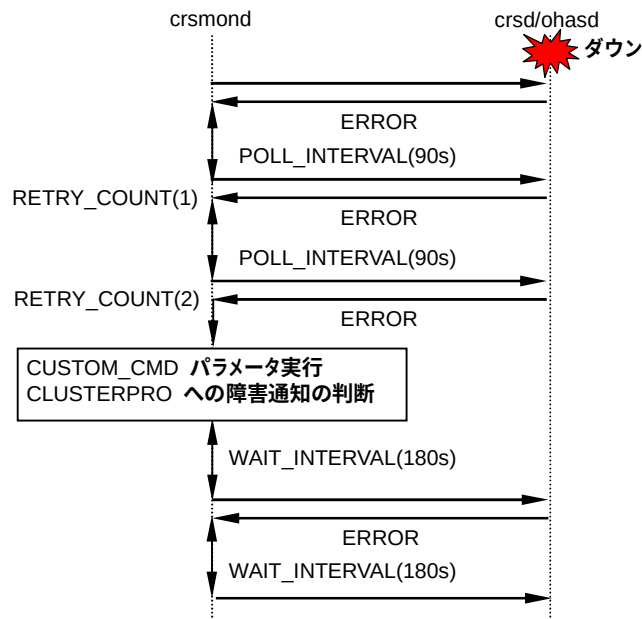
図 4-33 CRS 監視モニタ起動エラー時の動作
