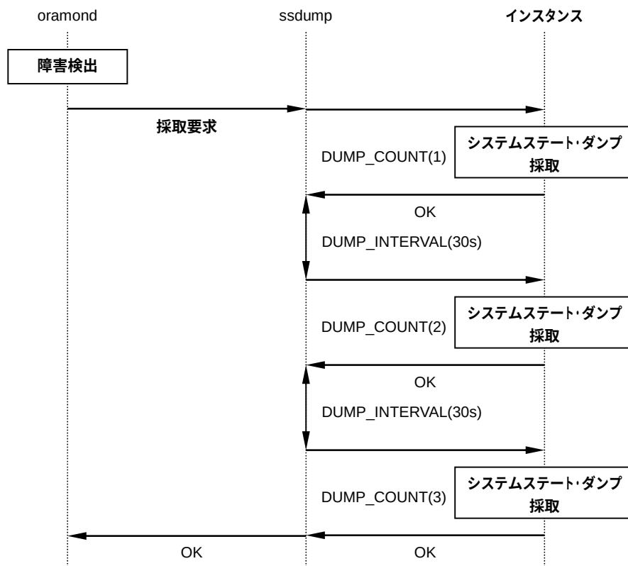
図 4-29 システムステート・ダンプ採取時の動作
