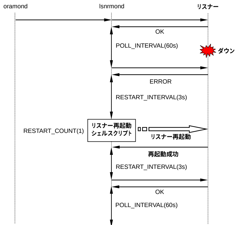
図 4-10 リスナー監視エラー時の動作 (ApplicationMonitor によってリスナーが再起動した場合)
