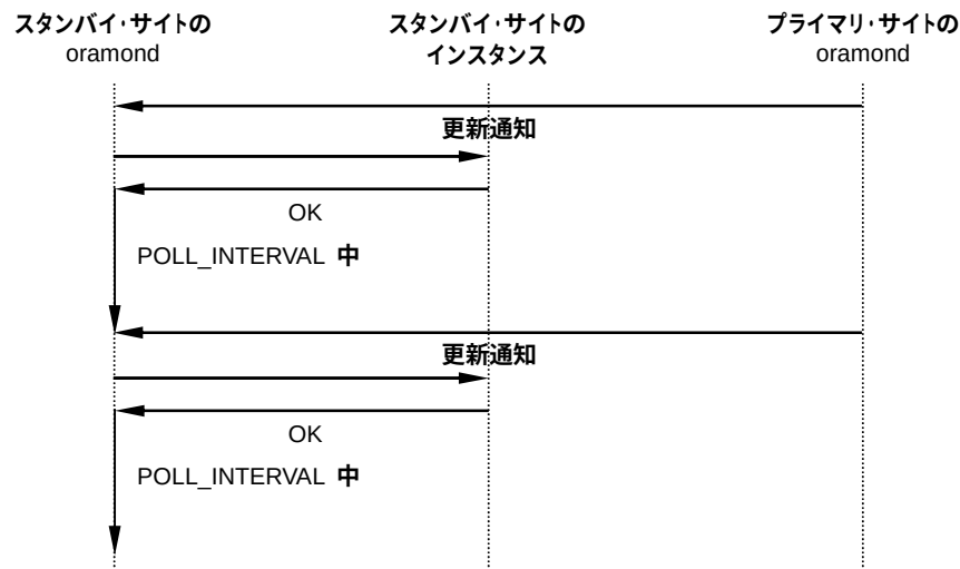
図 4-26 スタンバイ・インスタンスの Oracle Data Guard Broker プロセスの状態監視時の動作 (更新通知による監視)
