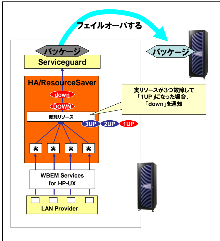
図 2-9 数による監視機能
