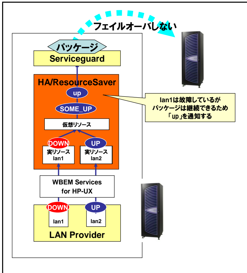
図 2-4 監視対象の抽象化機能
