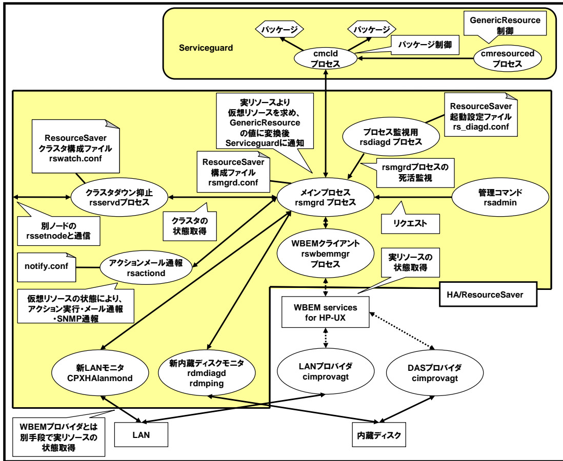
図 2-3 HA/ResourceSaver ソフトウェア構成
