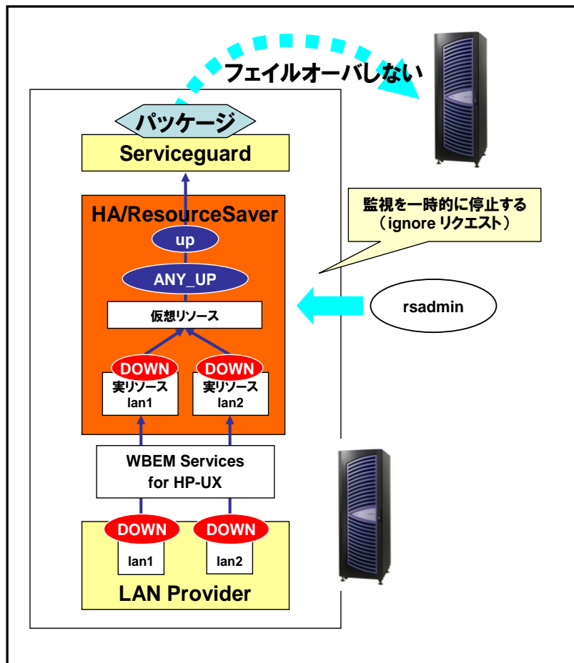
図 2-11 クラスタ暫定稼動機能
