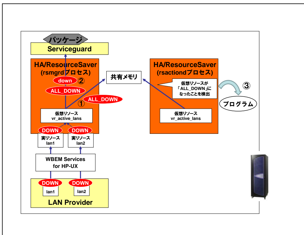
図 2-14 アクション機能
