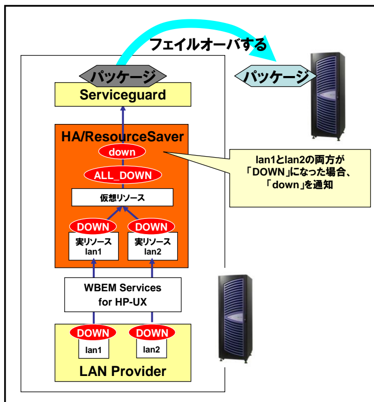
図 2-5 監視対象の抽象化機能
