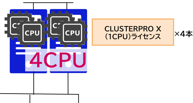
4. 非対象機種どうしの共有ディスク型の場合
