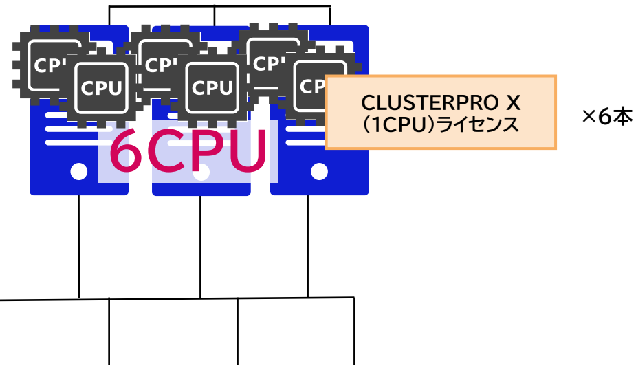
4. 2:1スタンバイでスタンバイのCPUが少ない場合
