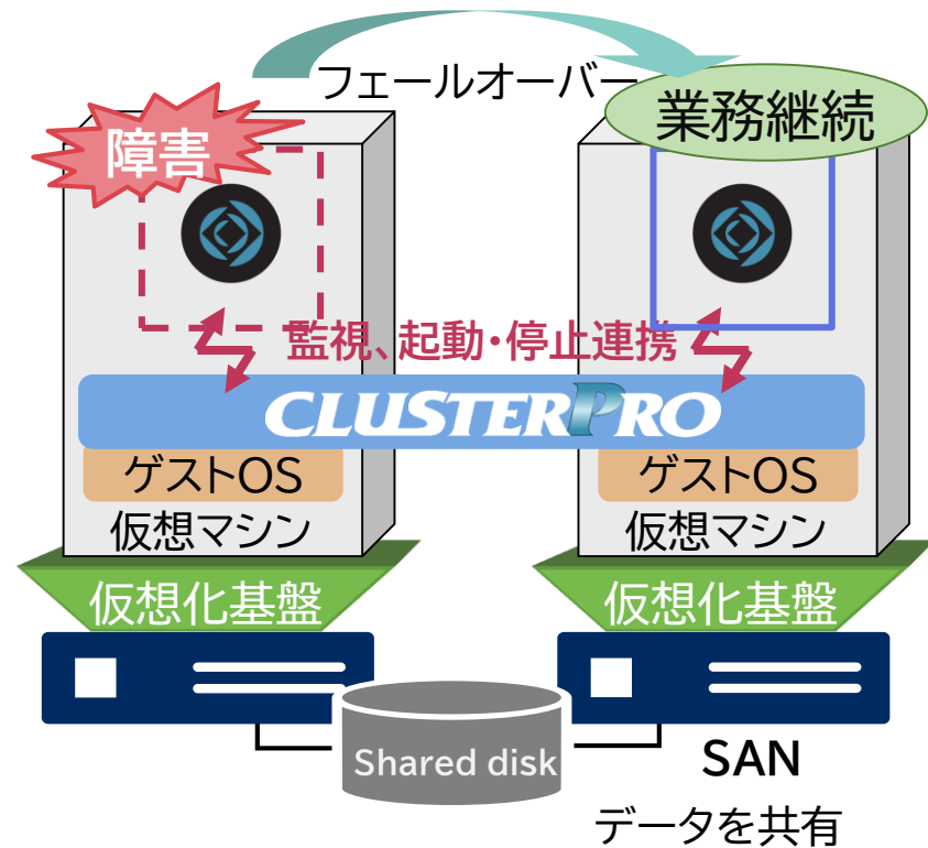
2ノード・共有ディスク型 ゲストOS間クラスター
