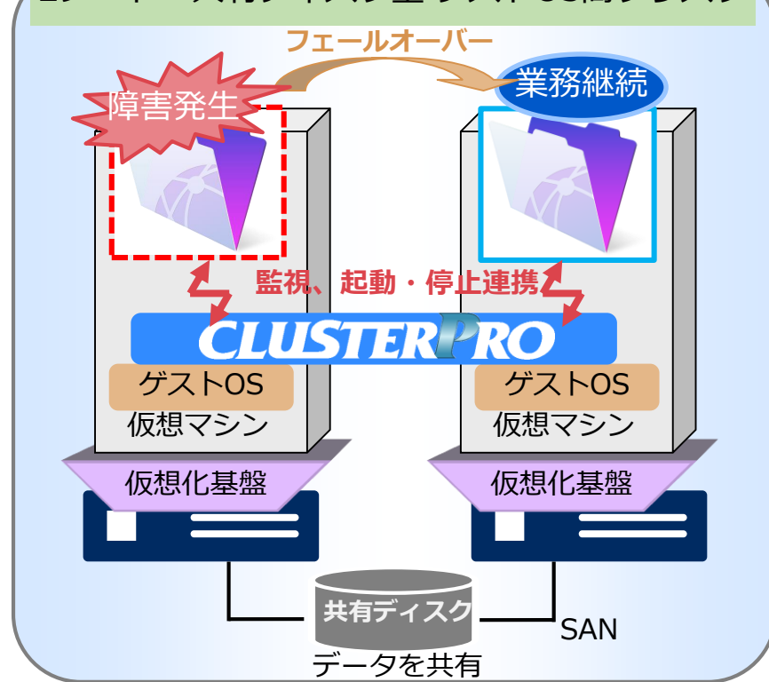
2ノード・共有ディスク型 ゲストOS間クラスタ
