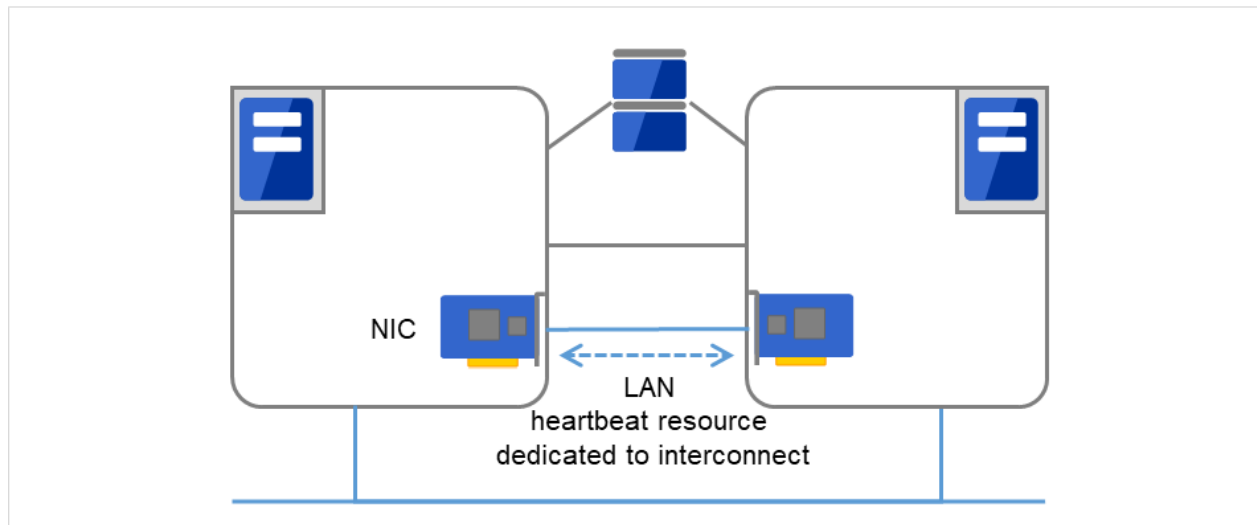
図 5.1 カーネルモード LAN ハートビート（プライマリインタコネクト）
