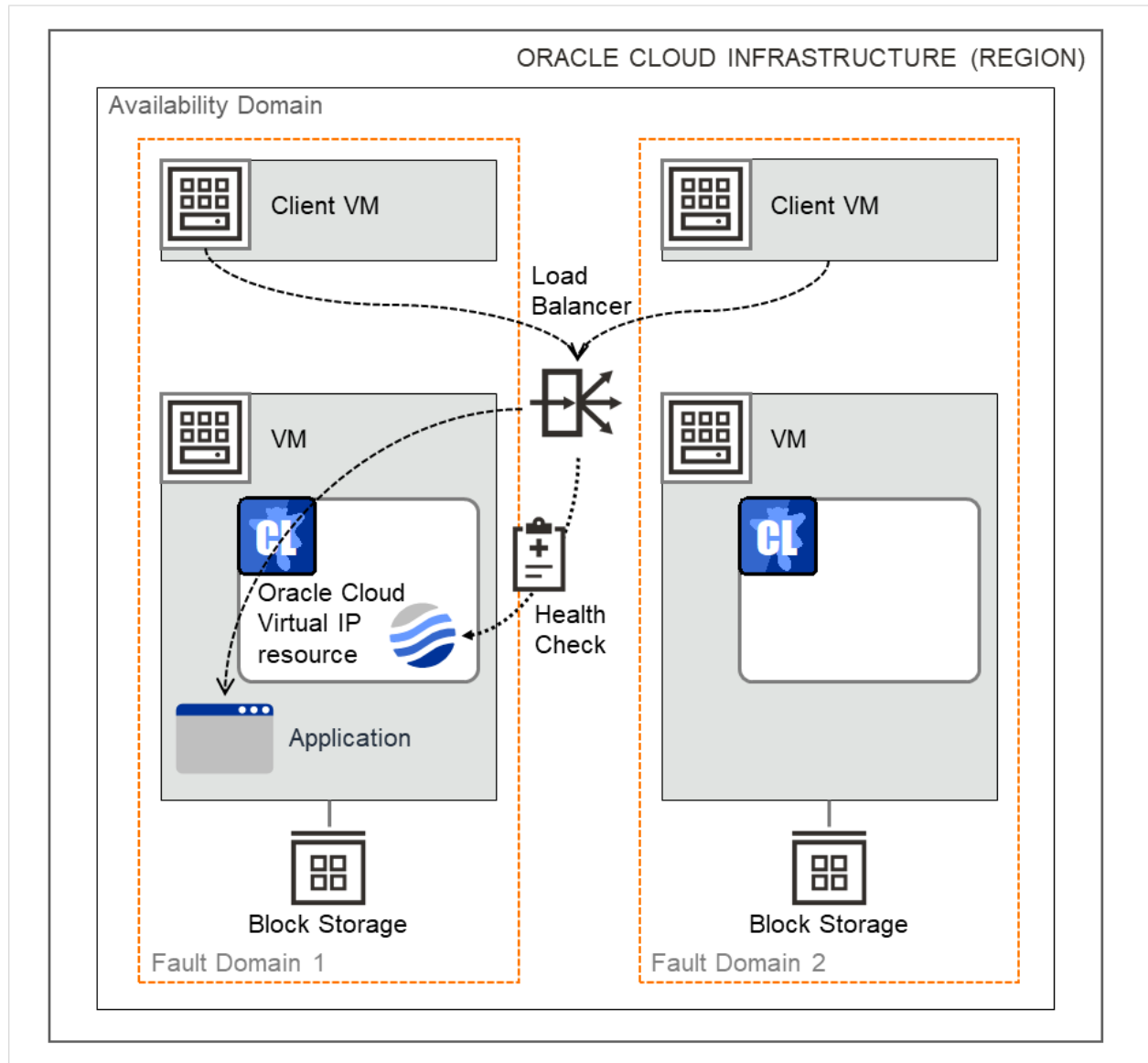
図 3.118 Oracle Cloud 仮想 IP リソースを使用する構成（プライベートロードバランサ）
