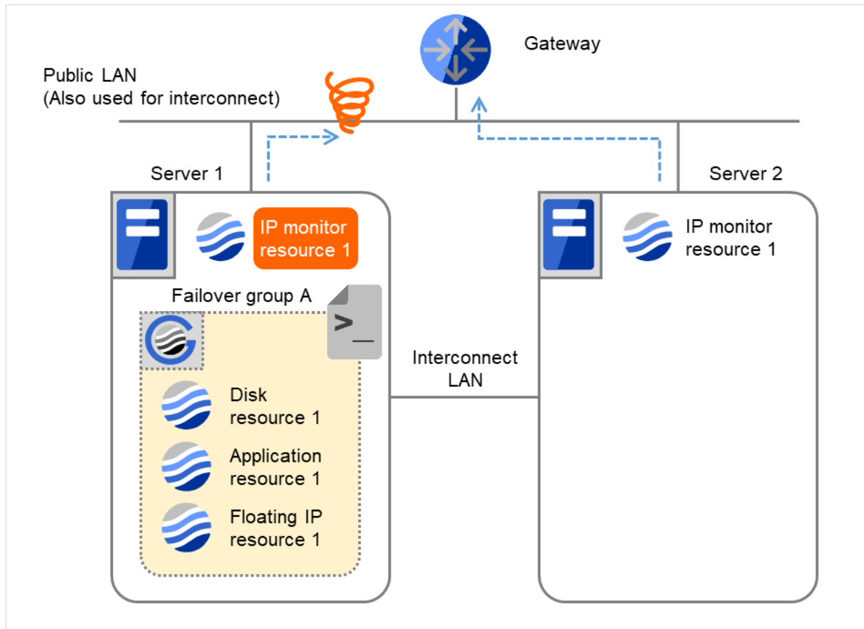
図 4.10 IP 監視リソース異常検出の流れ（片サーバのみ異常検出）（4）
