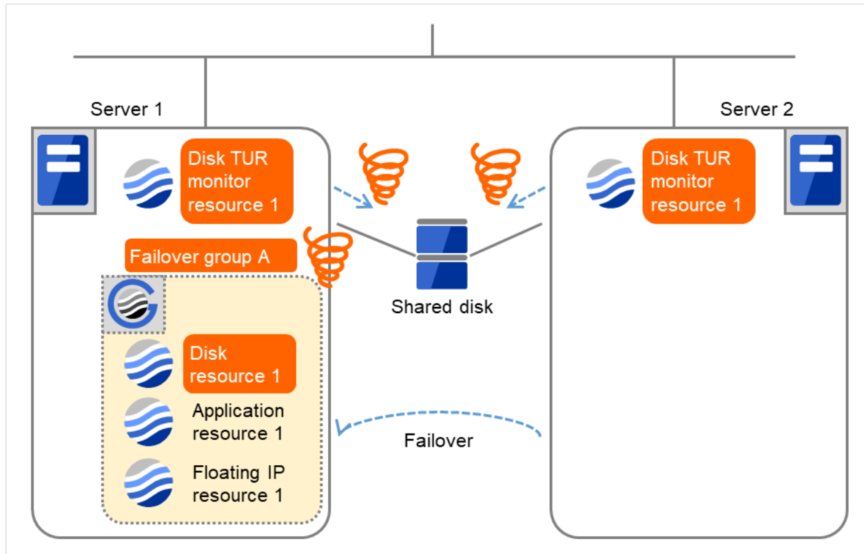
図 4.44 ディスク TUR 監視リソース異常検出の流れ (11)
