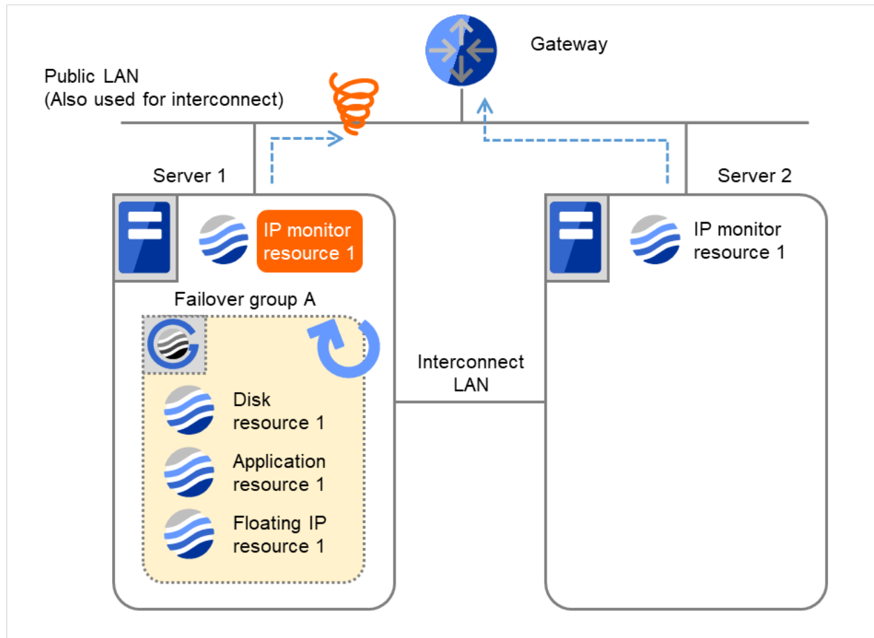
図 4.11 IP 監視リソース異常検出の流れ（片サーバのみ異常検出）（5）
