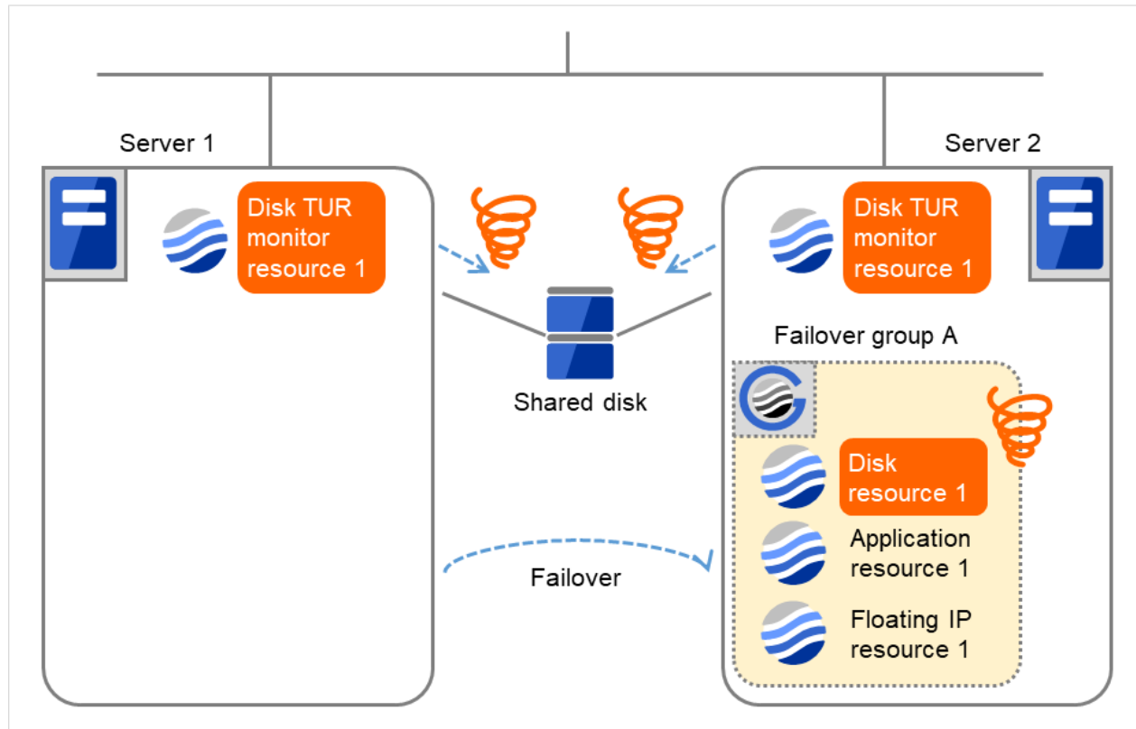
図 4.41 ディスク TUR 監視リソース異常検出の流れ (8)
