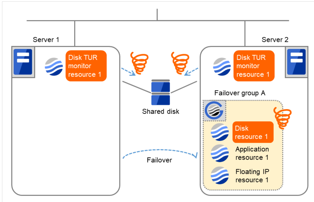
図 4.37 ディスク TUR 監視リソース異常検出の流れ (4)
