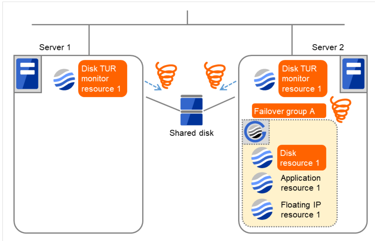
図 4.42 ディスク TUR 監視リソース異常検出の流れ (9)
