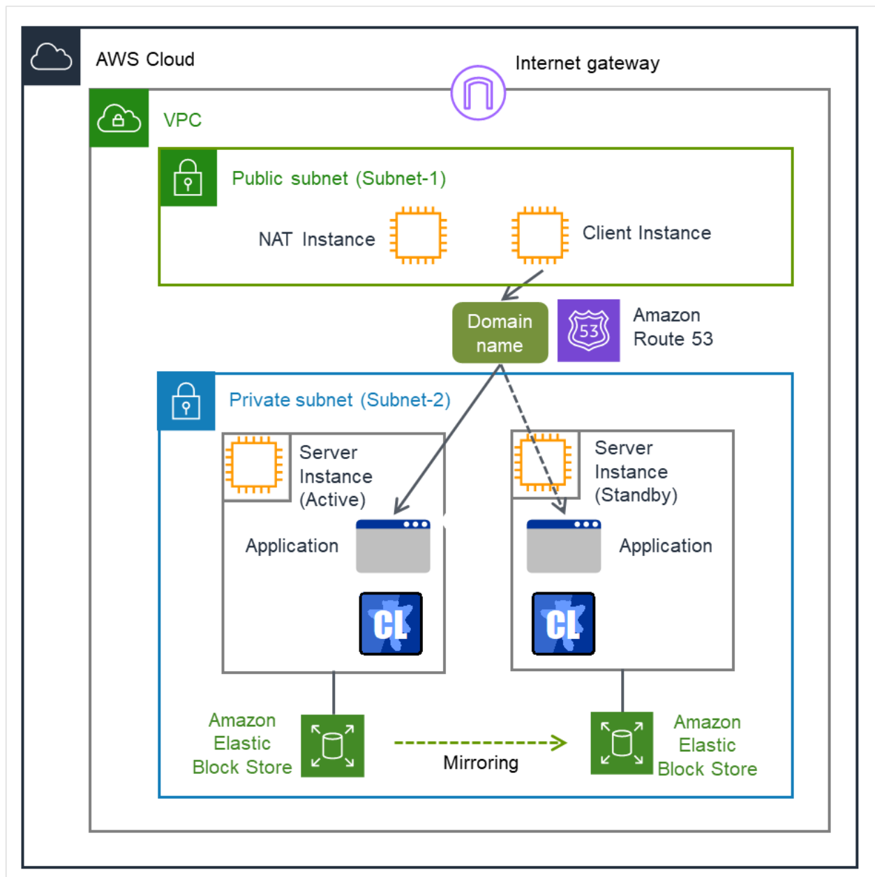
図 3.112 AWS DNS リソースを使用する構成
