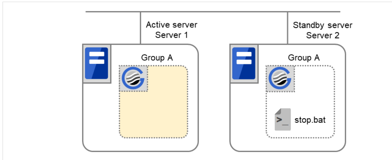
図 3.87 状態とスクリプト実行 (Group A の通常シャットダウン) (1)
