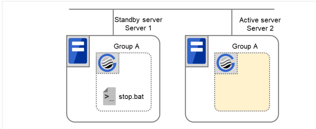
図 3.91 状態とスクリプト実行 (Group A の移動) (1)
