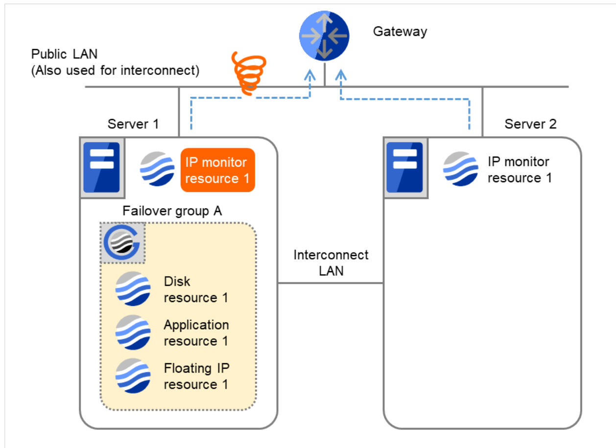
図 4.8 IP 監視リソース異常検出の流れ (片サーバのみ異常検出) (2)
