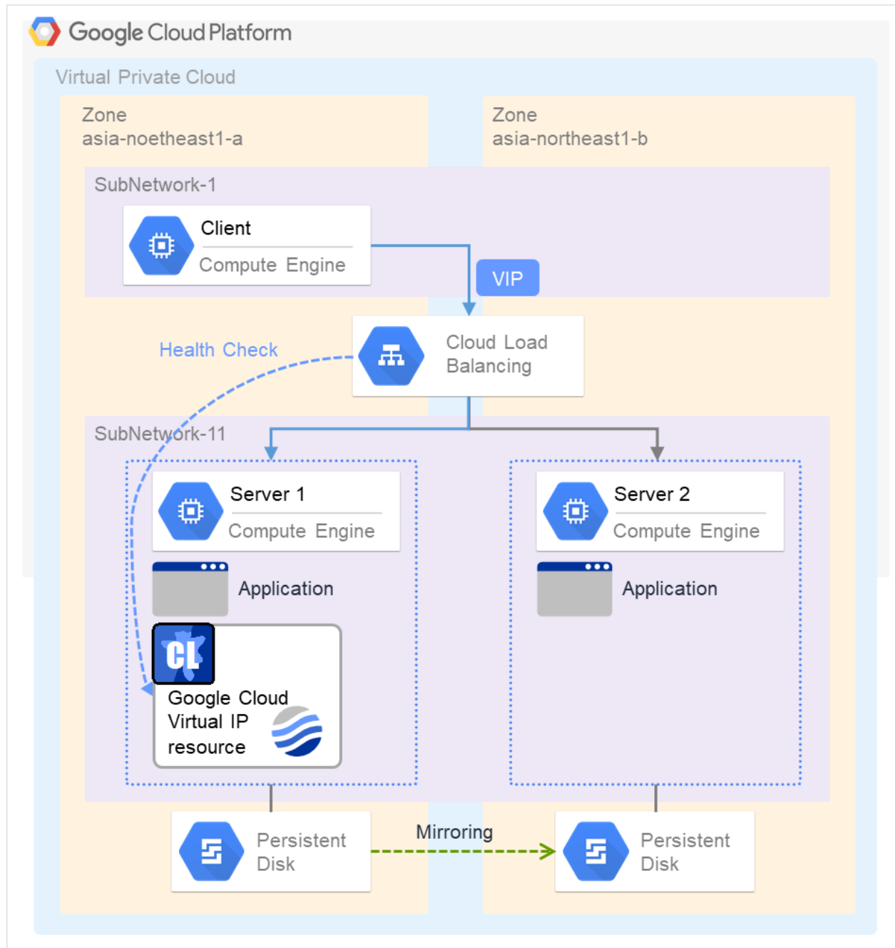
図 3.116 Google Cloud 仮想 IP リソースを使用する構成
