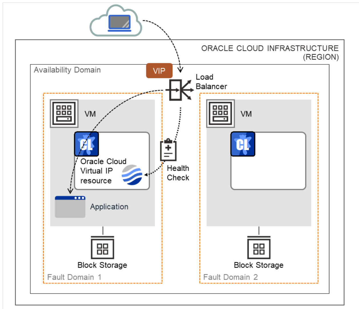
図 3.117 Oracle Cloud 仮想 IP リソースを使用する構成
