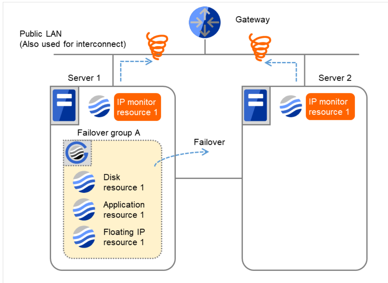
図 4.19 IP 監視リソース異常検出の流れ（両サーバで異常検出）(6)
