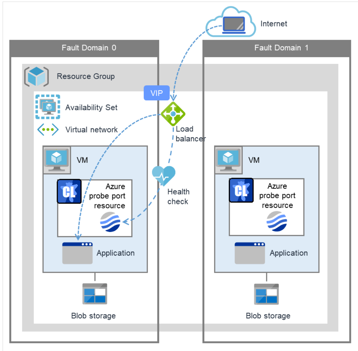
図 3.113 Azure プローブポートリソースを使用する構成
