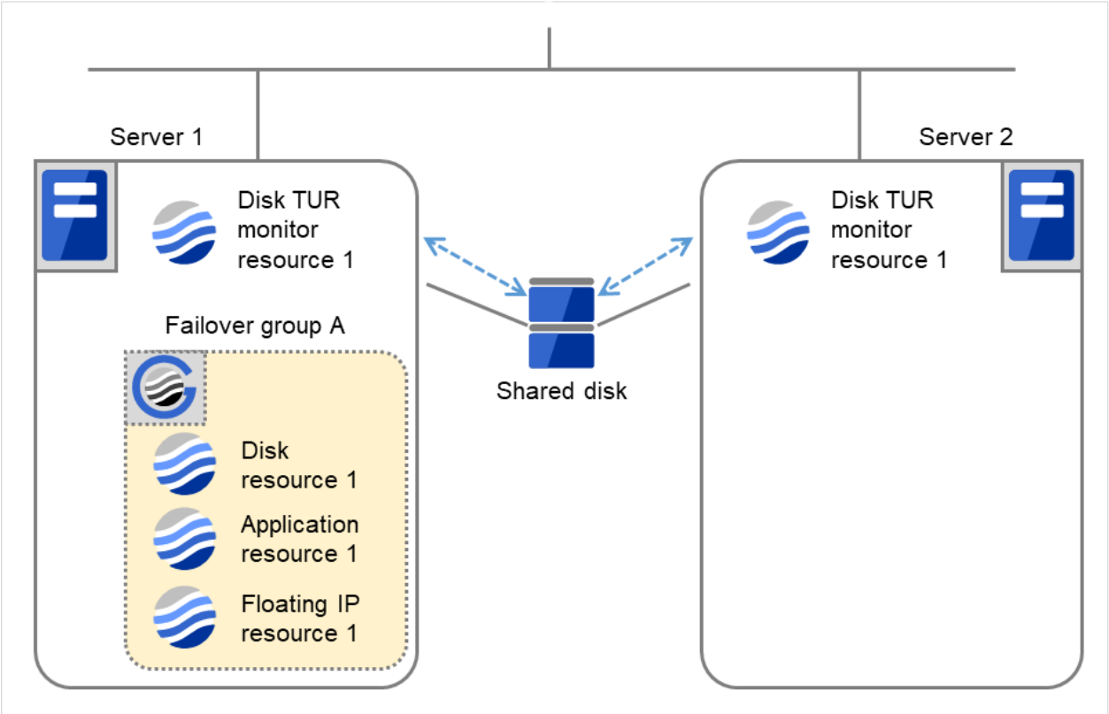
図 4.34 ディスク TUR 監視リソース異常検出の流れ (1)
