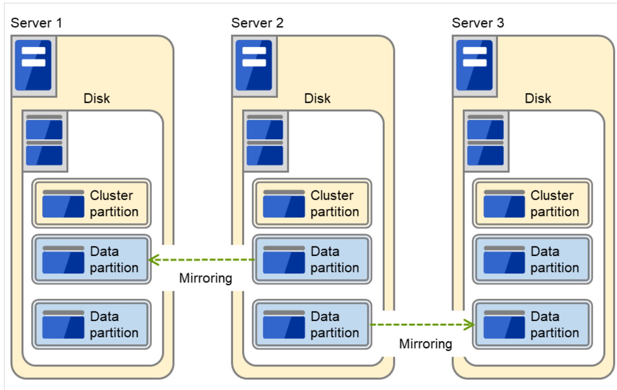
図 3.49 ディスク内の複数領域をミラーパーティションにする場合（サーバ 3 台）
