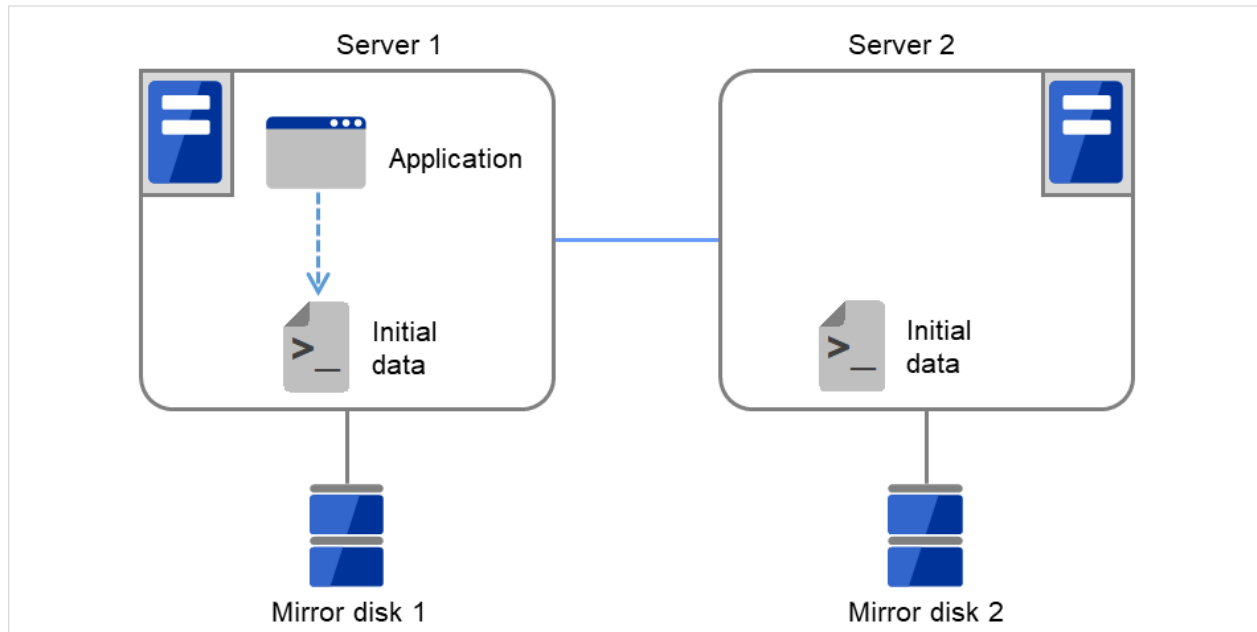
図 3.52 ミラーディスク構築例 (初期ミラー構築を行う) (1)
