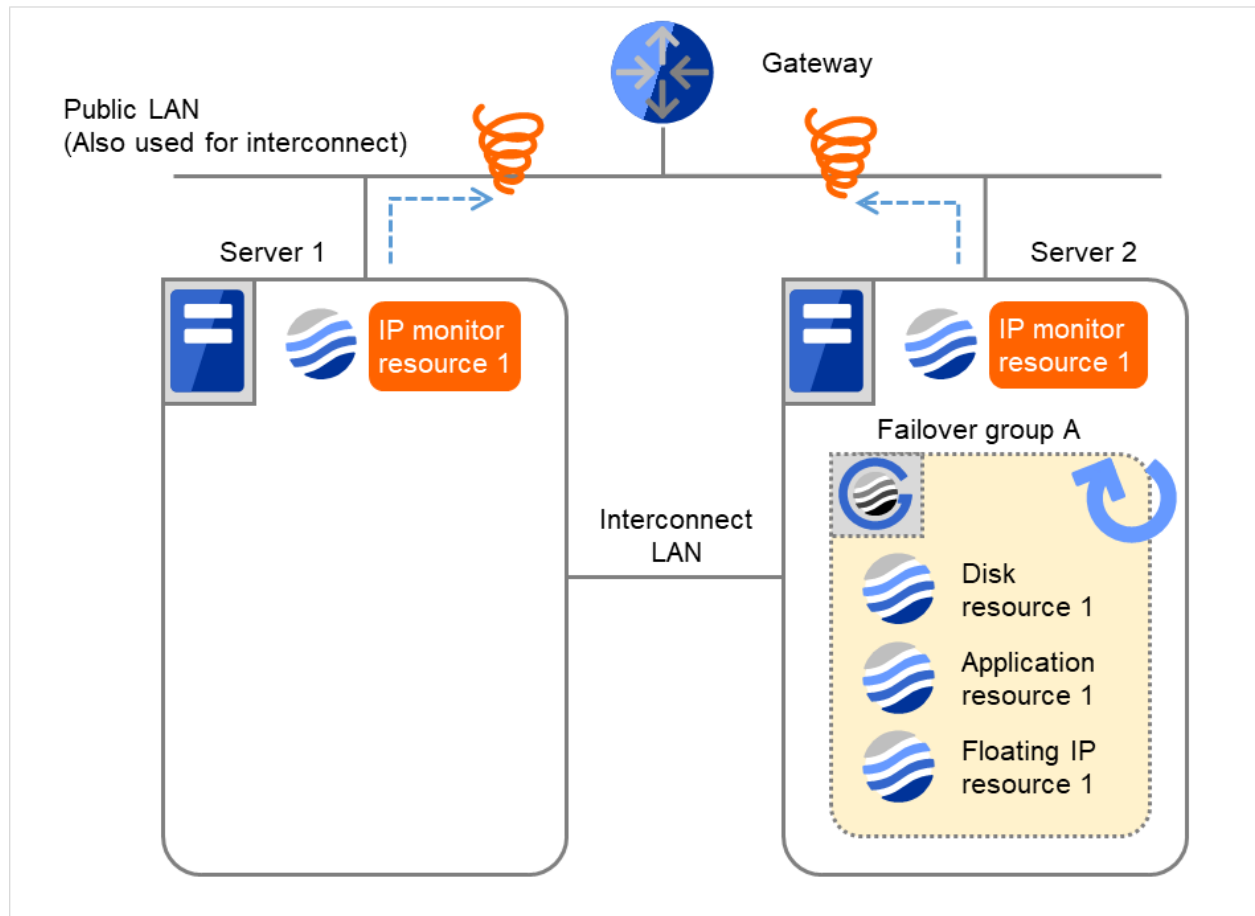
図 4.23 IP 監視リソース異常検出の流れ（両サーバで異常検出） (10)
