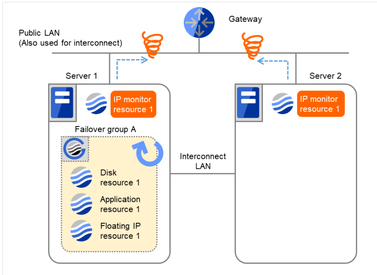
図 4.33 IP 監視リソース異常検出の流れ（監視異常からの復帰・正常）(6)
