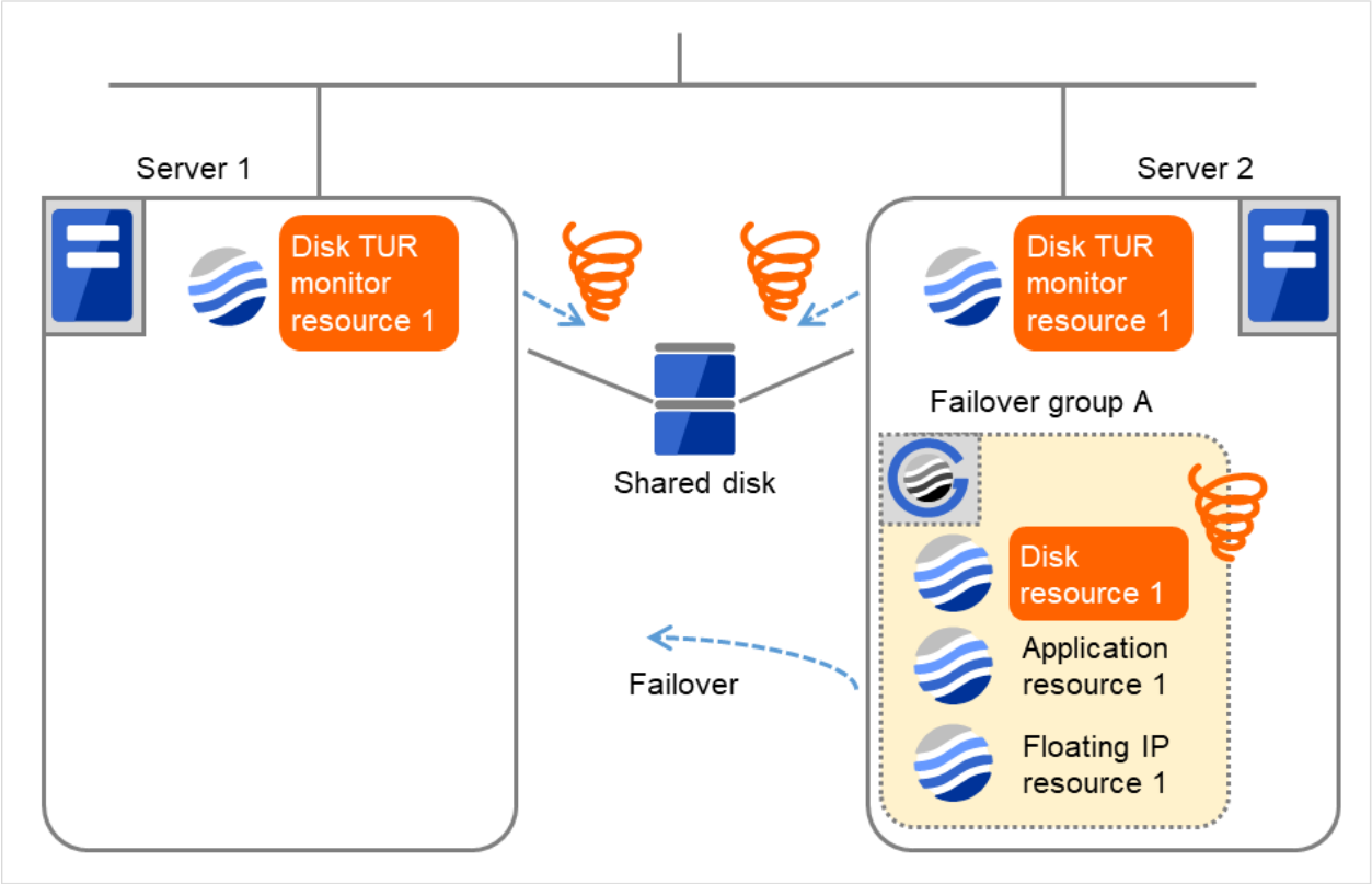
図 4.38 ディスク TUR 監視リソース異常検出の流れ (5)
