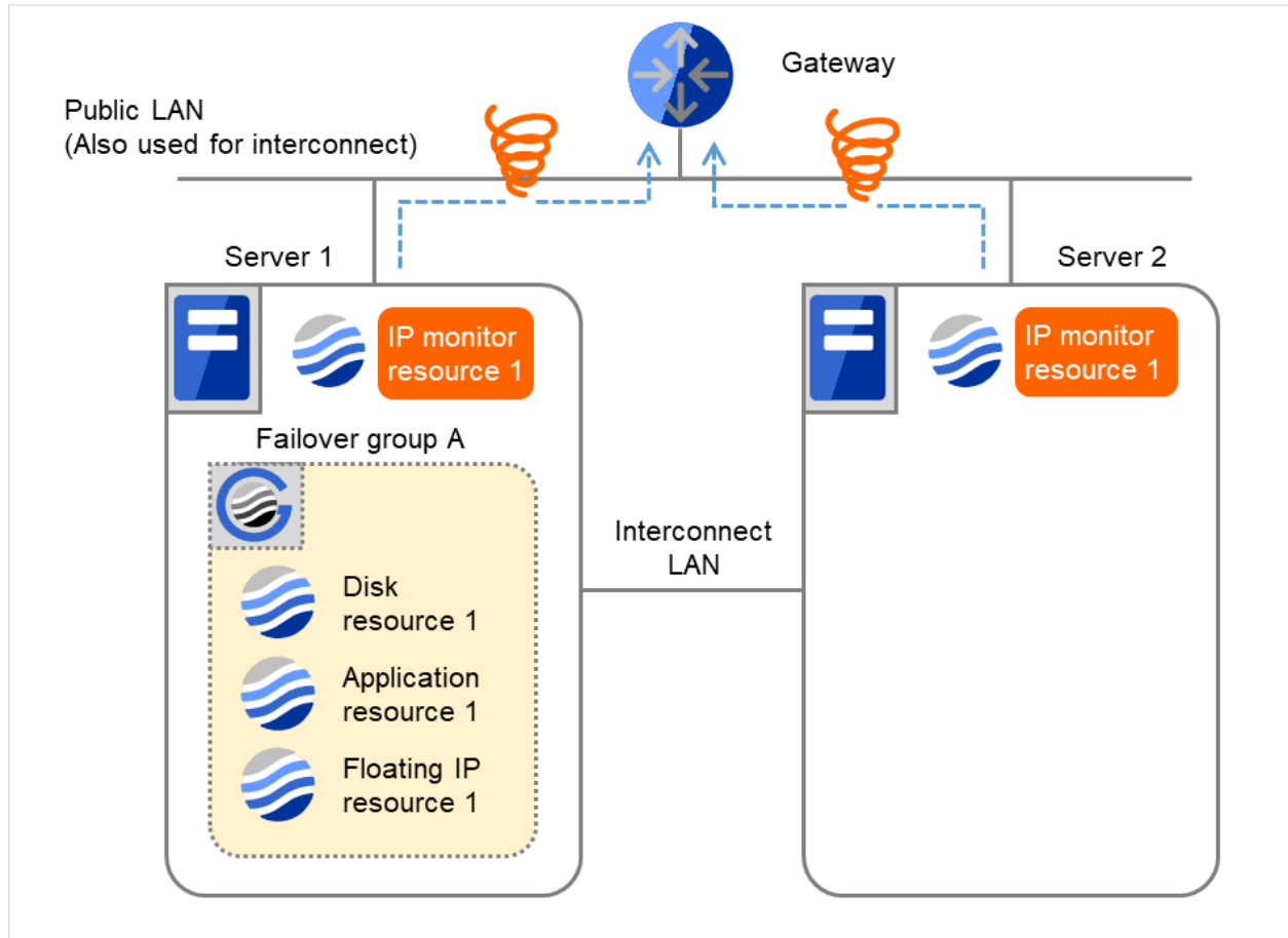
図 4.30 IP 監視リソース異常検出の流れ（監視異常からの復帰・正常）(3)
