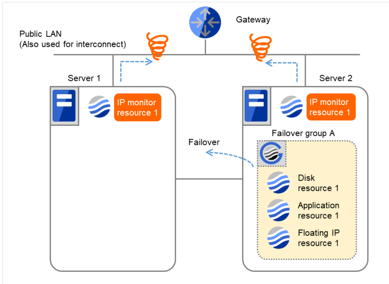
図 4.24 IP 監視リソース異常検出の流れ（両サーバで異常検出） (11)
