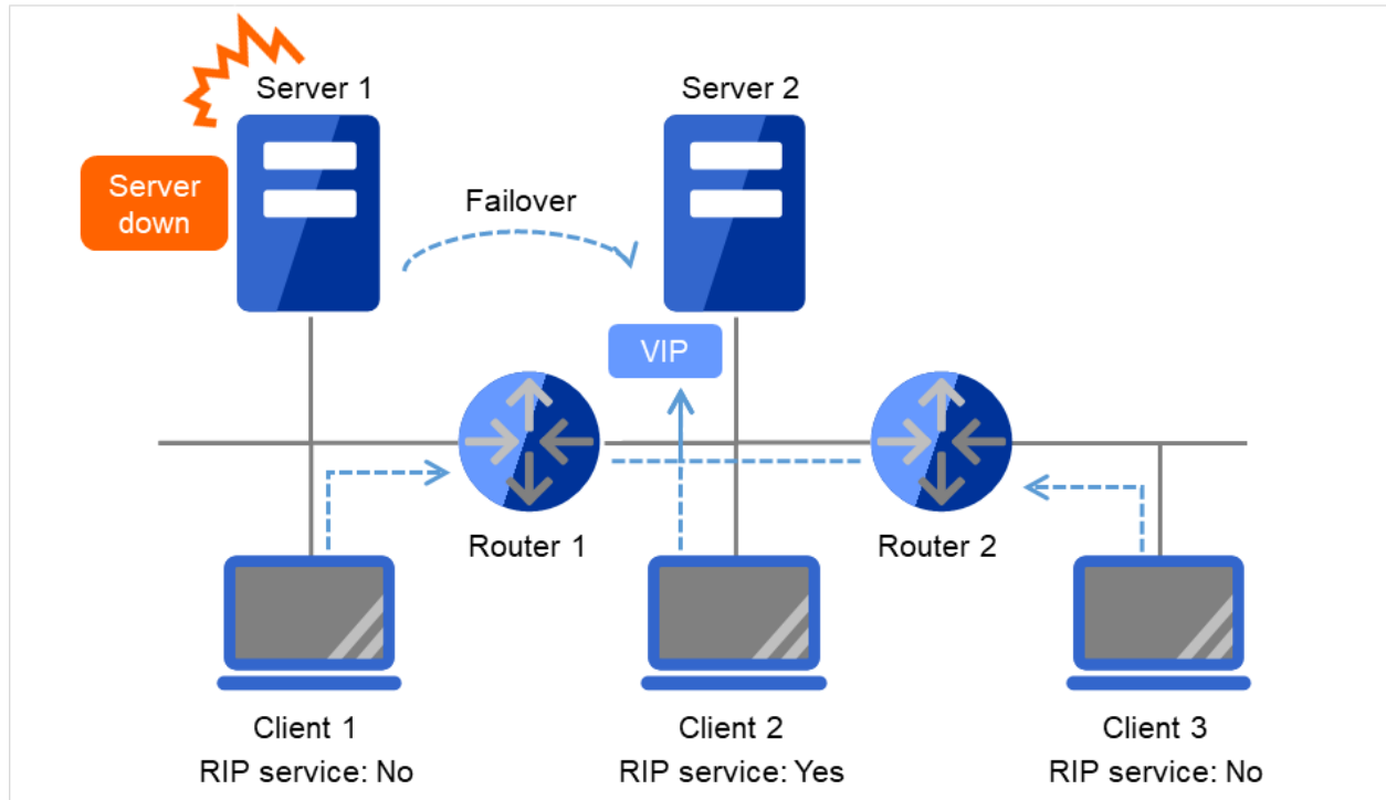
図 3.105 仮想 IP を使用した構成 (2)
