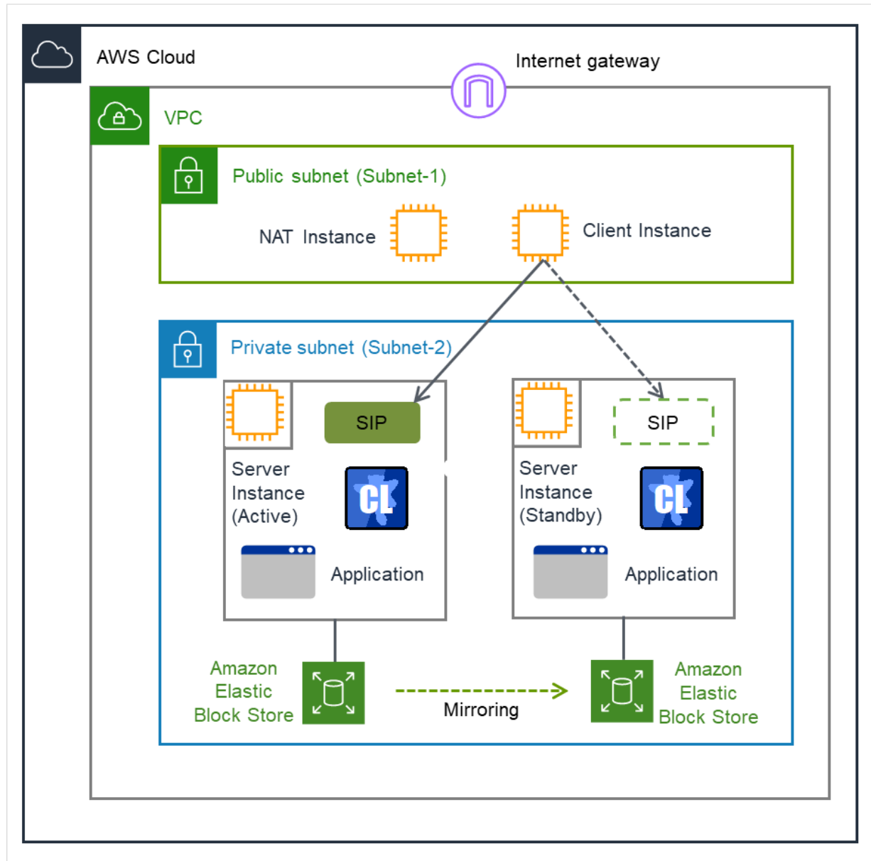
図 3.111 AWS セカンダリ IP リソースを使用する構成
