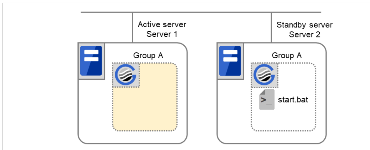
図 3.86 状態とスクリプト実行 (Group A の通常起動) (2)
