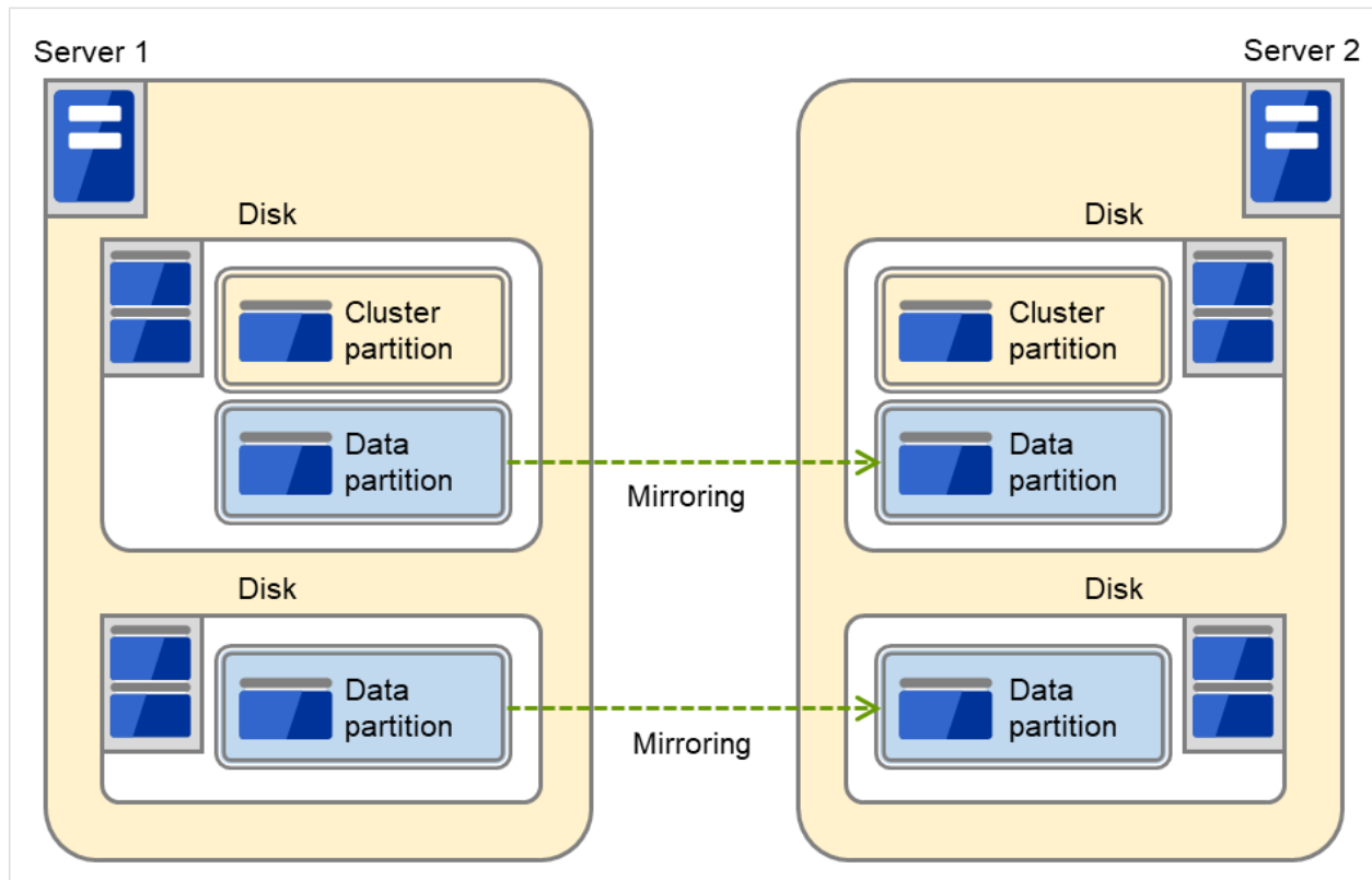
図 3.48 各ディスクをミラーパーティションにする場合
