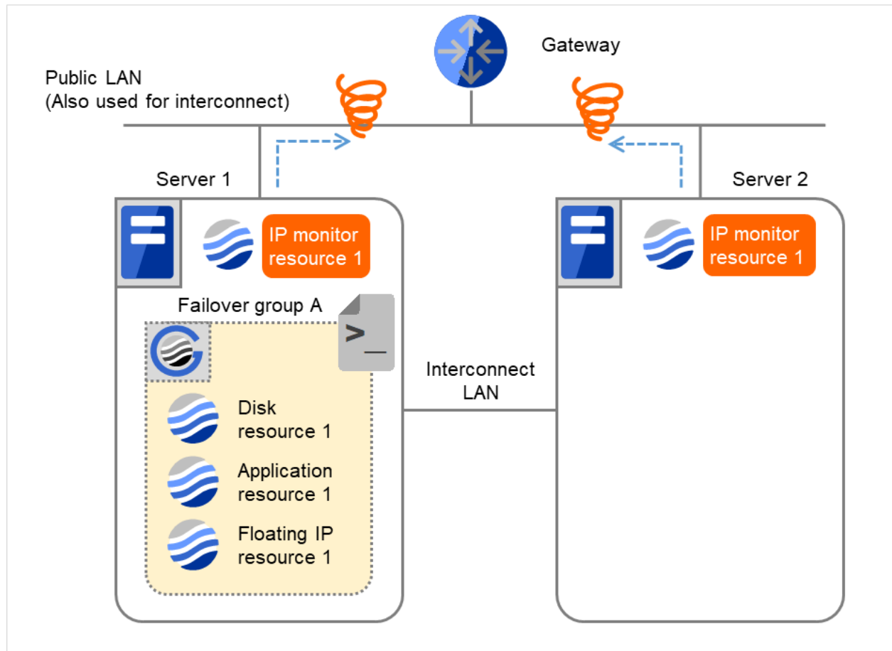
図 4.17 IP 監視リソース異常検出の流れ（両サーバで異常検出）（4）
