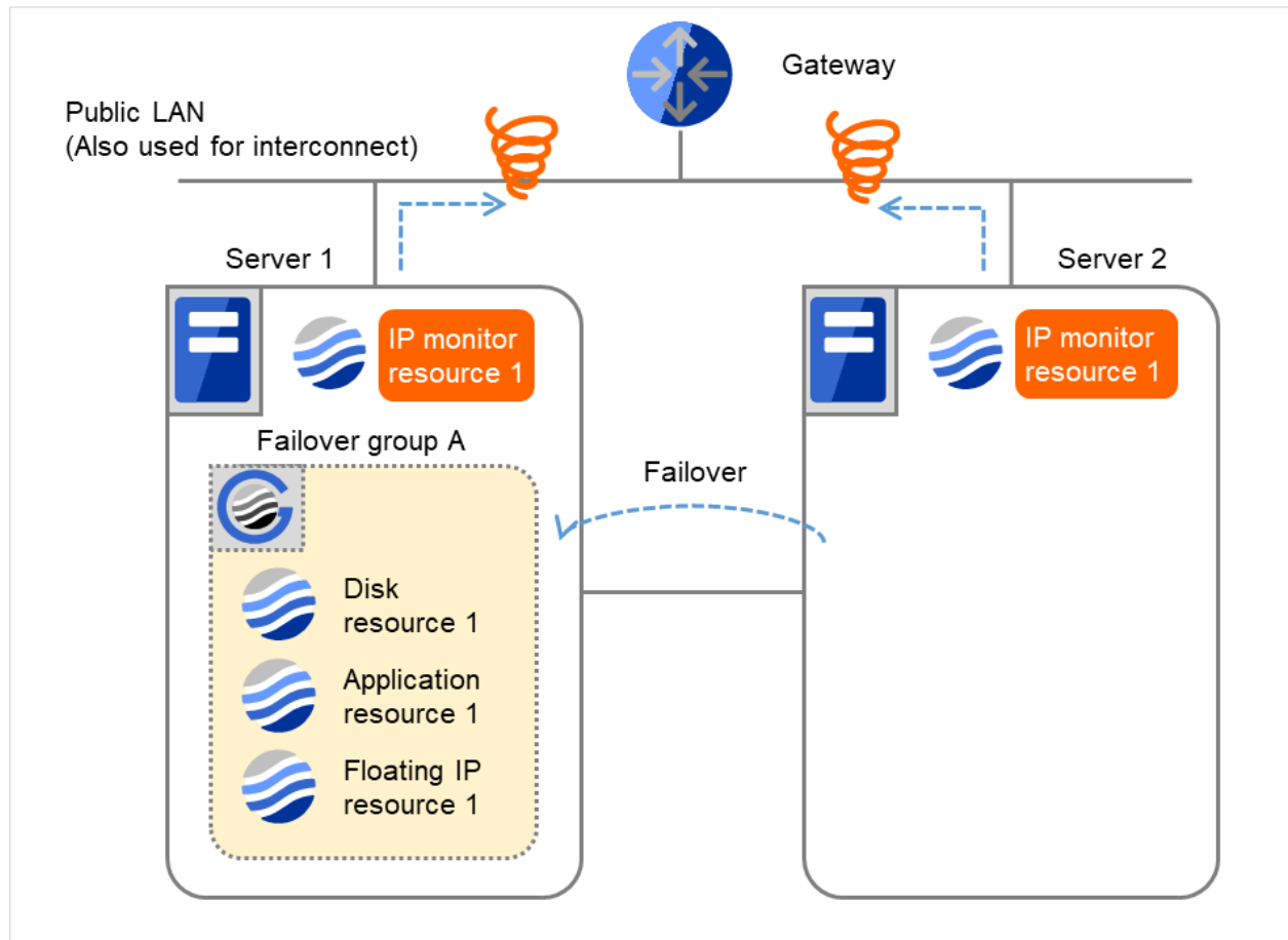
図 4.25 IP 監視リソース異常検出の流れ（両サーバで異常検出）(12)
