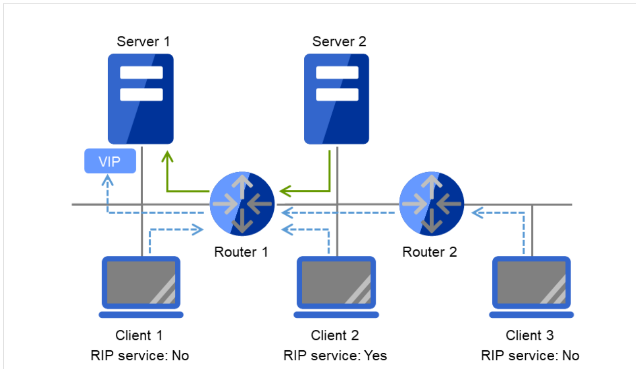
図 3.104 仮想 IP を使用した構成 (1)
