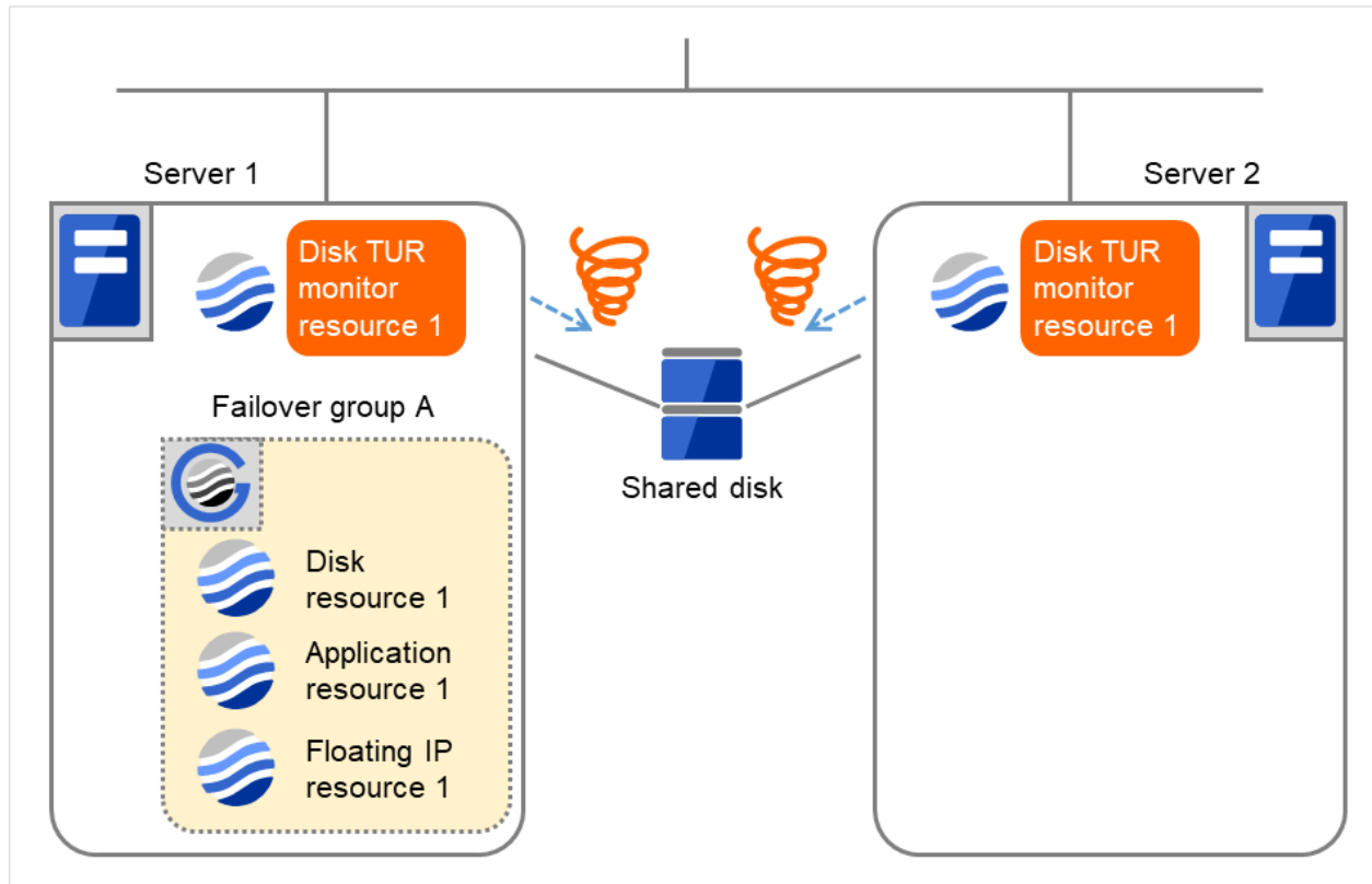
図 4.35 ディスク TUR 監視リソース異常検出の流れ (2)
