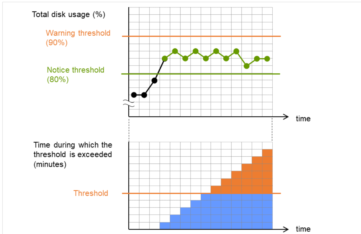
図 4.73 ディスク使用率において、通知レベル上限値以上の状態が一定時間続いた場合（異常検出する）
