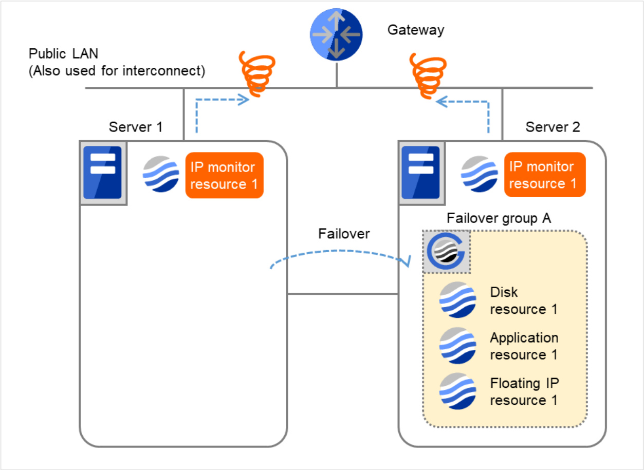
図 4.20 IP 監視リソース異常検出の流れ（両サーバで異常検出） (7)
