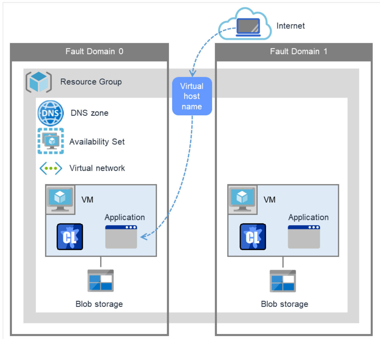
図 3.115 Azure DNS リソースを使用する構成
