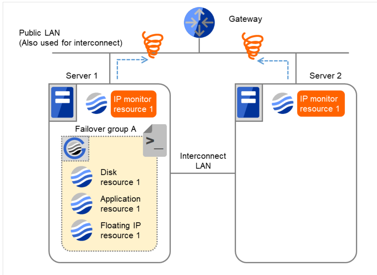
図 4.32 IP 監視リソース異常検出の流れ（監視異常からの復帰・正常）(5)
