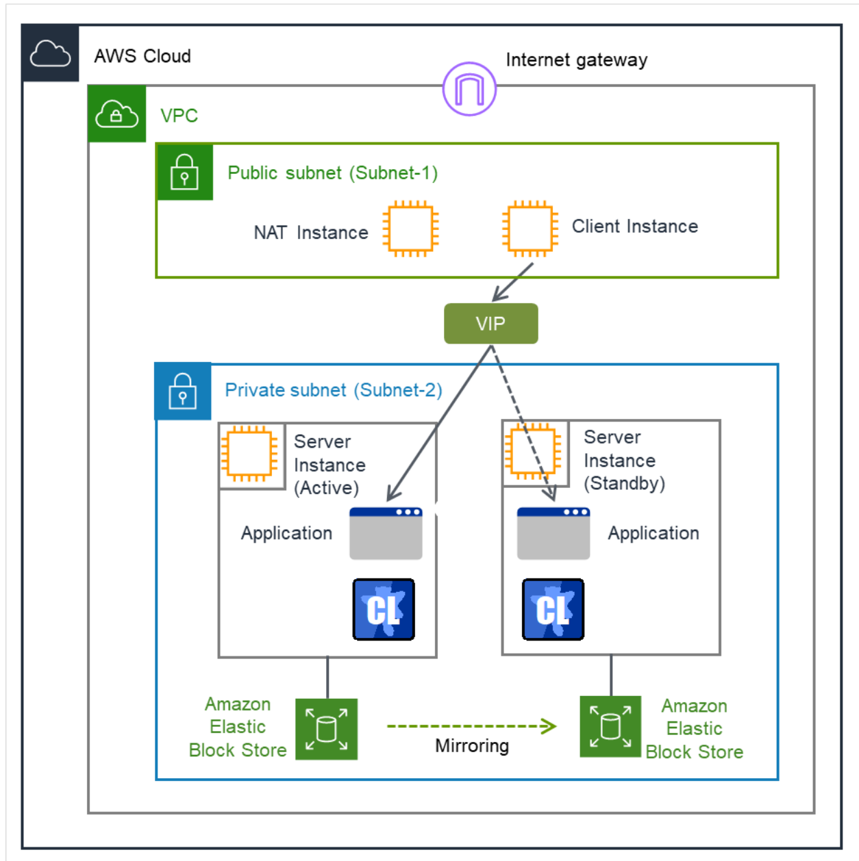
図 3.110 AWS 仮想 IP リソースを使用する構成
