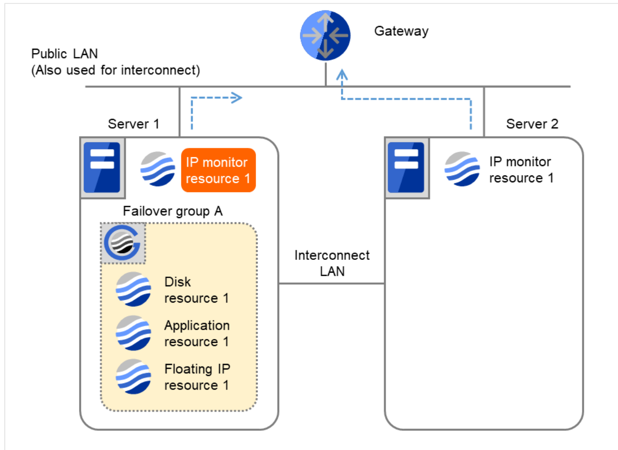
図 4.9 IP 監視リソース異常検出の流れ（片サーバのみ異常検出）(3)
