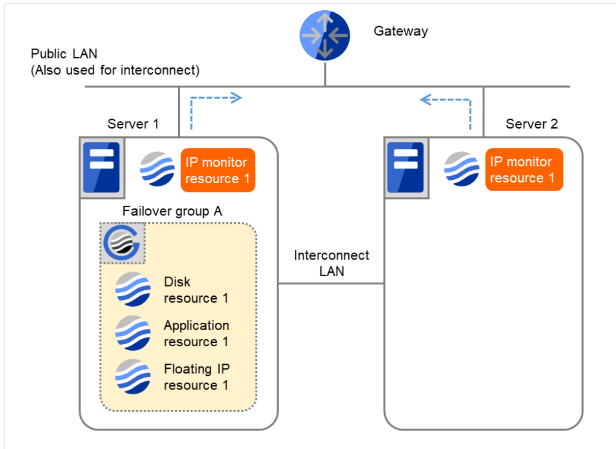
図 4.26 IP 監視リソース異常検出の流れ（両サーバで異常検出） (13)
