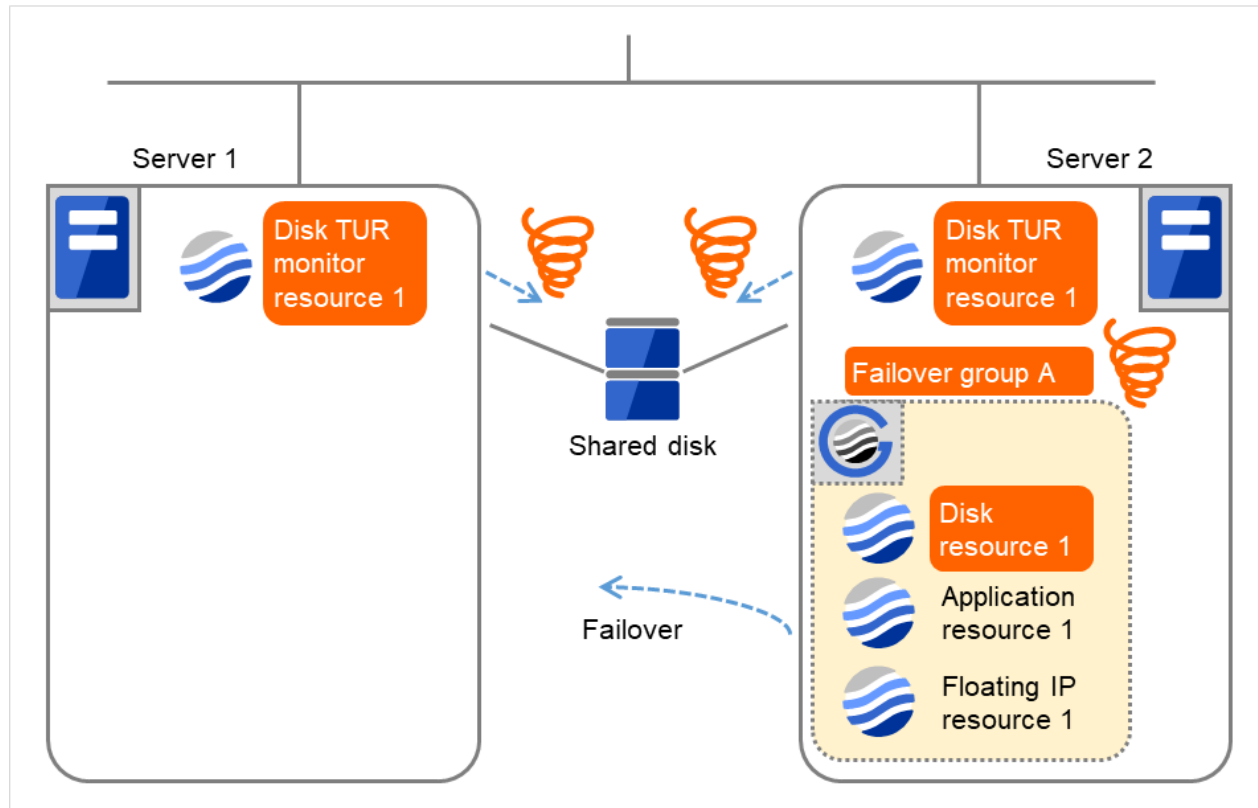
図 4.43 ディスク TUR 監視リソース異常検出の流れ (10)
