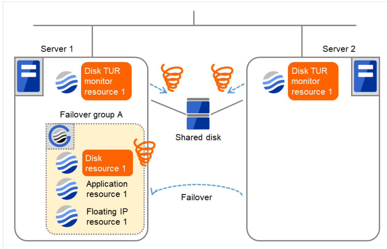
図 4.39 ディスク TUR 監視リソース異常検出の流れ (6)
