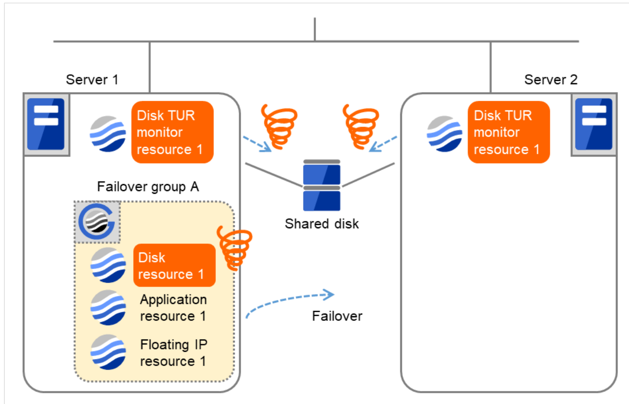
図 4.40 ディスク TUR 監視リソース異常検出の流れ (7)"
