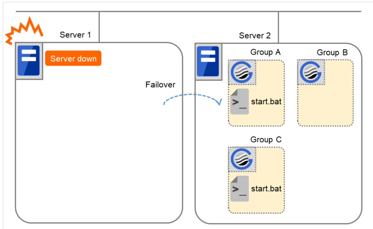
図 3.60 状態とスクリプト実行（サーバダウンによるフェイルオーバー）
