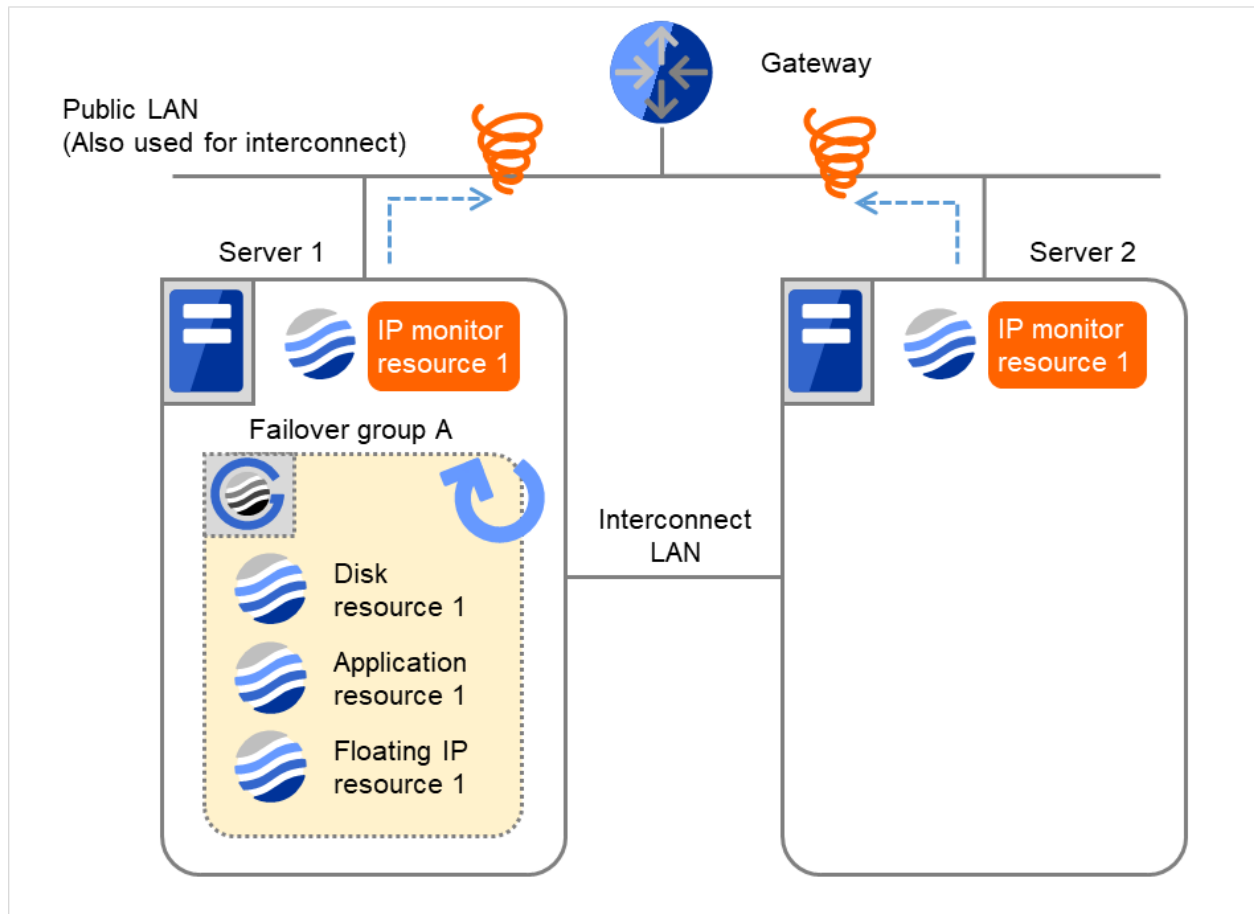
図 4.18 IP 監視リソース異常検出の流れ（両サーバで異常検出）(5)
