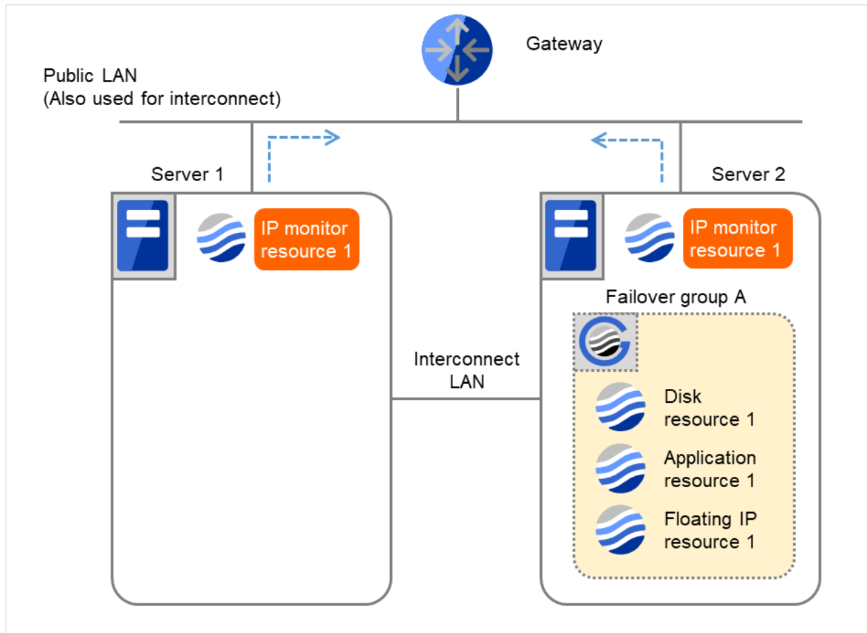
図 4.21 IP 監視リソース異常検出の流れ（両サーバで異常検出）(8)
