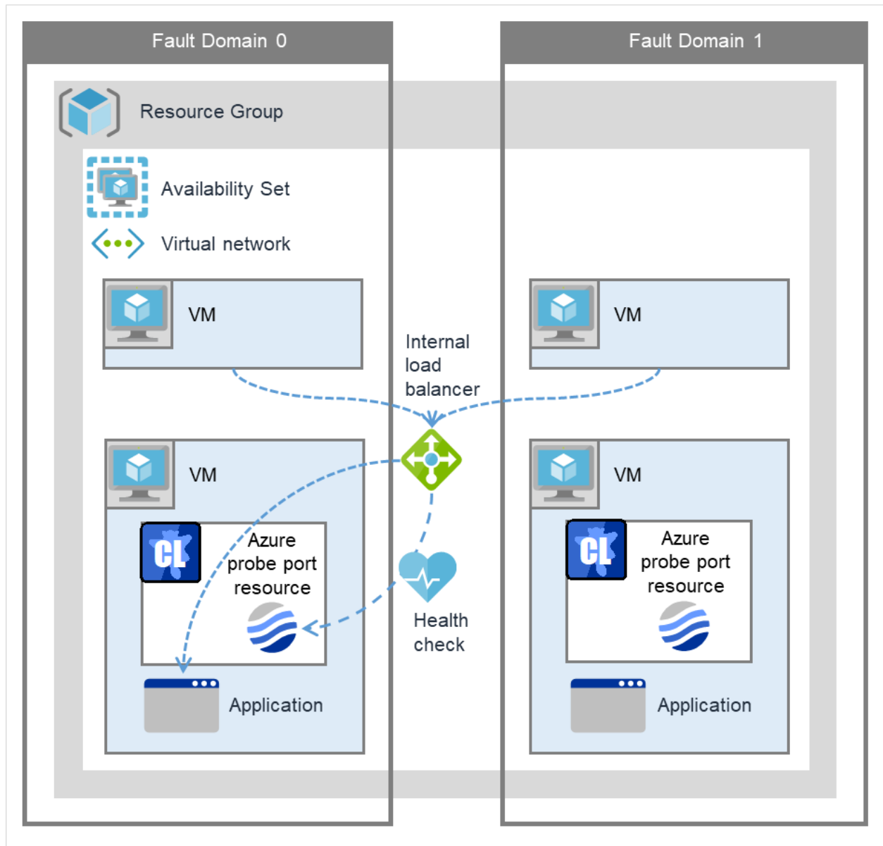
図 3.114 Azure プローブポートリソースを使用する構成 (内部負荷分散)
