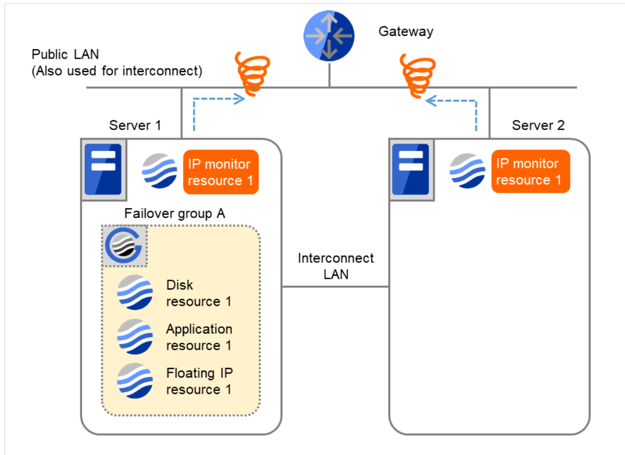
図 4.27 IP 監視リソース異常検出の流れ（両サーバで異常検出）(14)
