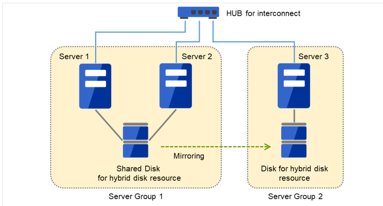
図 3.40 サーバグループ
