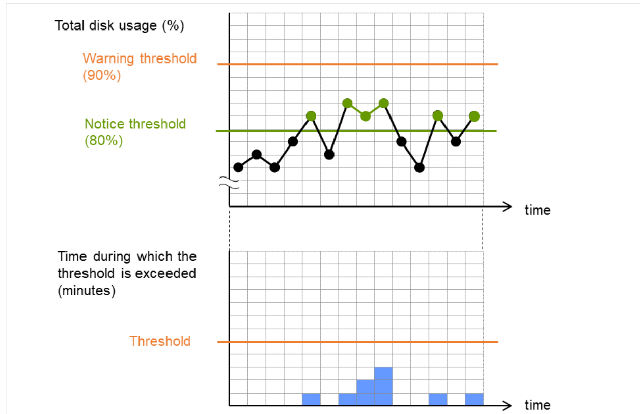
図 4.74 ディスク使用率において、通知レベル上限値以上の状態が一定時間続かない場合（異常検出しない）
