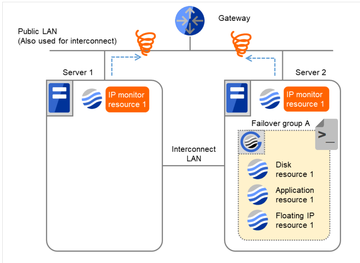
図 4.22 IP 監視リソース異常検出の流れ（両サーバで異常検出） (9)
