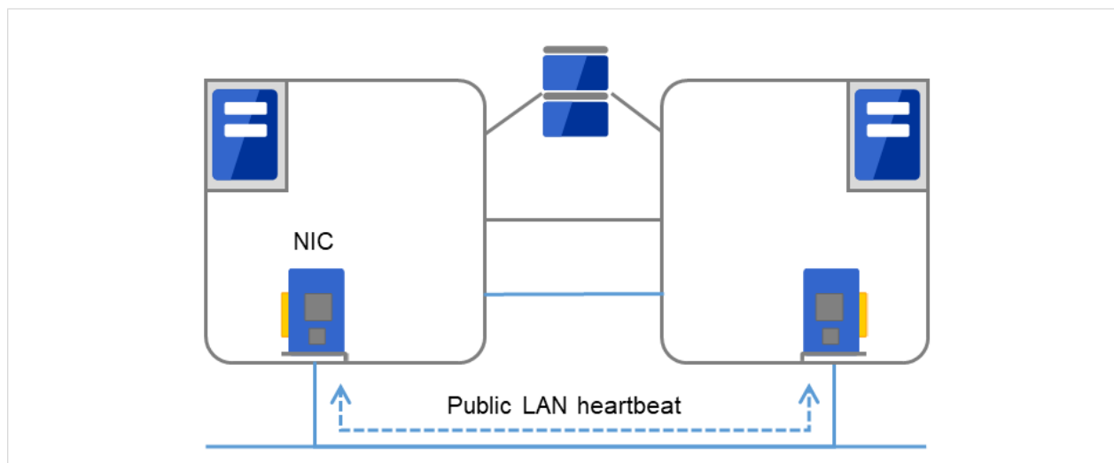
図 5.2 カーネルモード LAN ハートビート（セカンダリインタコネクト）
