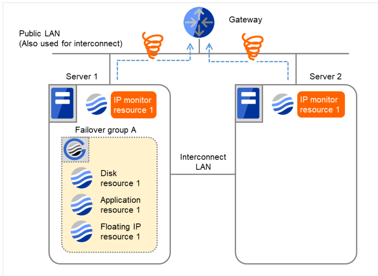
図 4.15 IP 監視リソース異常検出の流れ（両サーバで異常検出）(2)
