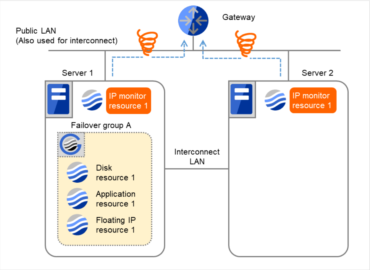
図 4.28 IP 監視リソース異常検出の流れ（監視異常からの復帰・正常）（1）
