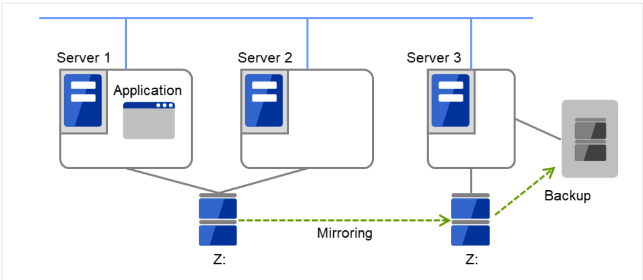
図 9.7 ハイブリッド構成でのバックアップ
