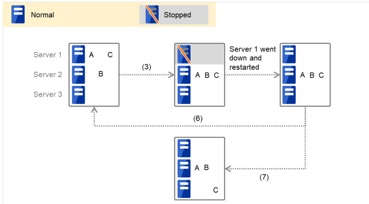
図 3.74 クラスタ状態遷移の例（サーバダウンによるフェイルオーバー）
