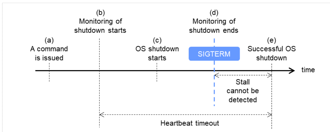
図 8.3 シャットダウン成功時 (監視方法が ipmi, SIGTERM が有効の場合)
