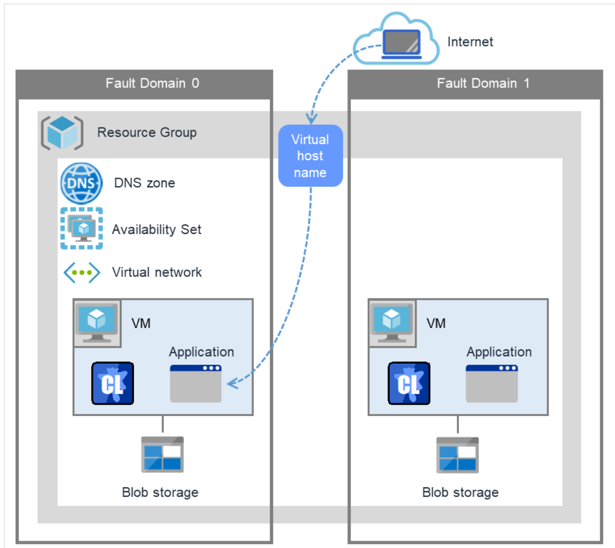
図 3.137 Azure DNS リソースを使用する構成
