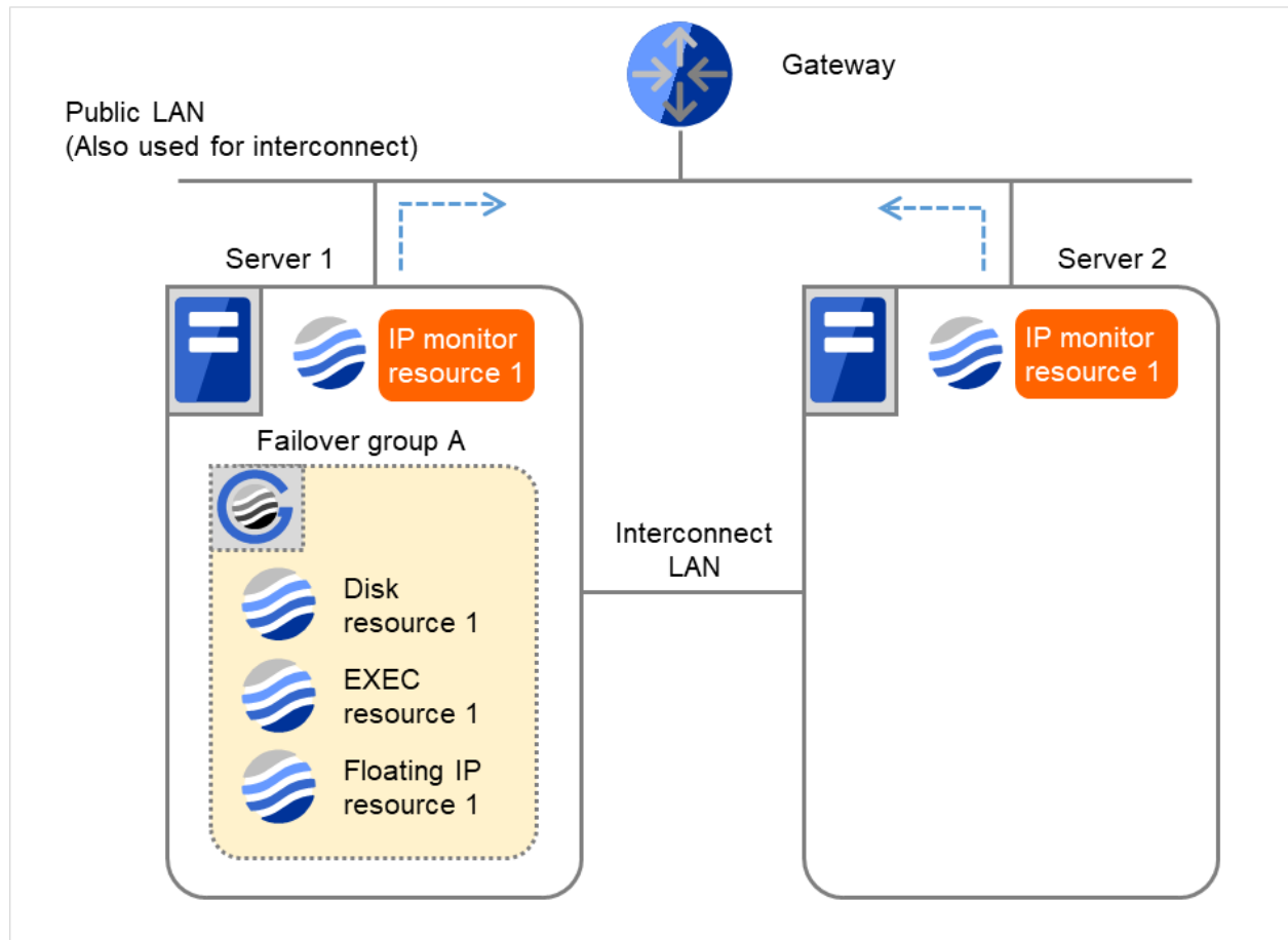
図 4.35 IP モニタリソース異常検出の流れ（監視異常からの復帰・正常）（4）
