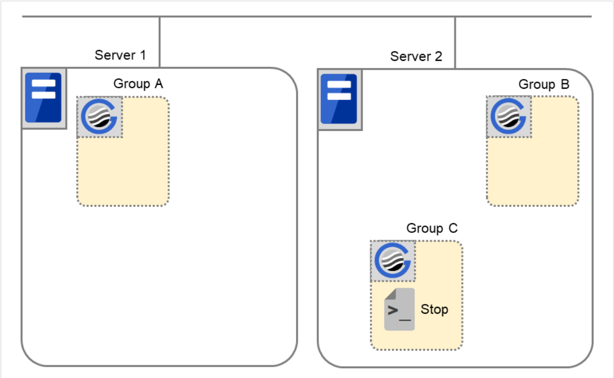
図 3.49 状態とスクリプト実行 (Group C の停止)
