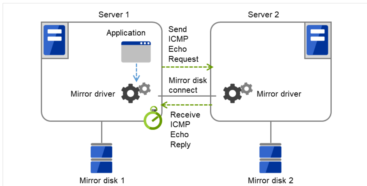
図 3.94 ICMP Echo Reply 受信タイムアウト
