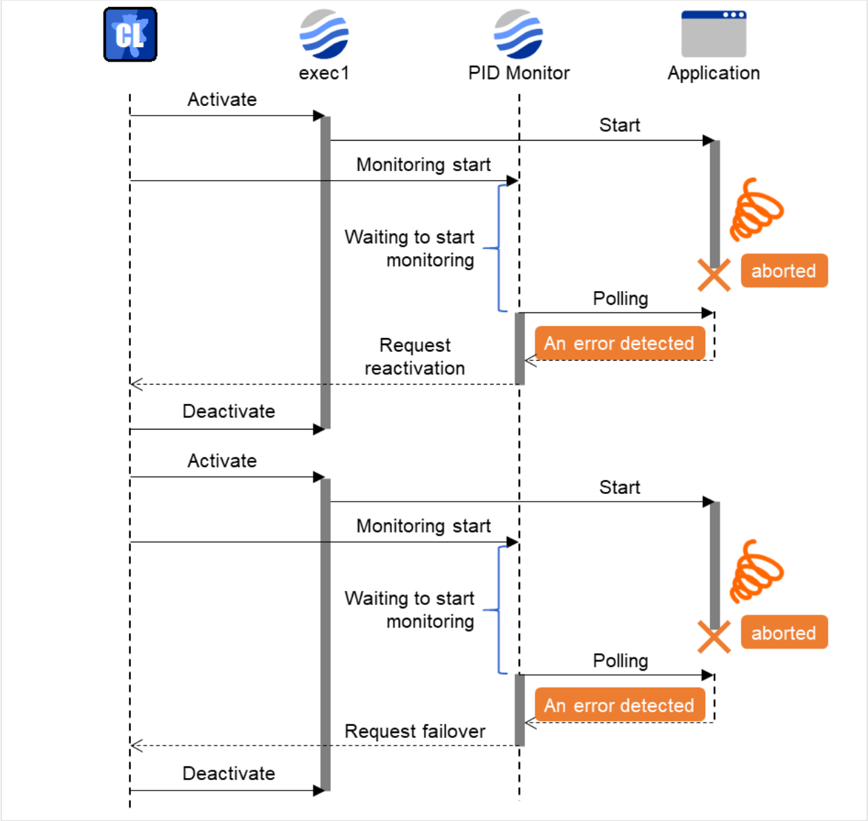
図 4.54 モニタリソースの監視開始待ち（監視開始待ち時間 60 秒）
