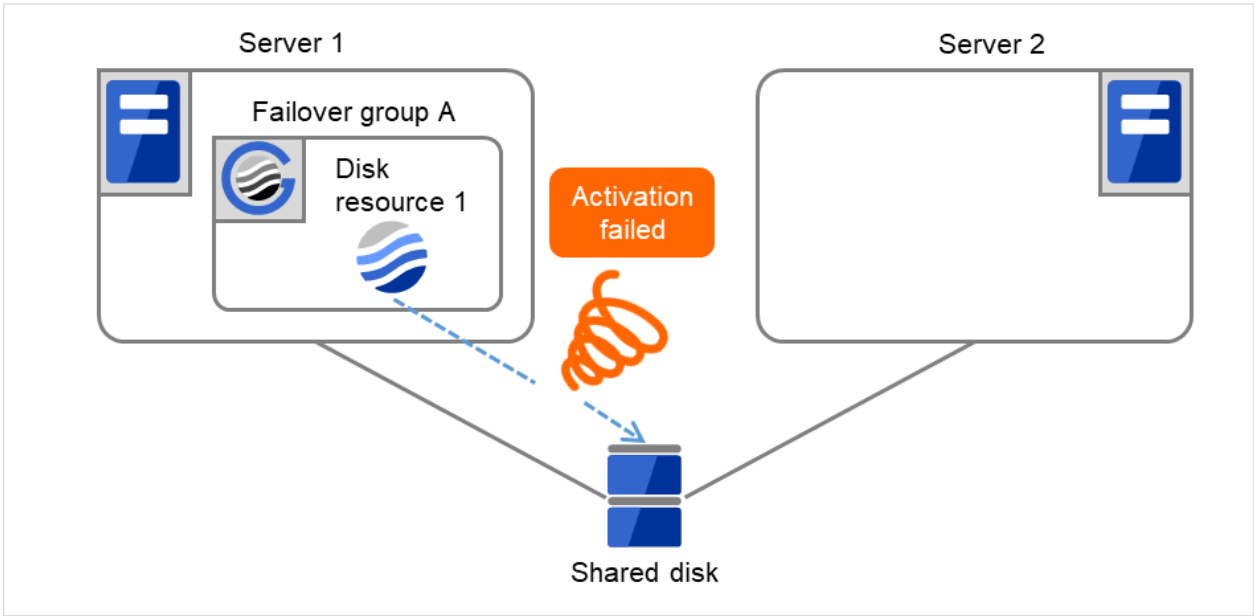
図 3.20 再起動回数制限時の処理 (8)
