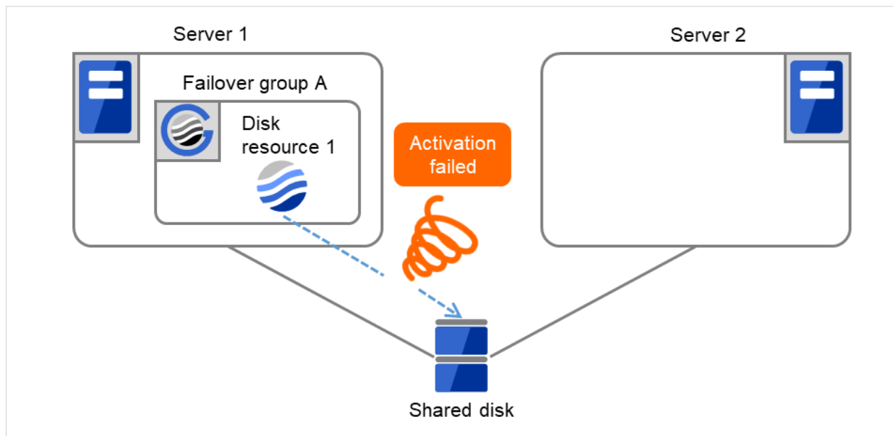
図 3.6 グループリソース活性異常検出時の流れ (2)
