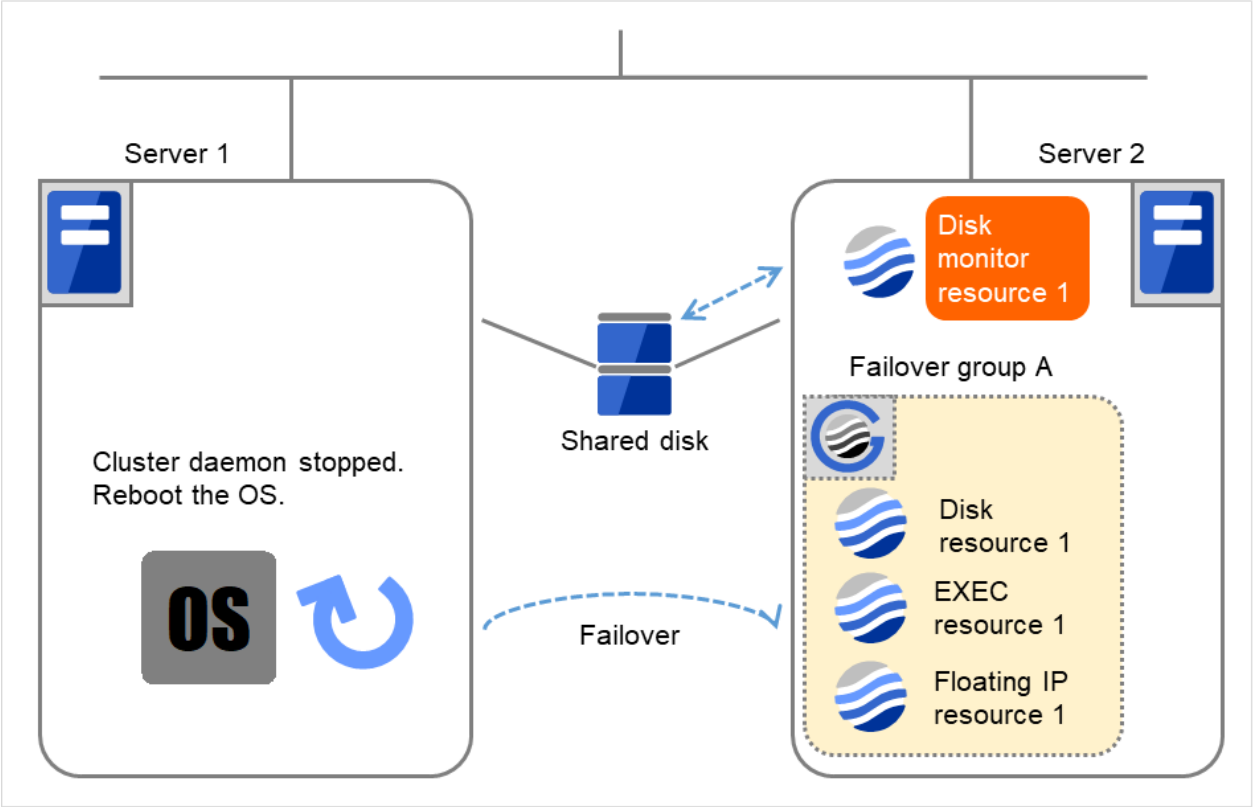
図 4.57 再起動回数制限 (3)
