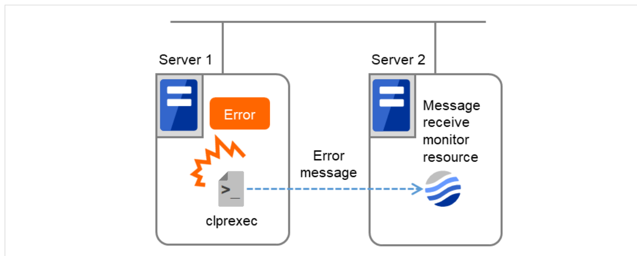
図 4.70 外部連携モニタリソースを使用する構成
