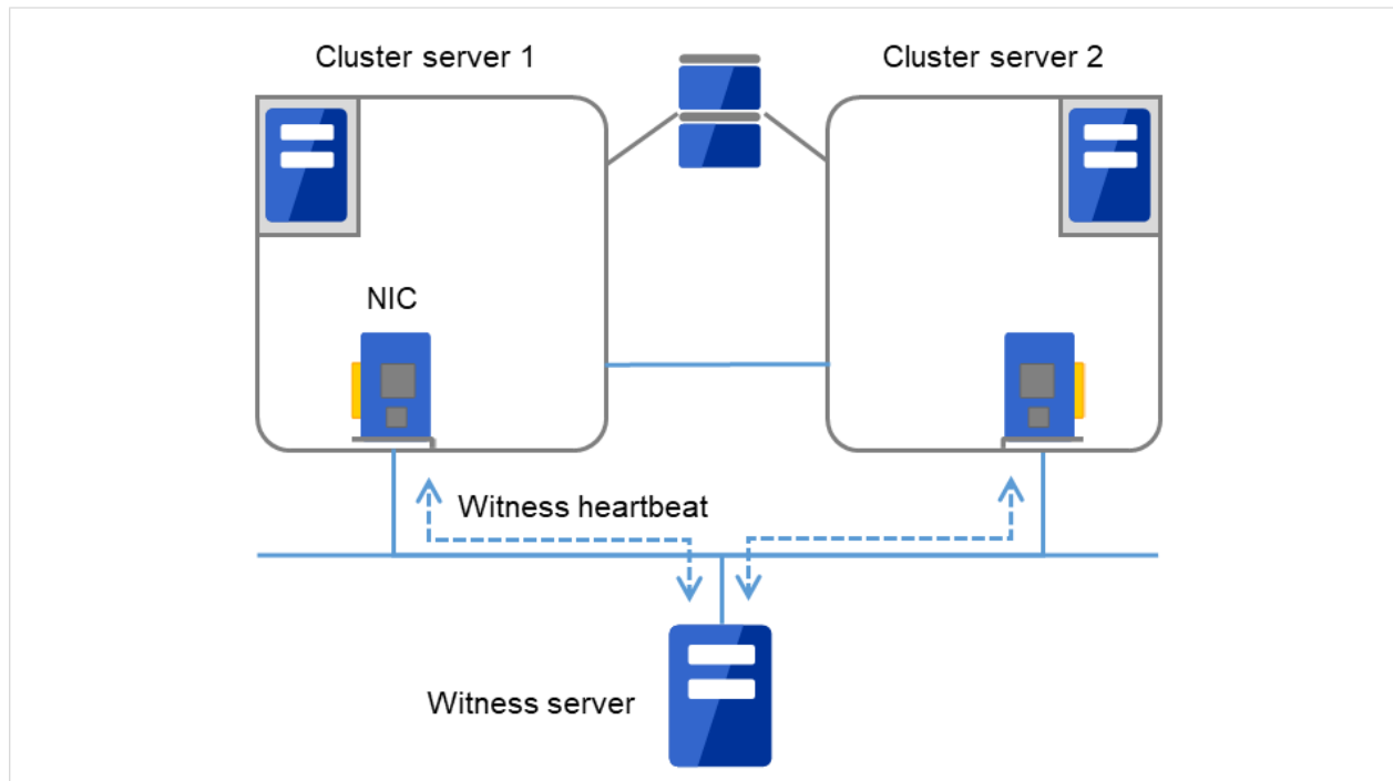
図 8.9 Witness サーバサービス
