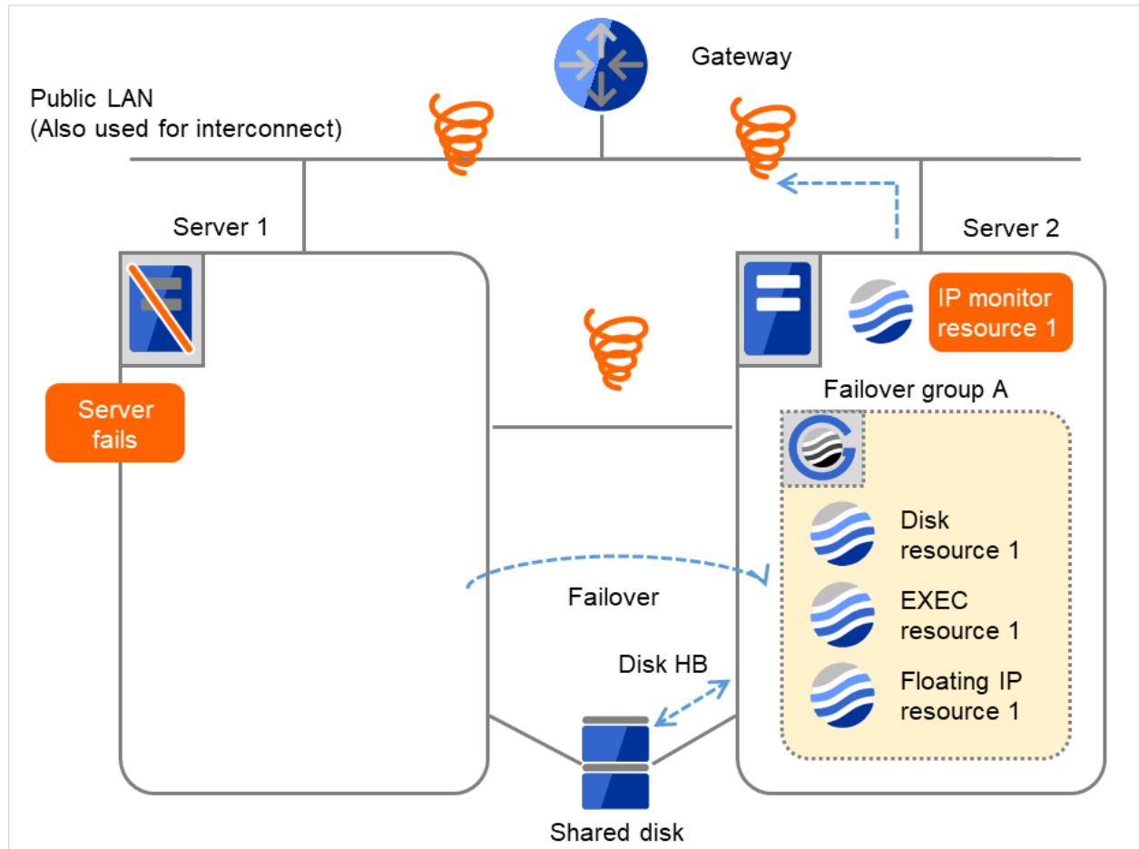
図 4.30 IP モニタリソース異常検出の流れ（全インタコネクト LAN が断線） (3)
