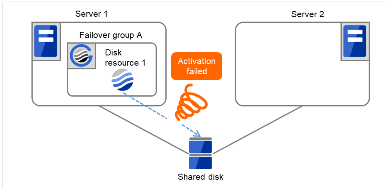
図 3.14 再起動回数制限時の処理 (2)
