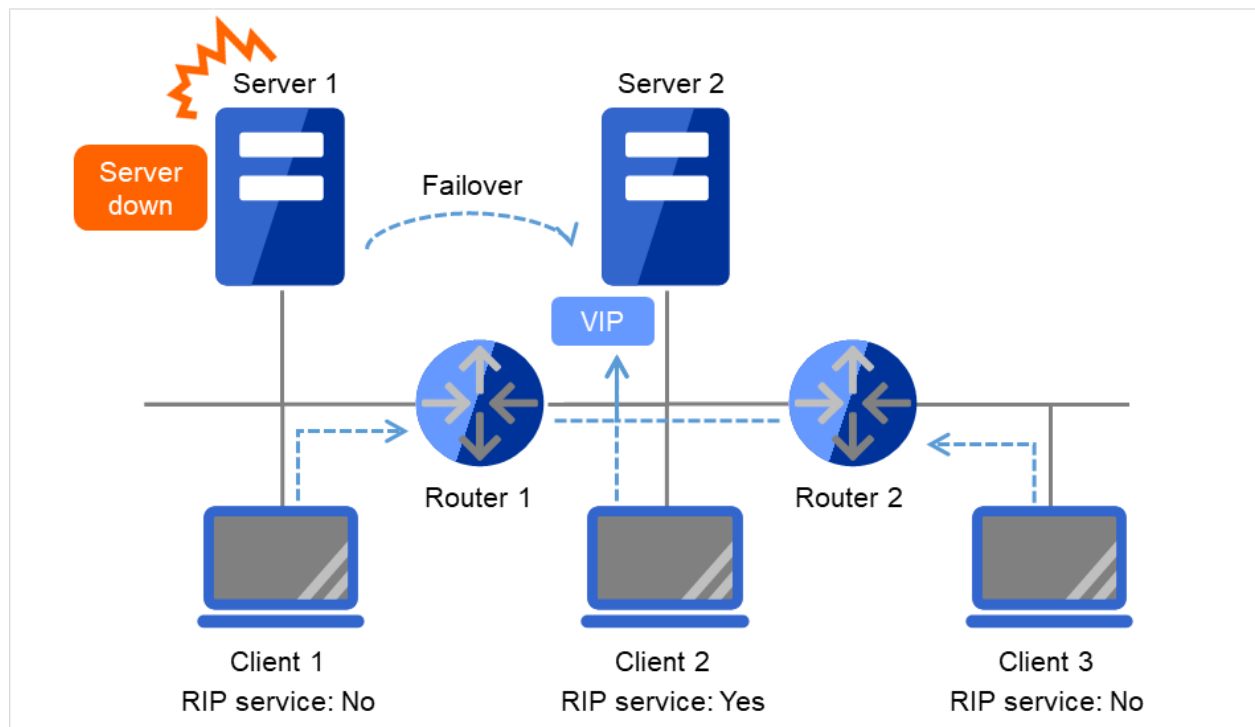
図 3.81 仮想 IP を使用した構成 (2)
