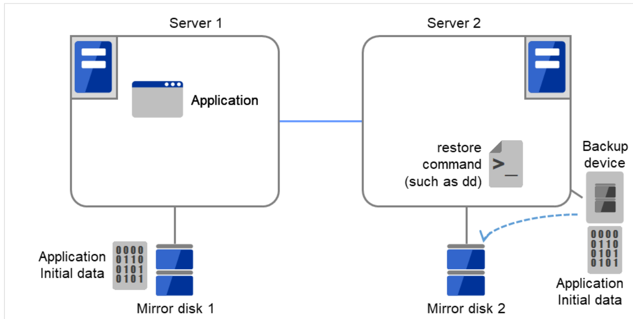
図 3.107 ミラーディスク構築例 (バックアップ装置使用) (3)
