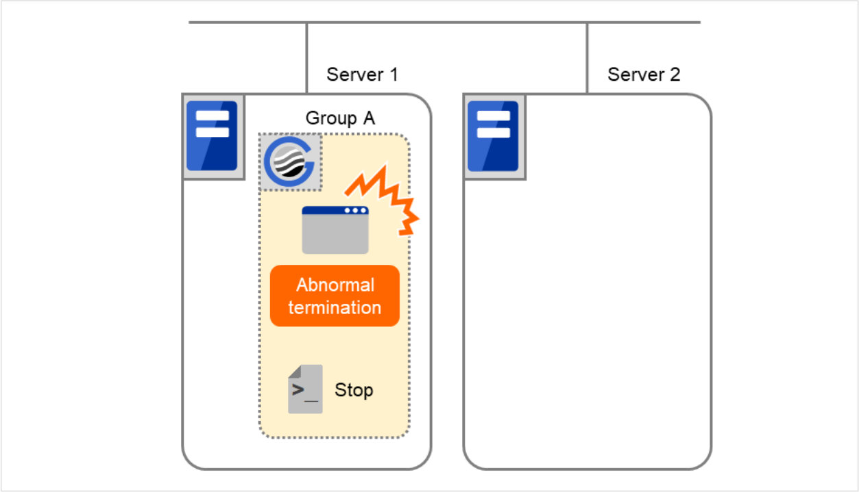
図 3.58 状態とスクリプト実行（Group A のフェイルオーバー）(1)
