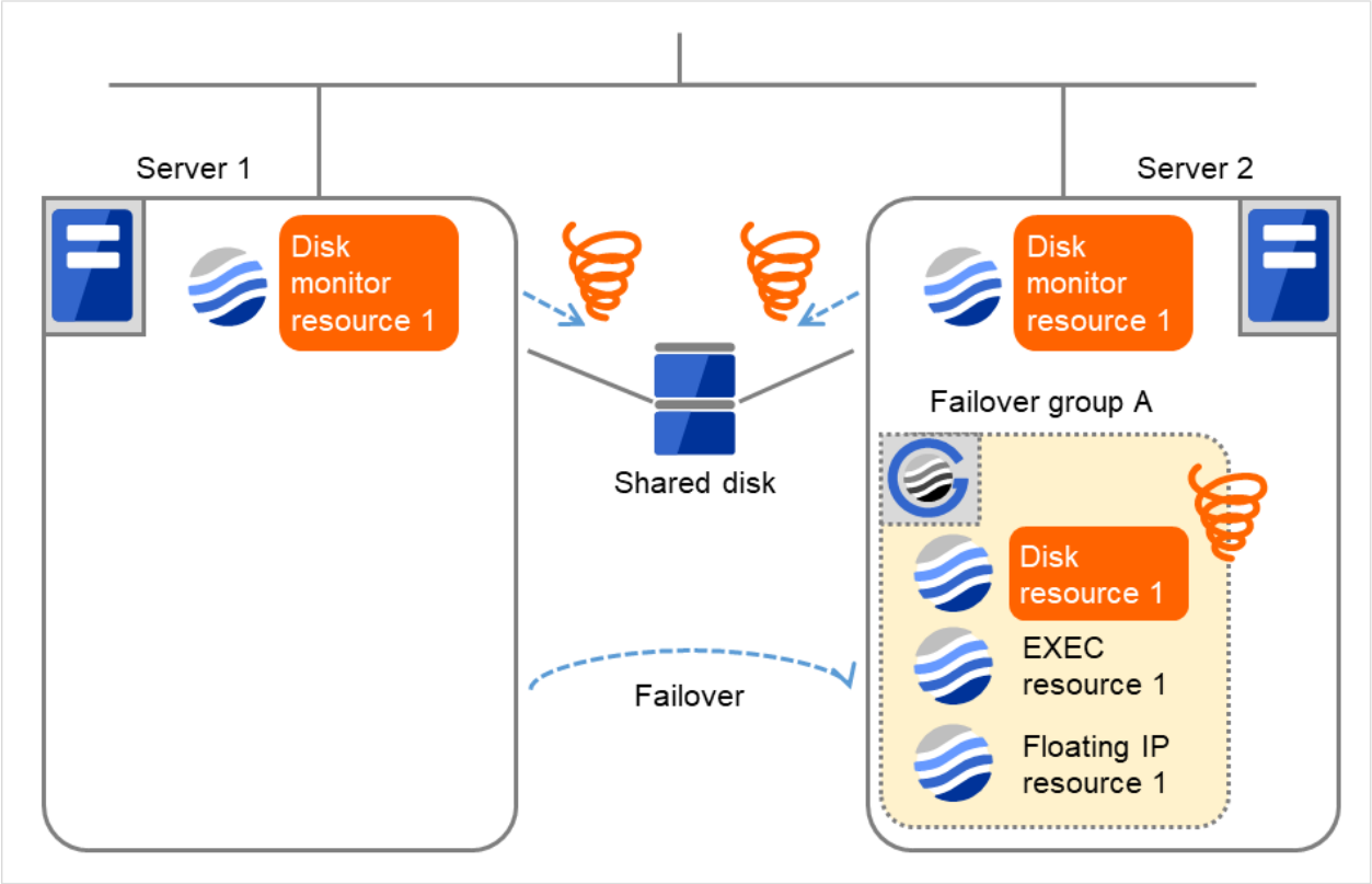
図 4.45 ディスクモニタリソース異常検出の流れ (8)
