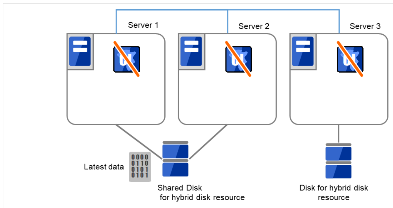
図 10.6 ハイブリッドディスク上のデータ保存 (1)
