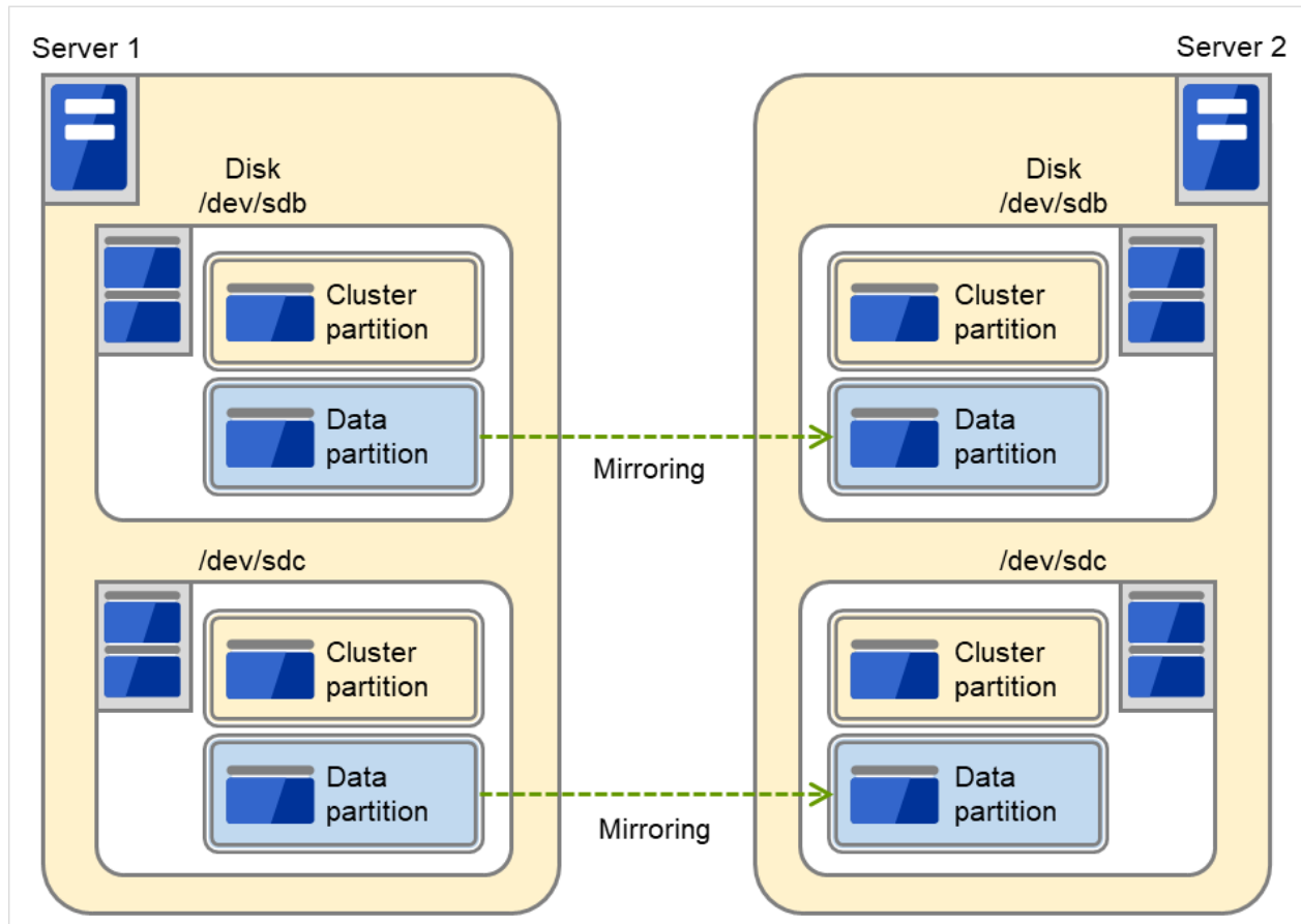
図 3.86 各ディスクをミラーパーティションにする場合
