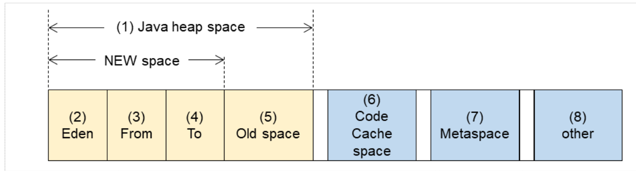
図 4.77 Java VM メモリ空間 (Oracle Java 8, Oracle Java 9/Oracle Java 11)
