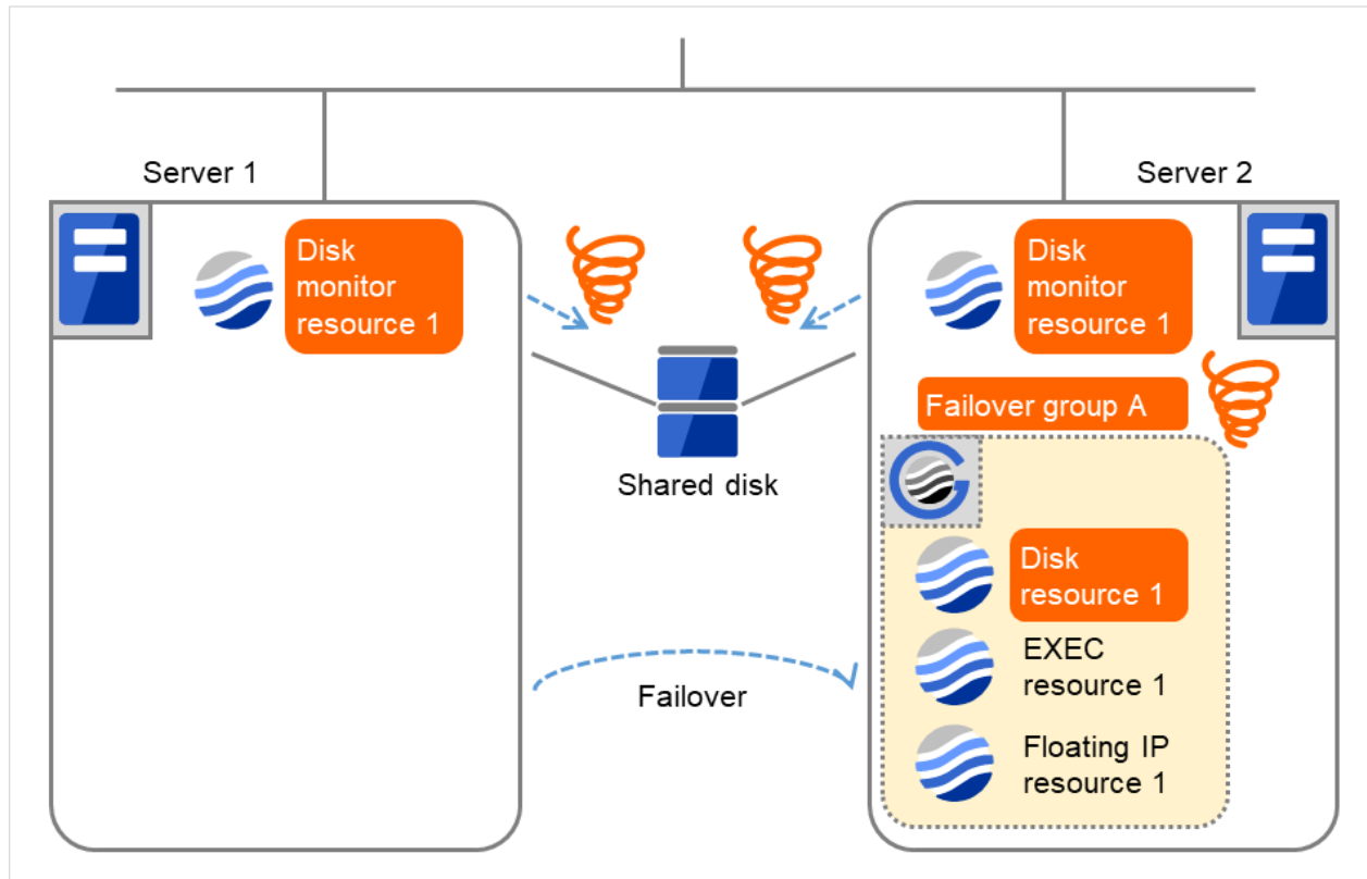
図 4.46 ディスクモニタリソース異常検出の流れ (9)
