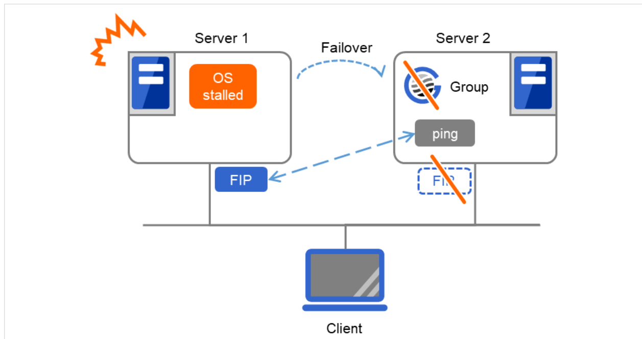
図 3.77 ping タイムアウトの設定が 0 以外かつ FIP 強制活性が OFF の場合
