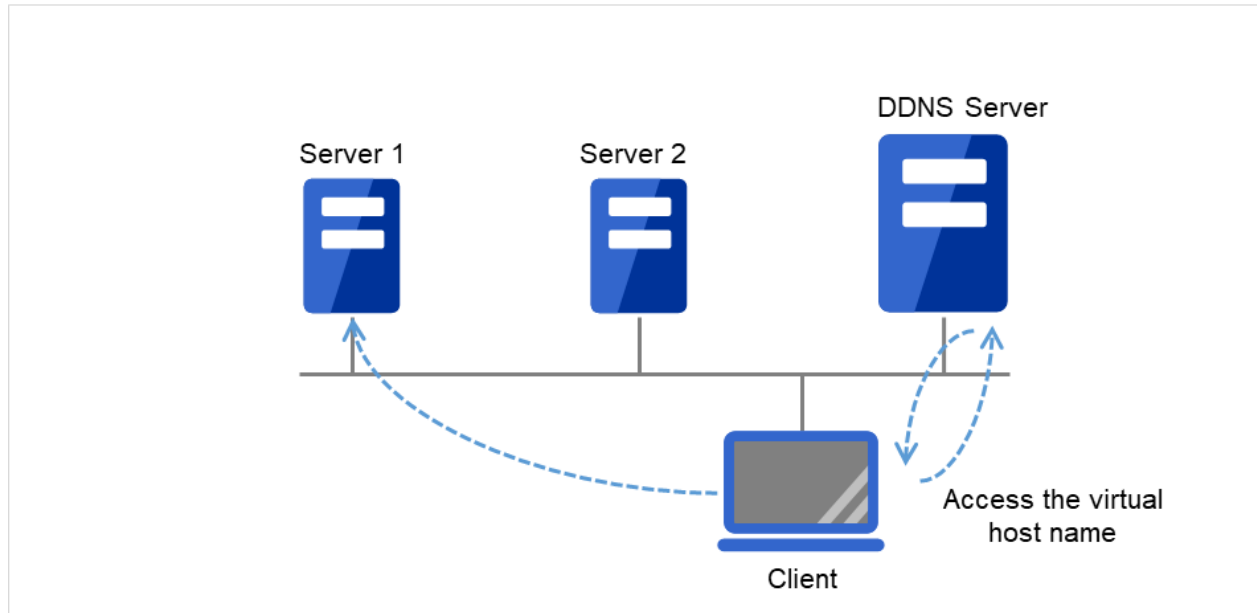
図 3.127 ダイナミック DNS サーバを使用する構成 (2)
