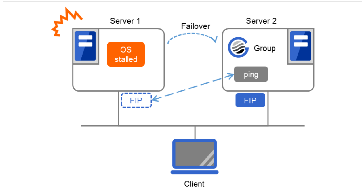
図 3.79 ping タイムアウトの設定が 0 以外かつ FIP 強制活性が ON の場合
