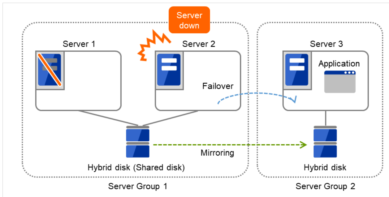
図 3.111 ハイブリッド構成 (3) (Server 2 ダウン)
