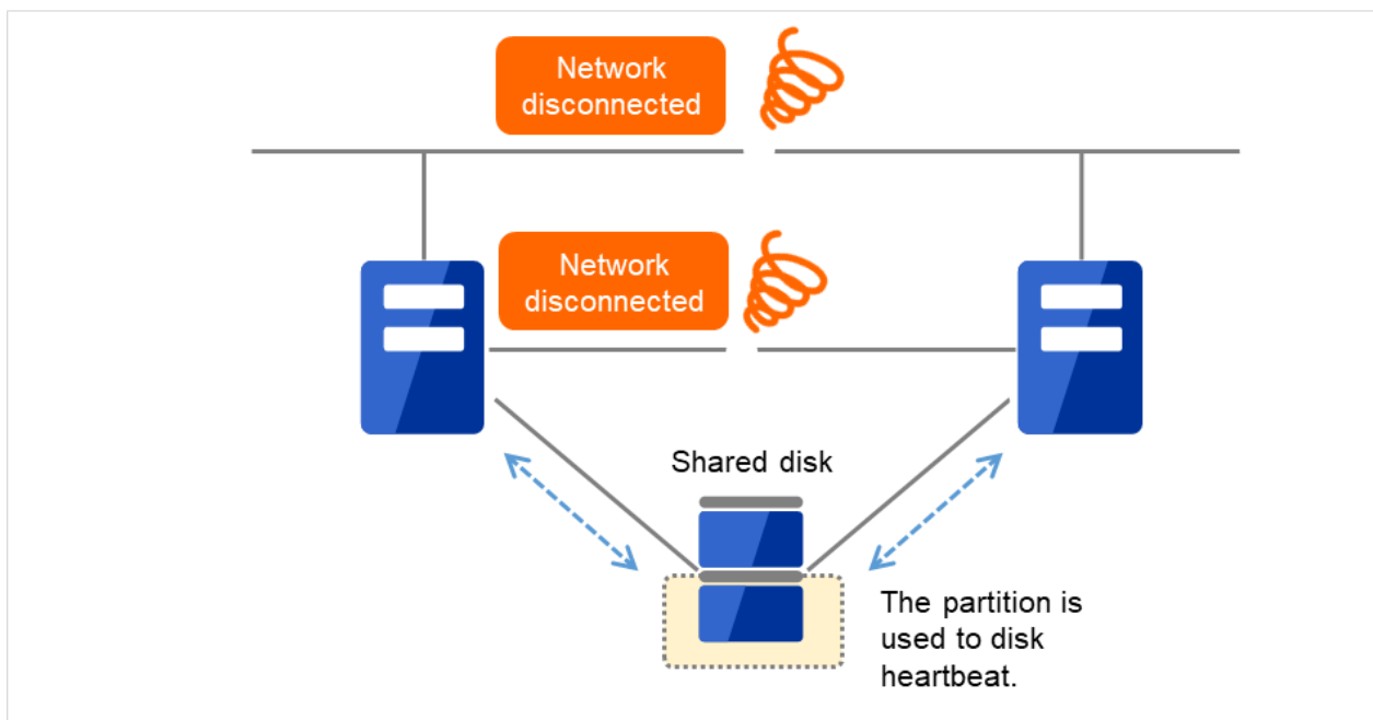
図 5.7 ディスクハートビートリソース (3)
