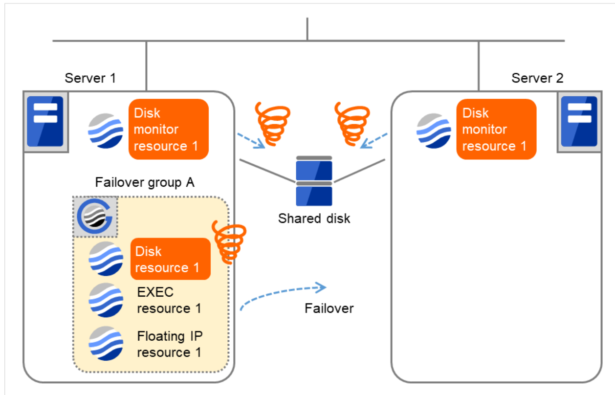
図 4.44 ディスクモニタリソース異常検出の流れ (7)
