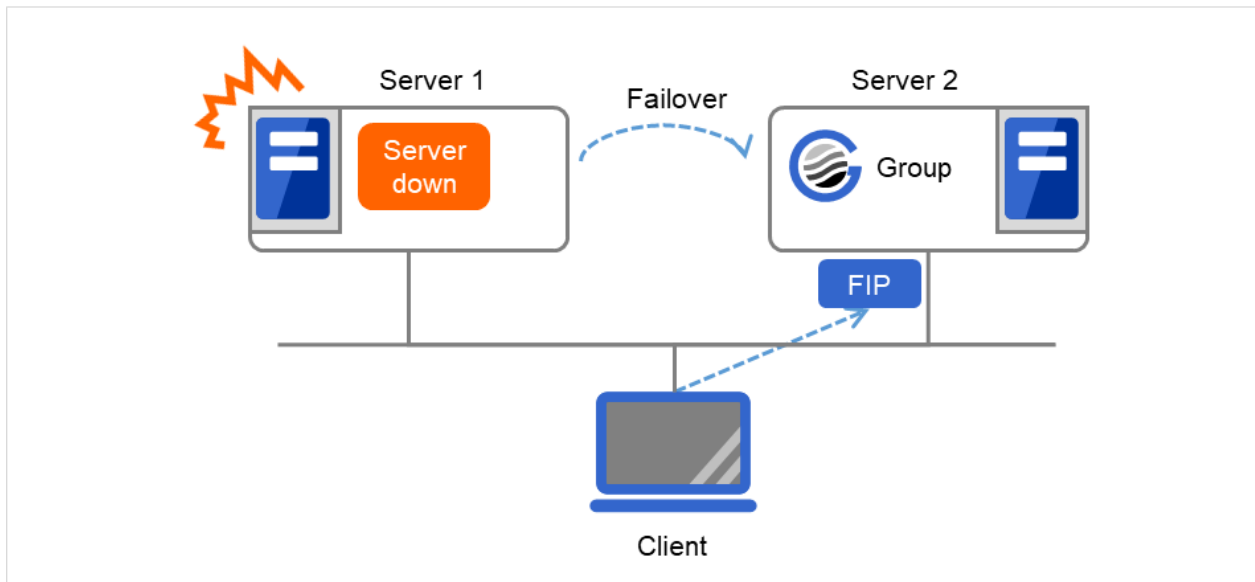
図 3.73 フローティング IP によるアクセス (2)
