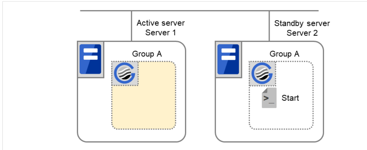
図 3.62 状態とスクリプト実行 (Group A の通常起動) (2)
