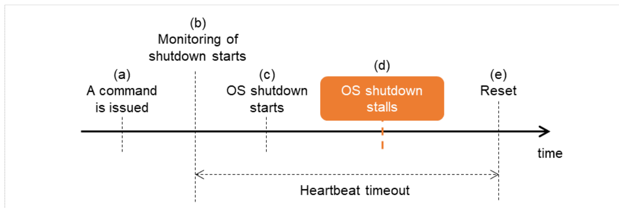
図 8.5 シャットダウンストール検出時
