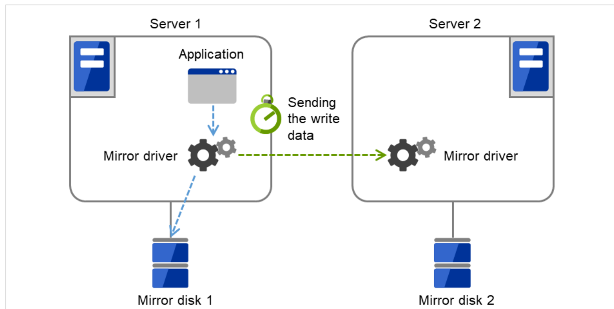
図 3.88 送信タイムアウト（write データ）
