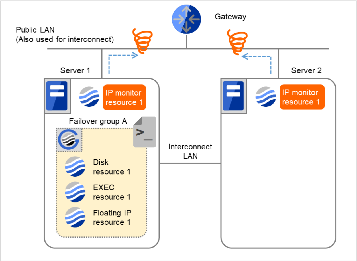
図 4.36 IP モニタリソース異常検出の流れ（監視異常からの復帰・正常）（5）
