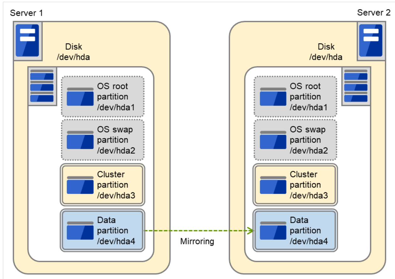
図 3.85 ディスクの空き領域をミラーパーティションにする場合
