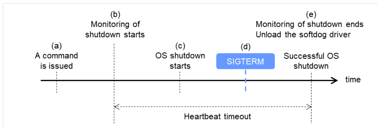
図 8.2 シャットダウン成功時（監視方法が softdog、SIGTERM が有効でない場合）
