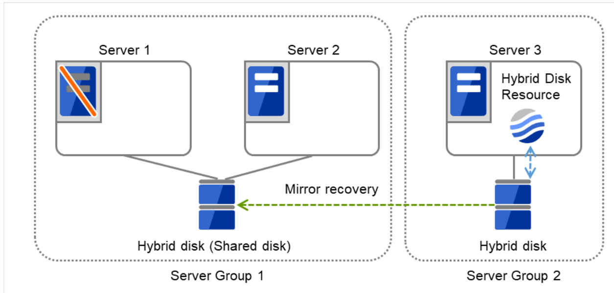
図 3.119 ハイブリッド構成 (4) (相手サーバグループ内でリソース活性, Server 1 ダウン後のミラー復帰)
