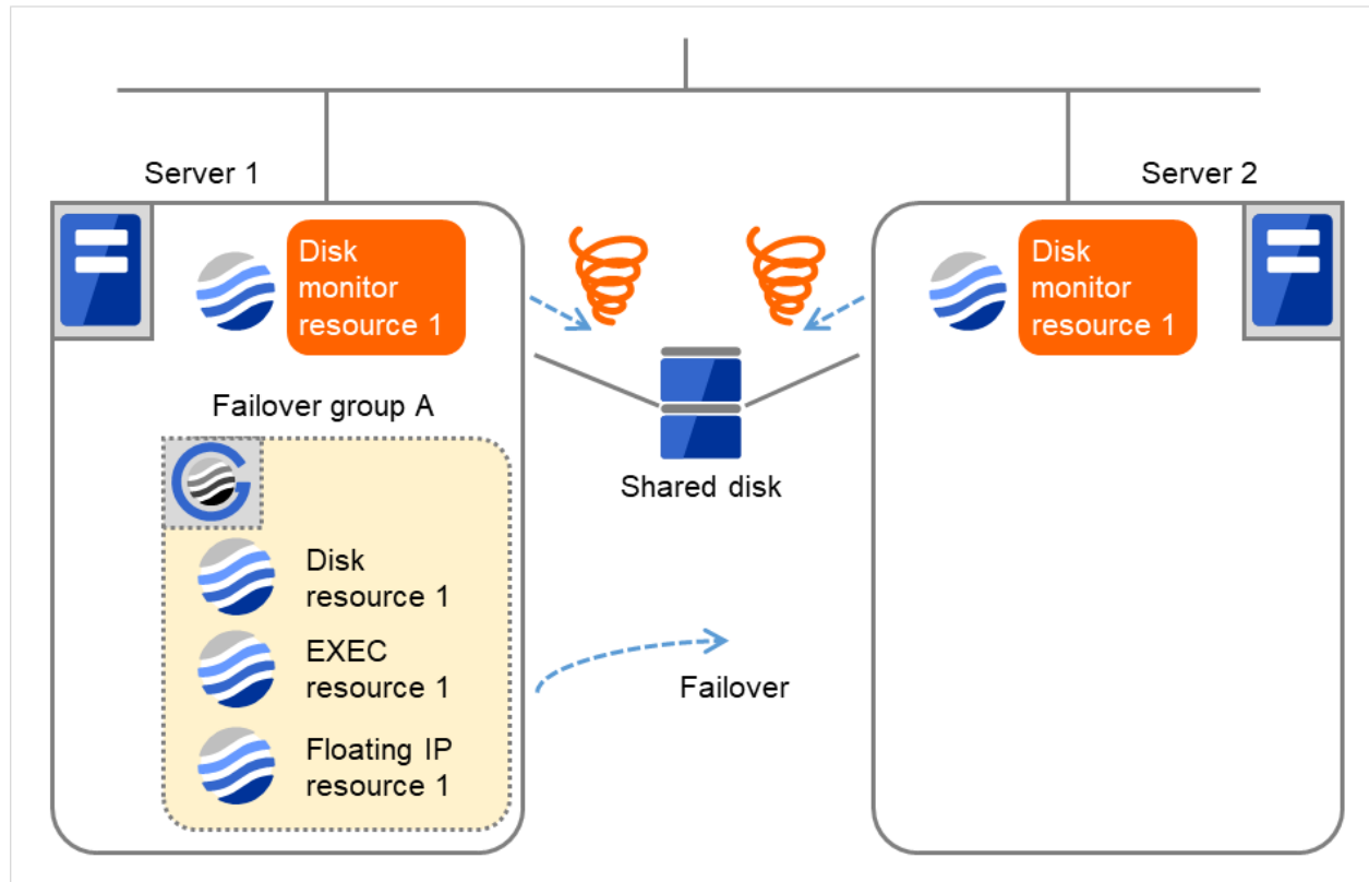
図 4.40 ディスクモニタリソース異常検出の流れ (3)
