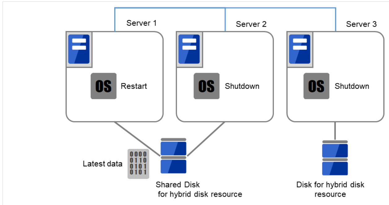
図 10.7 ハイブリッドディスク上のデータ保存 (2)
