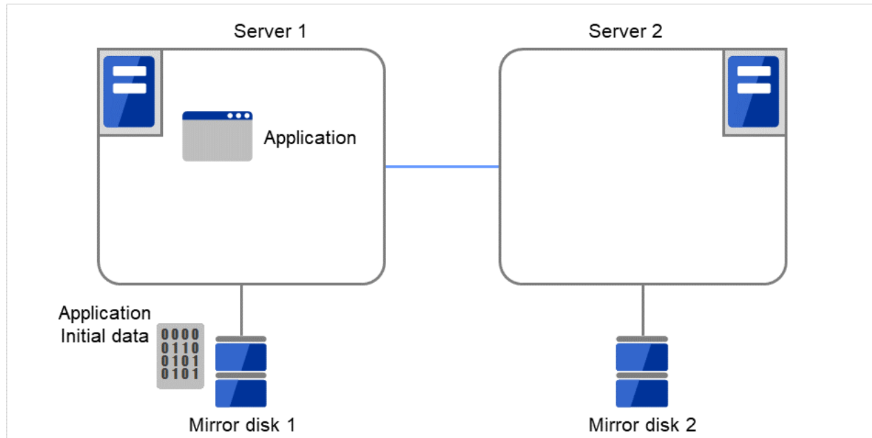
図 3.105 ミラーディスク構築例（バックアップ装置使用）(1)
