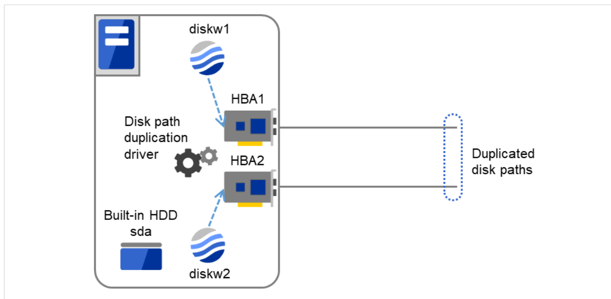
図 4.69 Disk パス二重化ドライバの使用例
