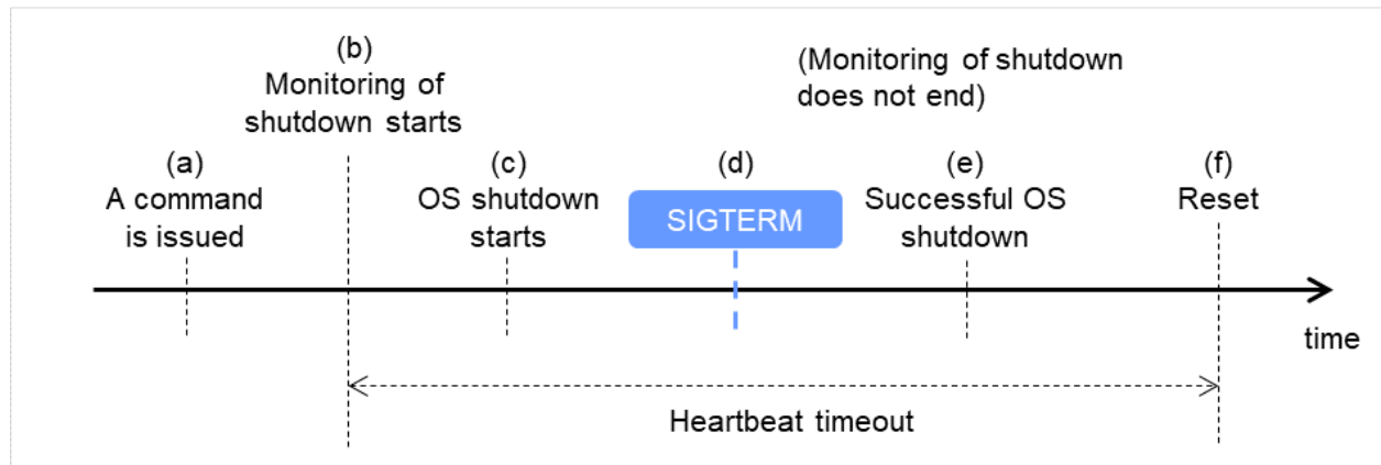
図 8.4 シャットダウン成功時（監視方法が ipmi、SIGTERM が有効でない場合）
