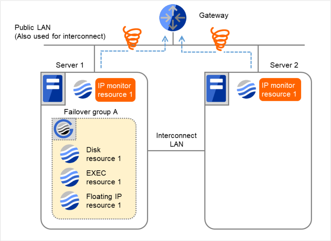
図 4.32 IP モニタリソース異常検出の流れ（監視異常からの復帰・正常）（1）
