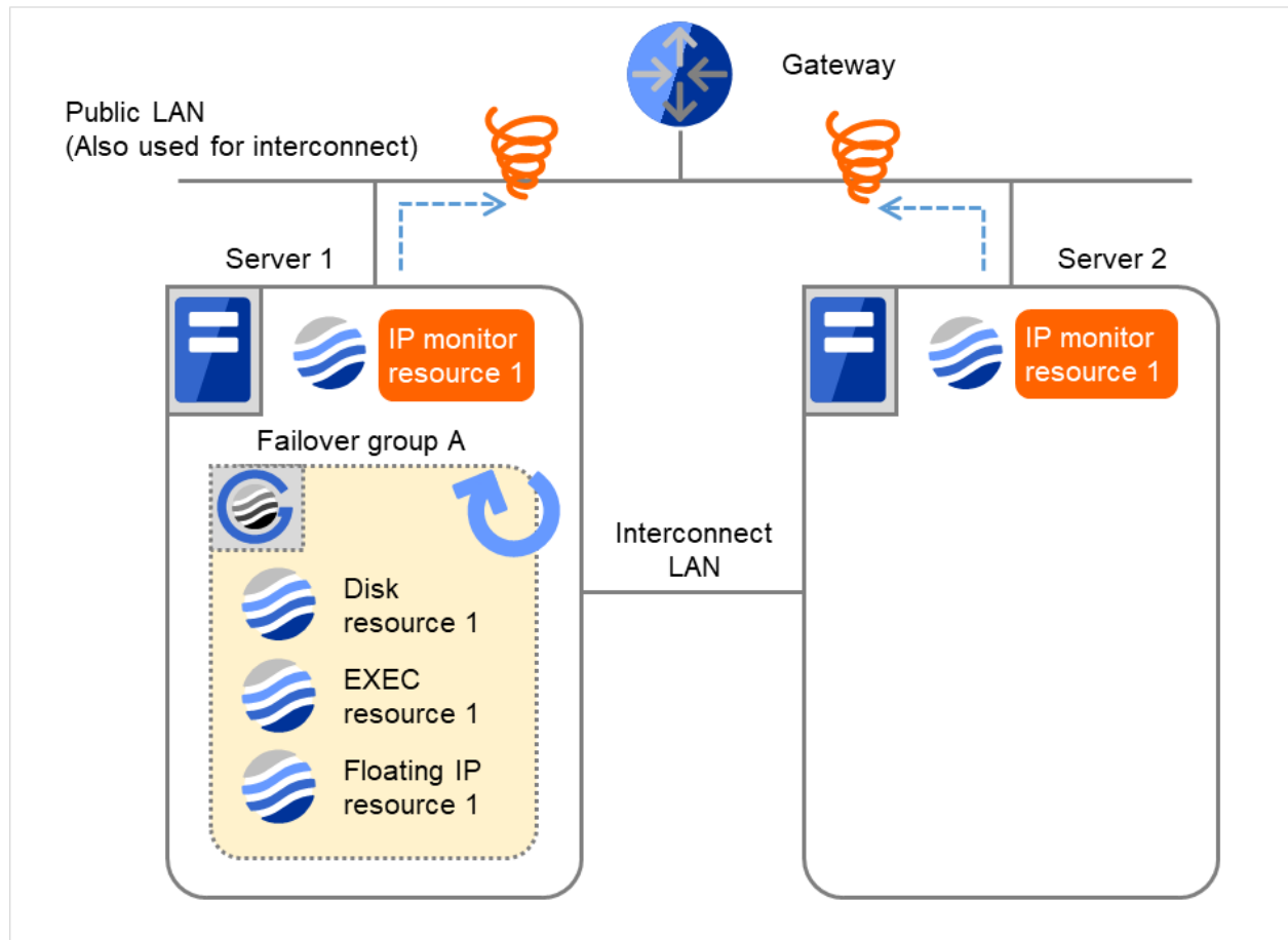
図 4.37 IP モニタリソース異常検出の流れ（監視異常からの復帰・正常） (6)
