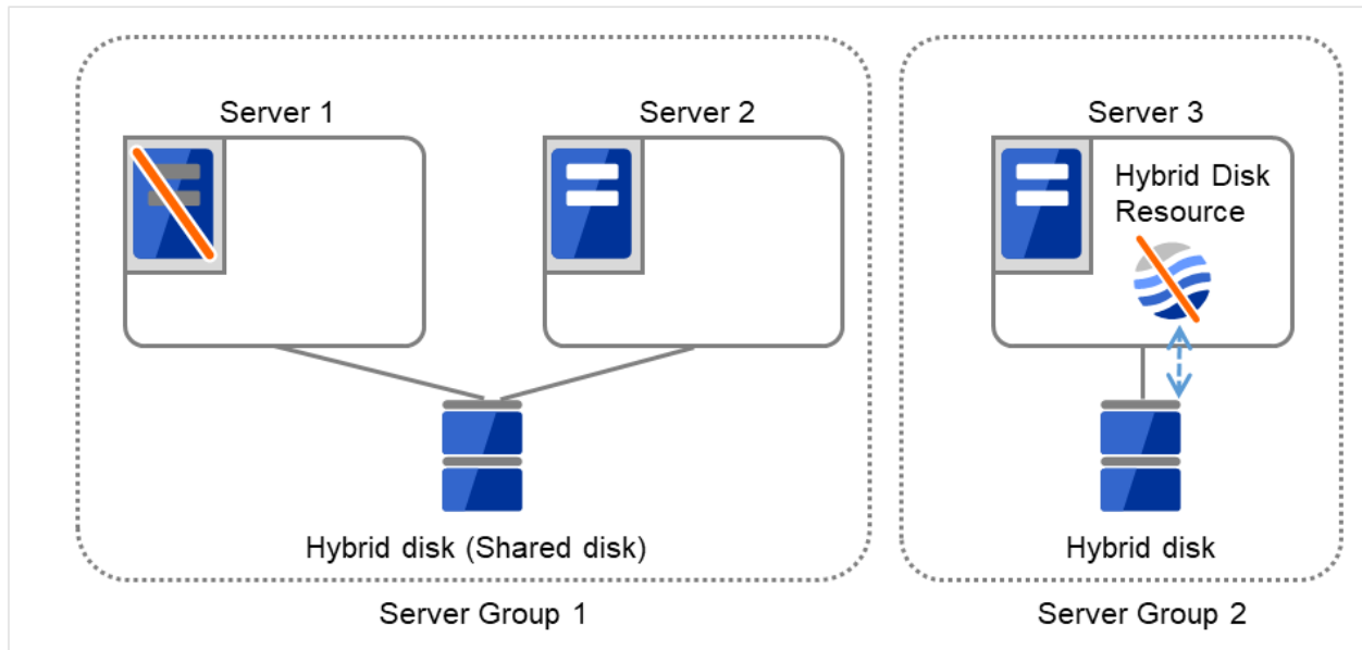
図 3.118 ハイブリッド構成 (3) (相手サーバグループ内でリソース活性, Server 1 ダウン後のミラー復帰)
