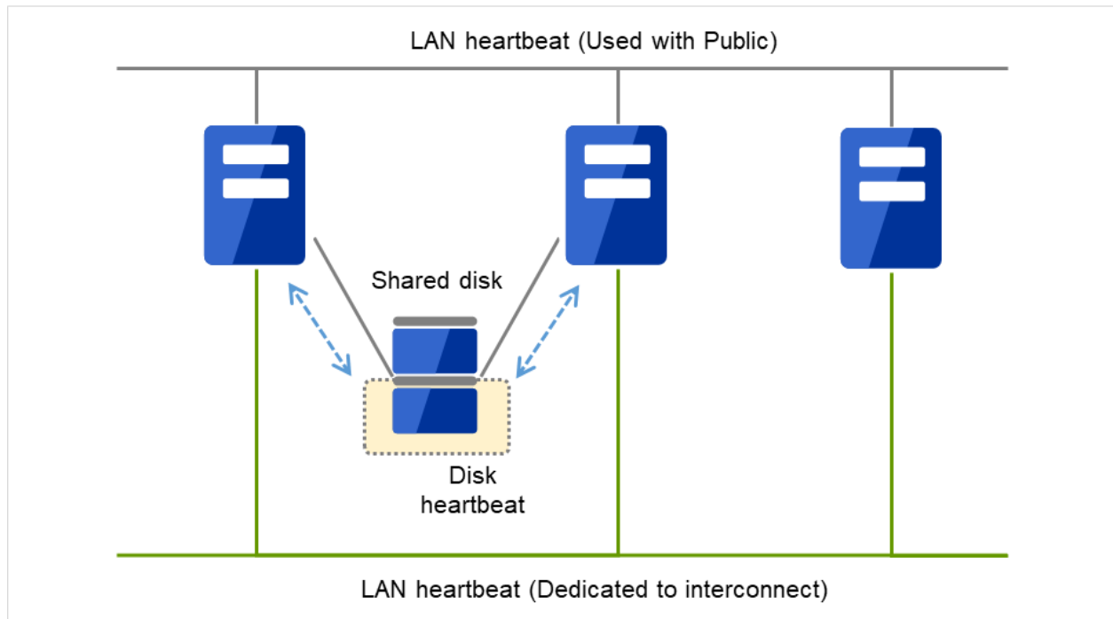
図 5.8 ディスクハートビートリソースを使用する構成（サーバ3台）
