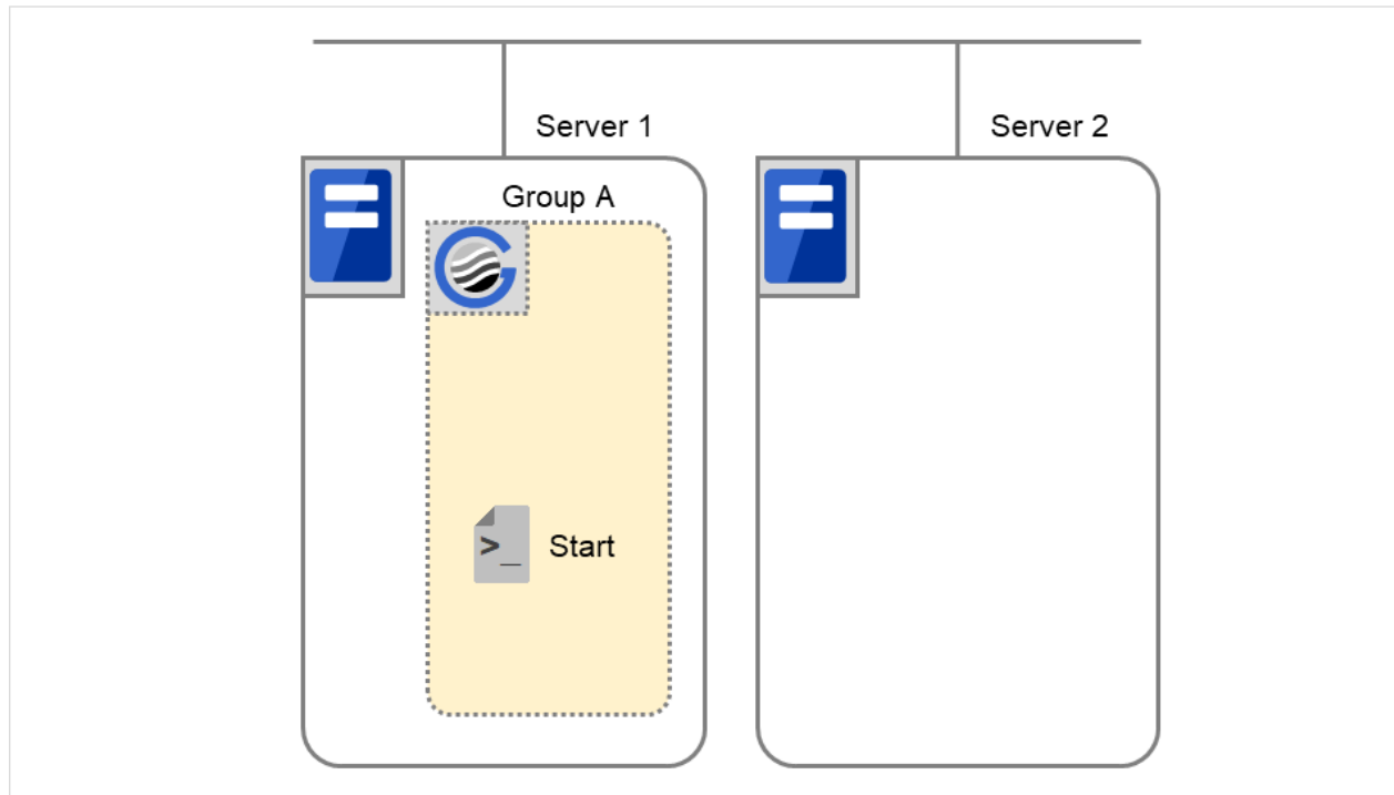
図 3.57 状態とスクリプト実行 (Group A の再起動) (2)
