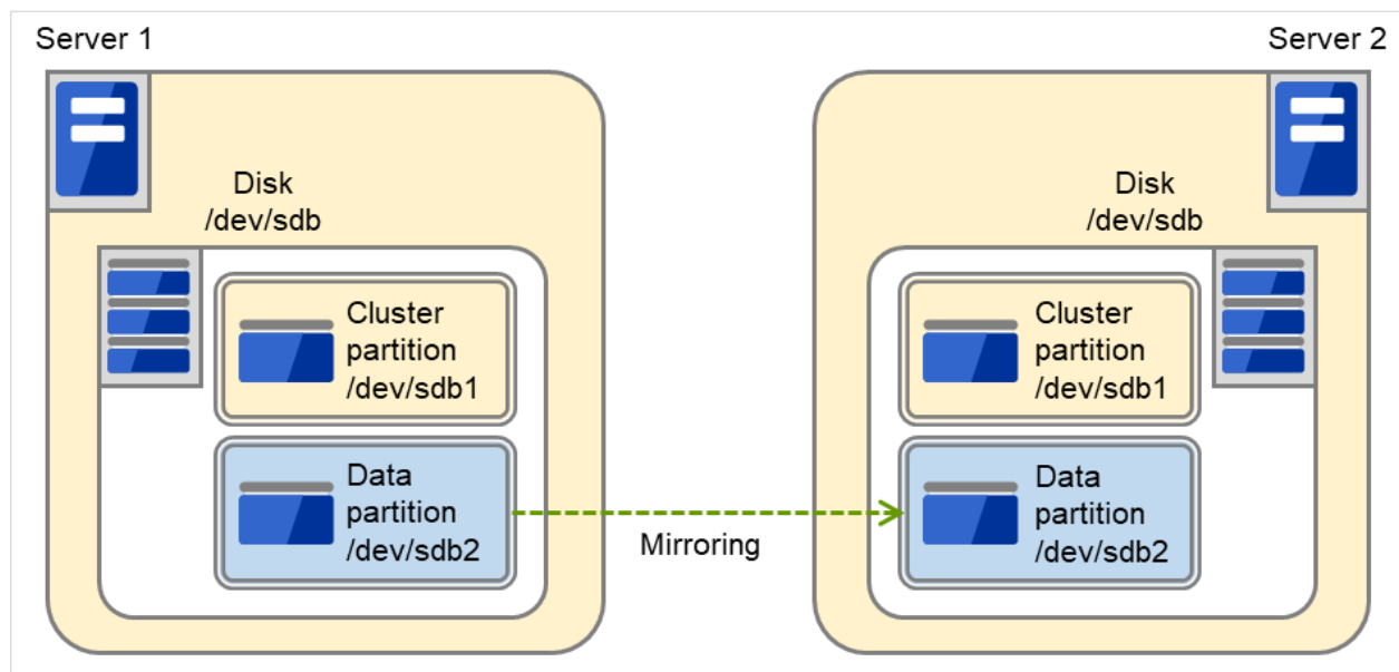
図 3.84 増設したディスク 1 つをミラーディスクのペアにする場合
