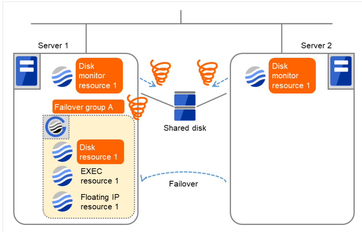
図 4.48 ディスクモニタリソース異常検出の流れ (11)
