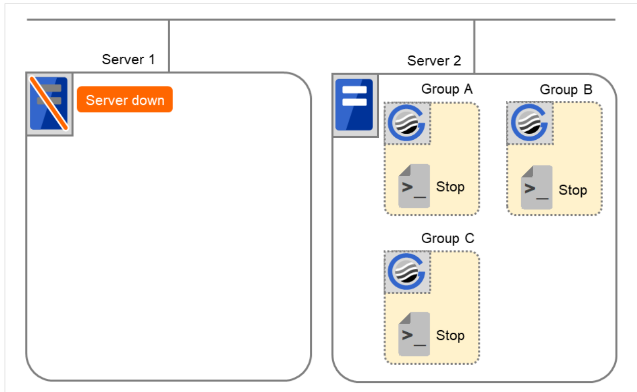
図 3.40 状態とスクリプト実行（フェイルオーバー後、クラスタシャットダウン）
