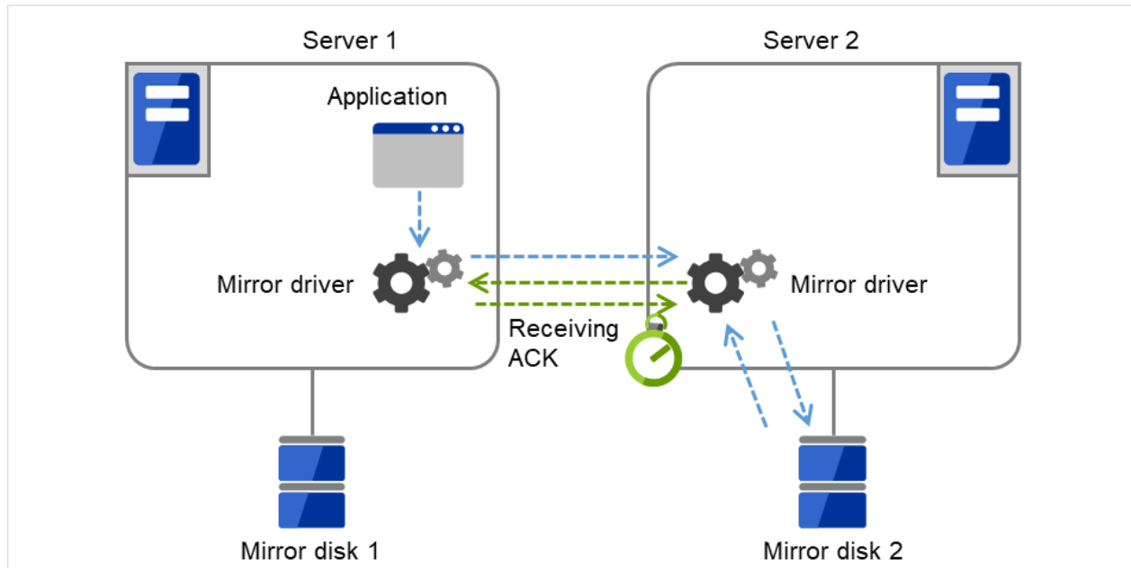
図 3.92 ACK タイムアウト（現用系サーバからの ACK 受信）
