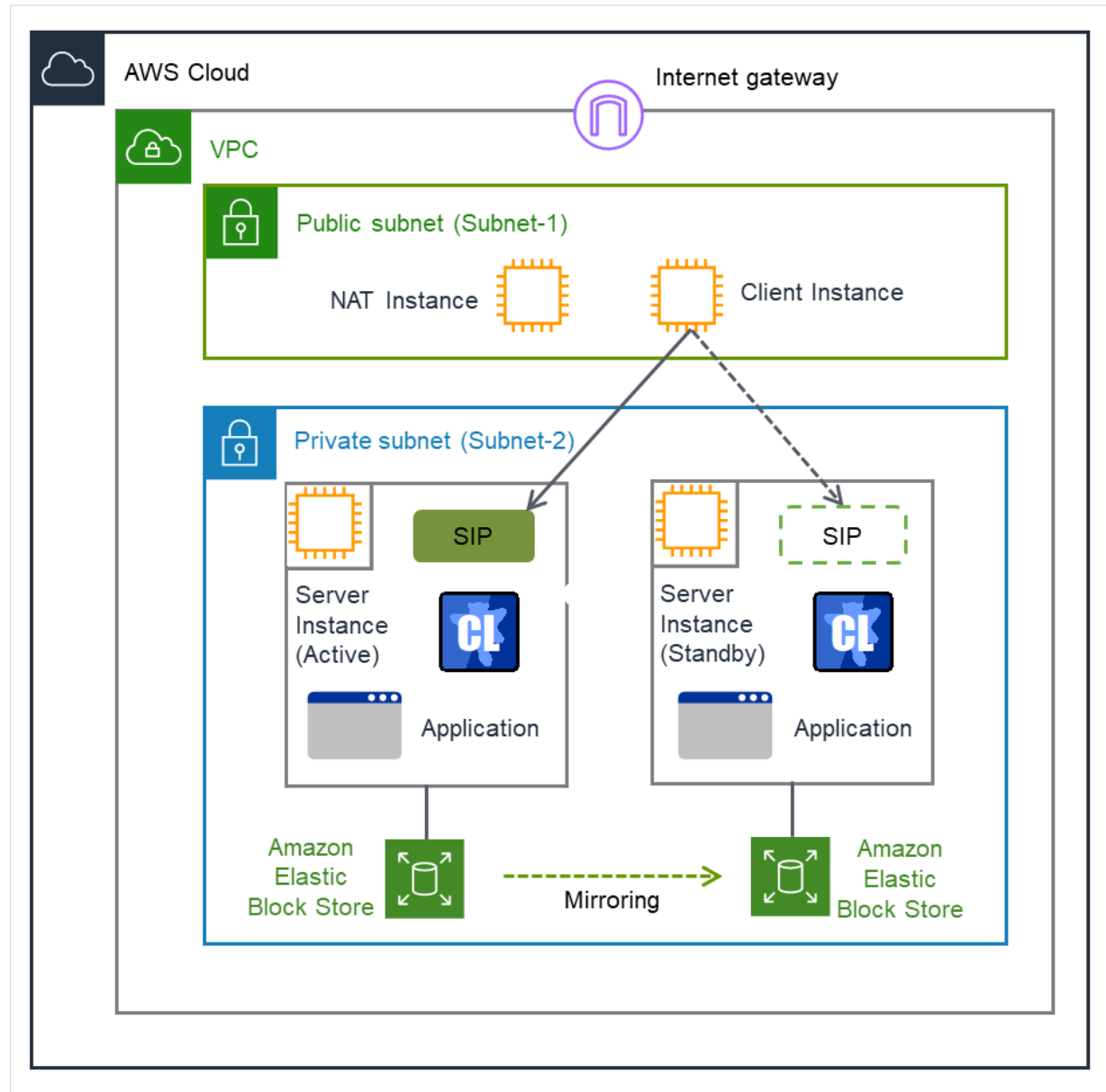
図 3.133 AWS セカンダリ IP リソースを使用する構成
