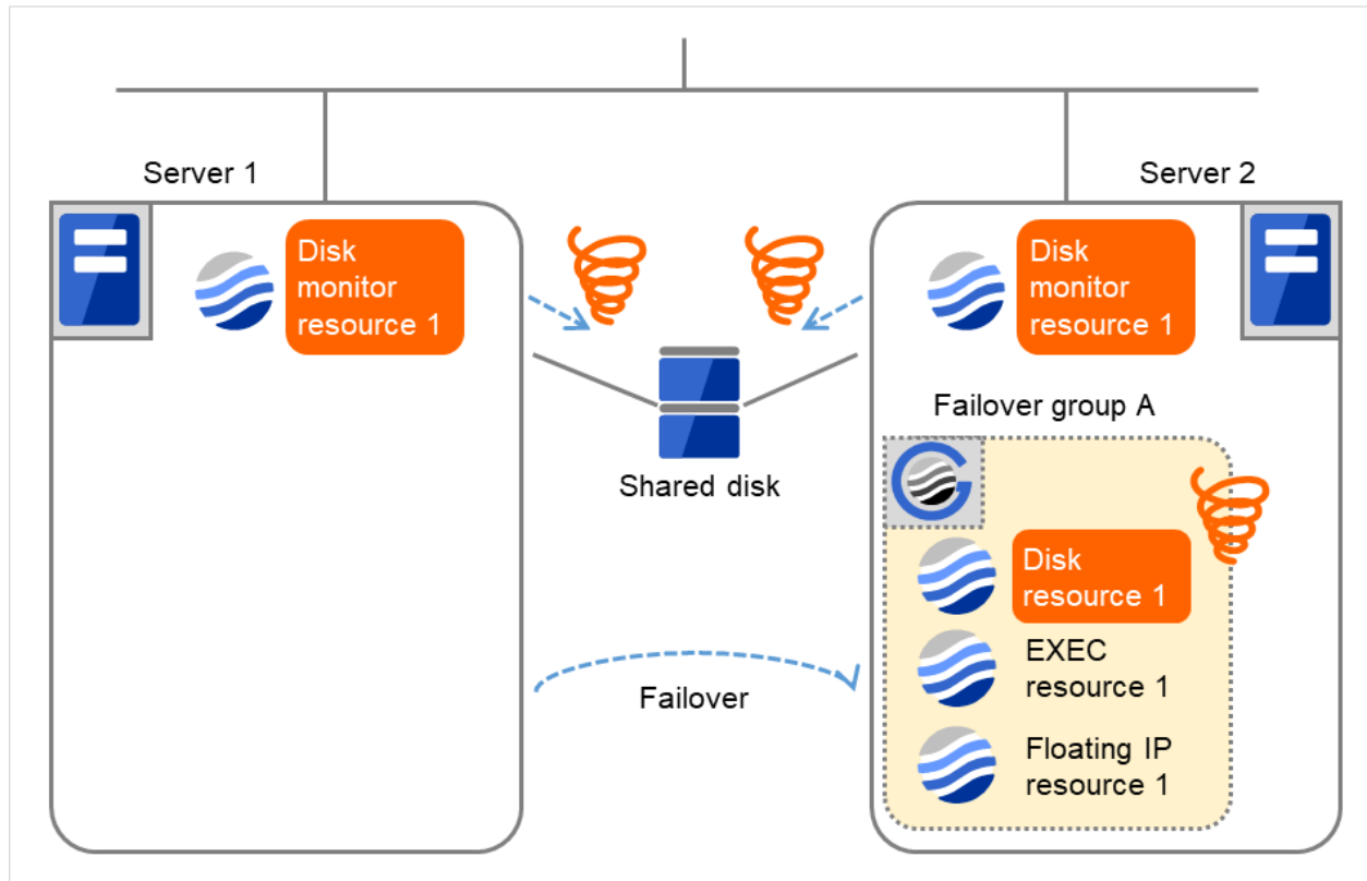
図 4.41 ディスクモニタリソース異常検出の流れ (4)
