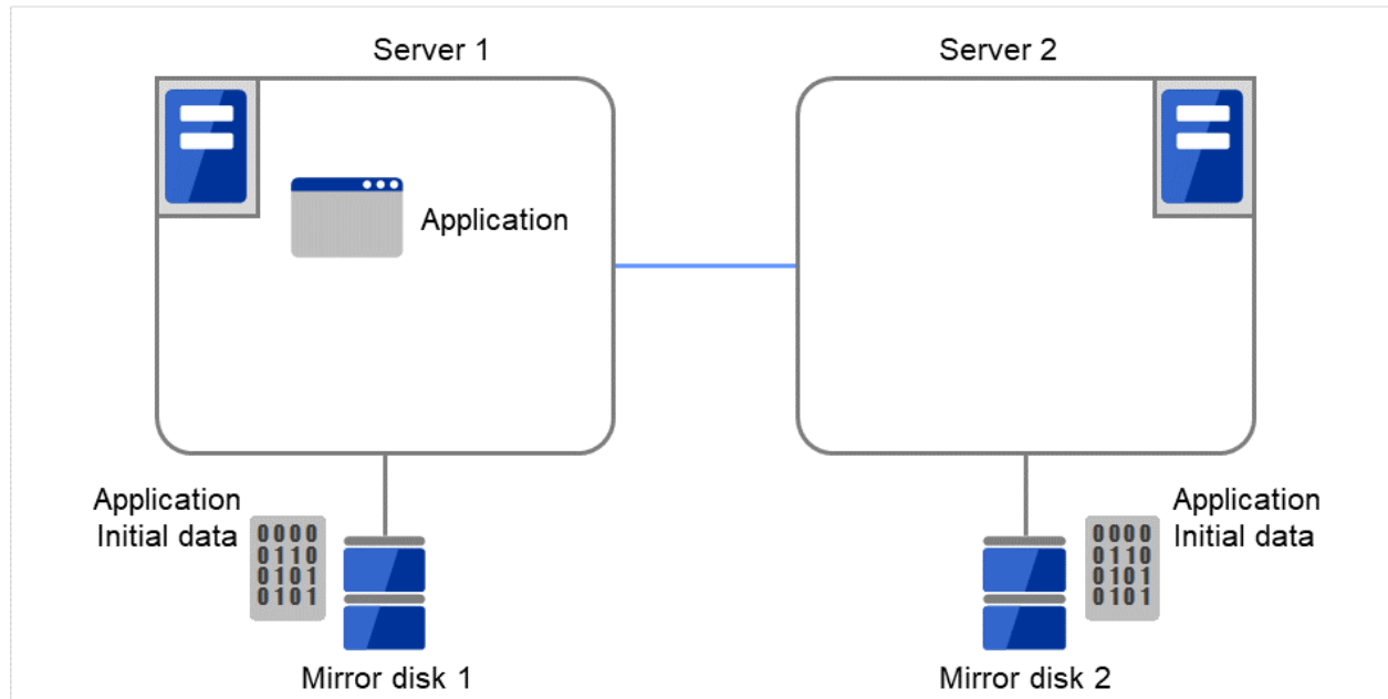
図 3.108 ミラーディスク構築例（バックアップ装置使用）(4)
