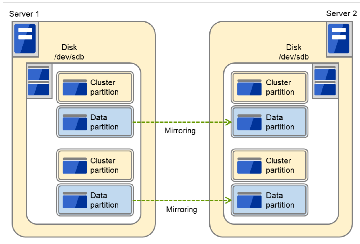
図 3.87 ディスク内の複数領域をミラーパーティションにする場合
