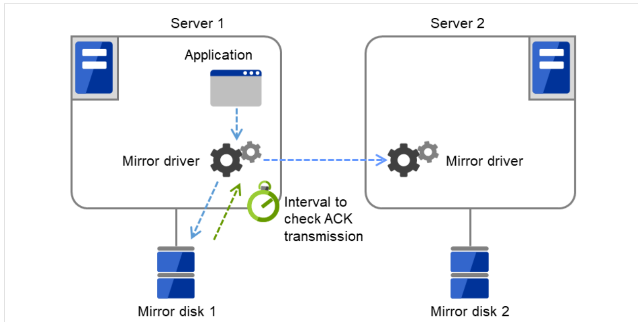
図 3.89 送信タイムアウト (ACK 送信チェック)
