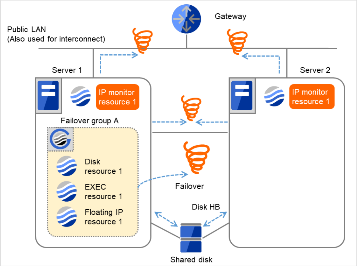
図 4.29 IP モニタリソース異常検出の流れ（全インタコネクト LAN が断線） (2)
