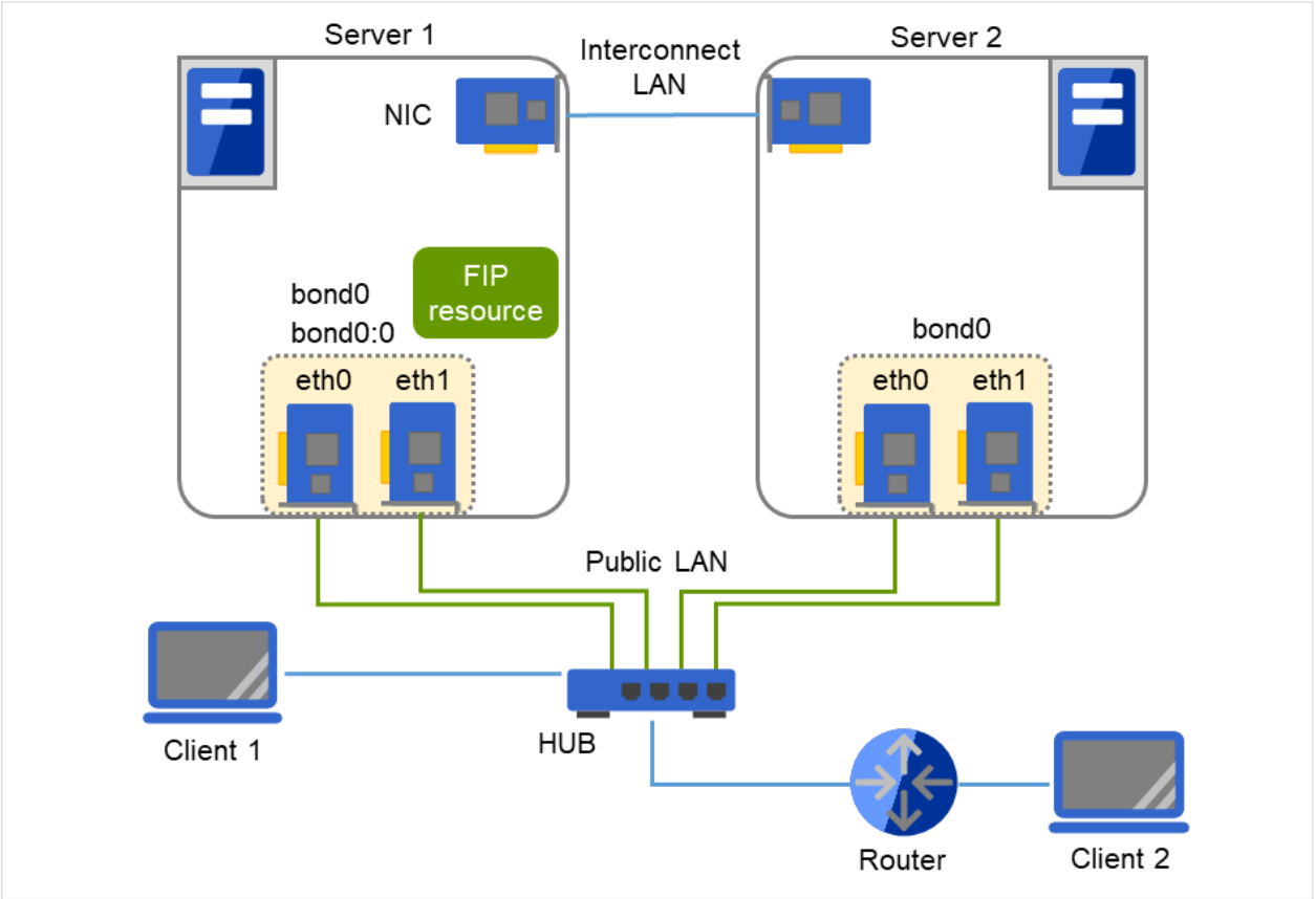
図 8.6 bonding 上でのフローティング IP リソース使用例
