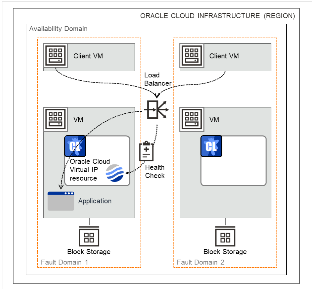
図 3.140 Oracle Cloud 仮想 IP リソースを使用する構成（プライベートロードバランサ）
