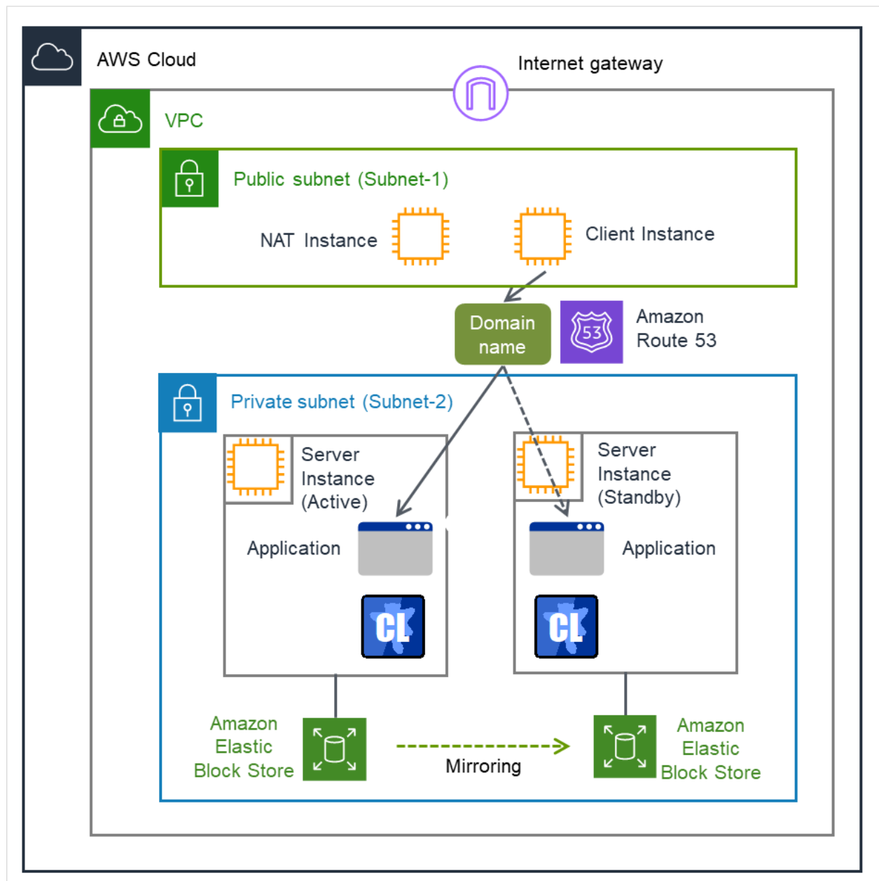
図 3.134 AWS DNS リソースを使用する構成
