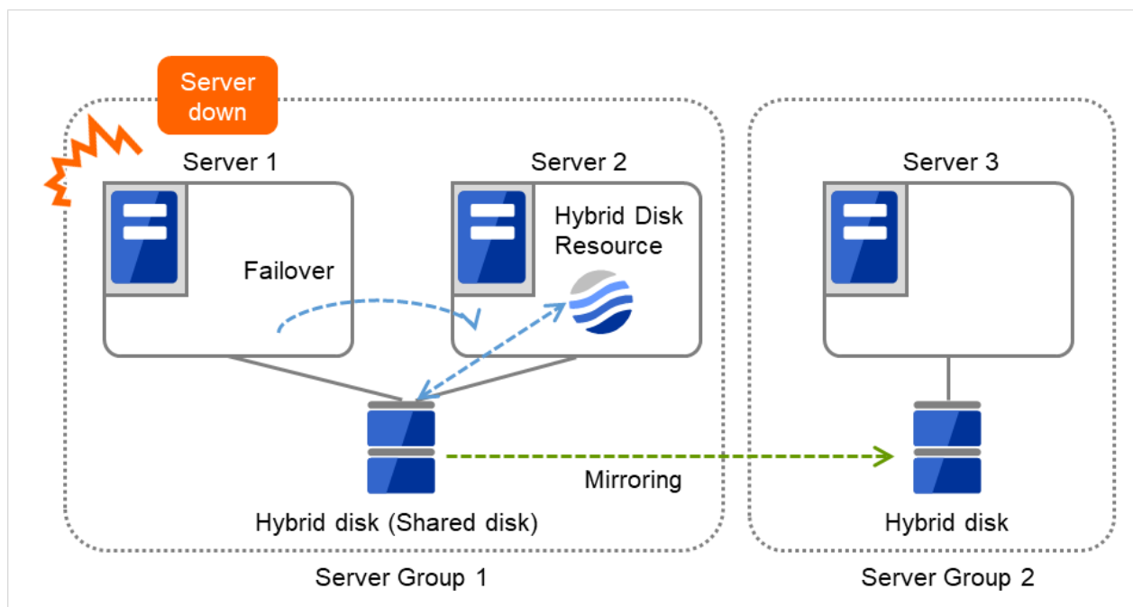
図 3.114 ハイブリッド構成 (2) (同一サーバグループ内でリソース活性, Server 1 ダウン)
