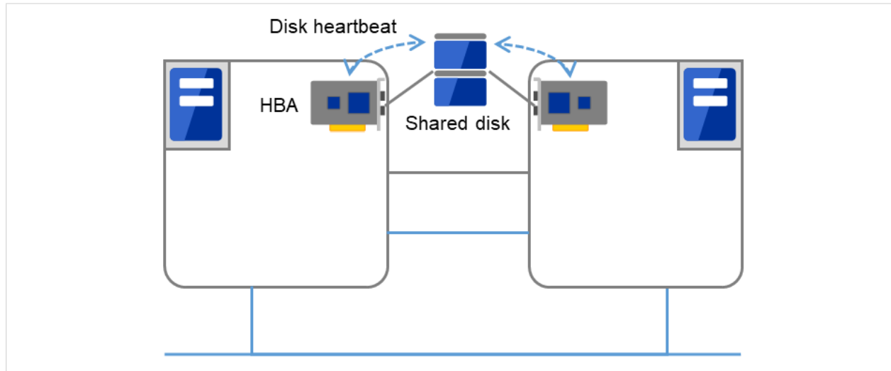
図 5.3 ディスクハートビート
