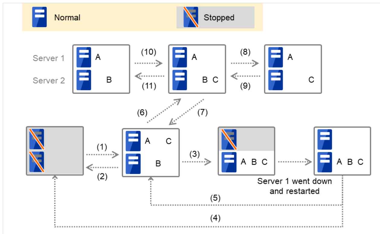
図 3.36 クラスタ状態遷移の例（概要）
