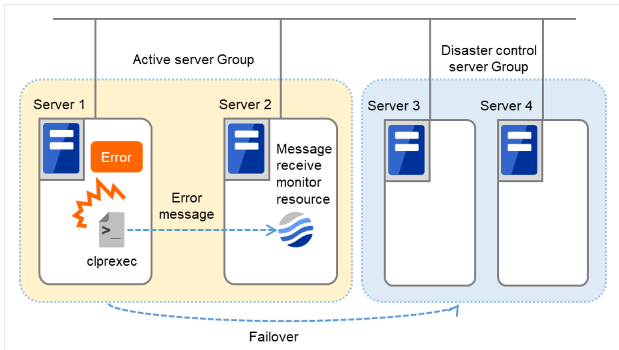
図 4.71 外部連携モニタリソースを使用する構成（サーバグループ外フェイルオーバー）
