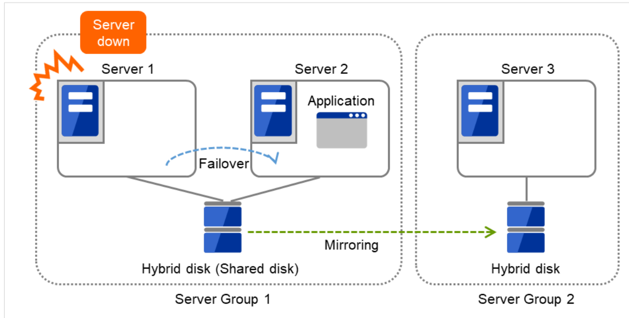
図 3.110 ハイブリッド構成 (2) (Server 1 ダウン)
