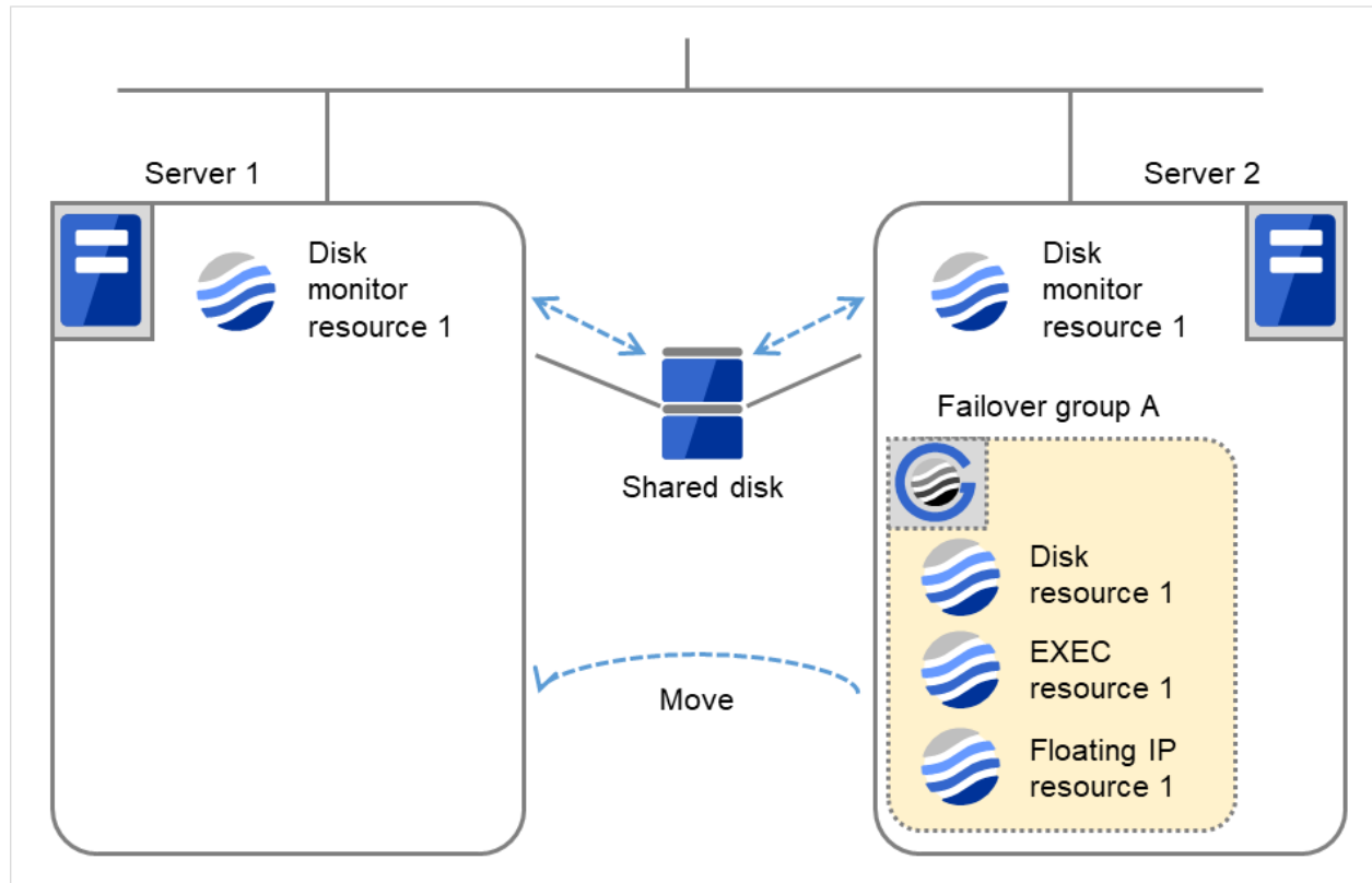
図 4.58 再起動回数制限 (4)
