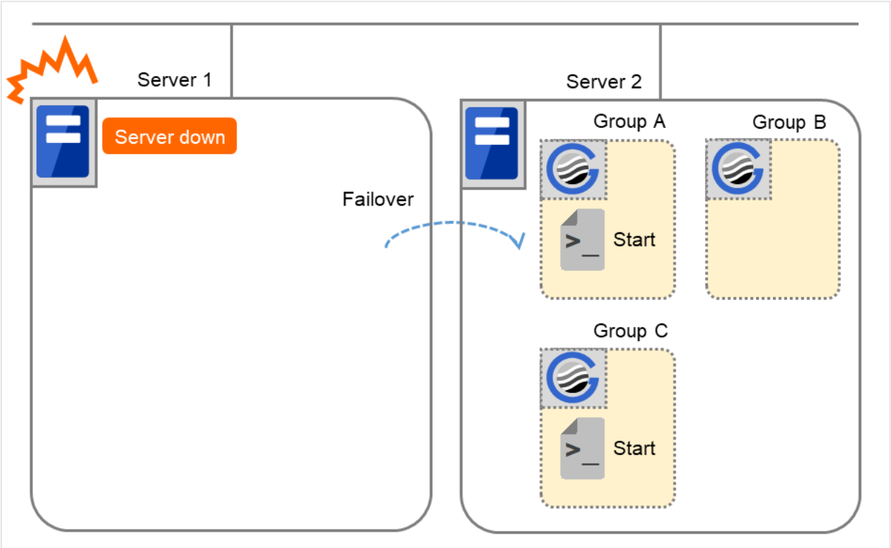
図 3.39 状態とスクリプト実行（サーバダウンによるフェイルオーバー）
