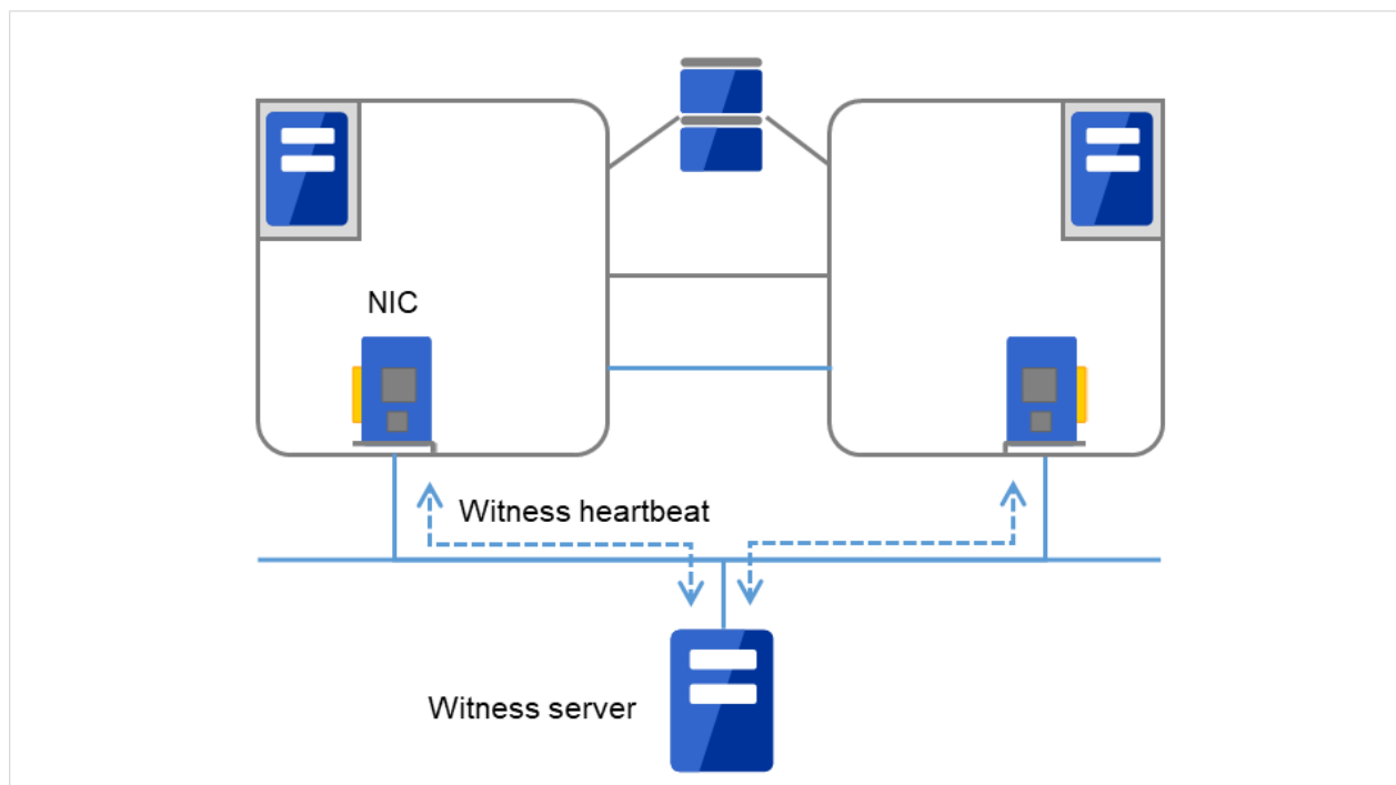
図 5.4 Witness ハートビート
