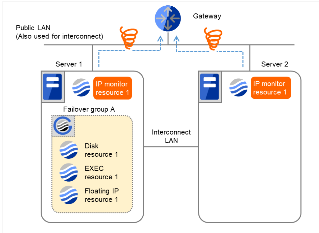
図 4.34 IP モニタリソース異常検出の流れ（監視異常からの復帰・正常）（3）
