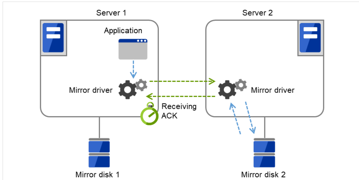
図 3.91 ACK タイムアウト（待機系サーバからの ACK 受信）
