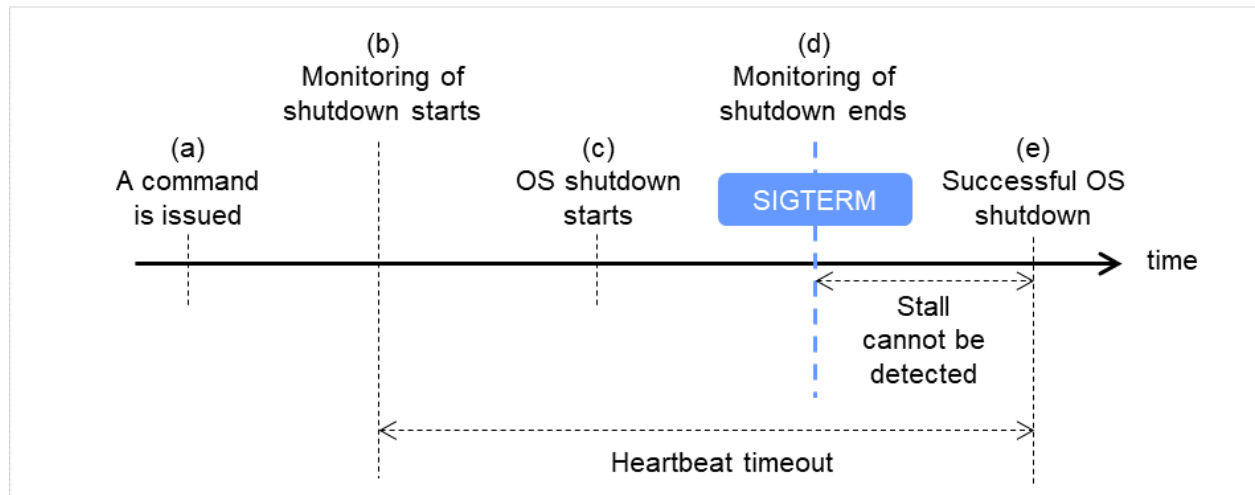
図 8.1 シャットダウン成功時（監視方法が softdog、SIGTERM が有効の場合）
