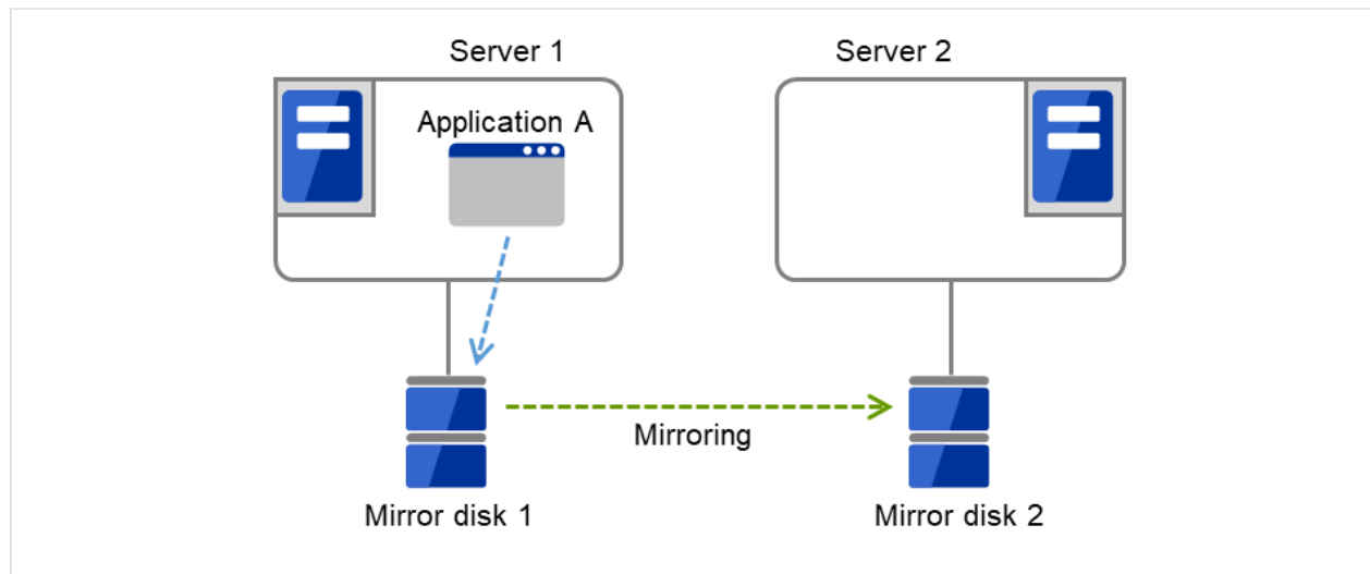
図 3.82 ミラーディスク構成 (1)
