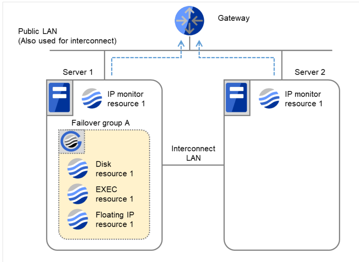
図 4.33 IP モニタリソース異常検出の流れ（監視異常からの復帰・正常）（2）
