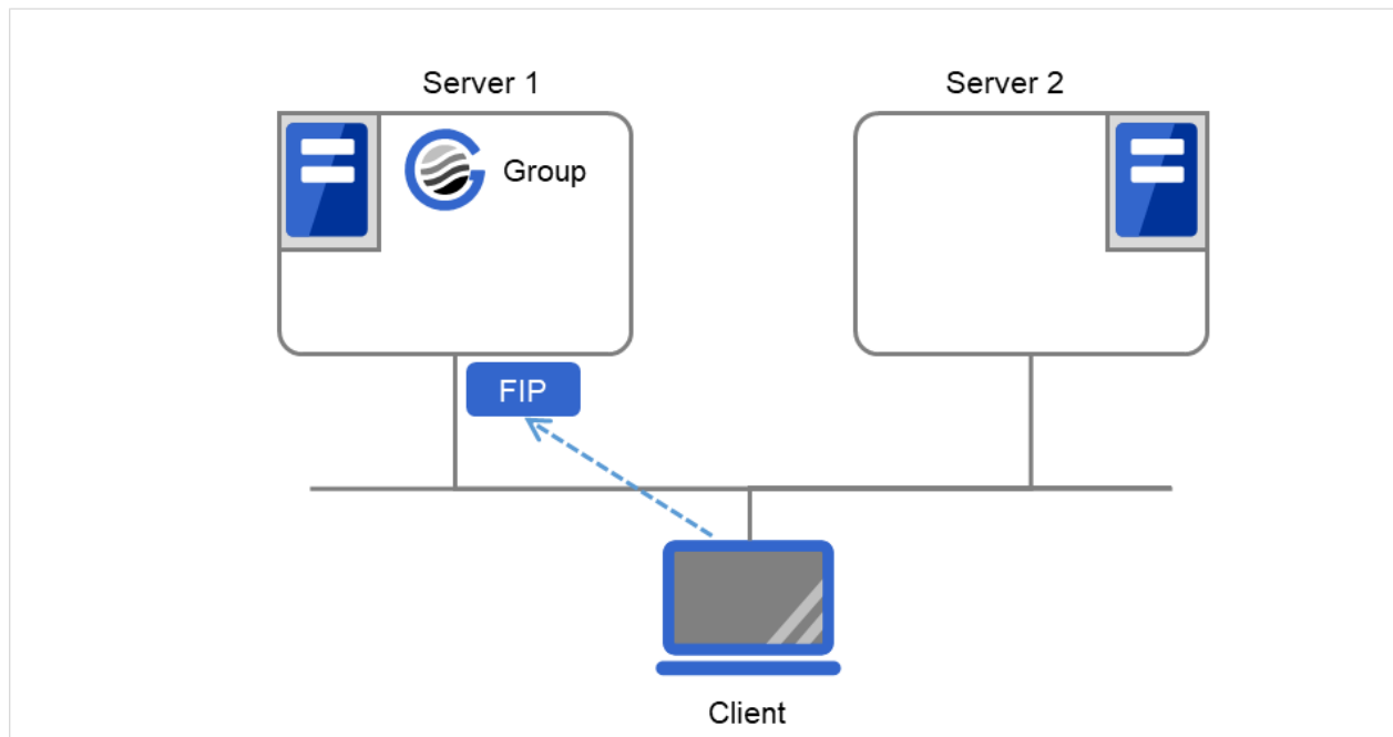
図 3.75 フローティング IP 構成 (1) (通常時)
