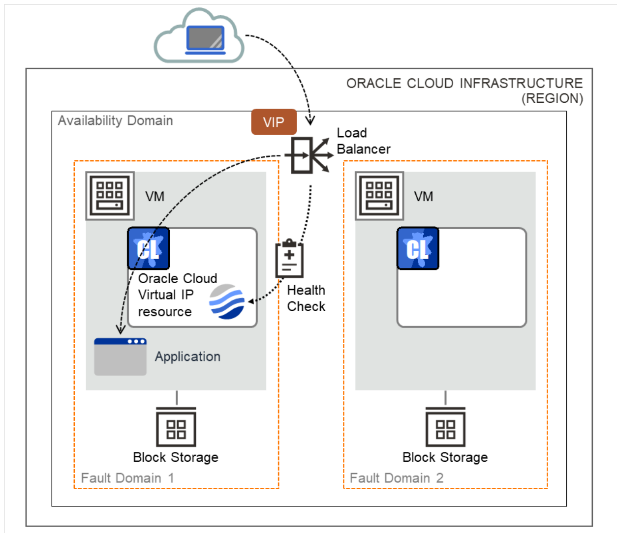
図 3.139 Oracle Cloud 仮想 IP リソースを使用する構成
