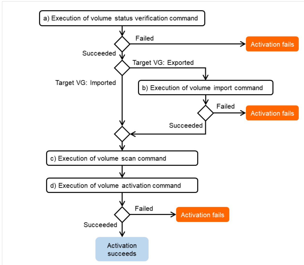
図 3.124 リソース活性時のシーケンス (lvm)
