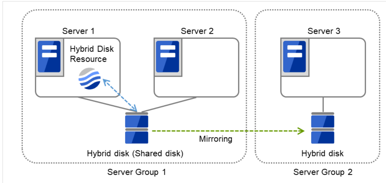
図 3.113 ハイブリッド構成 (1) (同一サーバグループ内でリソース活性, 通常時)
