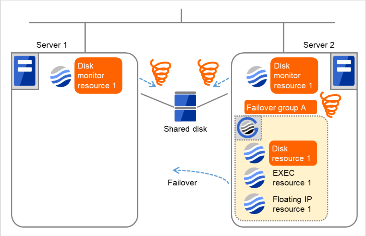
図 4.47 ディスクモニタリソース異常検出の流れ (10)
