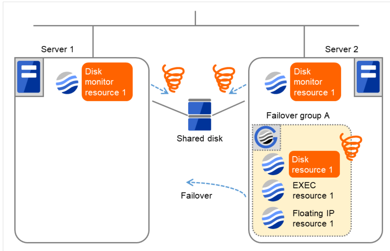
図 4.42 ディスクモニタリソース異常検出の流れ (5)
