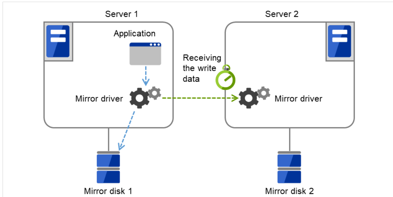
図 3.90 受信タイムアウト
