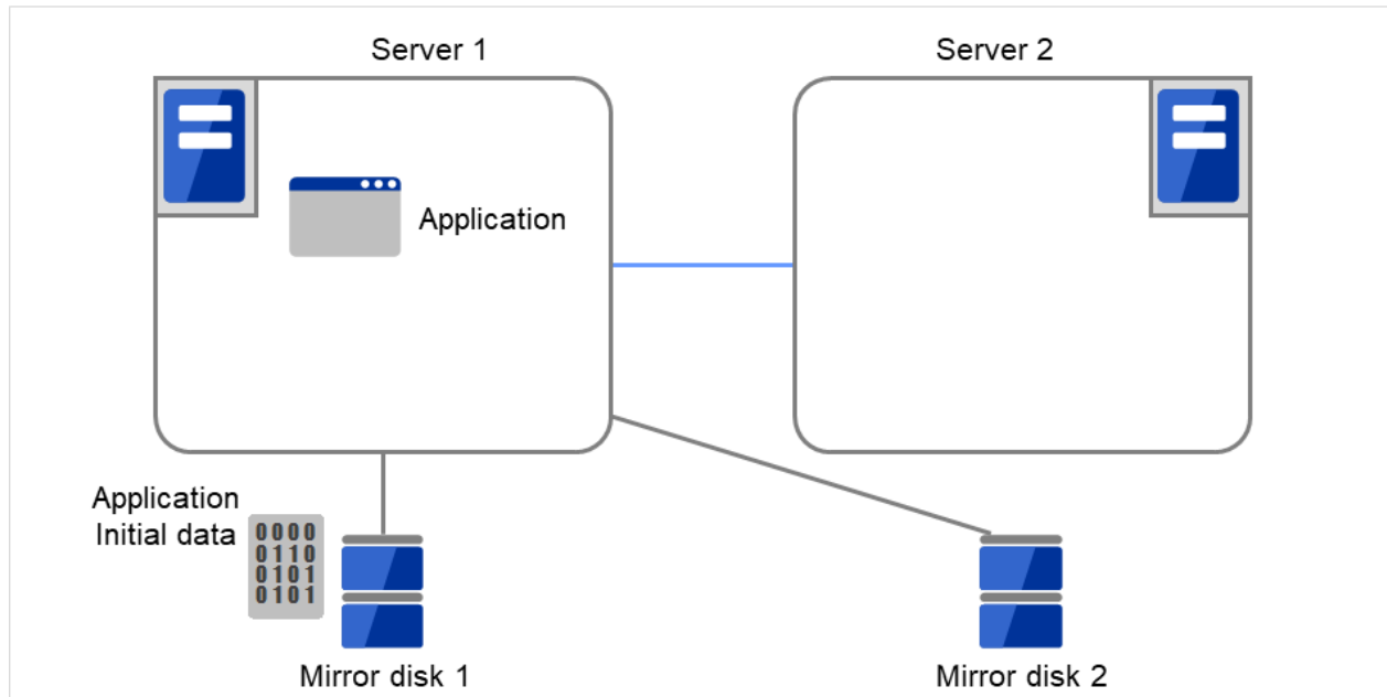
図 3.102 ミラーディスク構築例（パーティションイメージコピー）(2)
