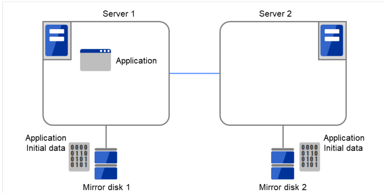
図 3.104 ミラーディスク構築例（パーティションイメージコピー）(4)
