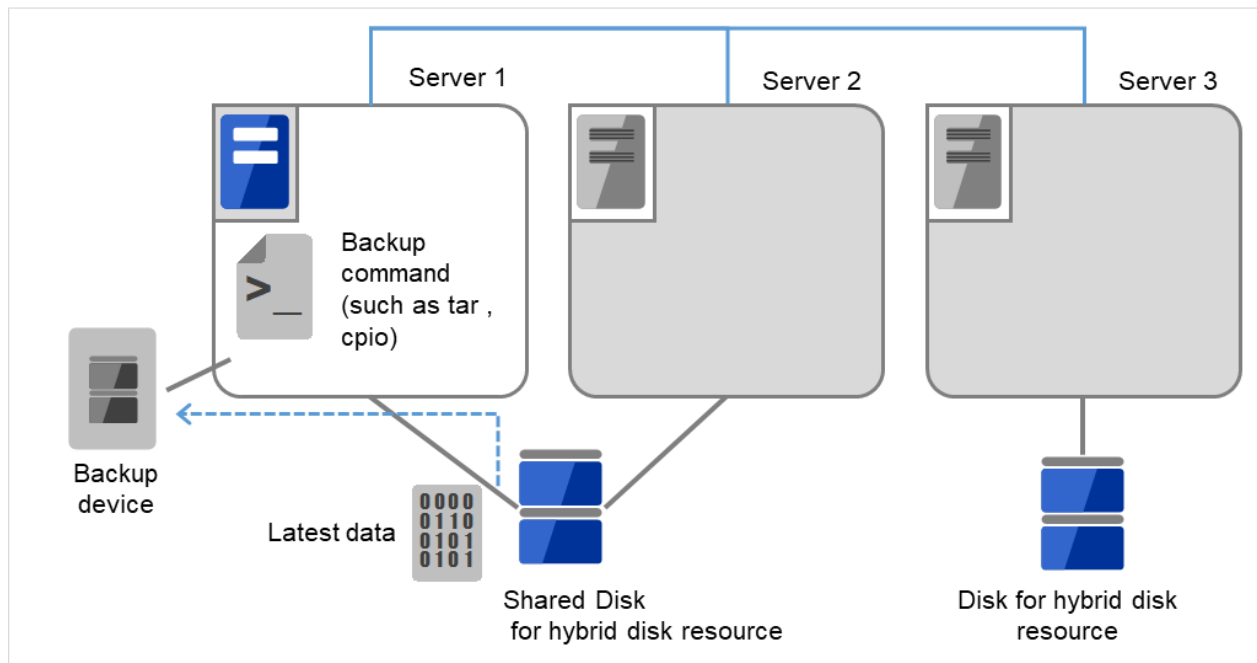
図 10.9 ハイブリッドディスク上のデータ保存 (4)
