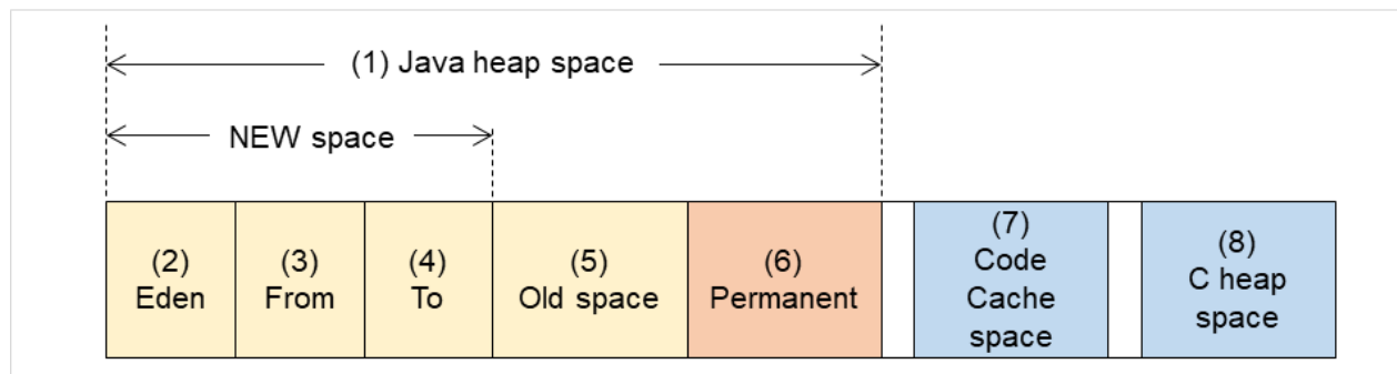
図 4.76 Java VM メモリ空間 (Oracle Java 7)
