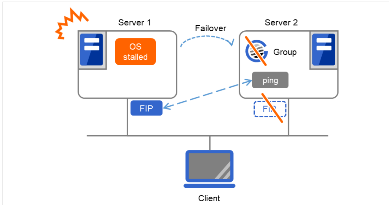
図 3.76 フローティング IP 構成 (2) (フェイルオーバー失敗)
