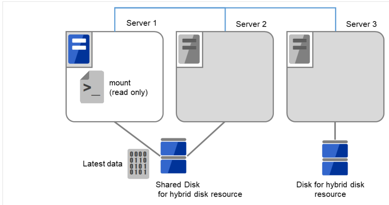
図 10.8 ハイブリッドディスク上のデータ保存 (3)
