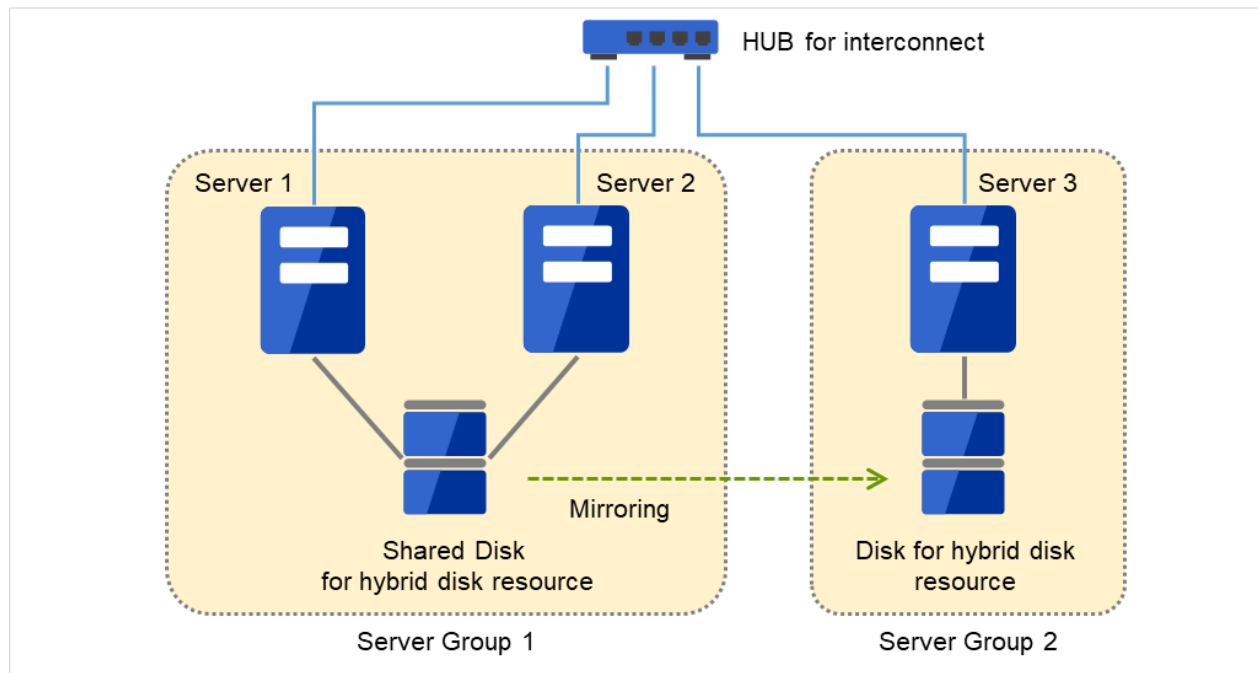
図 3.32 サーバグループ
