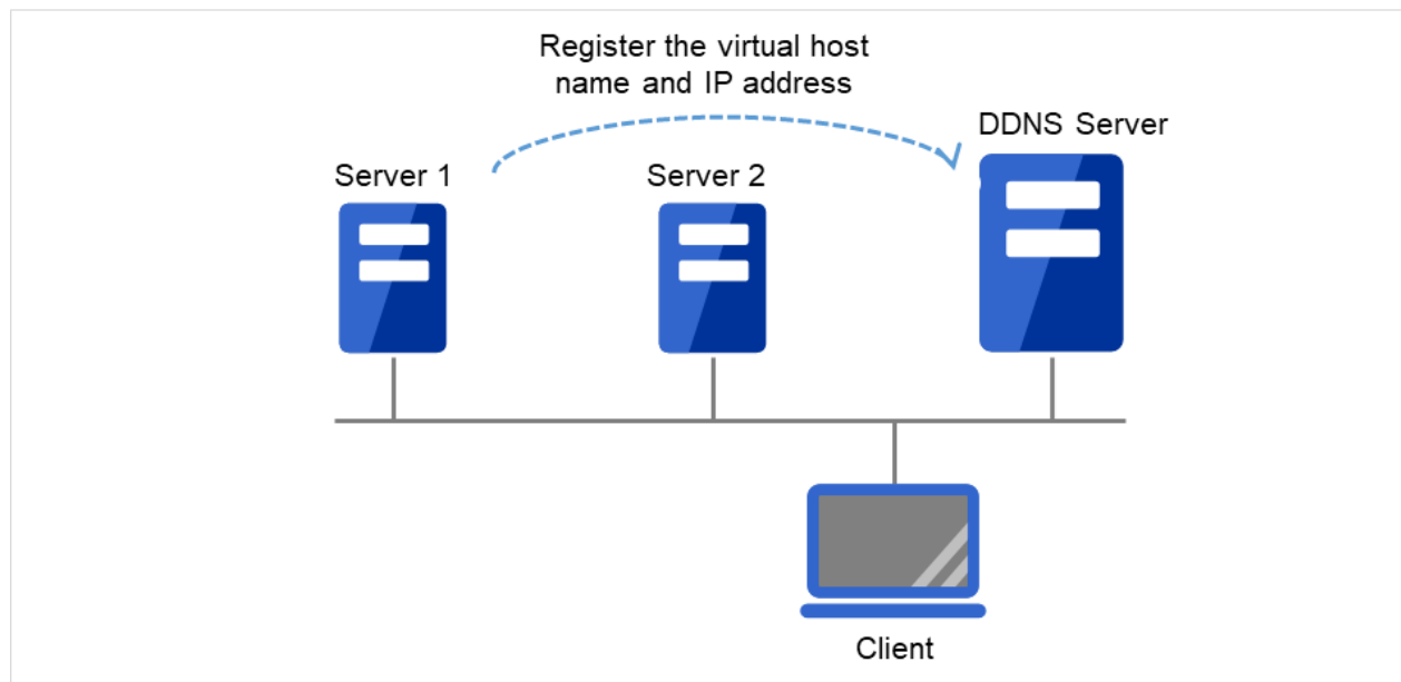
図 3.126 ダイナミック DNS サーバを使用する構成 (1)
