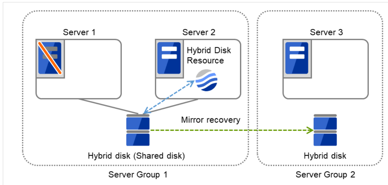
図 3.115 ハイブリッド構成 (3)（同一サーバグループ内でリソース活性, Server 1 ダウン後のミラー復帰）
