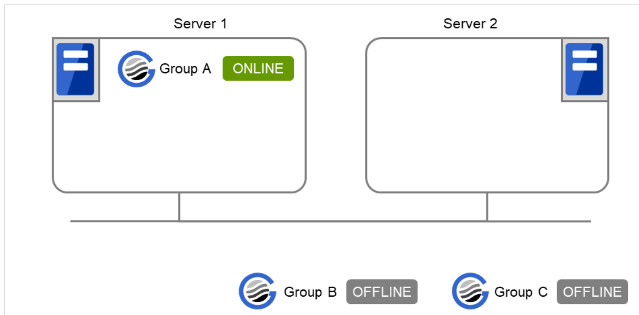
図 3.30 Server 1 で Group A が起動
