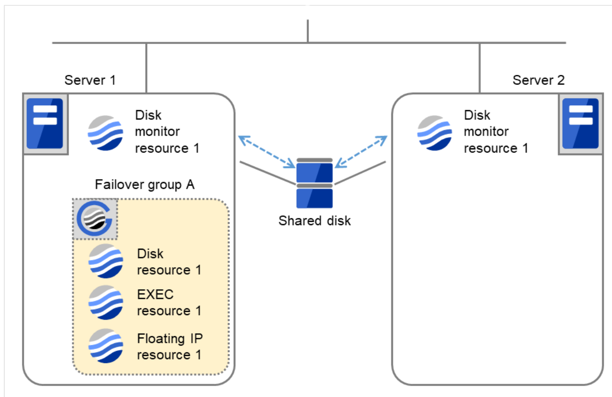
図 4.38 ディスクモニタリソース異常検出の流れ (1)
