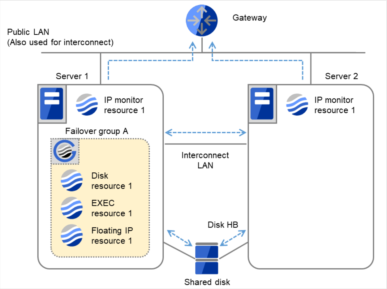
図 4.28 IP モニタリソース異常検出の流れ（全インタコネクト LAN が断線）（1）
