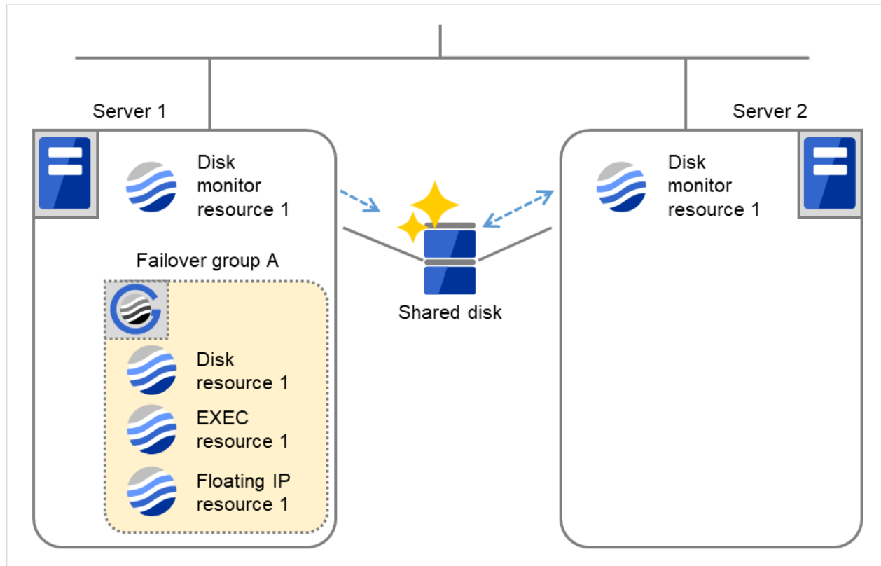
図 4.60 再起動回数制限 (6)
