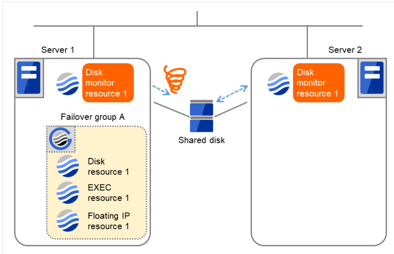
図 4.56 再起動回数制限 (2)
