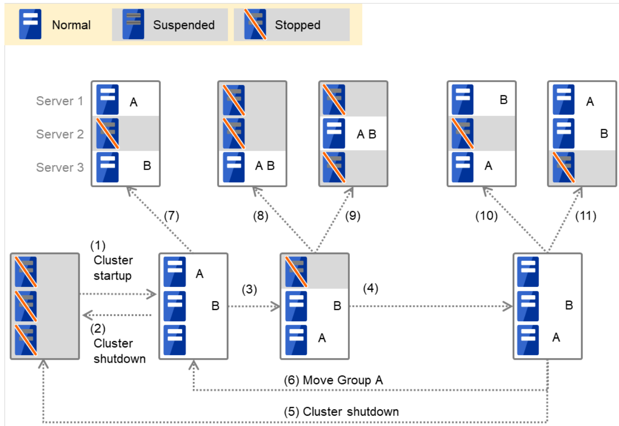
図 3.2 各サーバの状態と Group A、Group B の起動状況（A、B は通常排他）
