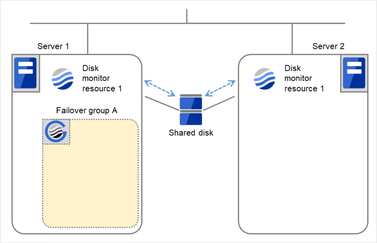
図 4.61 再起動回数制限 (7)
