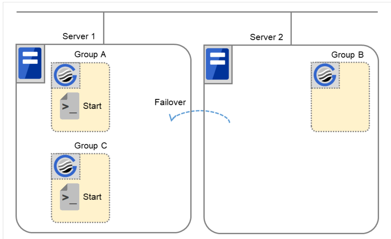
図 3.42 状態とスクリプト実行 (Group A、Group C の移動) (2)
