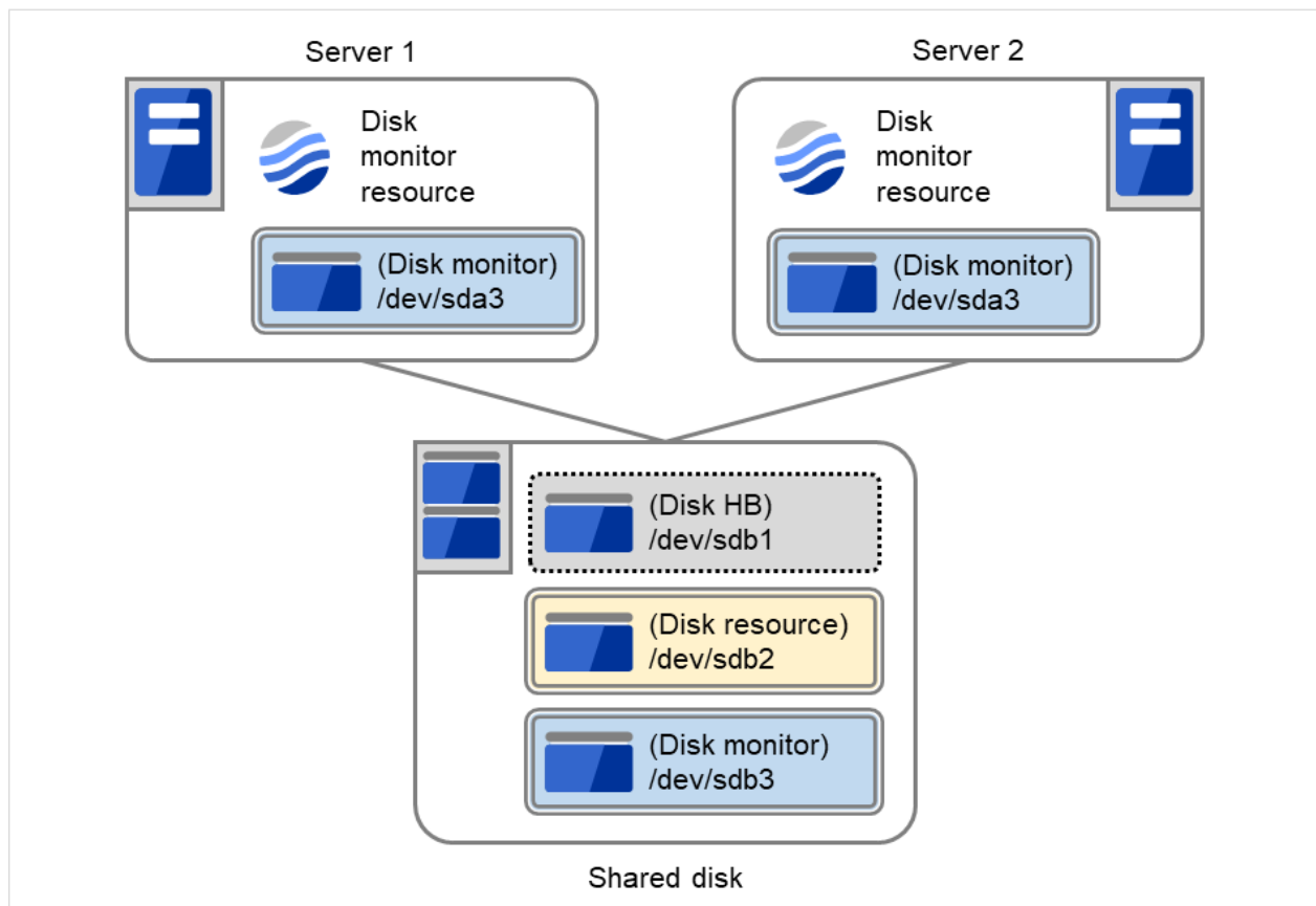
図 4.63 ディスクリソース、ディスクモニタの設定例
