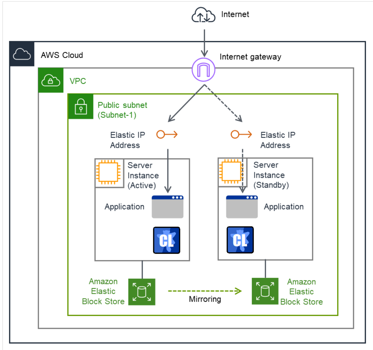
図 3.131 AWS Elastic IP リソースを使用する構成
