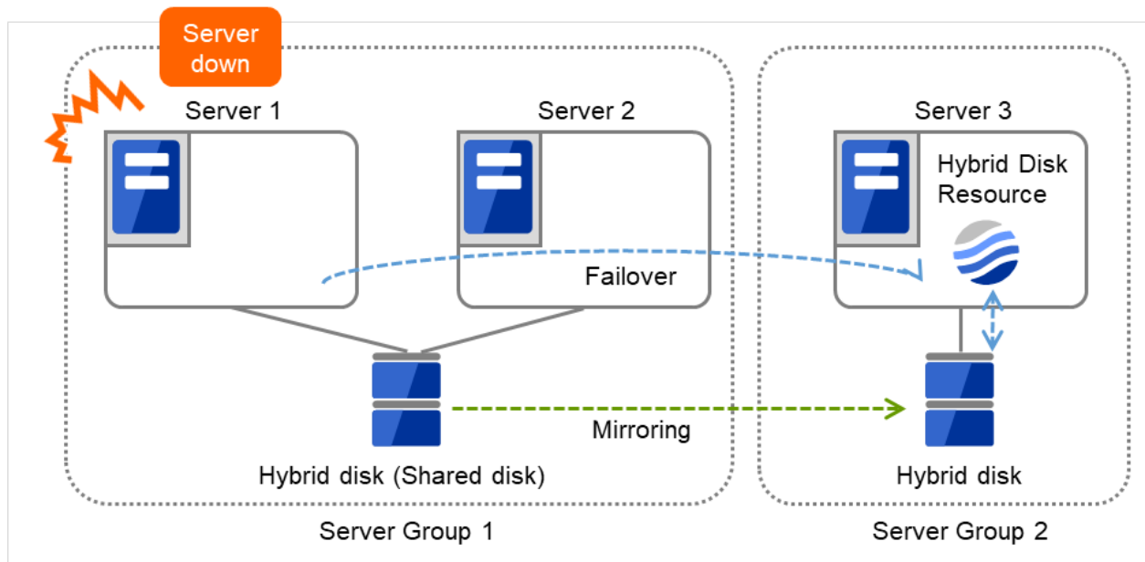
図 3.117 ハイブリッド構成 (2) (相手サーバグループ内でリソース活性, Server 1 ダウン)
