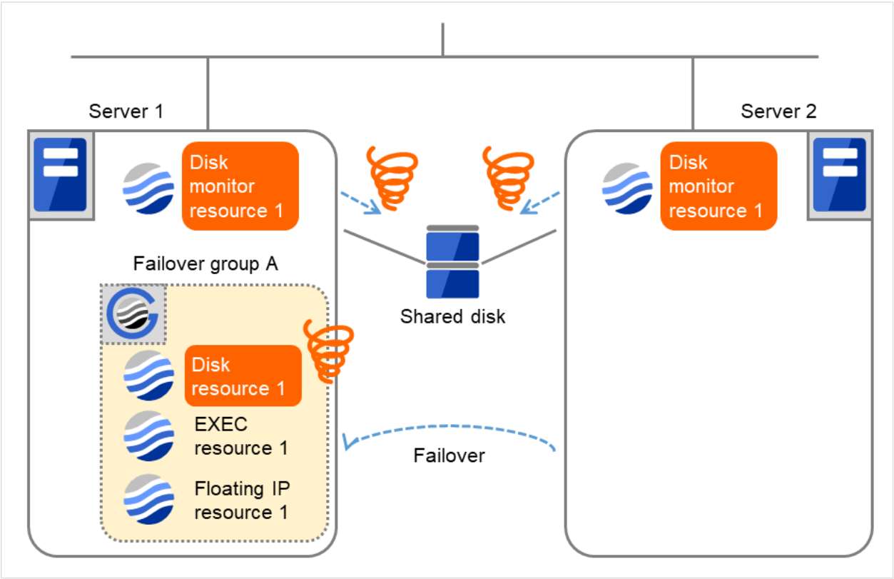
図 4.43 ディスクモニタリソース異常検出の流れ (6)
