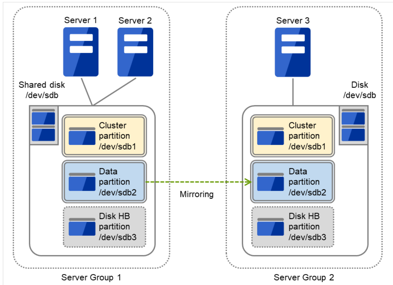
図 3.112 ハイブリッド構成におけるパーティション
