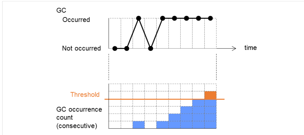
図 4.75 監視イメージ (異常判定しきい値を 5 回に設定した場合)
