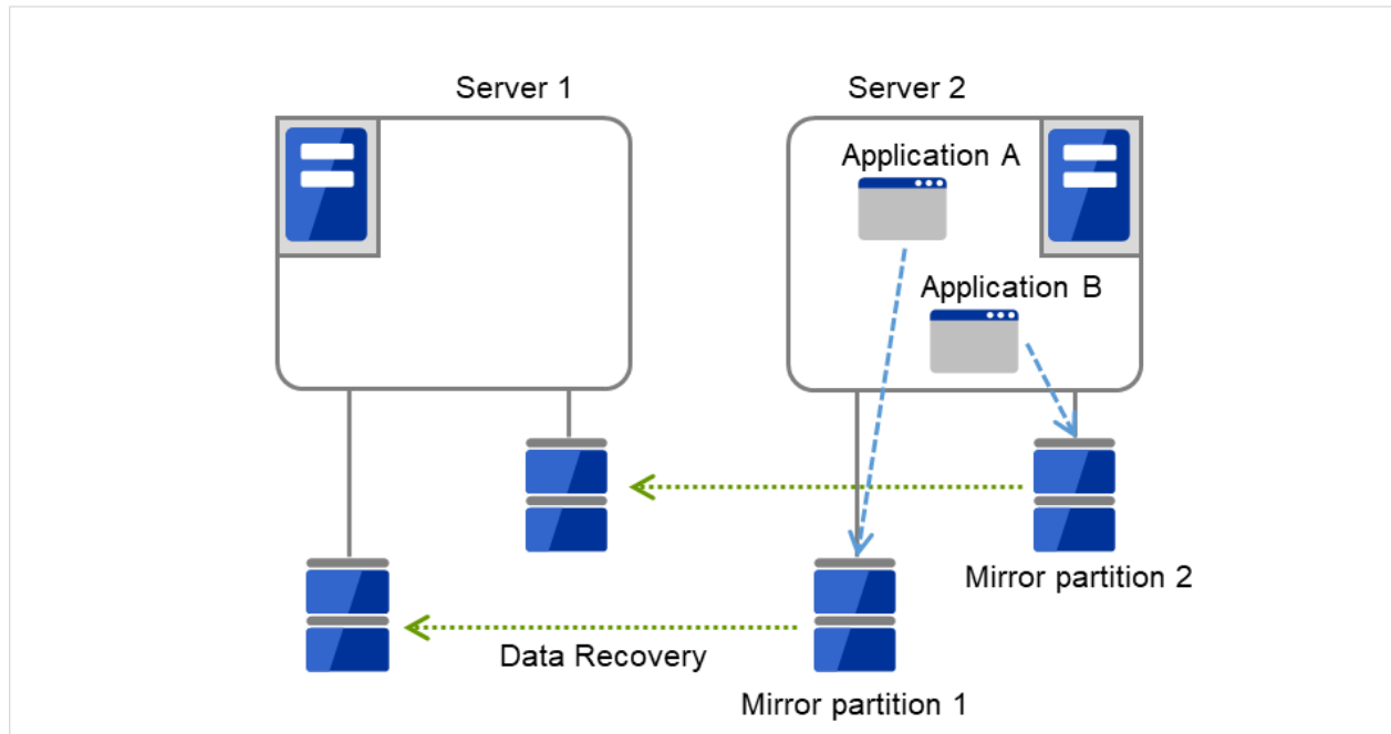
図 3.21 双方向スタンバイクラスター（ミラーディスク使用）：(4) データ復旧時
