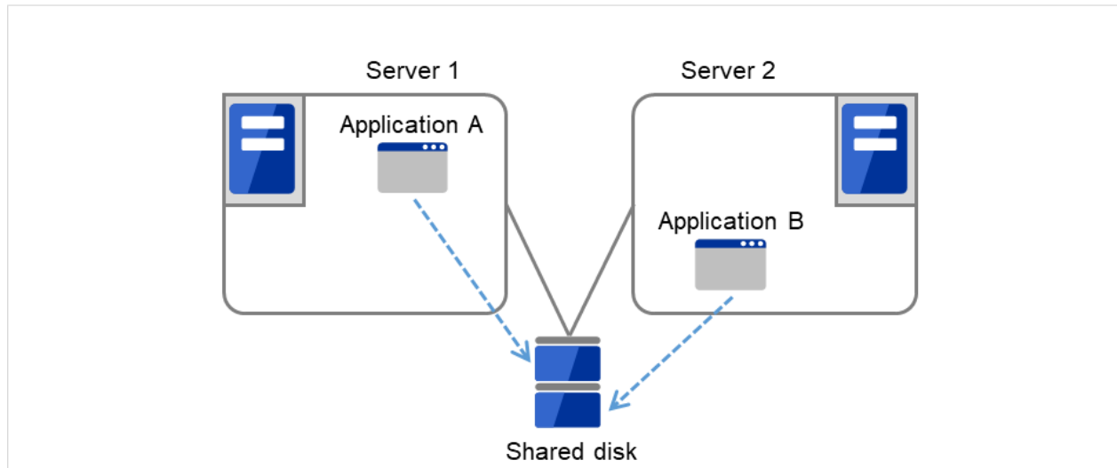
図 3.14 異種アプリケーション双方向スタンバイクラスタ (1)
