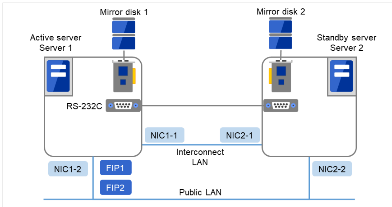
図 3.20 クラスタ構成例 (2) (ミラーディスク型)
