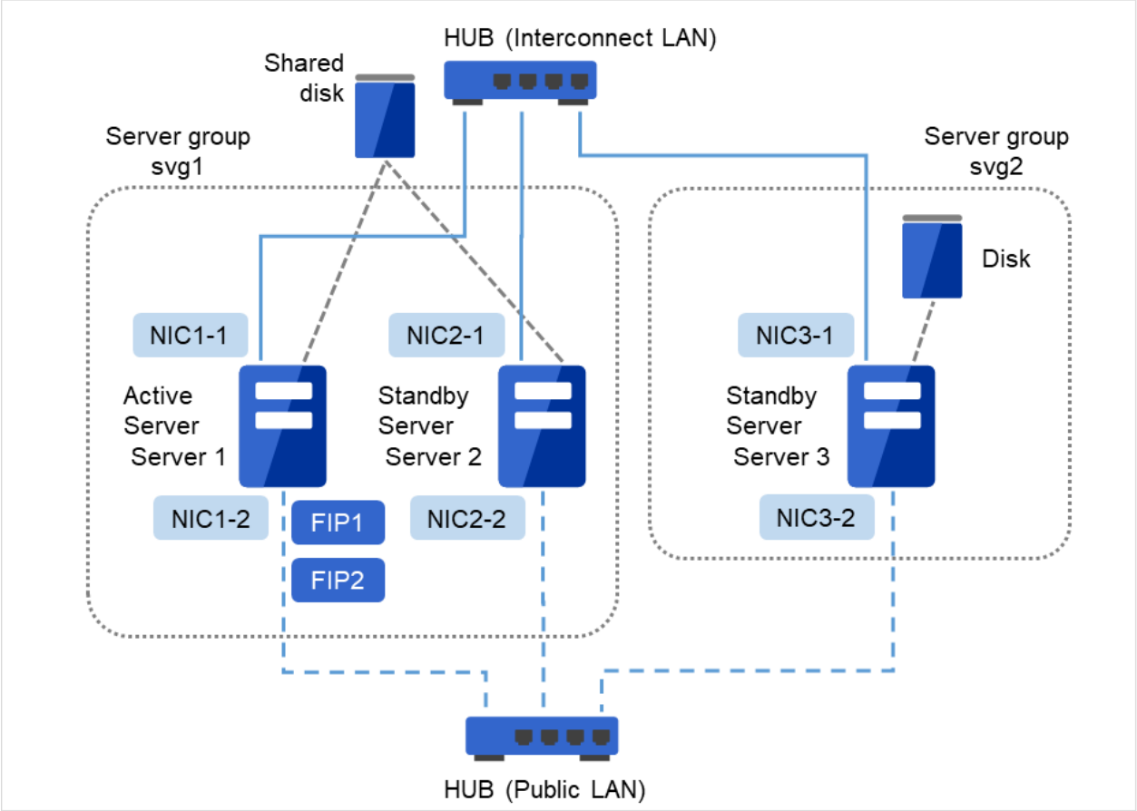
図 3.21 クラスタ構成例 (ハイブリッドディスク型)
