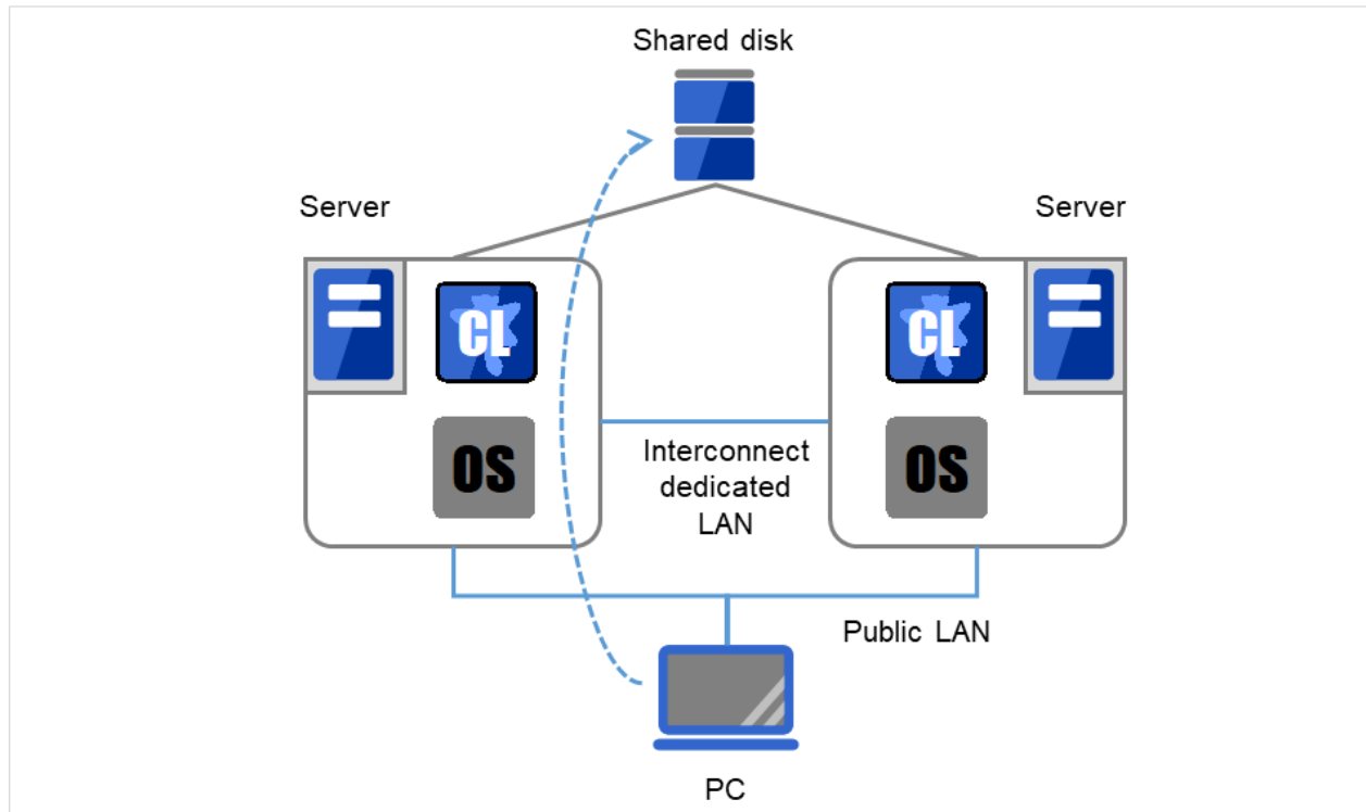
図 3.9 フェイルオーバー型クラスタのシステム構成
