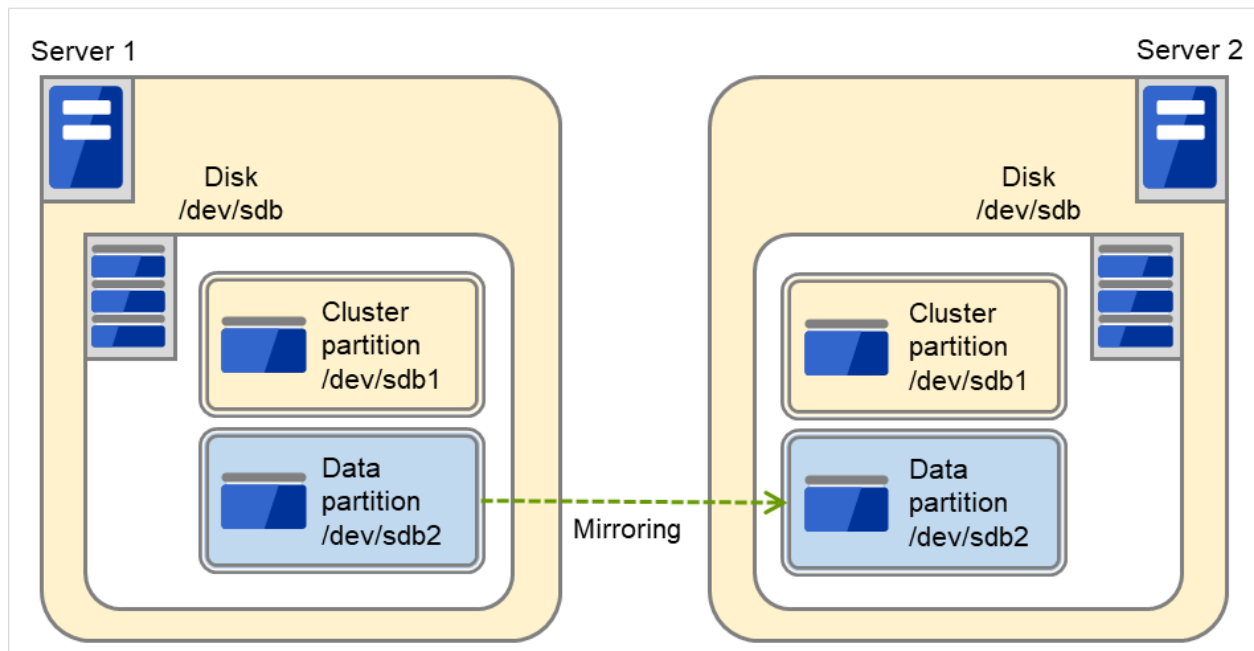
図 6.3 ディスクとパーティション構成（SCSI ディスク増設時）
