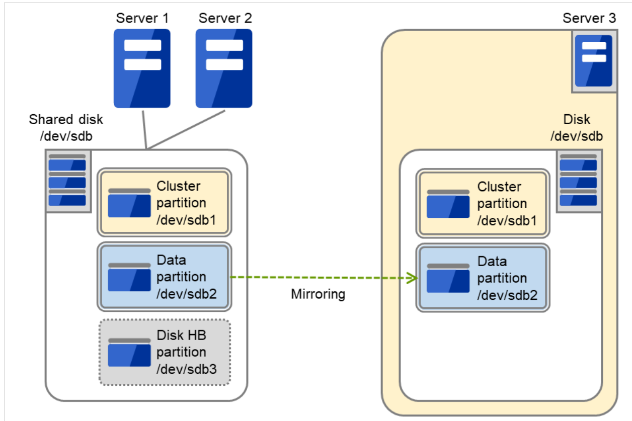
図 6.7 ディスクとパーティション構成（共有ディスクと内蔵ディスク使用時）
