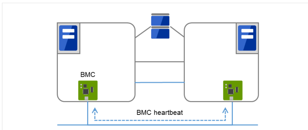
図 3.6 BMC ハートビート
