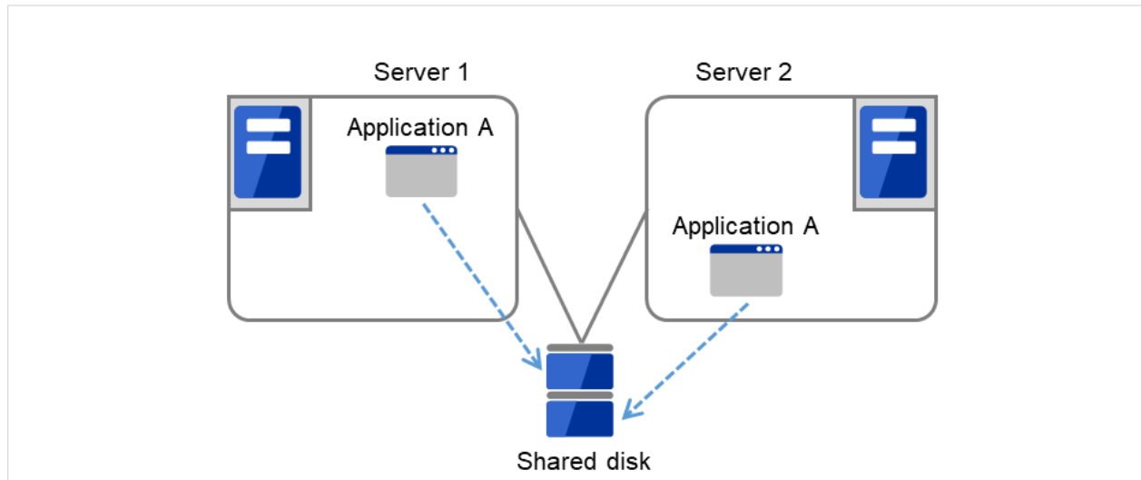
図 3.12 同一アプリケーション双方向スタンバイクラスタ (1)
