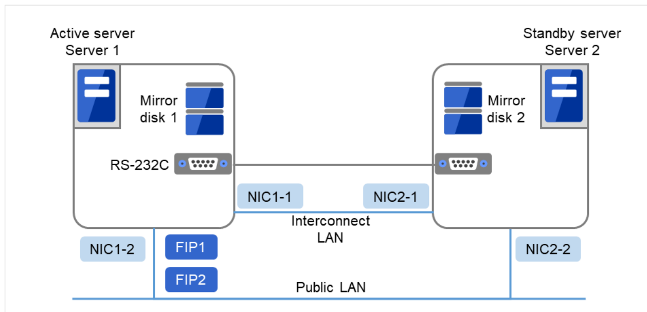
図 3.19 クラスタ構成例 (1) (ミラーディスク型)
