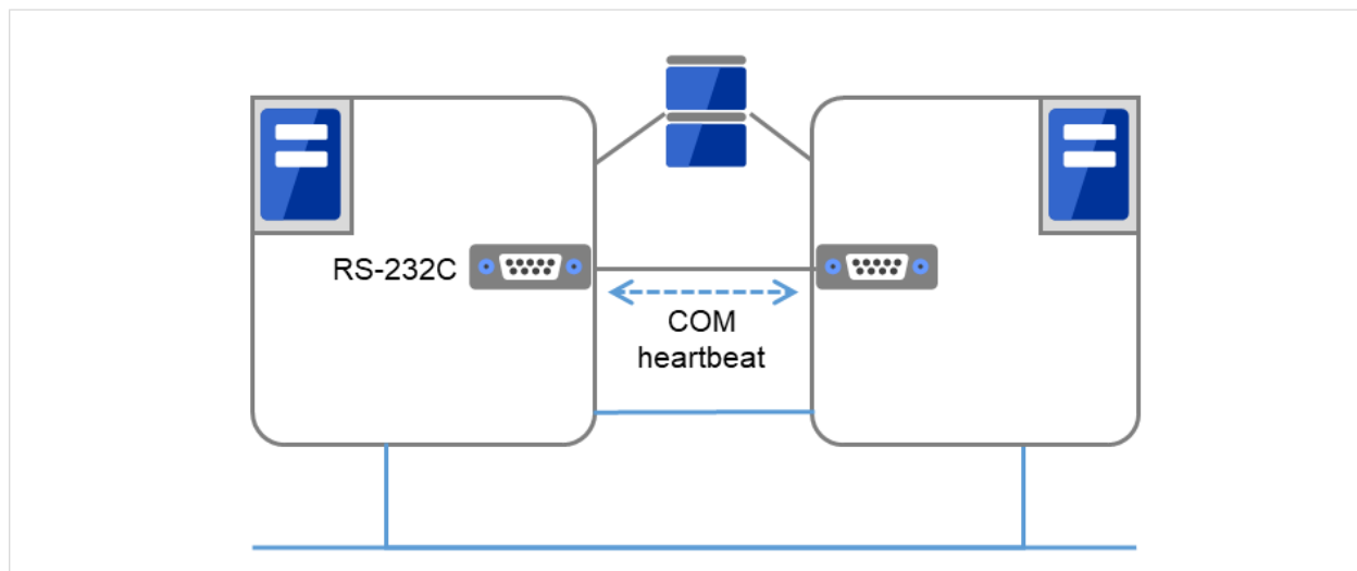
図 3.5 COM ハートビート
