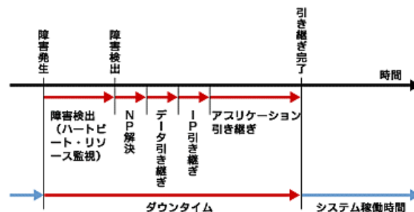
図 2.12 フェイルオーバタイムチャート
