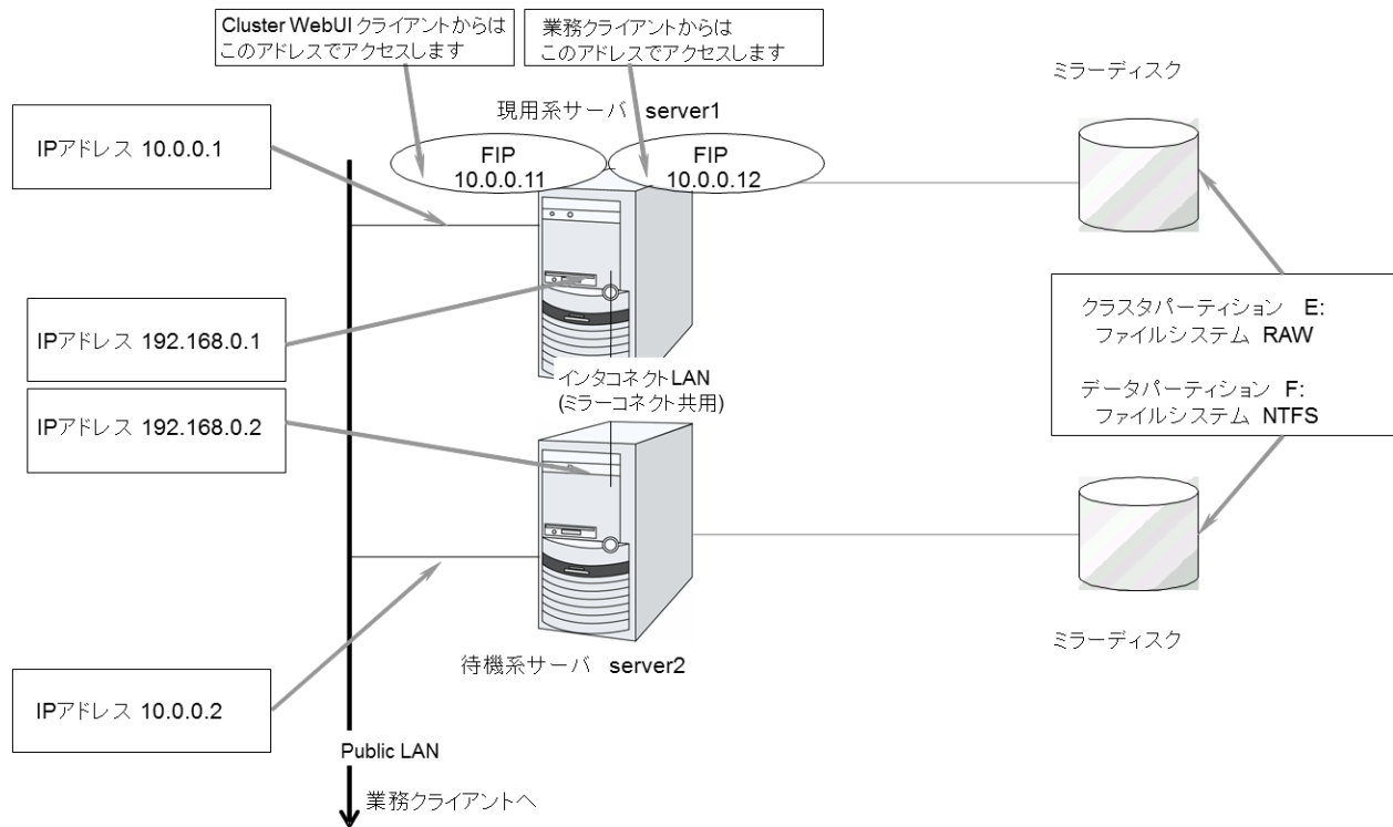
図 3.6 ミラーディスク使用時のクラスタ環境のサンプル
