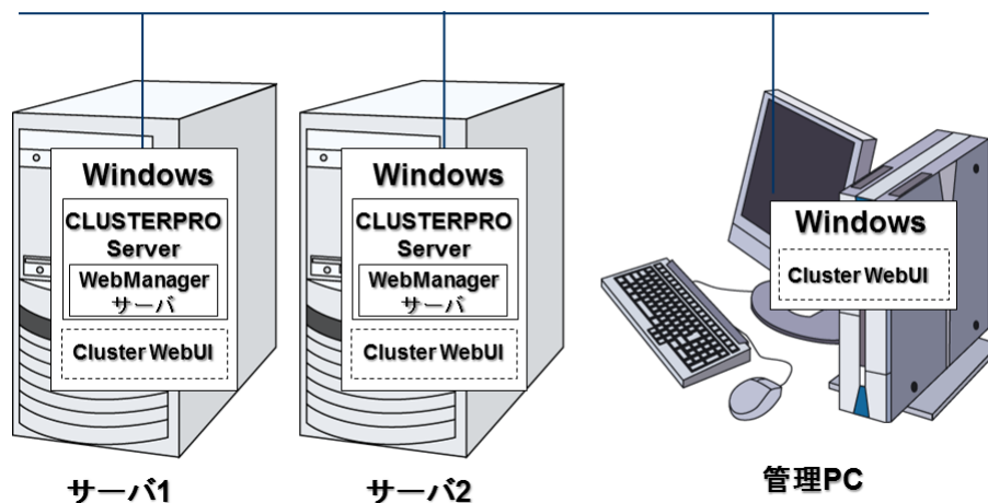
図 3.1 CLUSTERPRO のソフトウェア構成
