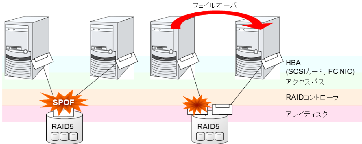
図 2.13 共有ディスクの RAID コントローラとアクセスパスが SPOF となっている例 (左) と RAID コントローラとアクセスパスを分割した例
