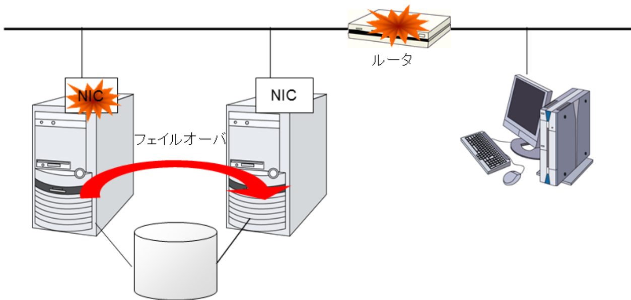
図 2.15 ルータが SPOF となる例
