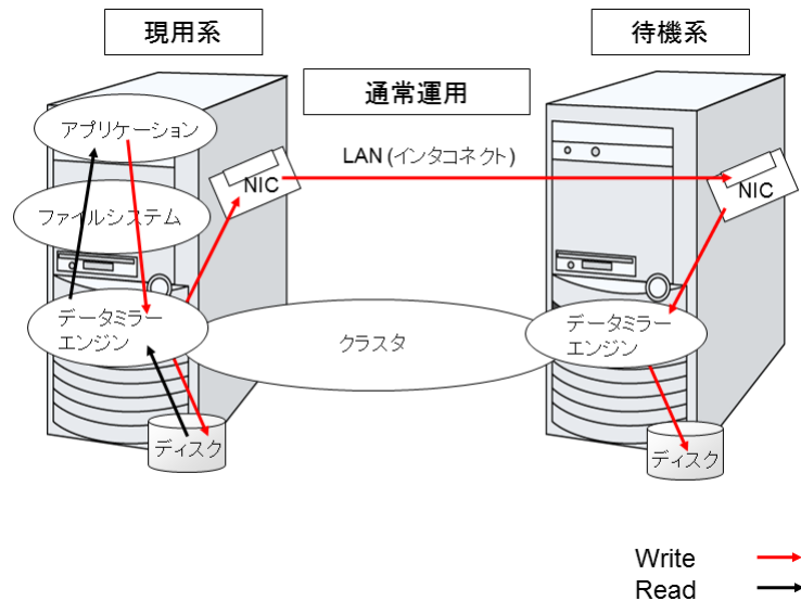
図 2.4 データミラーの仕組み
