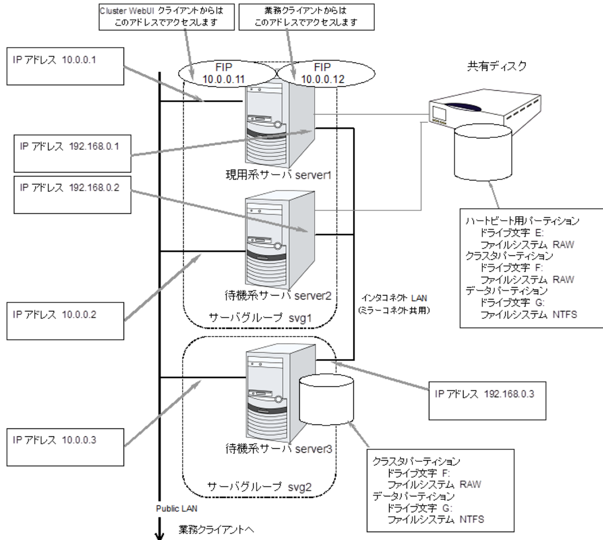
図 3.7 ハイブリッドディスク使用時のクラスタ環境のサンプル
