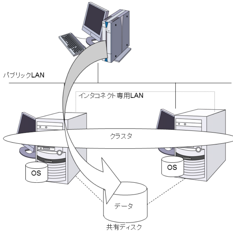
図 2.5 システム構成
