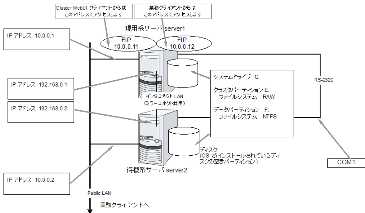
図 3.5 ミラーディスク使用時のクラスタ環境のサンプル
