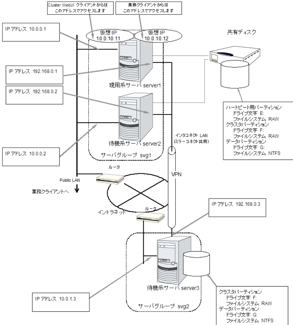
図 3.8 ハイブリッドディスク使用時の遠隔クラスタ環境のサンプル
