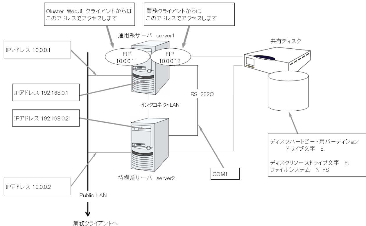
図 3.4 共有ディスク使用時のクラスタ環境のサンプル
