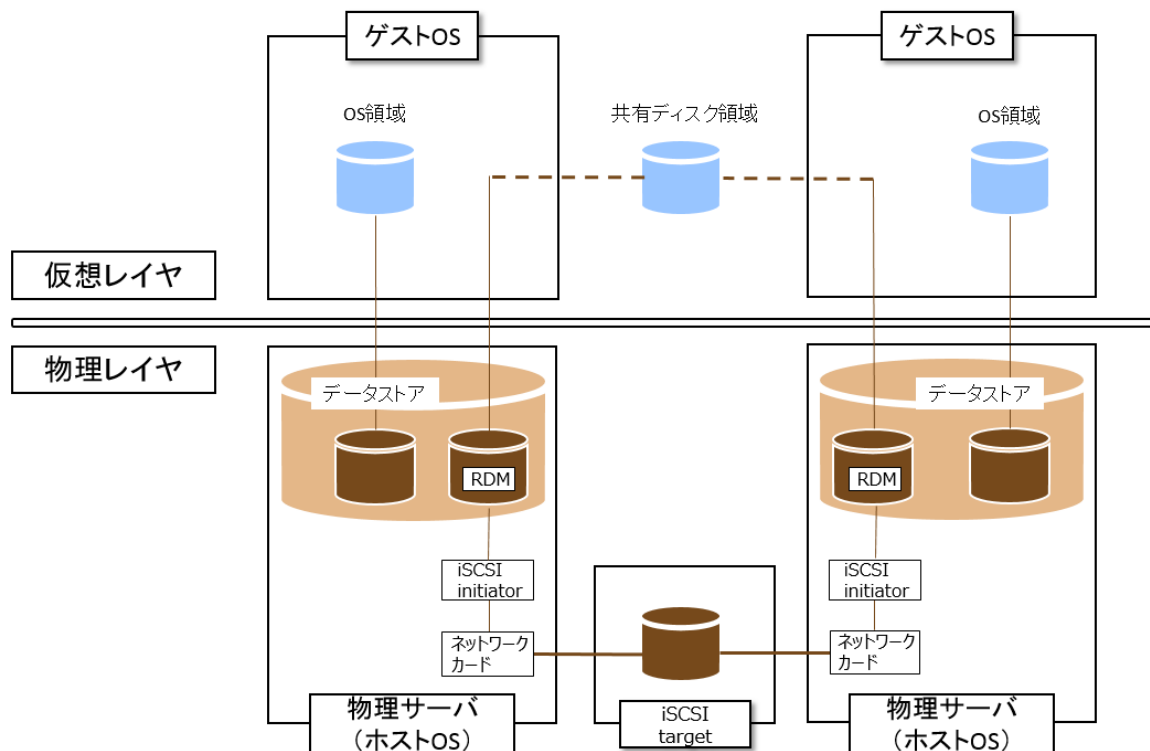
図 5 共有ディスク構成例(iSCSI 接続(ホスト iSCSI) + RDM 接続の場合)
