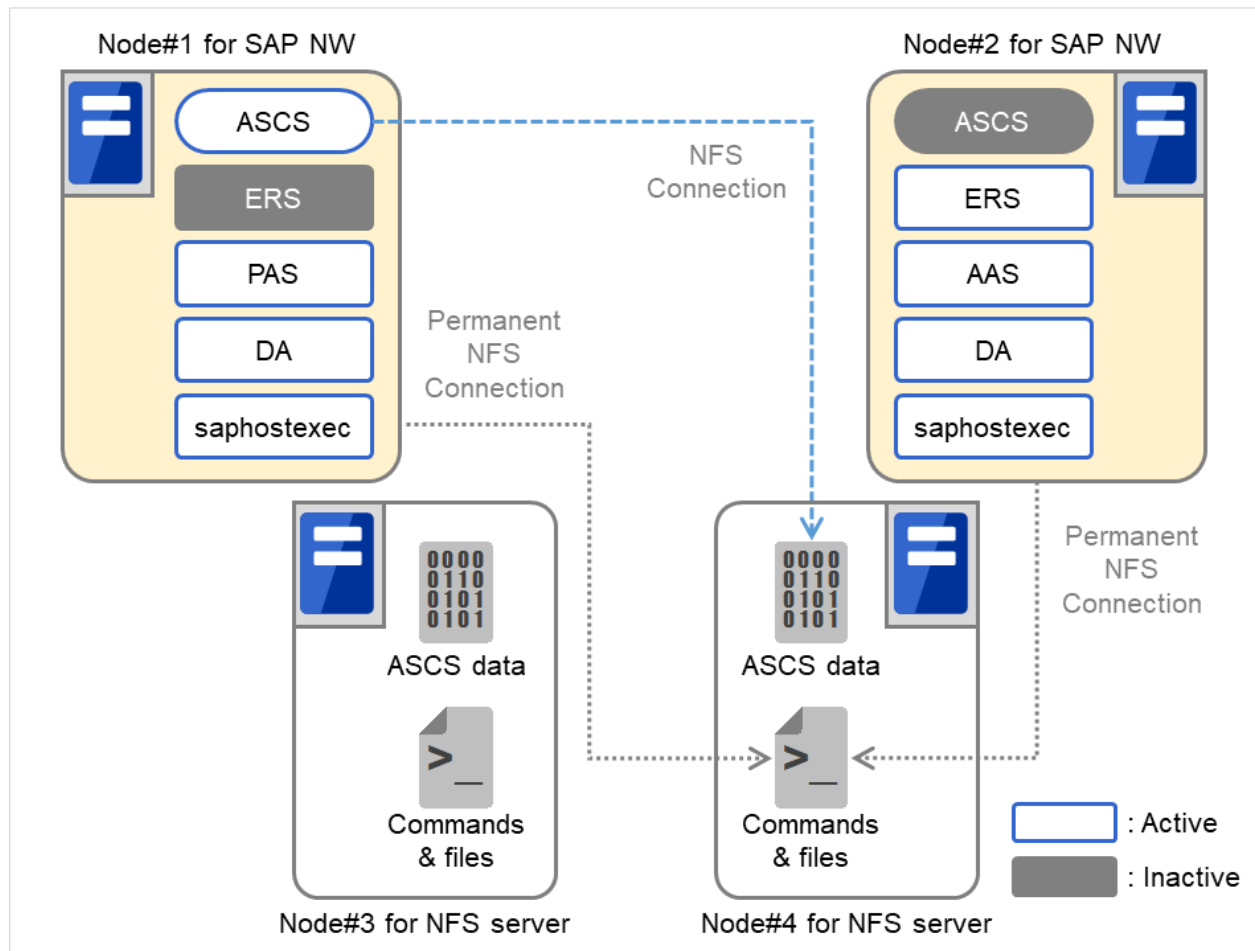
図 3.6 NFS サーバが 2 台の構成、NFS サーバ障害時 (2)
