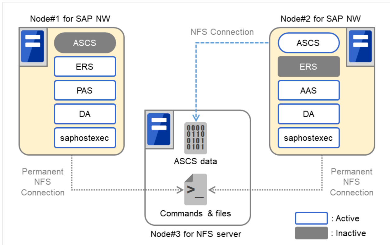
図 3.2 NFS サーバが 1 台の構成 (2)
