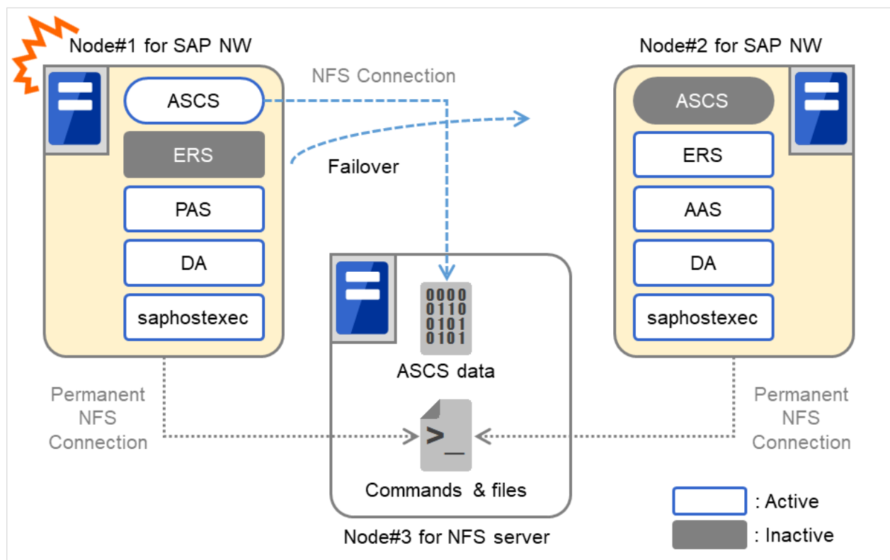
図 3.1 NFS サーバが 1 台の構成 (1)
