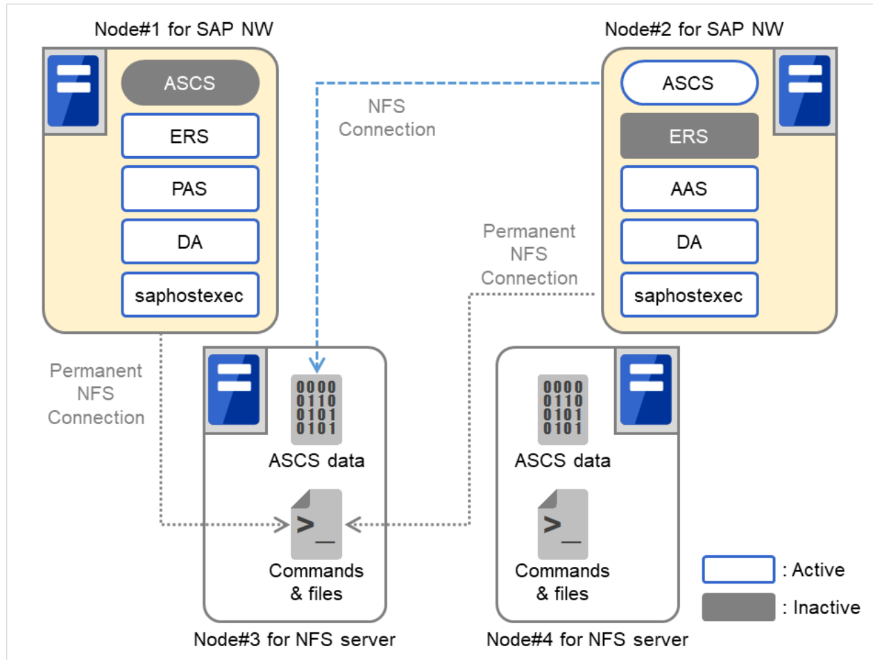
図 3.4 NFS サーバが 2 台の構成、SAP NW サーバ障害時 (2)
