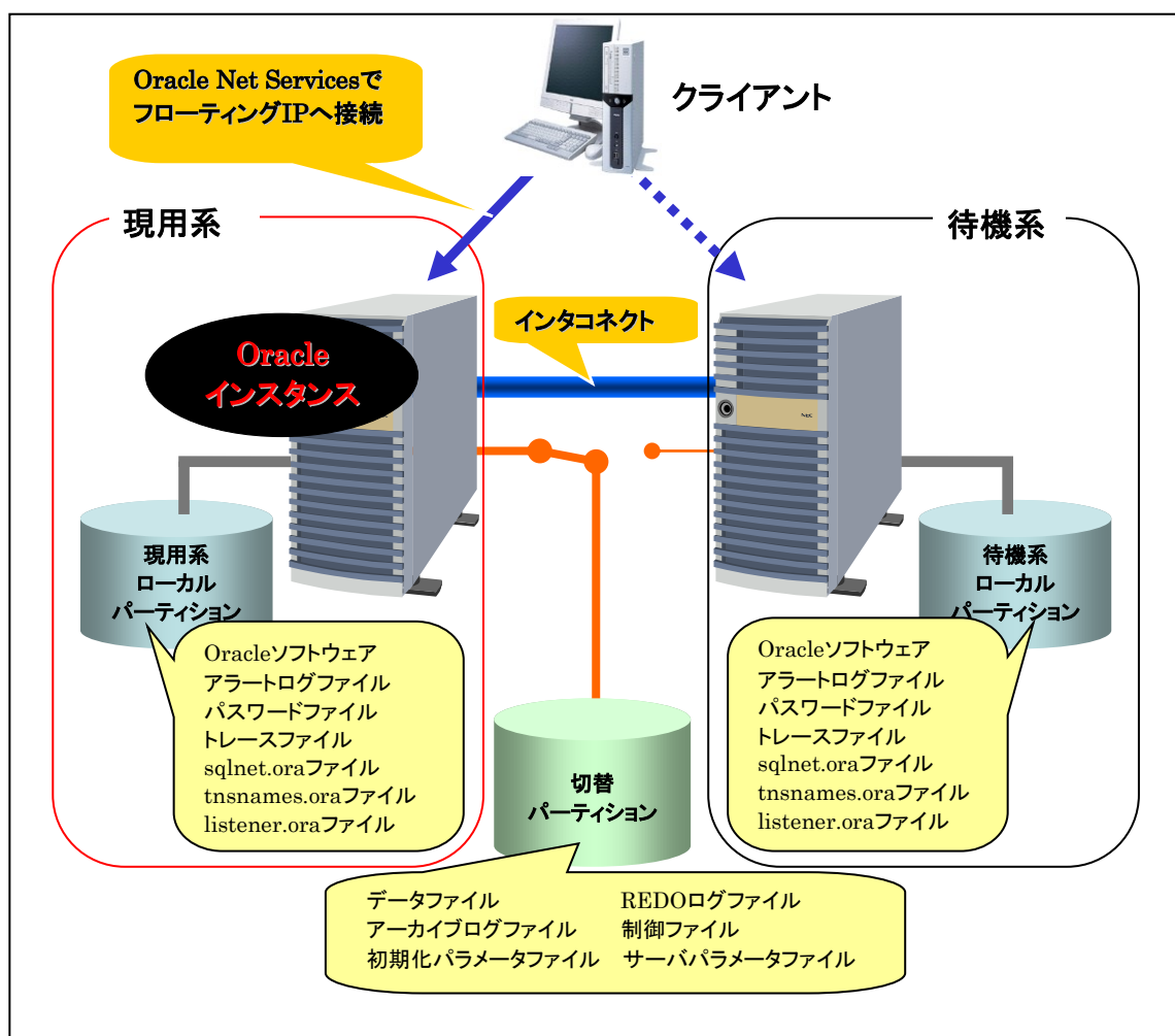
片方向スタンバイの共有ディスク構成イメージ
