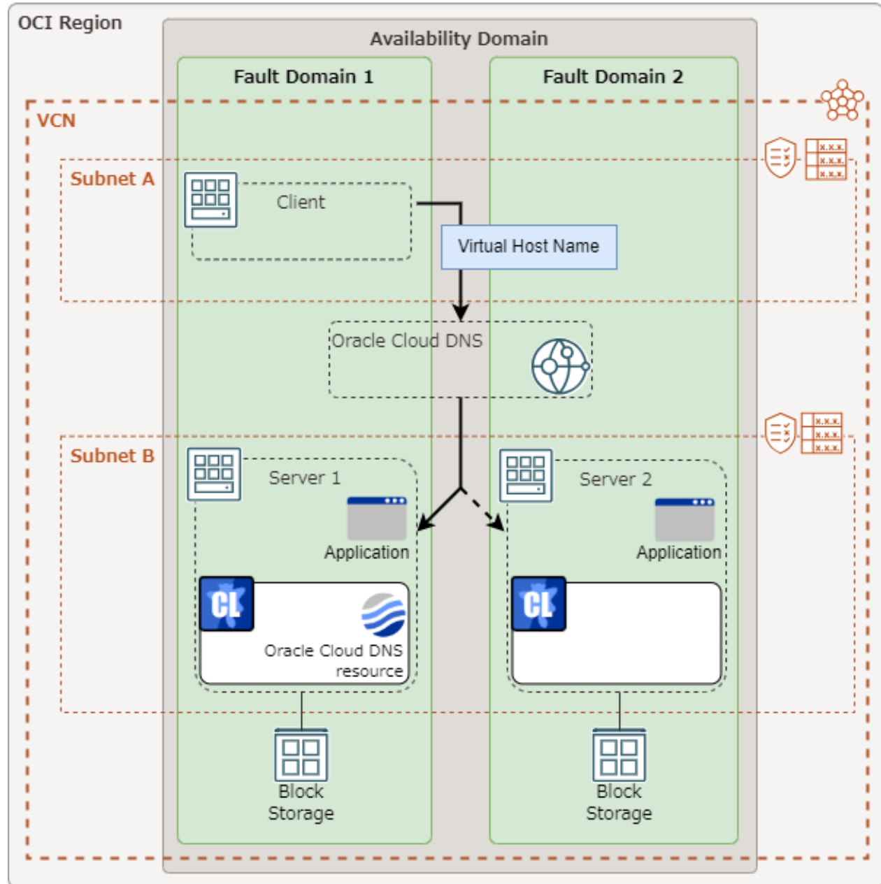
図 2.3 OCI DNS をシングルリージョン環境で使した HA クラスタ
