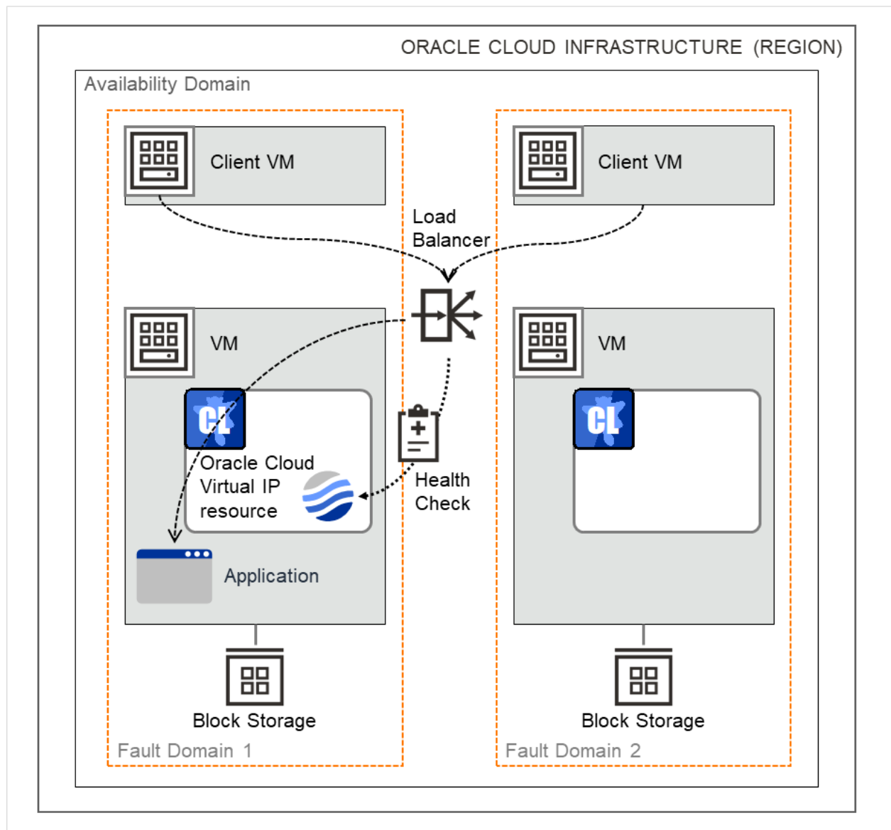
図 2.1 プライベート・ロード・バランサを使用した HA クラスタ
