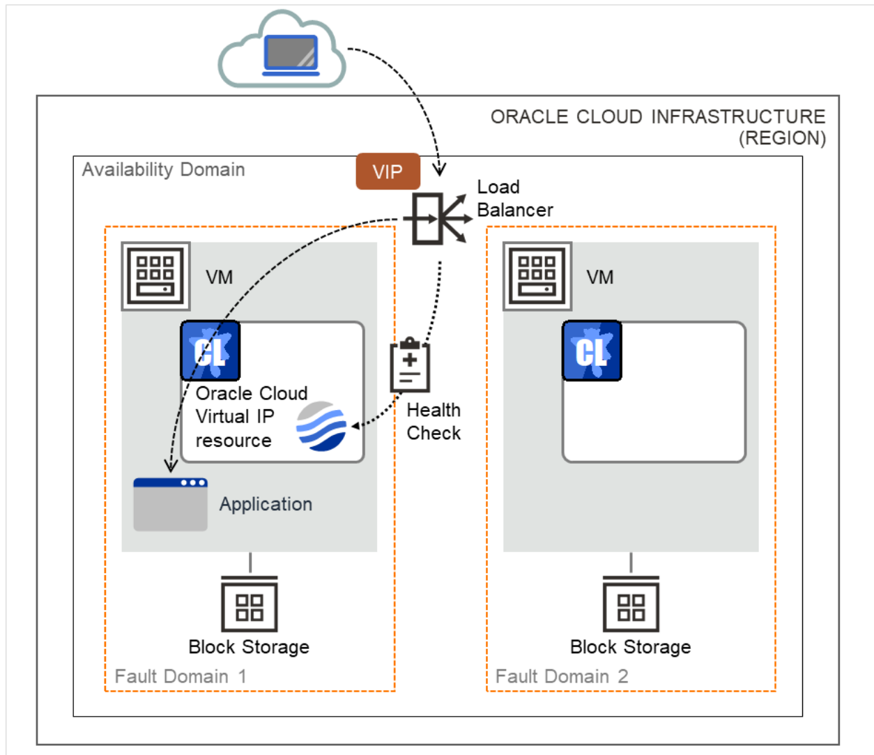
図 2.2 パブリック・ロード・バランサを使用した HA クラスター
