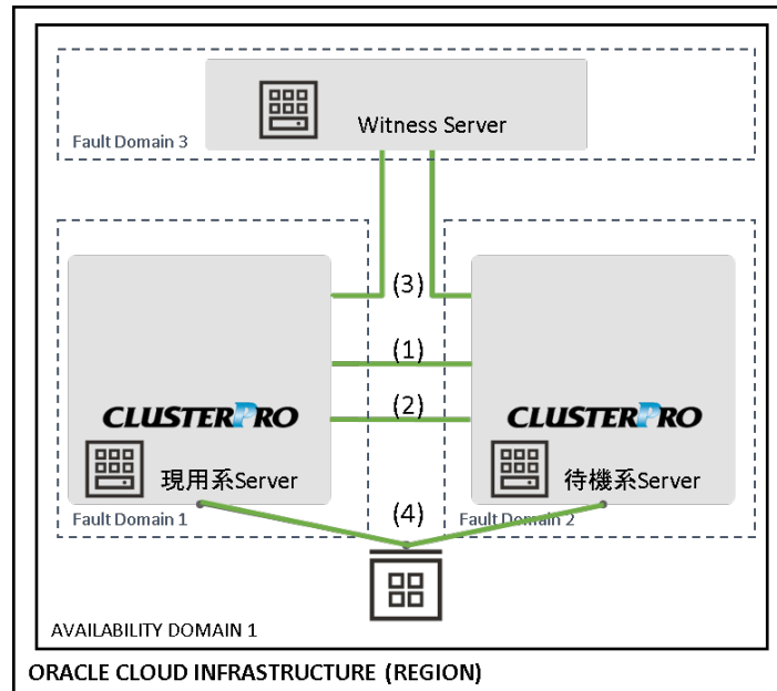
図 2.4 ハートビート 及び NP 解決構成 (共有ディスク型クラスター)
