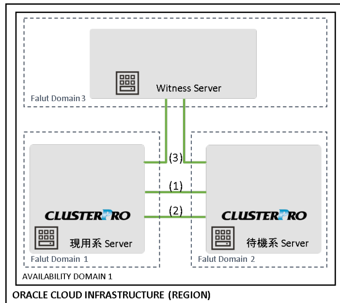
図 2.3 ハートビート 及び NP 解決構成 (ミラーディスク型クラスタ)
