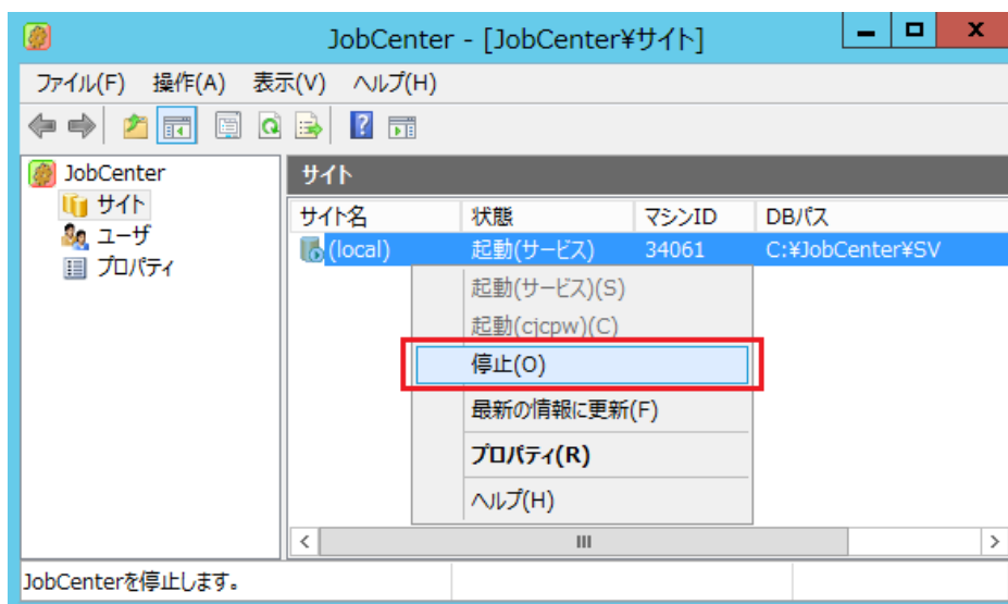
図 3: ローカルサービスの停止
