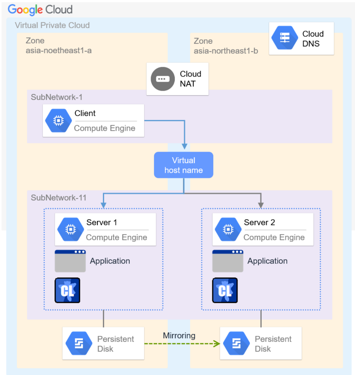
図 2.2 Cloud DNS を使用した HA クラスタ
