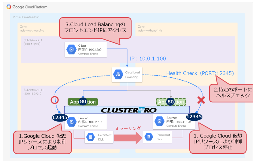
図 2.1 内部 TCP ロードバランサを使用した HA クラスタ
