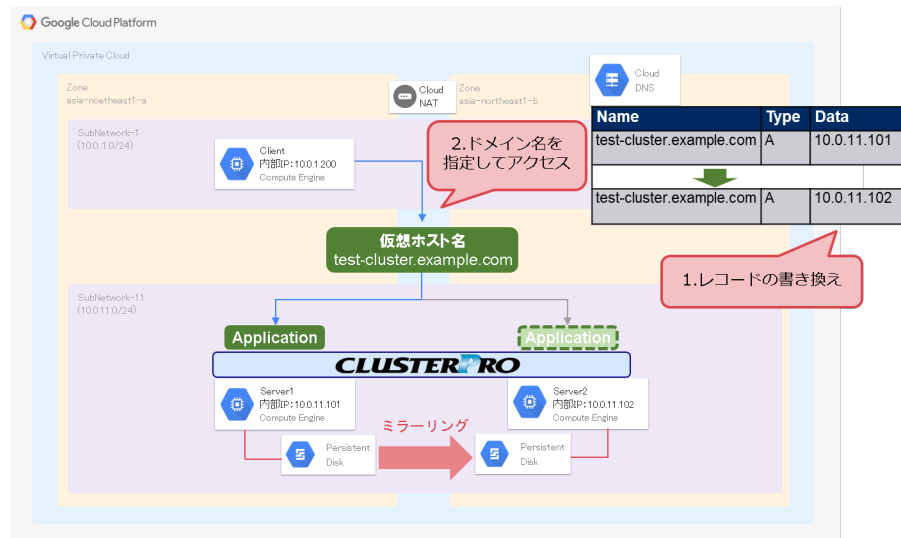
図 2.2 Cloud DNS を使用した HA クラスタ
