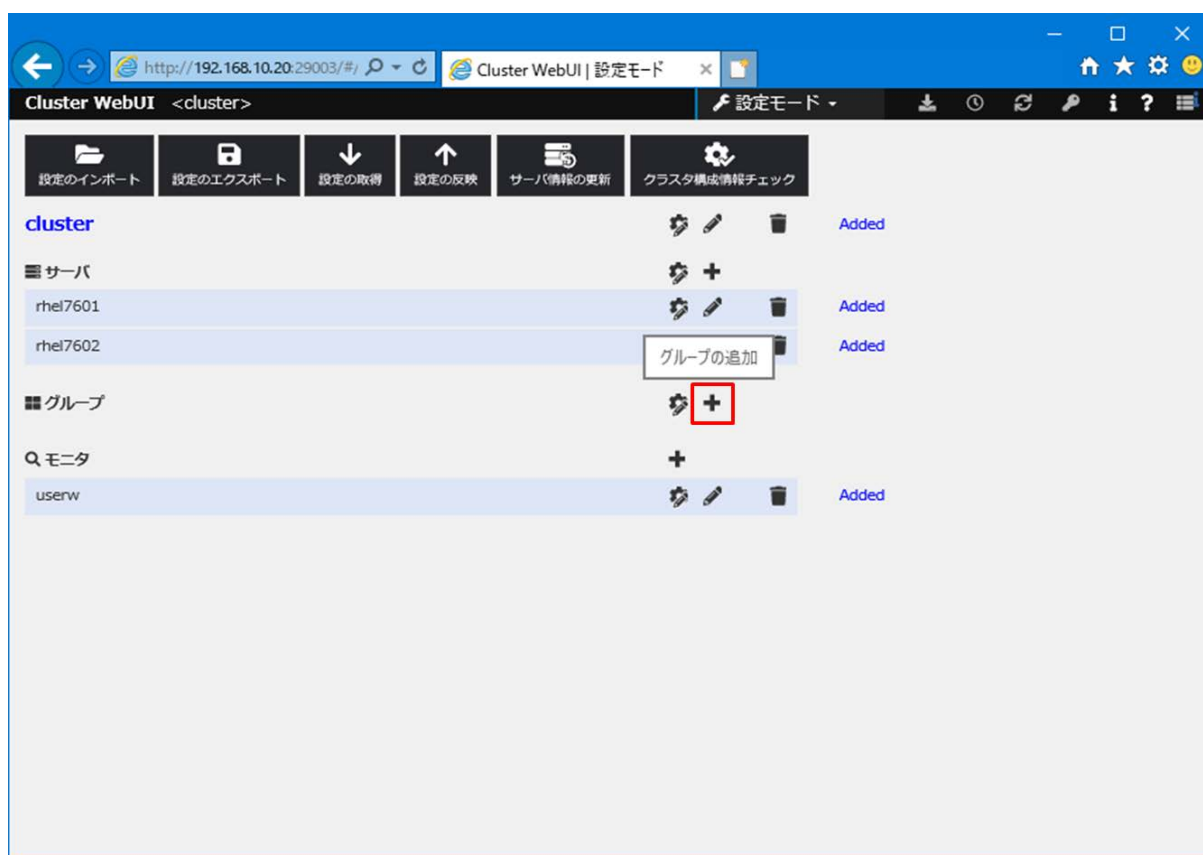
図 3-1-2 Cluster WebUI
