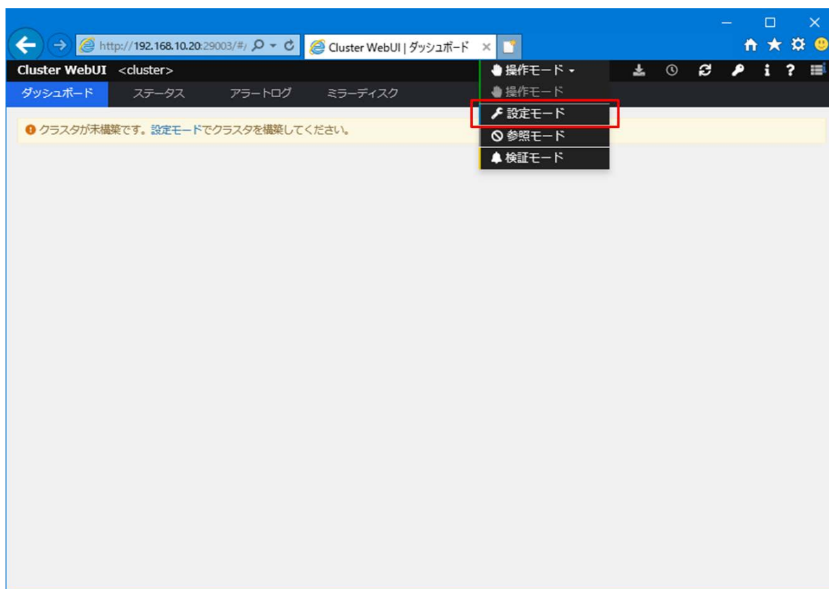
図 3-1-1 Cluster WebUI
