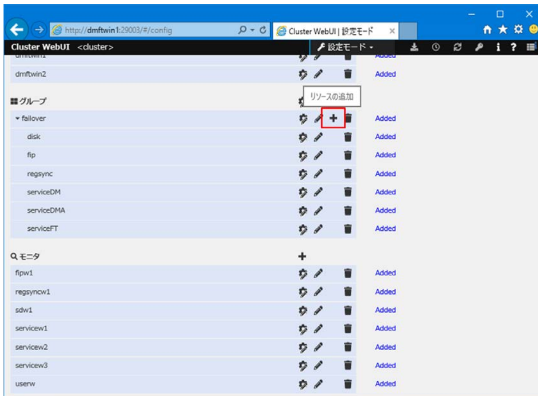
図 4-6-3-1 起動、停止スクリプトの設定
