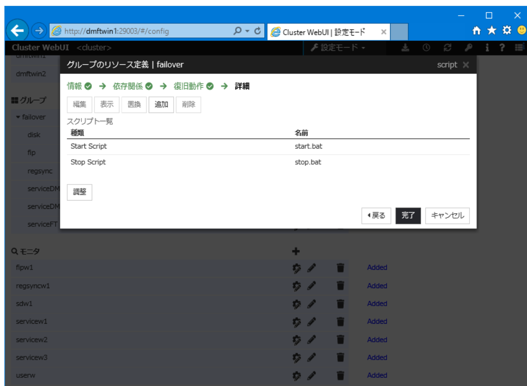
図 4-6-3-5 起動、停止スクリプトの設定
