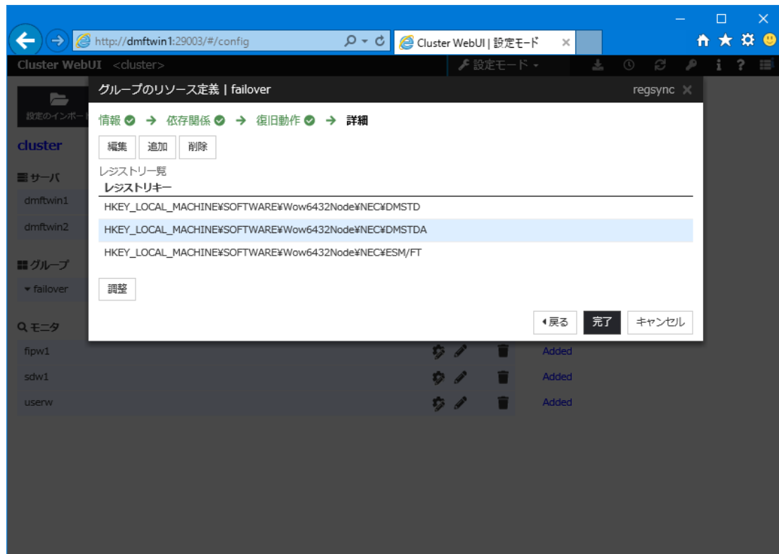
図 4-5-1-7 レジストリ同期リソースの設定
