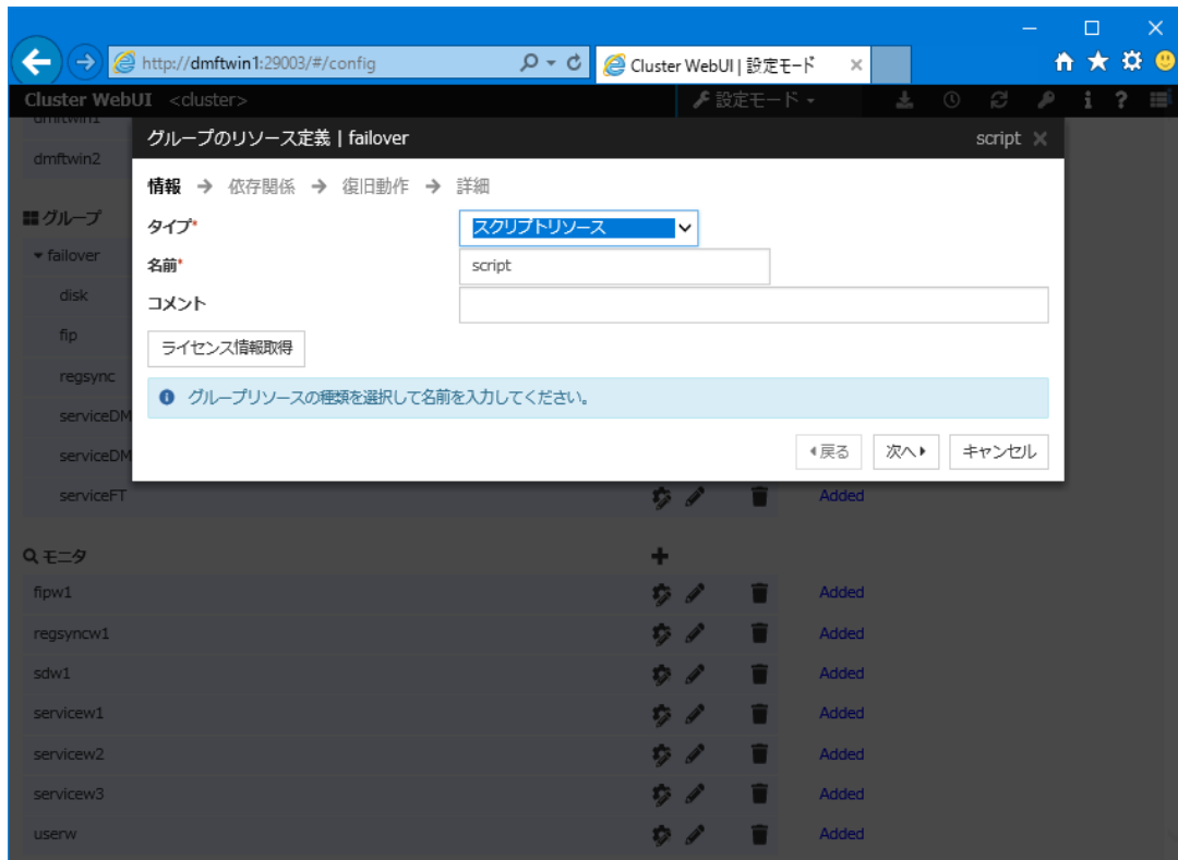
図 4-6-3-2 起動、停止スクリプトの設定
