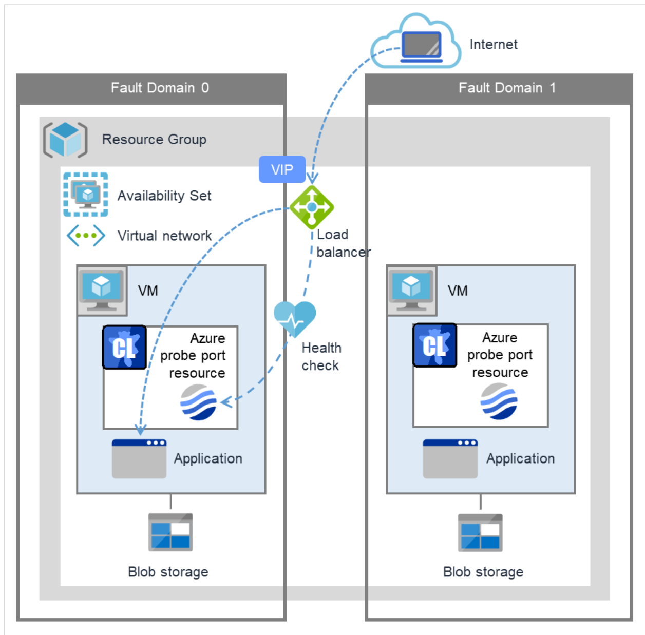
図 2.2 パブリックロードバランサーを使用した HA クラスタ
