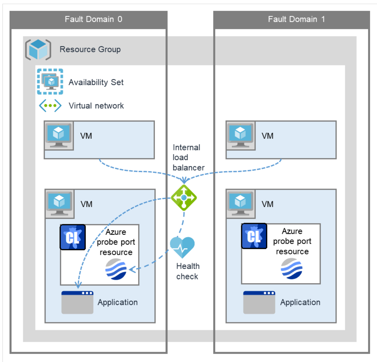
図 2.3 内部ロードバランサーを使用した HA クラスタ
