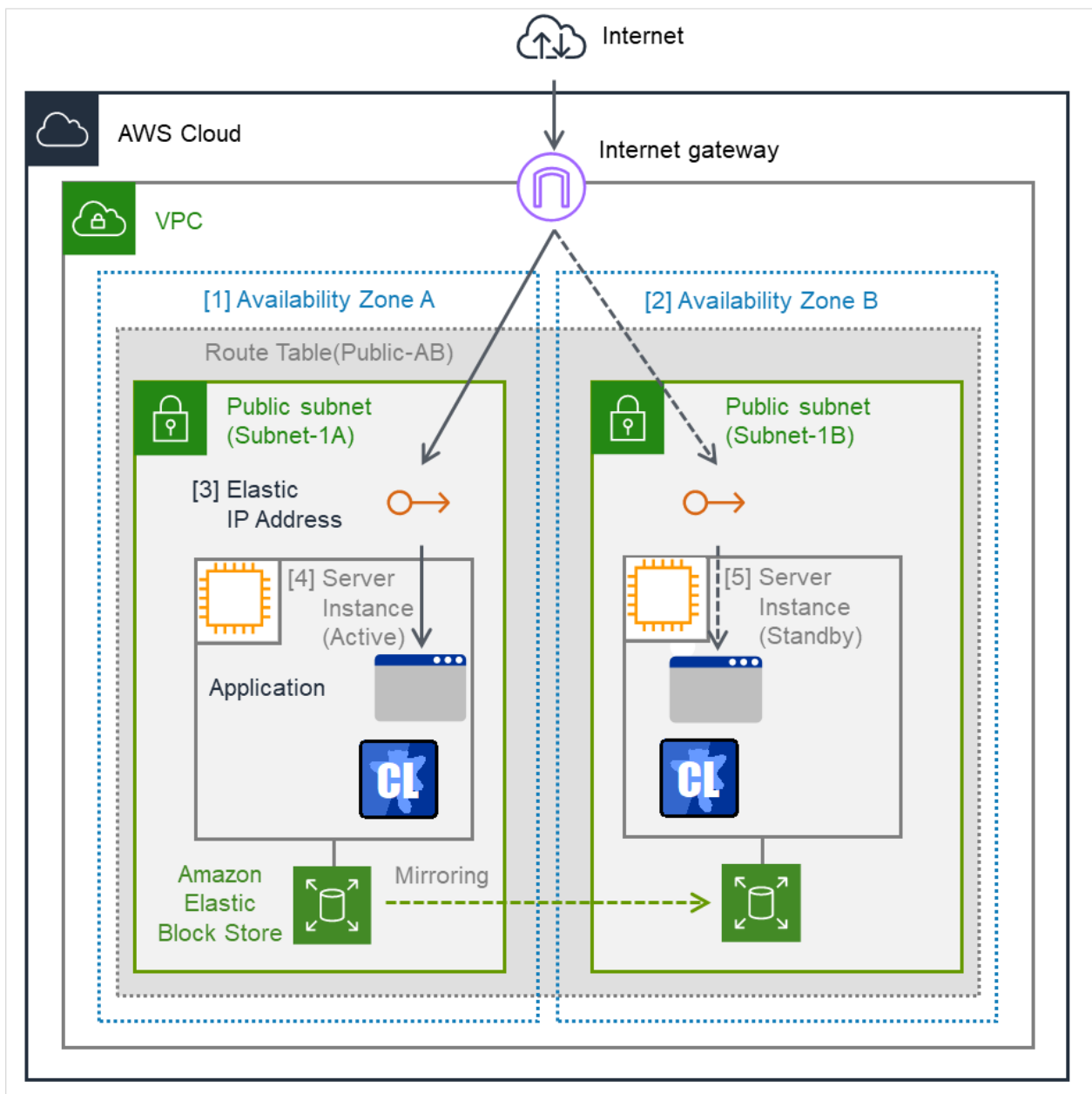
図 5.1 システム構成 EIP 制御による HA クラスター
