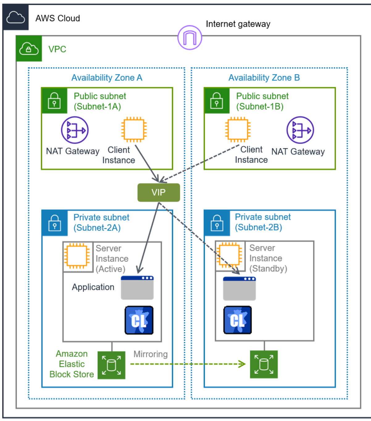
図 2.5 Multi-AZ を使用した HA クラスタの例
