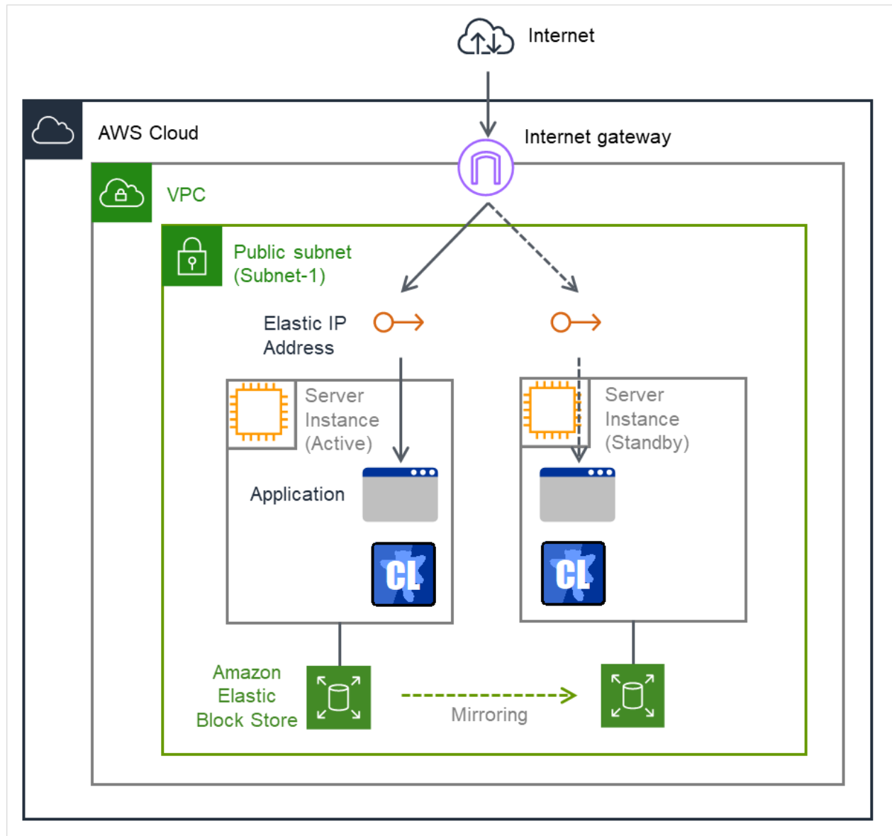
図 2.3 EIP 制御による HA クラスター
