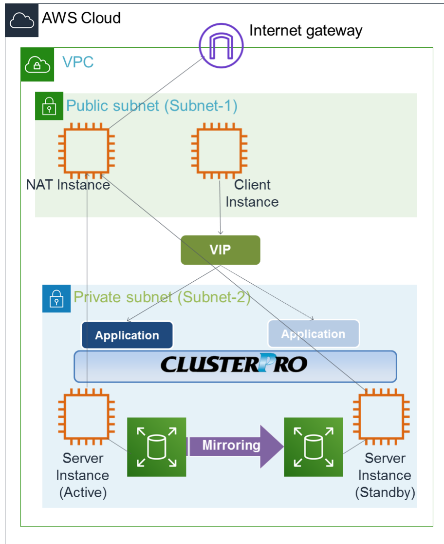
図 2.2 VIP 制御による HA クラスタ
