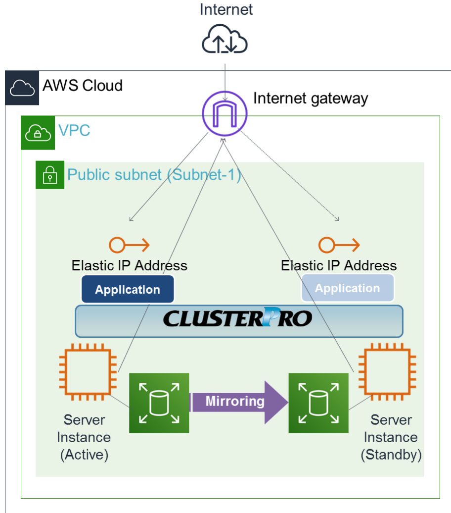
図 2.3 EIP 制御による HA クラスタ
