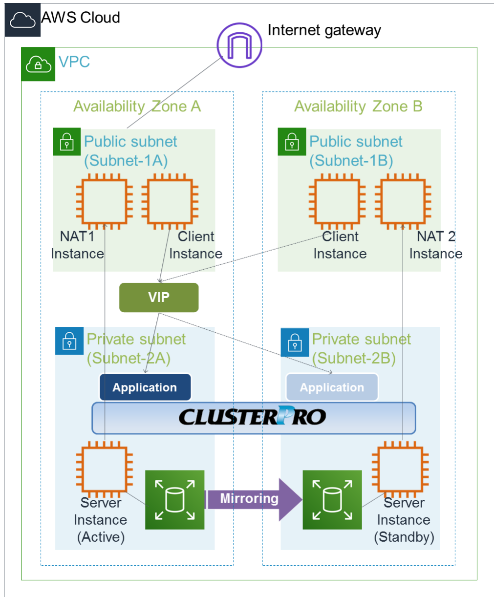
図 2.5 Multi-AZ を使用した HA クラスタの例
