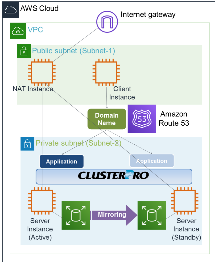
図 2.4 DNS 名制御による HA クラスタ
