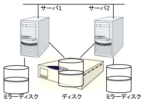
ディスクリソースとミラーディスクリソース
