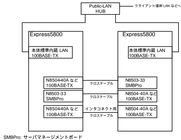
接続例 2(NEC 製品構成例)
