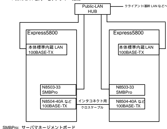
接続例 1(NEC 製品構成例)
