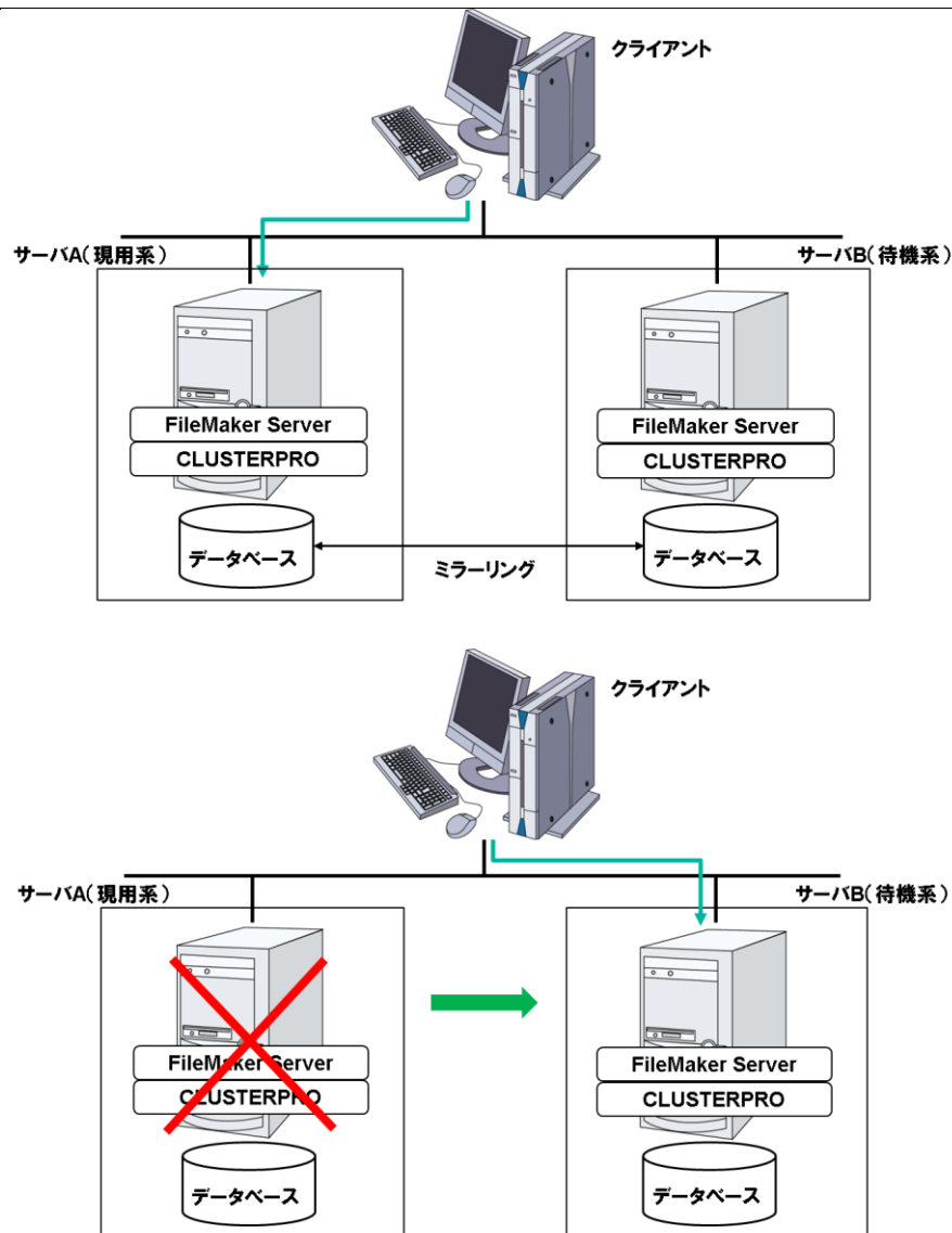
図1-2. ミラーディスク型クラスタ 概要図
