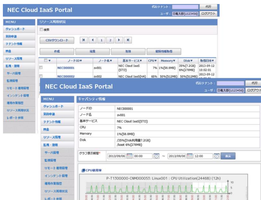
図 3 監視状況画面例
