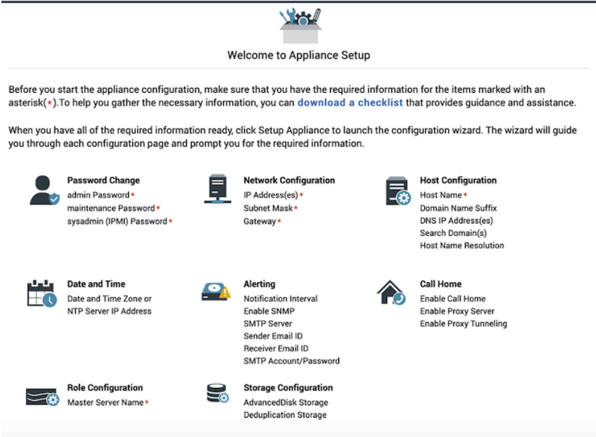
図 1-1 アプライアンスの設定へようこそ (Welcome to Appliance Setup)
