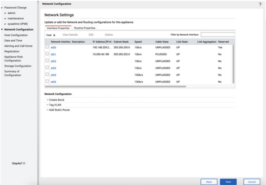
図 1-3 [ネットワーク構成 (Network Configuration)]ページ
