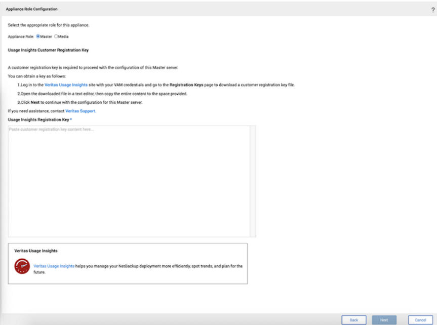
図 1-8 [アプライアンスの役割の構成 (Appliance Role Configuration)] - [プライマリ (Primary)] ページ
