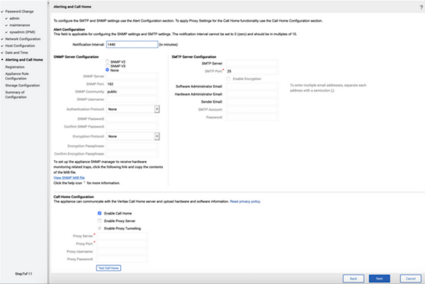
図 1-6 [警告とコールホーム (Alerting and Call Home)]ページ
