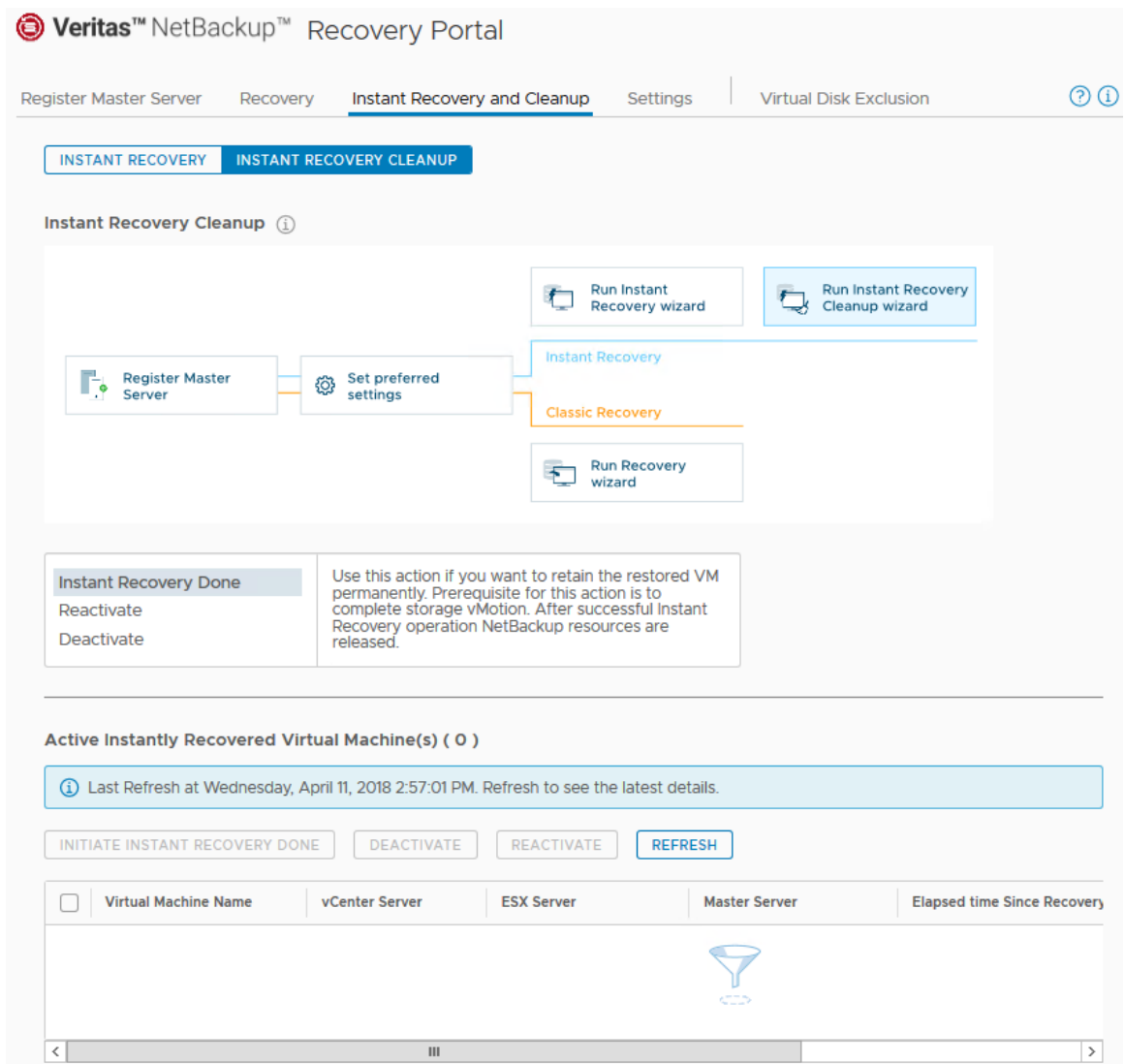
図 5-16 [インスタントリカバリのクリーンアップ (Instant Recovery Cleanup)] 画面
