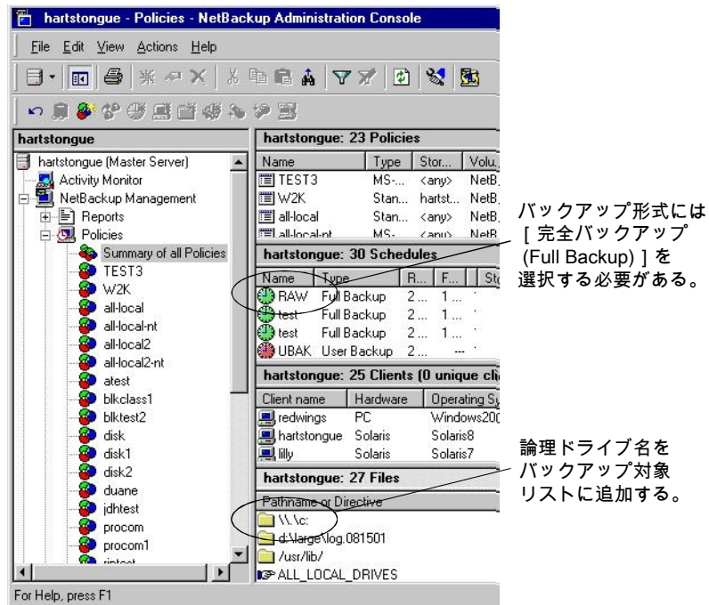
図 21-23 ディスクイメージのバックアップ
