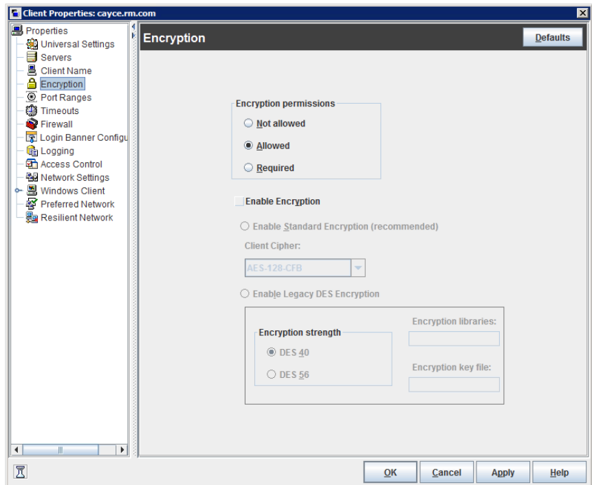
図 3-15 [暗号化 (Encryption)]ダイアログボックス
