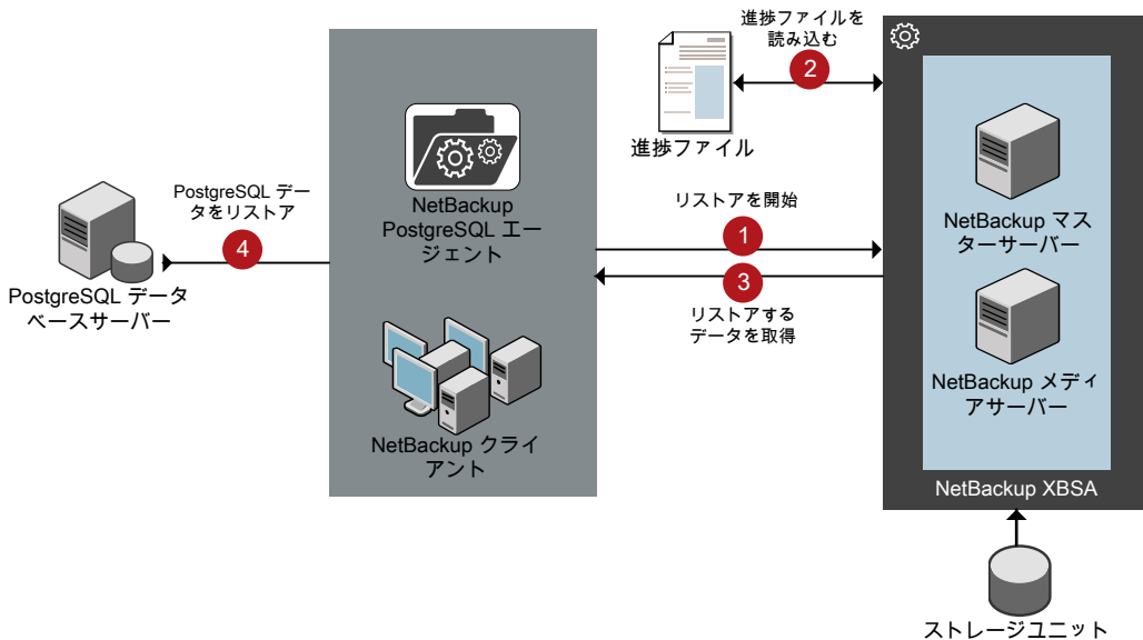
図 4-2 NetBackup for PostgreSQL のリストアのワークフロー
