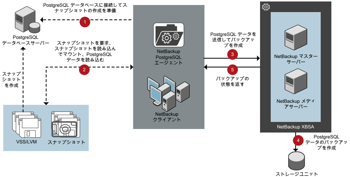
図 4-1 NetBackup for PostgreSQL のバックアップのワークフロー
