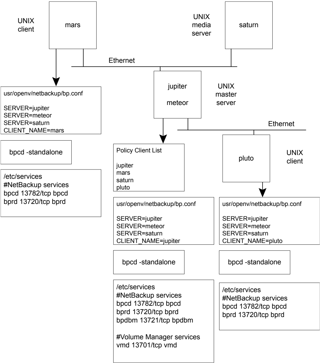
図 2-4 複数のネットワークに接続する UNIX サーバー
