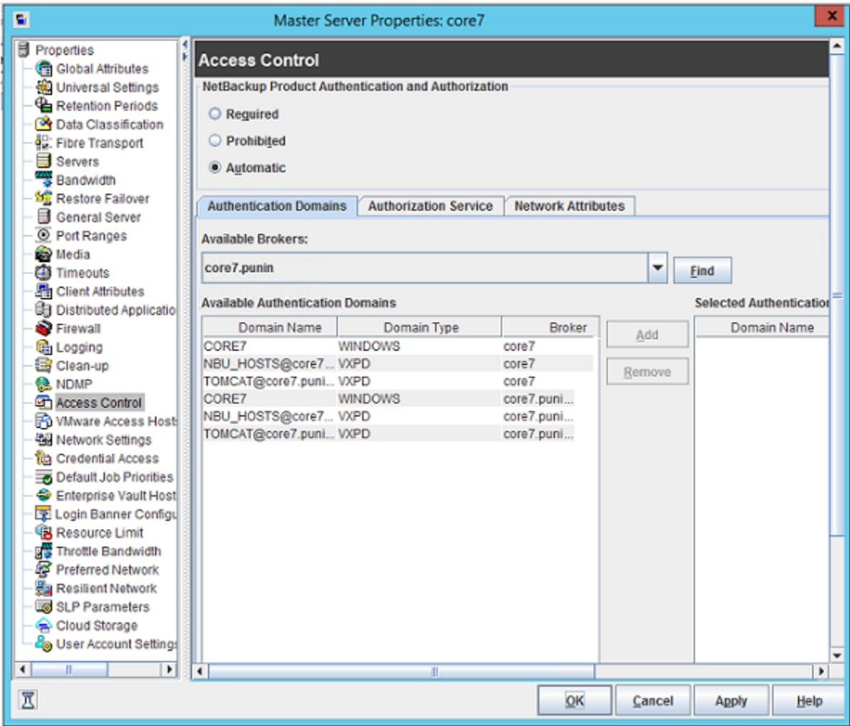
図 6-5 クロスプラットフォームの認証ドメイン
