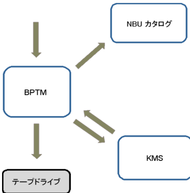
図 12-1 暗号化テープへの書き込み処理の流れ
