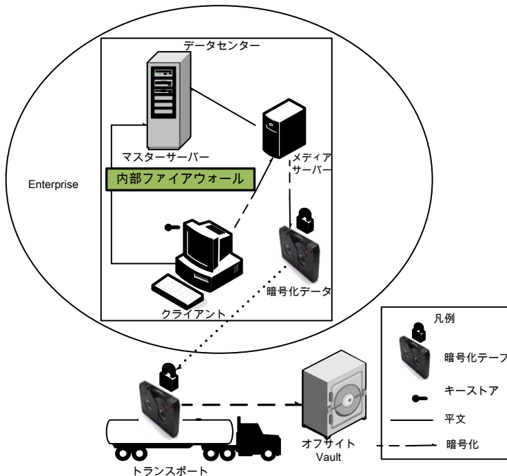
図 1-6 クライアント側の暗号化
