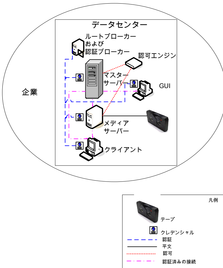
図 1-8 すべてに NBAC を使用
