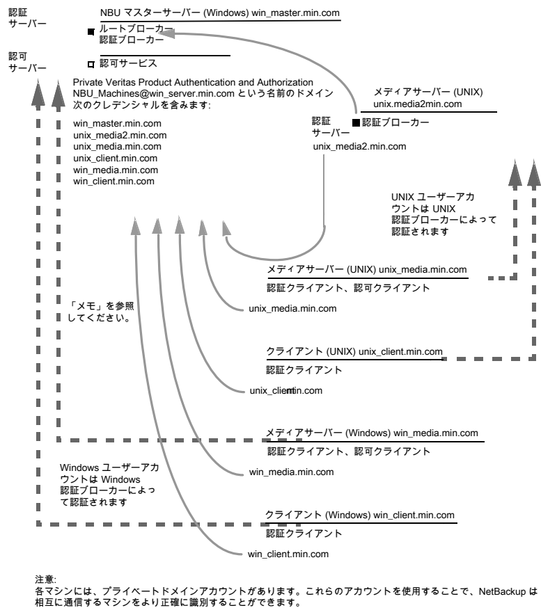
図 6-6 Windows マスターサーバーが存在する複合構成の例
