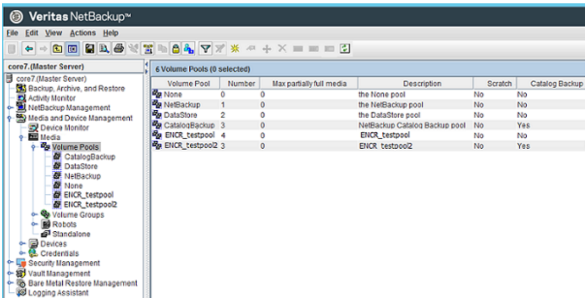
図 12-3 KMS を使用するための 2 つのボリュームプールの設定が表示された NetBackup 管理コンソール
