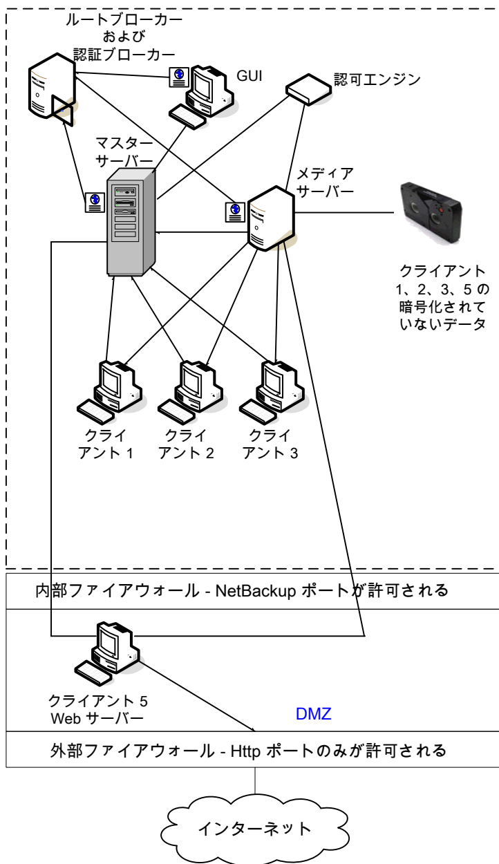
図 2-4 マスターサーバーとメディアサーバーで NBAC を使用する単一のデータセンター
