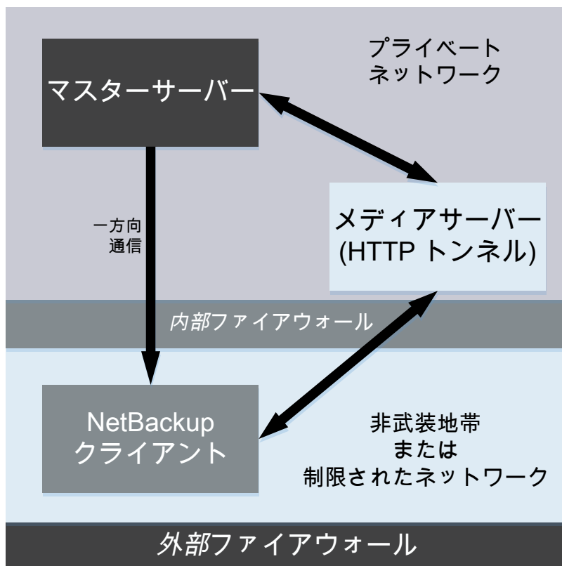
図 8-2 DMZ 設定での NetBackup クライアントとマスターサーバーの通信
