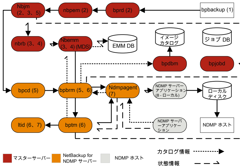
図 6-1 NDMP バックアップ処理
