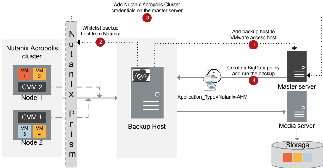
図 3-1 NetBackup と Nutanix AHV の間の通信チャンネル
