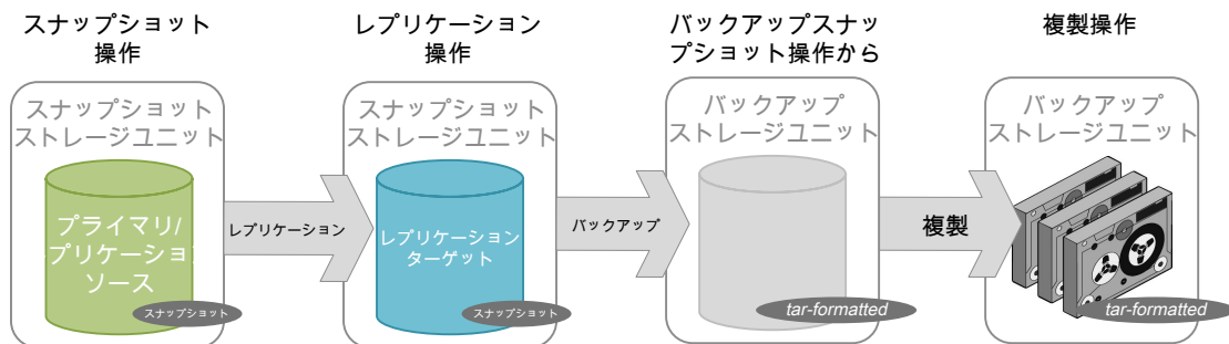
図 6-5 スナップショット操作、レプリケーション操作、スナップショットからのバックアップ操作、および複製操作を含む SLP
