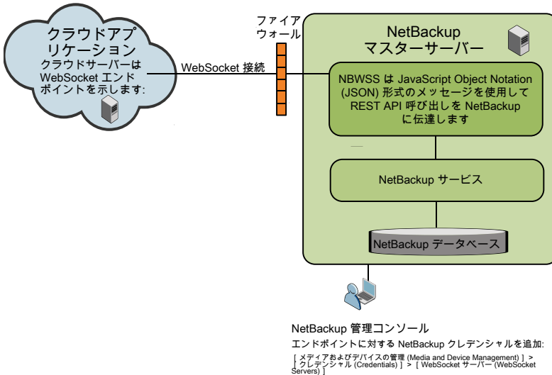
図 1-1 NBWSS の概要
