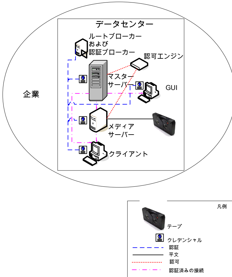
図 1-9 すべての NBAC を使用
