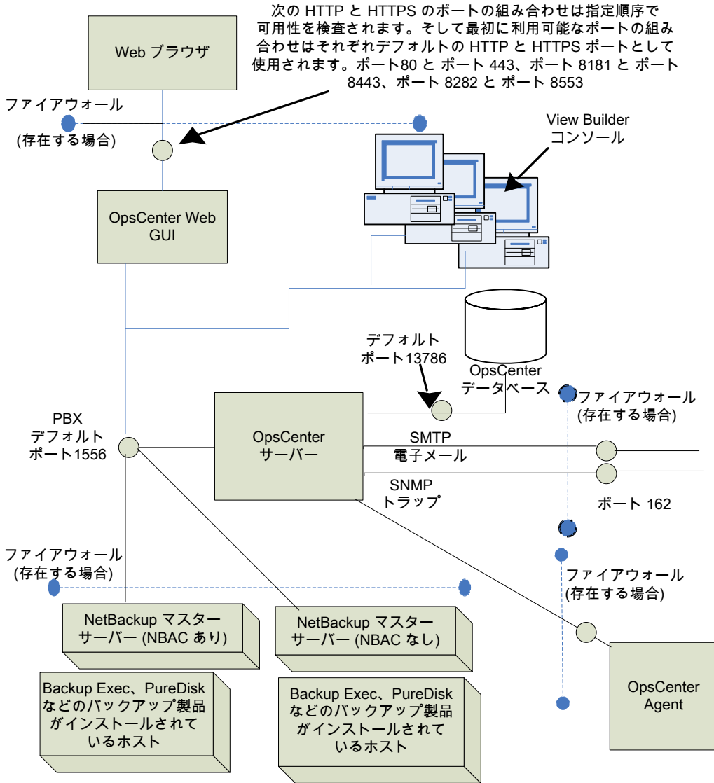
図 3-1 NetBackup の主要なコンポーネントと通信方法
