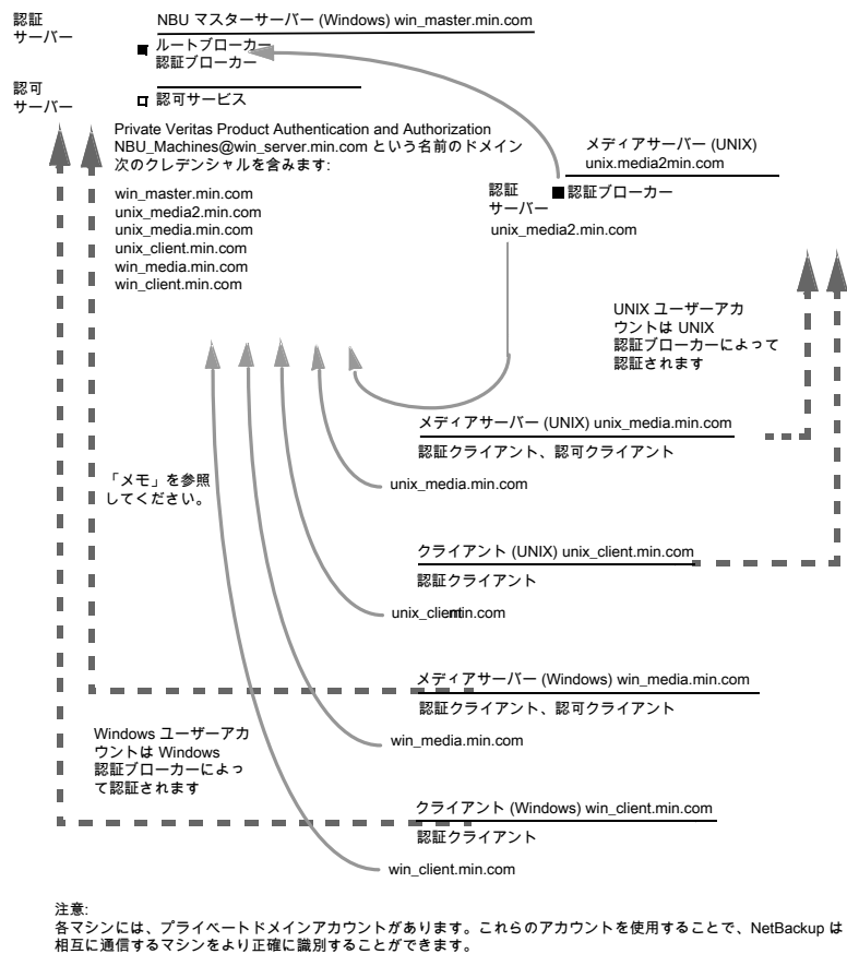
図 6-12 Windows マスターサーバーが存在する複合構成の例
