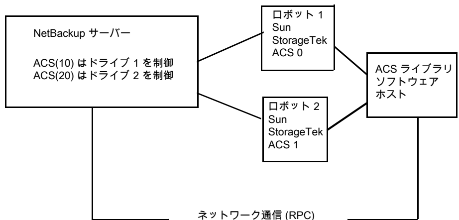
図 8-4 複数の ACS ロボット、1 台の ACS ライブラリソフトウェアホスト
