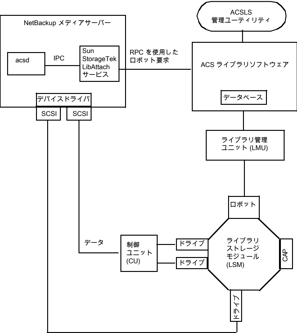
図 8-2 一般的な ACSLS 構成 (Windows の場合)
