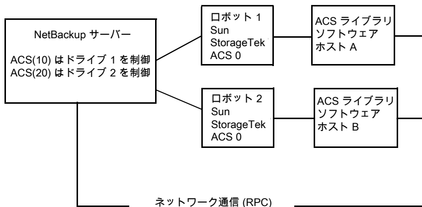
図 8-5 複数の ACS ロボット、複数の ACS ライブラリソフトウェアホスト
