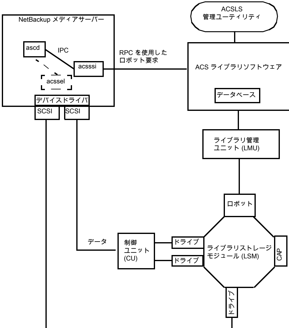
図 8-1 一般的な ACSLS 構成 (UNIX の場合)
