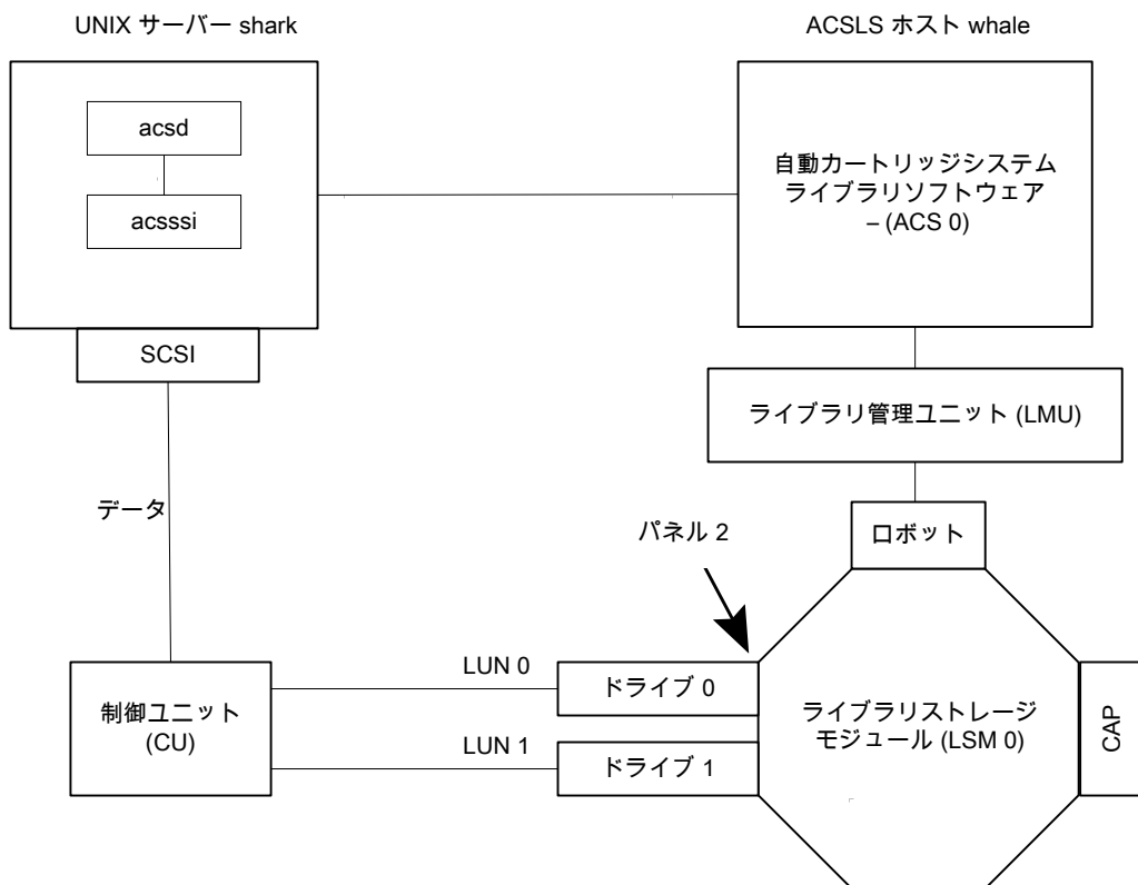
図 9-2 UNIX サーバーおよび ACS ロボットの構成例
