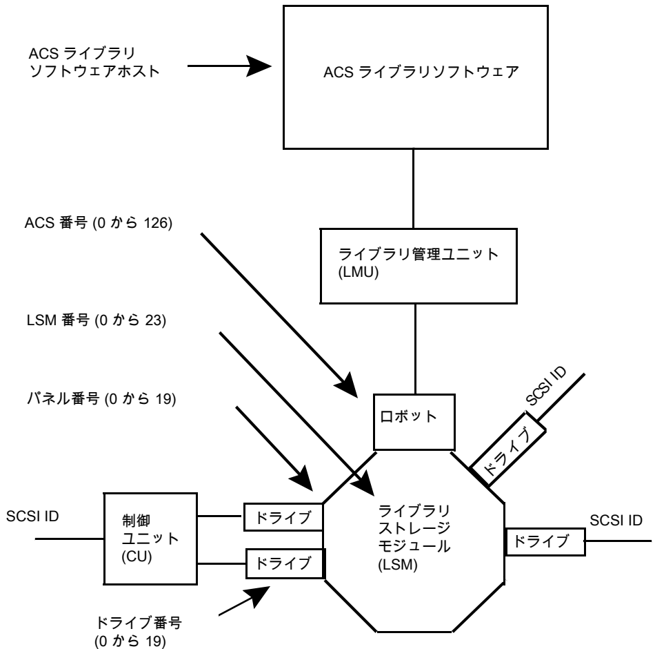
図 8-3 ACSLS ロボットおよびドライブの構成情報
