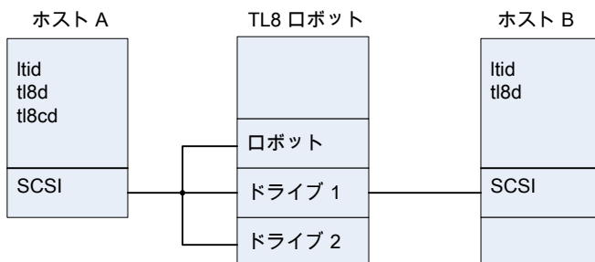
図 A-4 TL8 ロボットに接続した 2 台のホストでの t18cd の使用
