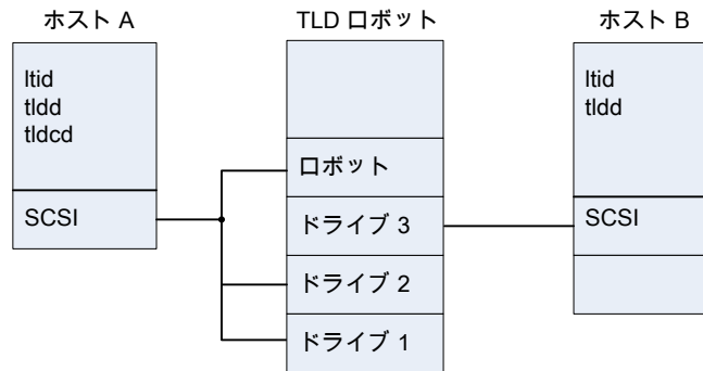
図 A-6 TLD ロボットに接続した 2 台のホストでの tidd の使用
