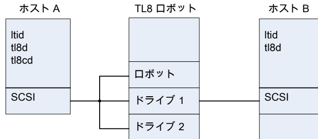
図 A-2 TL8 ロボットに接続した 2 台のホストでの t18d の使用
