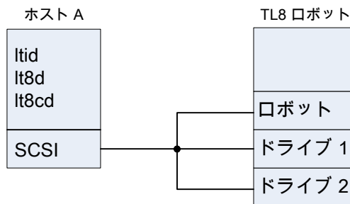
図 A-1 TL8 ロボットに接続した 1 台のホストでの t18d の使用
