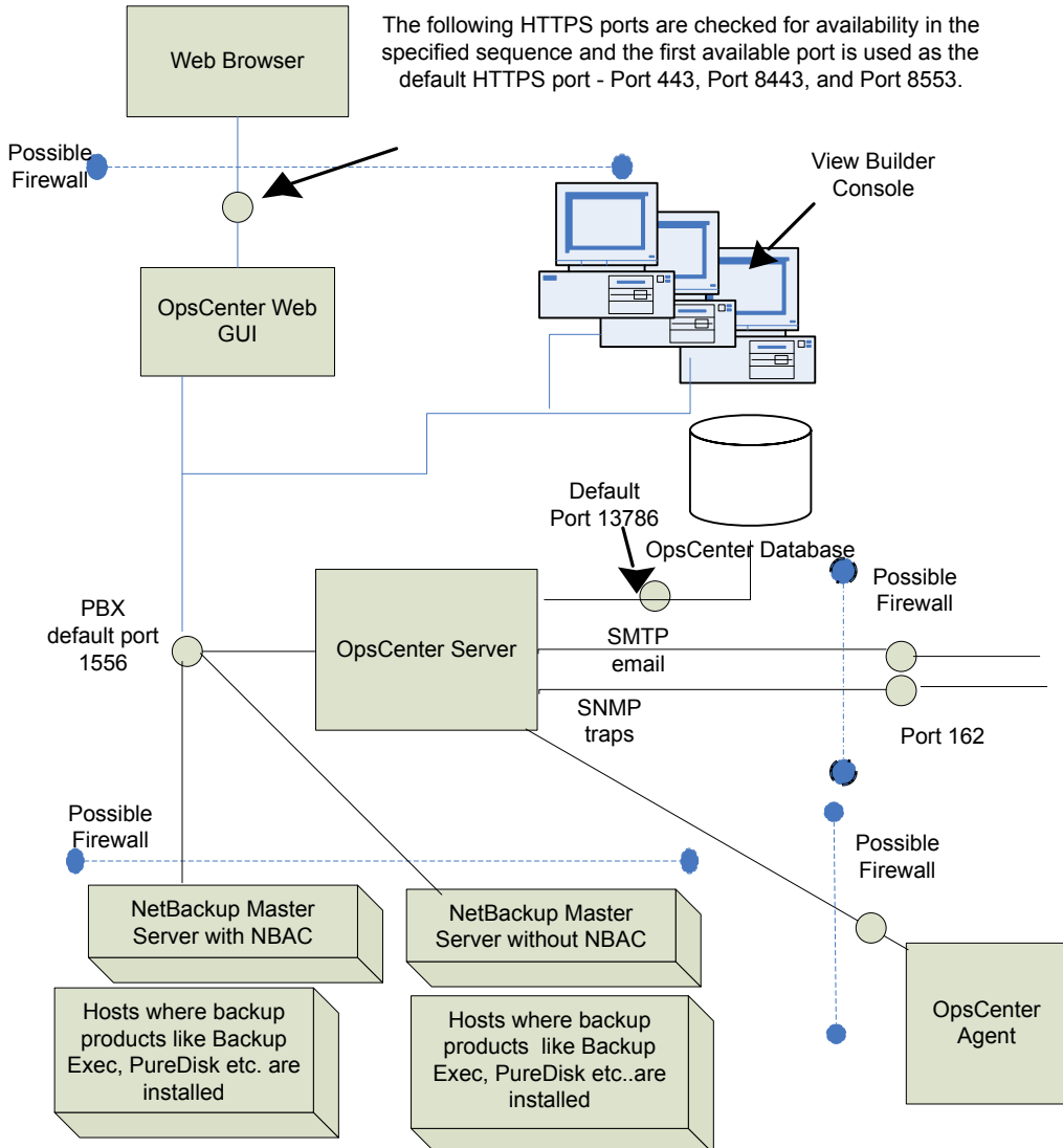
図 4-1 OpsCenter の主要なコンポーネントと通信方法
