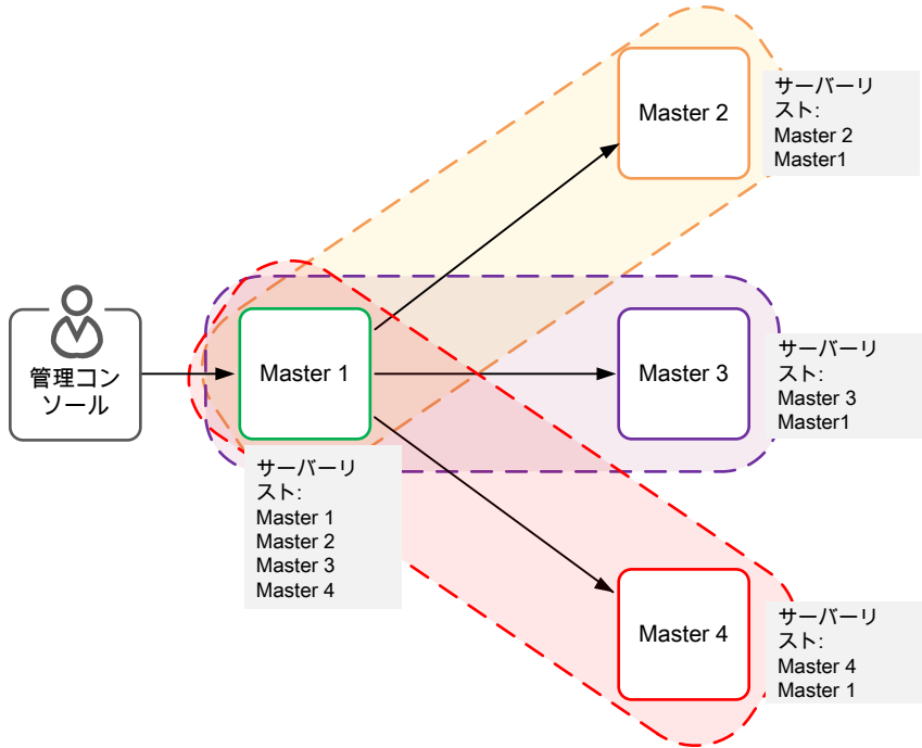
図 30-4 制限された[サーバーの変更 (Change Server)]機能を提供する制限モデル
