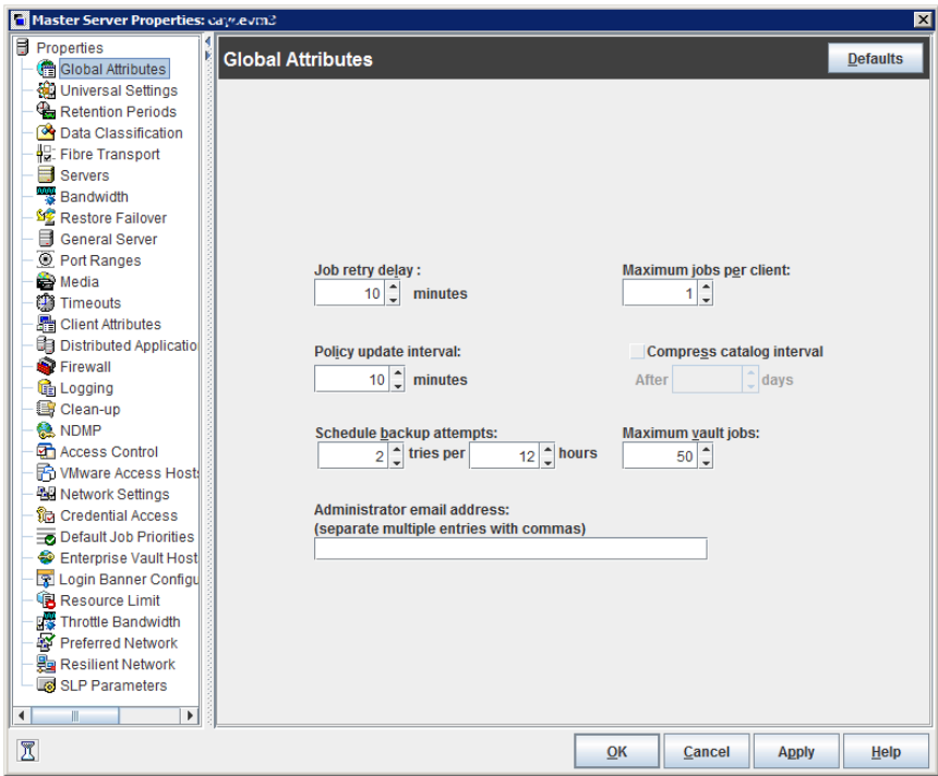
図 3-29 [グローバル属性 (Global Attributes)]ダイアログボックス
