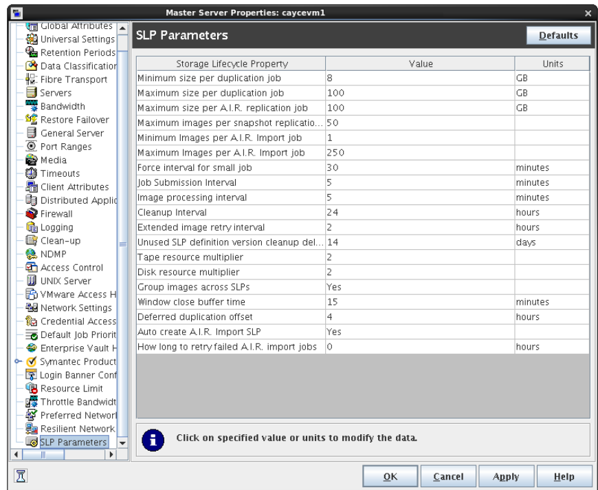
図 3-65 [SLP パラメータ (SLP Parameters)] ダイアログボックス
