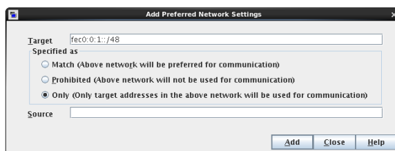
図 3-56 ソースバインドなしのアドレスの制限
