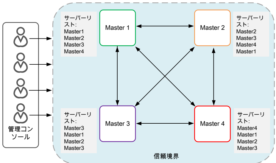
図 30-3 [サーバーの変更 (Change Server)]操作の最も柔軟なモデル
