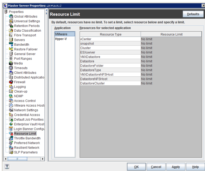
図 3-58 VMware アプリケーションが選択されている[リソース制限 (Resource Limit)]ダイアログボックス
