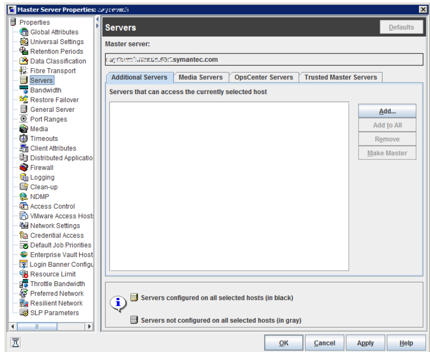
図 3-63 [サーバー (Servers)] ダイアログボックスの [追加サーバー (Additional Servers)] タブ
