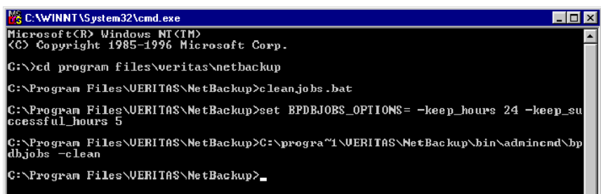
図 26-4 Windows での cleanjobs.bat の実行
