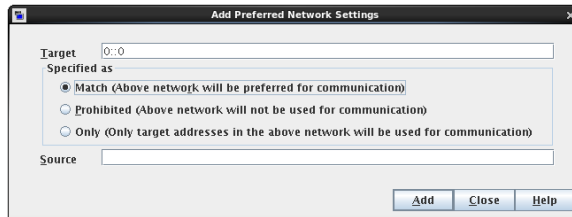
図 3-47 ターゲットとしての IPv6 アドレスの一致
