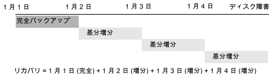
図 20-11 完全バックアップおよび差分増分バックアップの例
