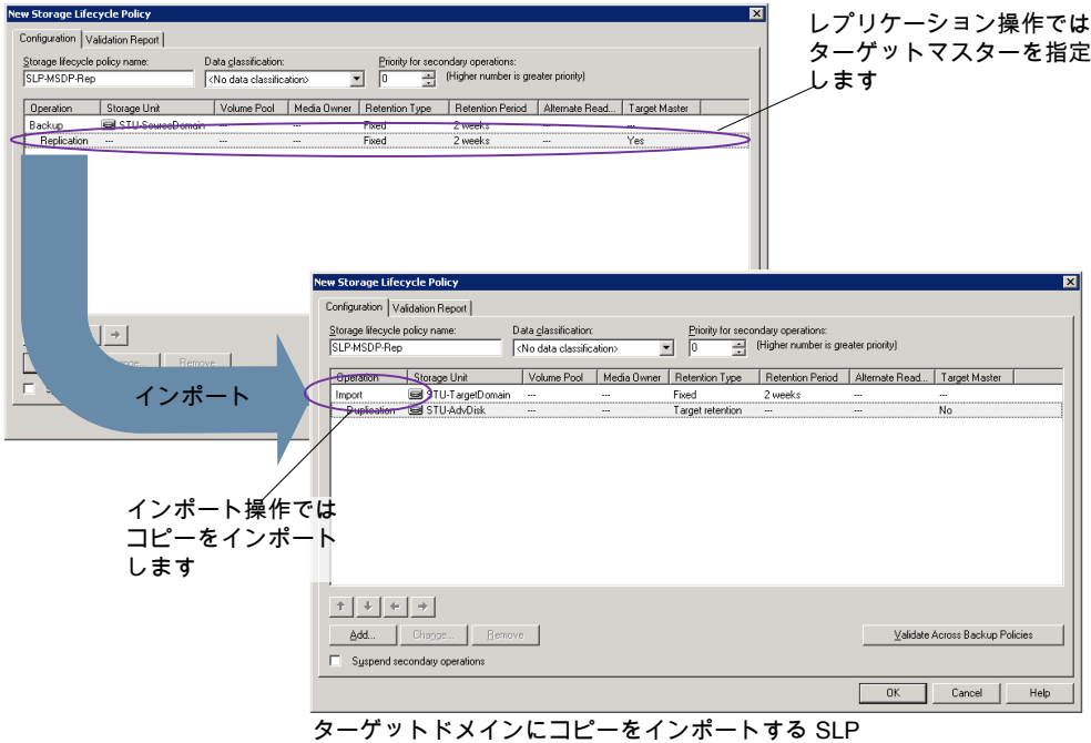
図 25-3 自動イメージレプリケーションに必要なストレージライフサイクルポリシーのペア
