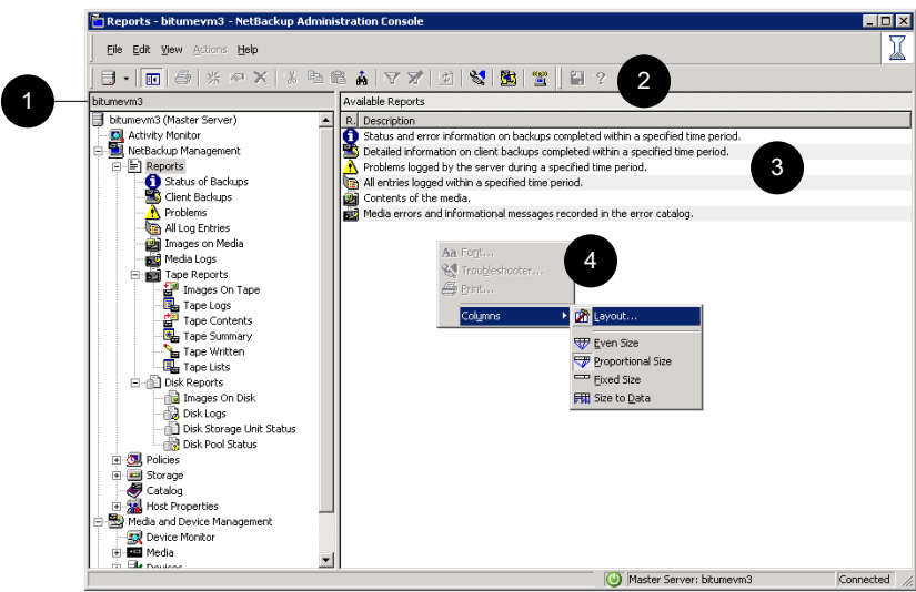
図 27-2 Java ベースの NetBackup 管理コンソールのレポートユーティリティ
