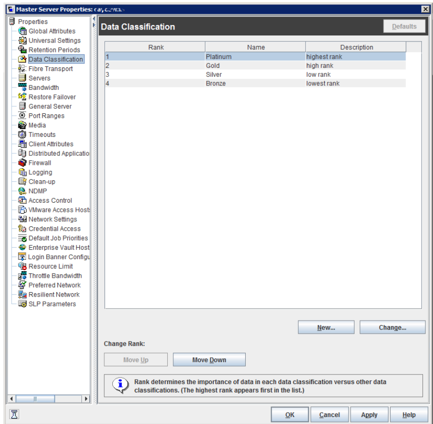
図 3-17 [データの分類 (Data Classification)]ダイアログボックス
