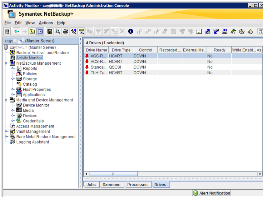
図 26-3 アクティビティ 모니터の[ドライブ (Drives)]タブ
