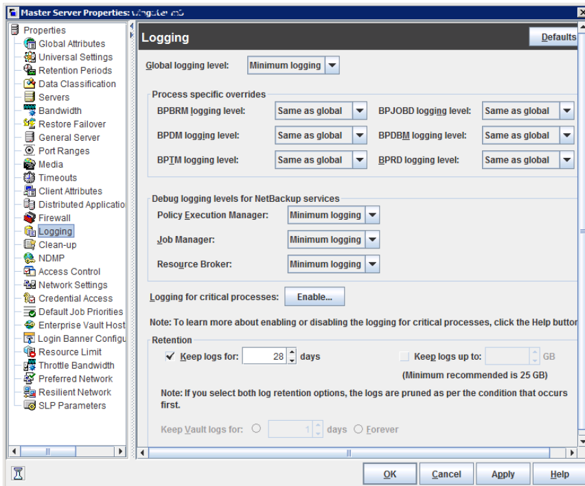
図 3-31 [ログ (Logging)] ダイアログボックス
