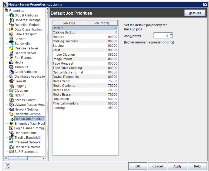
図 3-18 [デフォルトのジョブの優先度 (Default Job Priorities)] ダイアログボックス
