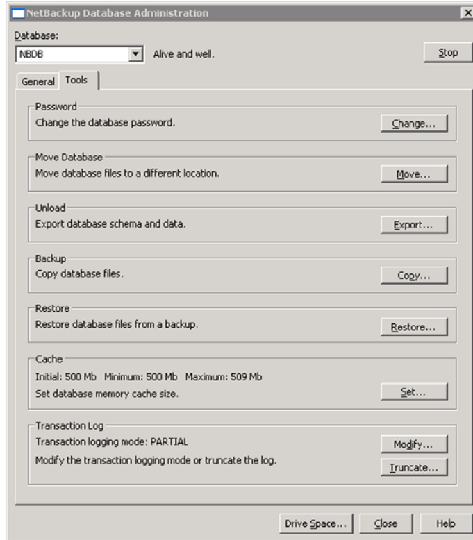
図 23-2 データベース管理ユーティリティの[ツール (Tools)]タブ
