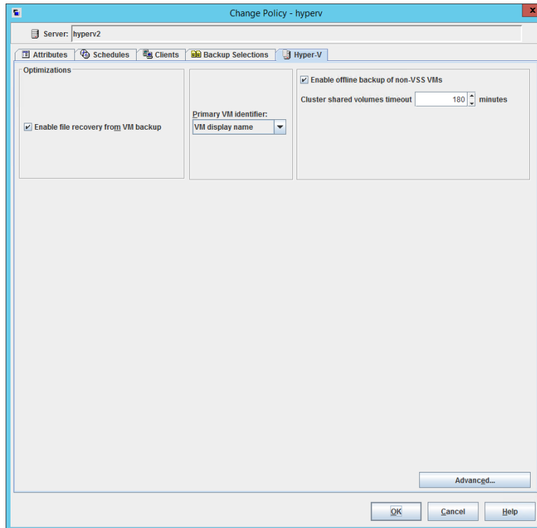
図 20-32 Hyper-V のポリシータブ
