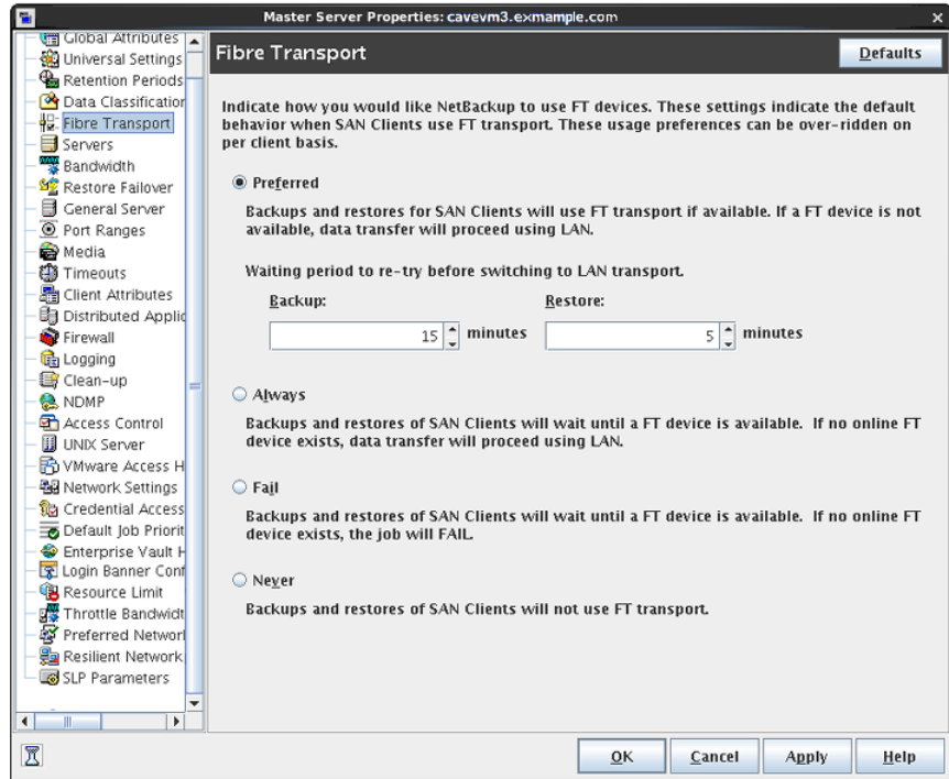
図 3-26 マスターサーバーの[ファイバートランスポート (Fibre Transport)]ホストプロパティ
