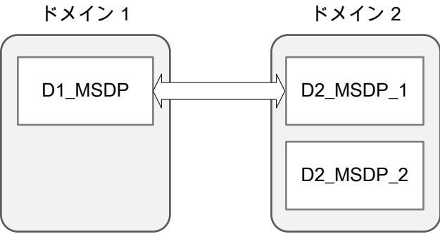
図 25-9 処理前のレプリケーショントポロジの例
