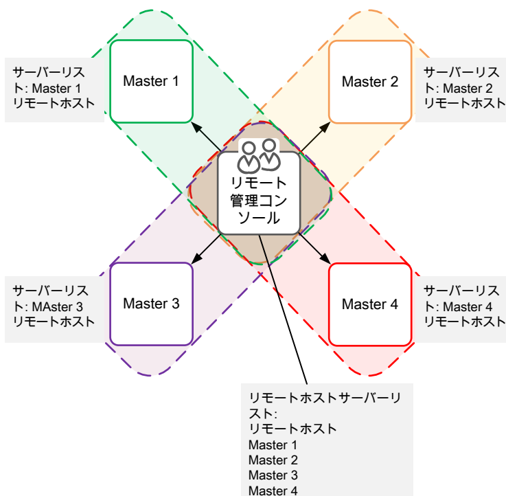
図 30-2 Windows 管理コンソールのホストベースのセキュリティモデル
