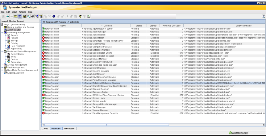
図 26-2 アクティビティ 모니터の[デーモン (Daemons)]タブ
