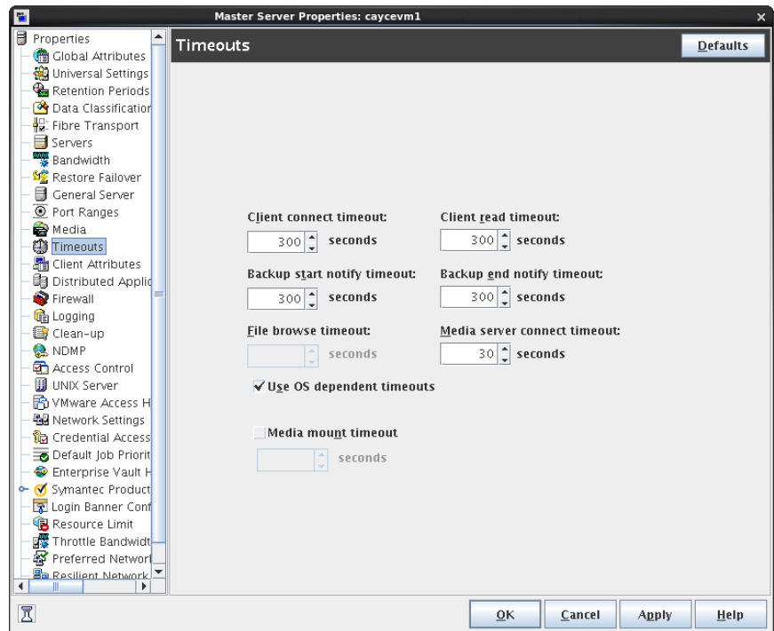
図 3-67 [タイムアウト (Timeouts)] ダイアログボックス
