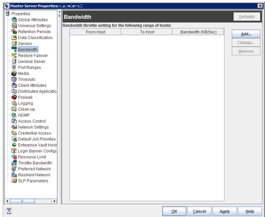
図 3-7 [帯域幅 (Bandwidth)] ダイアログボックス
