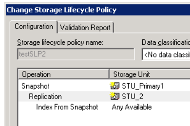
図 15-8 [スナップショットからのインデックス (Index From Snapshot)] 操作の有効な配置の例 1
