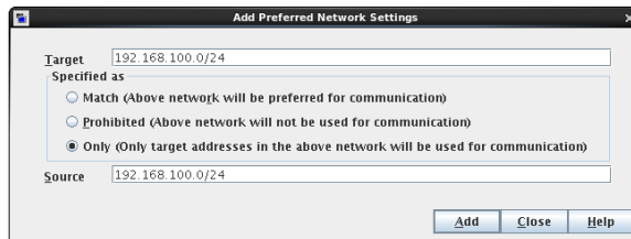
図 3-55 同じソースバインドアドレスでの[単独 (Only)]ネットワークの選択
