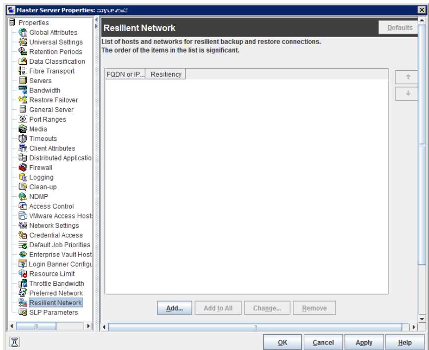
図 3-57 マスターサーバーの耐性ネットワークホストのプロパティ
