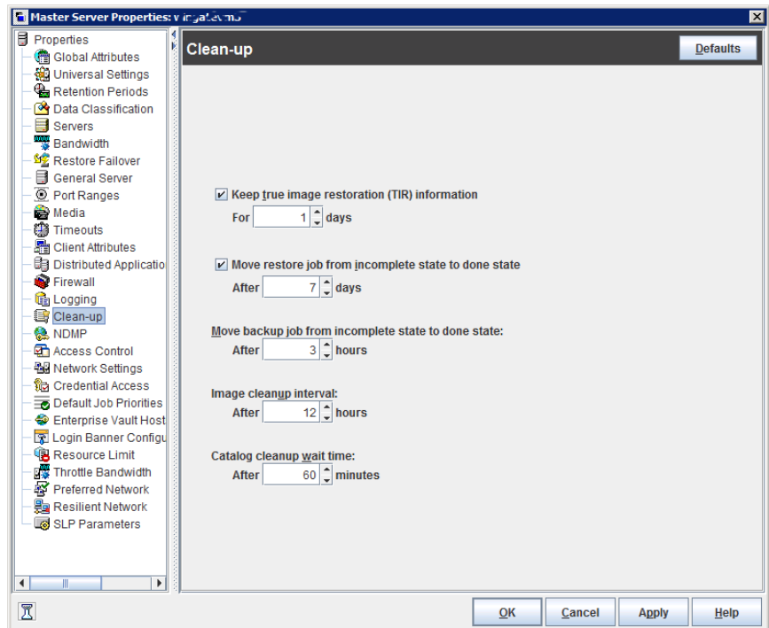
図 3-9 [クリーンアップ (Clean-up)] ダイアログボックス
