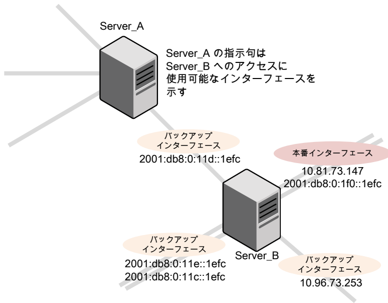
図 3-43 マルチホームサーバーの例
