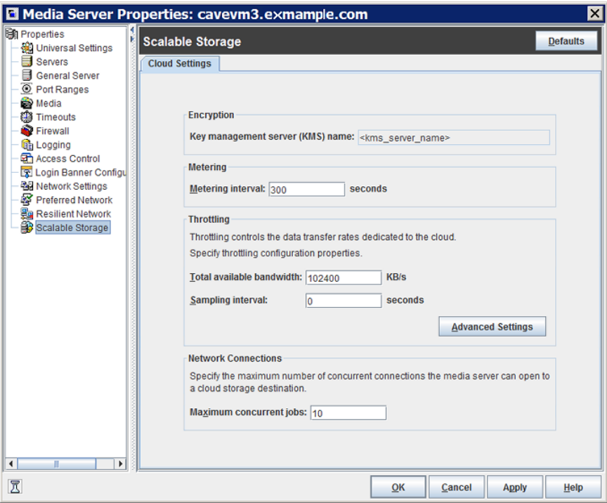
図 3-62 [拡張性のあるストレージ (Scalable Storage)]の[クラウドの設定 (Cloud Settings)]ホストプロパティ
