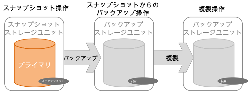
図 15-13 スナップショット操作、スナップショットからのバックアップ操作、および複製操作を含む SLP
