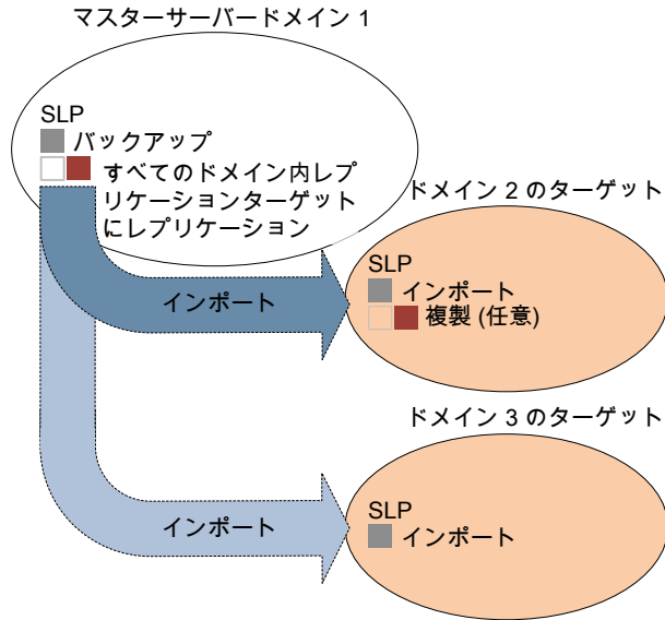
図 25-4 1 つのドメインからすべてのドメイン間マスターサーバーへのレプリケーション
