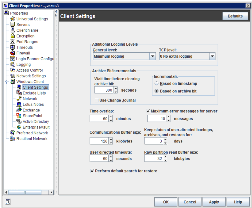
図 3-15 Windows の [クライアントの設定 (Client Settings)] ダイアログボックス
