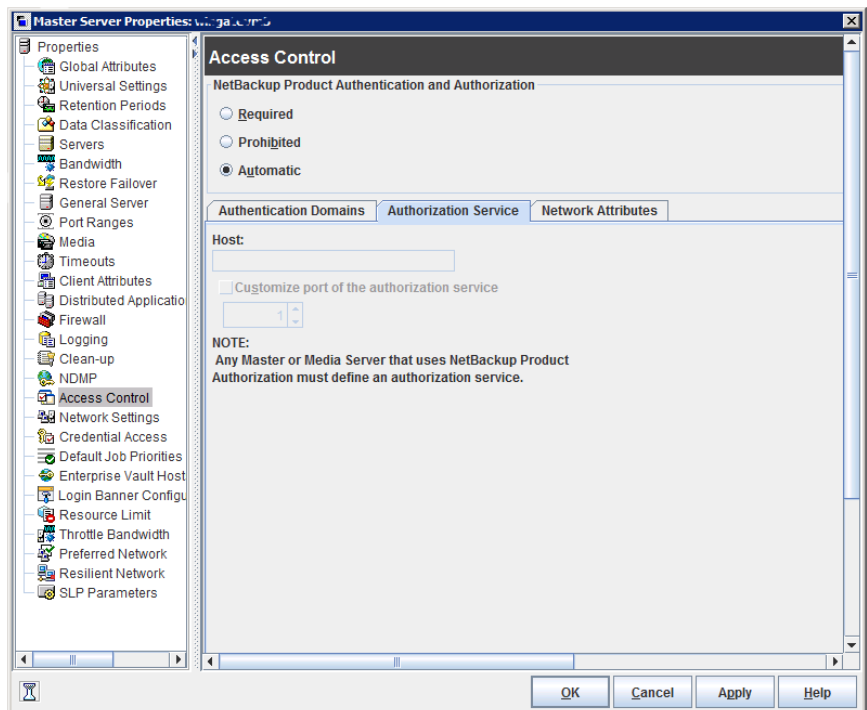
図 3-3 [認可サービス (Authorization Service)]タブ
