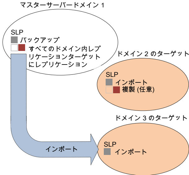
図 25-5 1つのドメインから特定のドメイン間マスターサーバーへのレプリケーション
