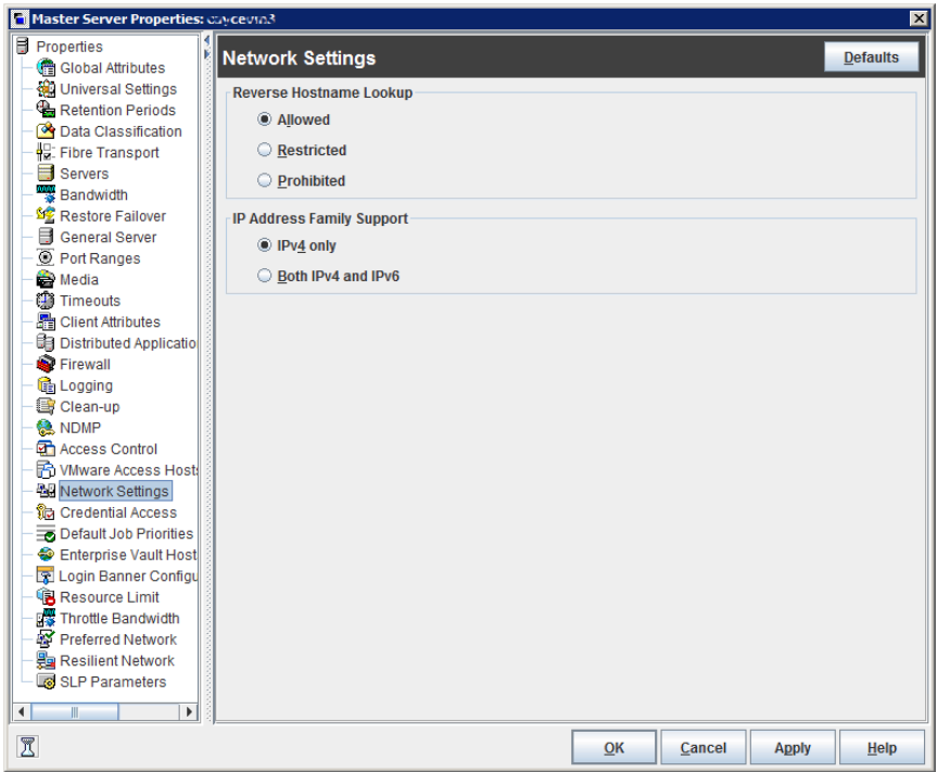
図 3-40 [ネットワーク設定 (Network Settings)]ダイアログボックス
