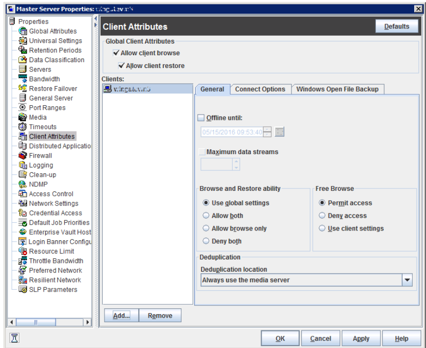
図 3-11 [クライアント属性 (Client Attributes)]ダイアログボックスの[全般 (General)]タブ
