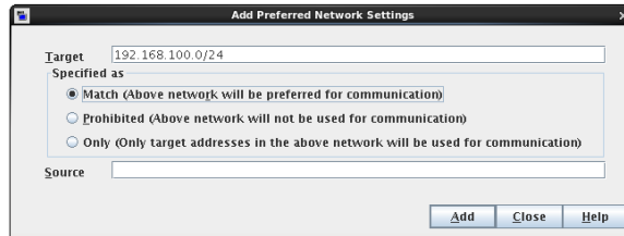
図 3-54 ソースでの[一致 (Match)]ネットワークの選択
