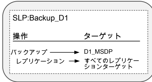
図 25-10 ストレージライフサイクルポリシーのトポロジーの例
