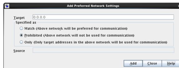
図 3-46 ターゲットとしての IPv4 アドレスの禁止
