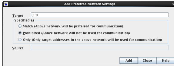
図 3-49 ターゲットとしての IPv6 アドレスの禁止
