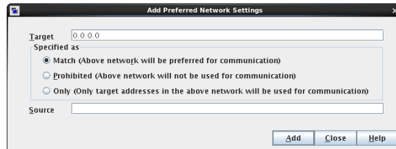
図 3-50 ターゲットとしての IPv4 アドレスの一致
