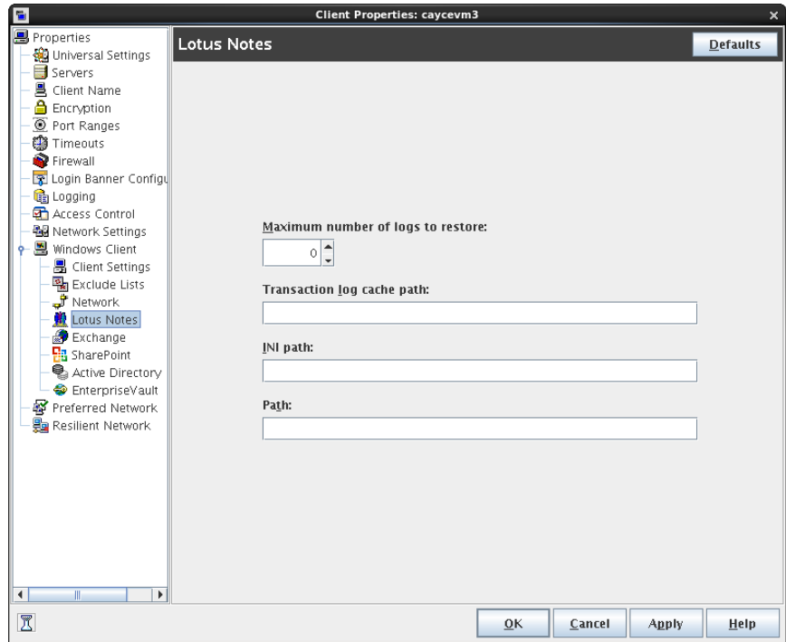
図 3-35 [Lotus Notes]ダイアログボックス
