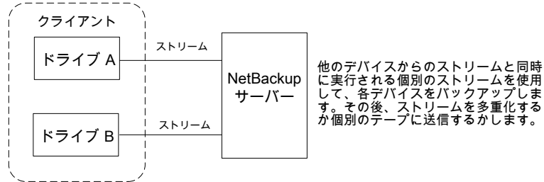
図 20-6 推奨する複数ストリームの使用方法
