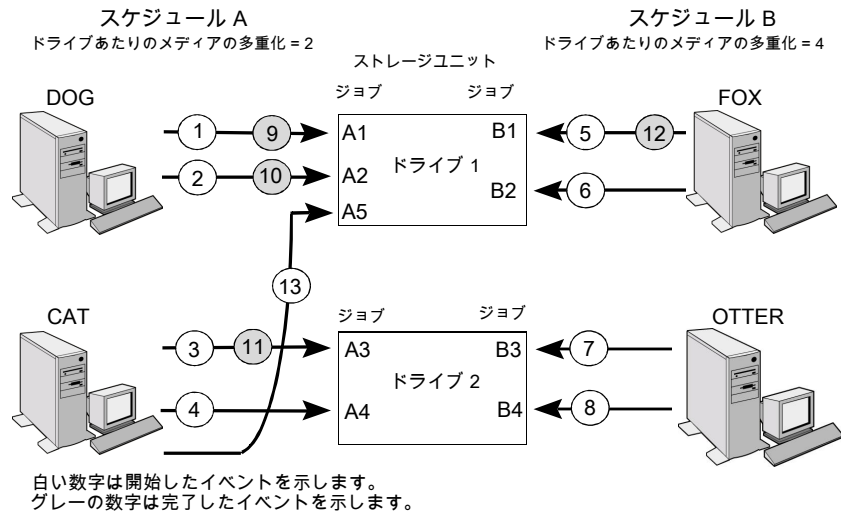
図 20-14 多重化処理のシナリオ
