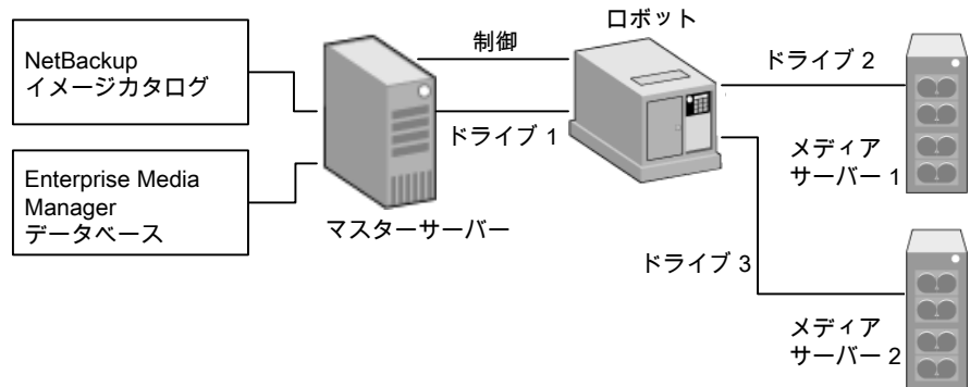
図 32-1 ロボットの周辺機器を共有する NetBackup サーバー
