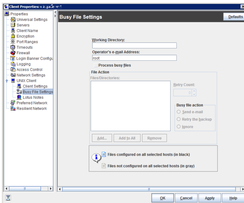
図 3-8 [ビジー状態のファイルの設定 (Busy File Settings)]ダイアログボックス
