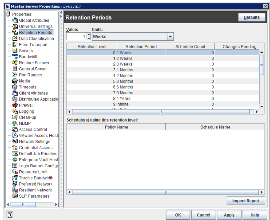
図 3-61 [保持期間 (Retention Periods)]ダイアログボックス
