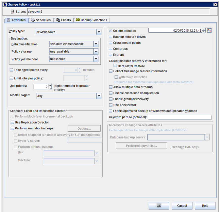
図 20-2 ポリシーの[属性 (Attributes)]タブ
