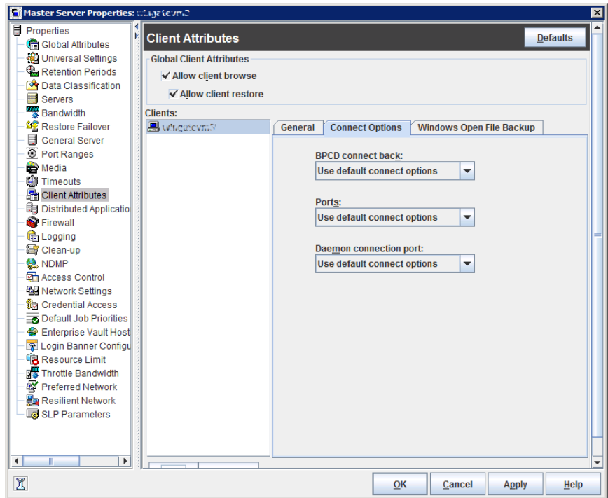
図 3-12 [クライアント属性 (Client Attributes)]ダイアログボックスの[接続オプション (Connect Options)]タブ
