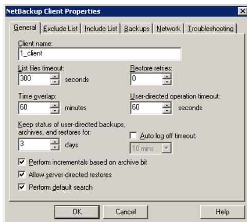
図 22-3 クライアントの[ファイルリスト取得のタイムアウト (List Files Timeout)]一般プロパティ
