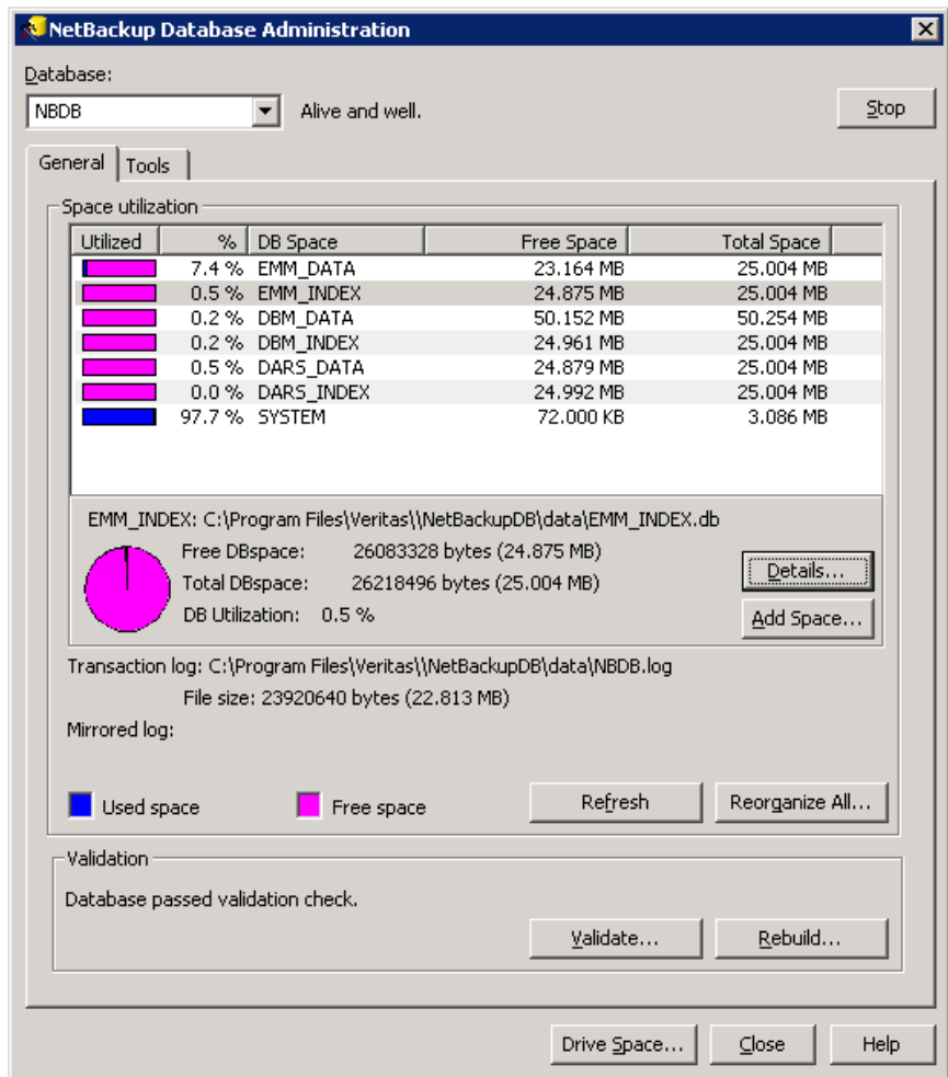
図 23-1 NetBackup データベース管理ユーティリティの[一般 (General)]タブ
