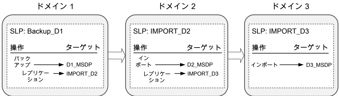
図 25-12 ストレージライフサイクルポリシーのトポロジーの例
