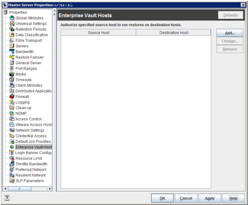
図 3-22 [Enterprise Vault ホスト (Enterprise Vault Hosts)] マスターサーバープロパティ
