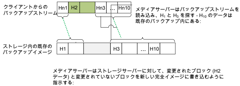
図 20-8 NetBackup メディアサーバーはバックアップイメージを構築する
