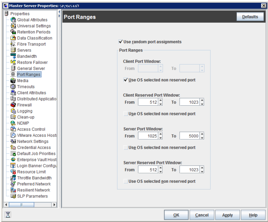
図 3-41 [ポートの範囲 (Port Ranges)]ダイアログボックス
