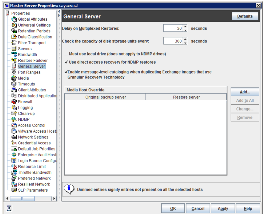
図 3-28 [一般的なサーバー (General Server)]ダイアログボックス
