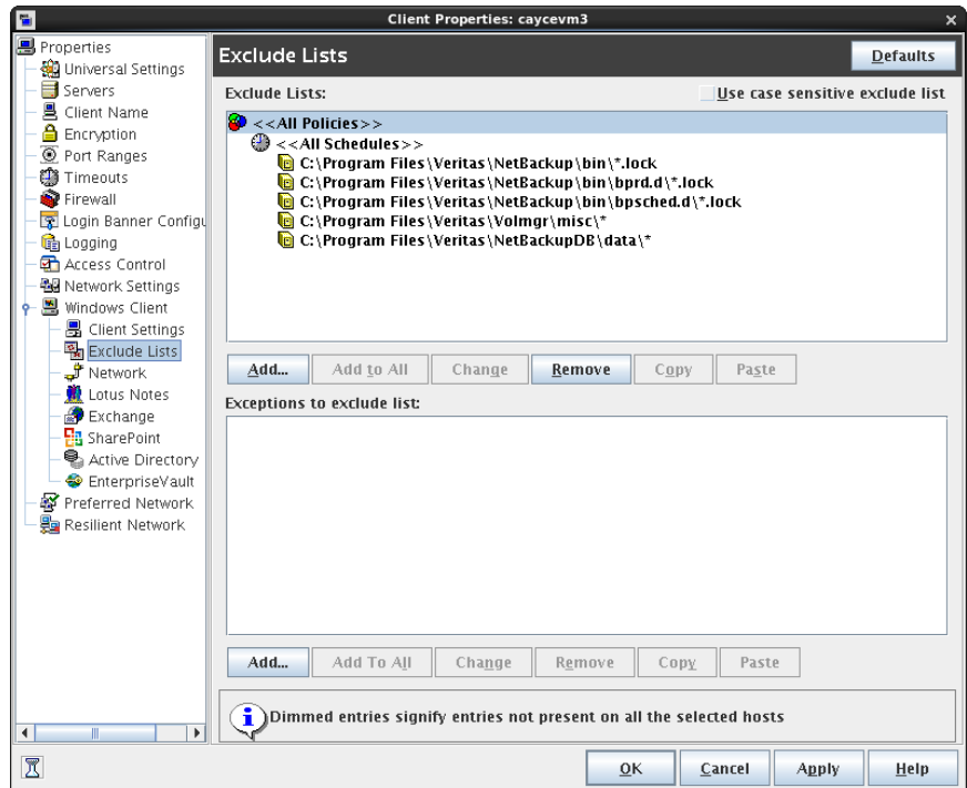
図 3-24 [エクスクルードリスト (Exclude Lists)] ダイアログボックス
