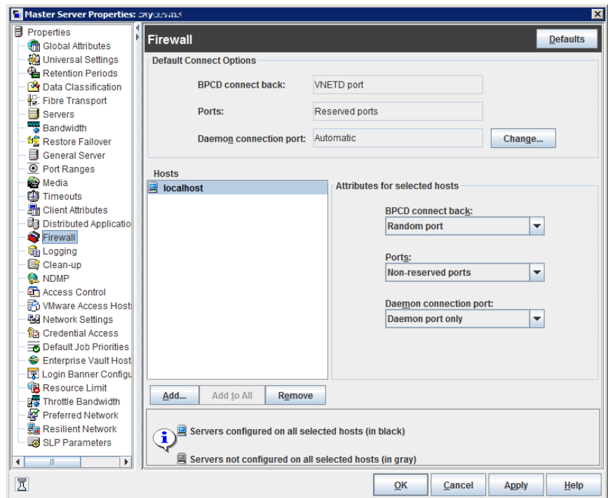
図 3-27 [ファイアウォール (Firewall)] ダイアログボックス
