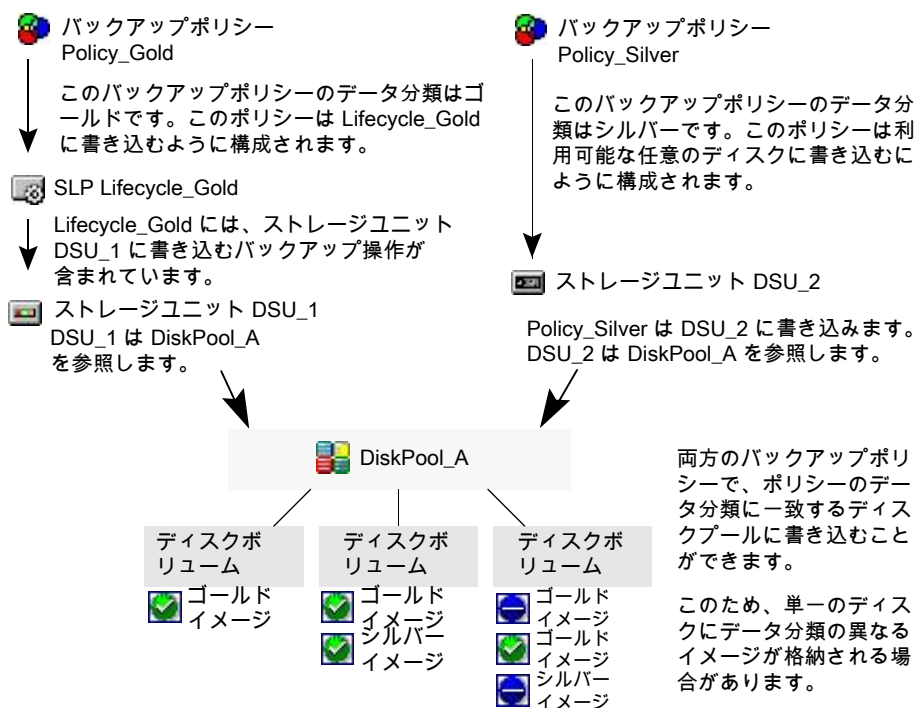
図 11-4 ディスクプールを参照するストレージライフサイクルポリシーおよびディスクストレージユニット
