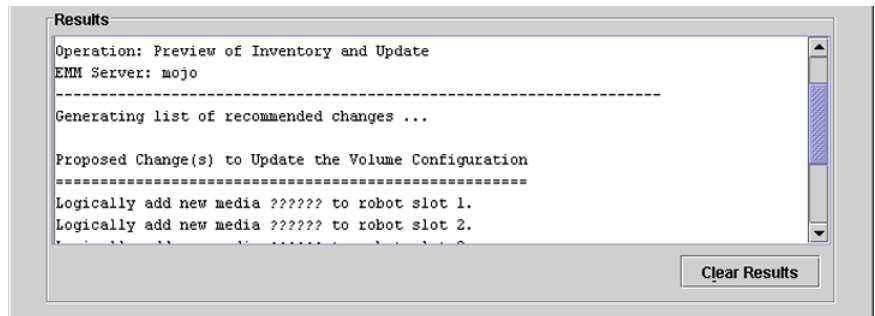
図 10-4 [ボリューム構成の変更をプレビュー表示 (Preview volume configuration changes)](API 以外のロボット)
