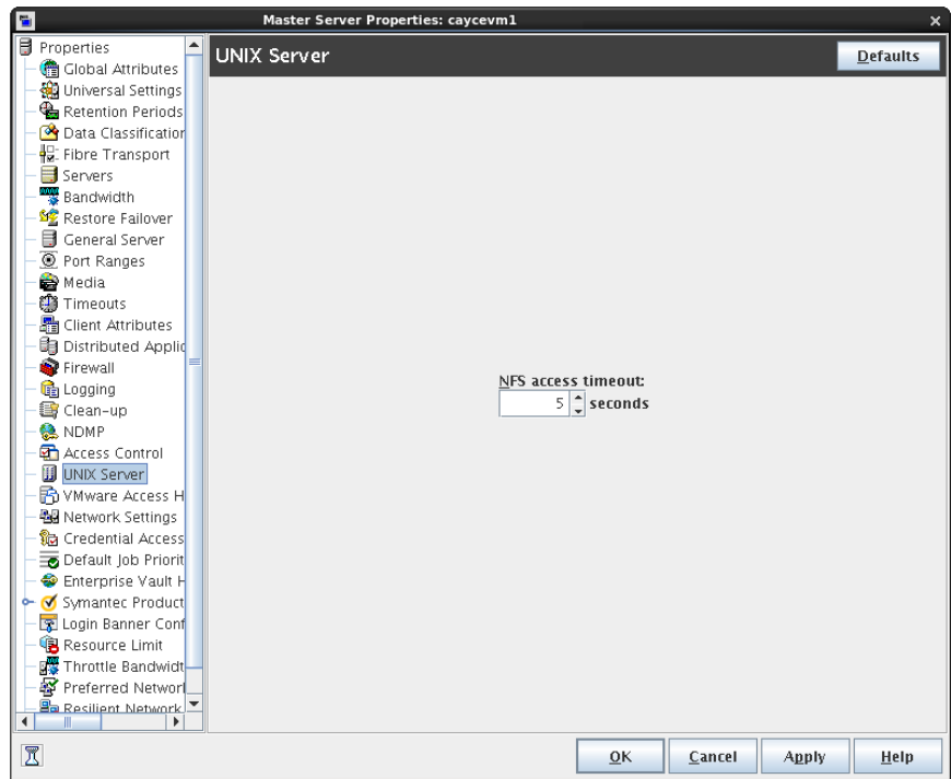
図 3-70 [UNIX サーバー (Unix Server)]ダイアログボックス
