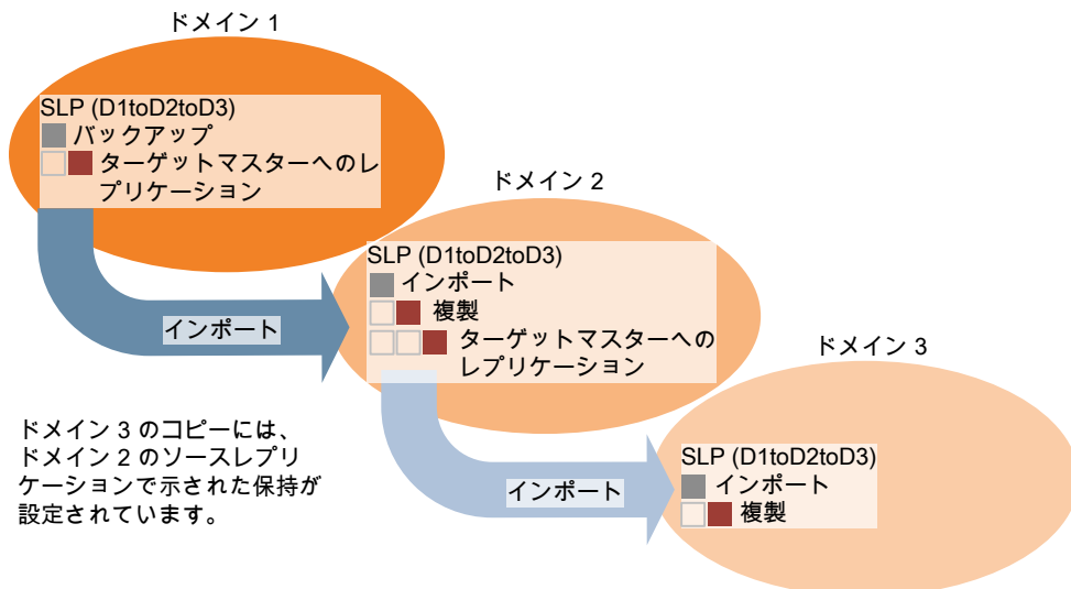
図 25-2 ささまざまなターゲットの保持によるターゲットのマスターサーバーへのレプリケーションのカスケード
