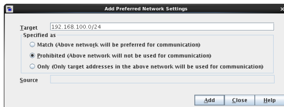
図 3-53 禁止されたターゲットの例
