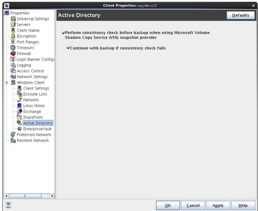
図 3-6 [Active Directory]ダイアログボックス
