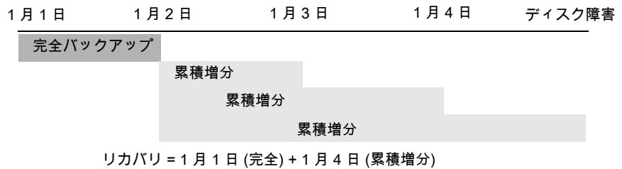
図 20-12 完全バックアップおよび累積増分バックアップの例
