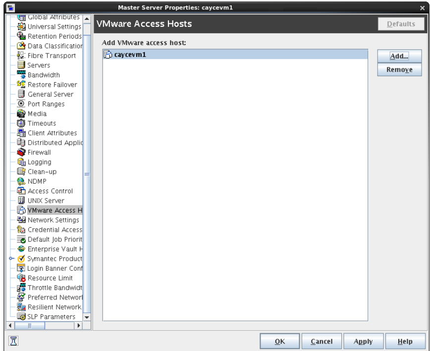
図 3-71 [VMware アクセスホスト (VMware Access Hosts)]ダイアログボックス
