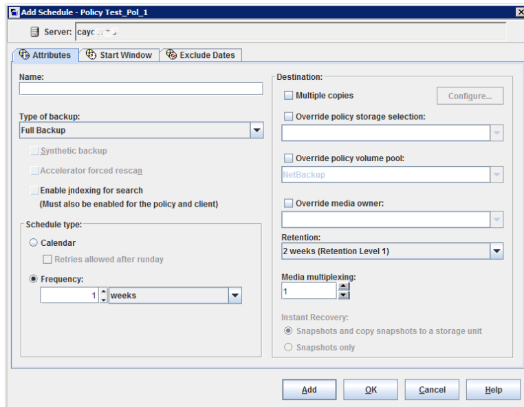
図 20-10 スケジュールの[属性 (Attributes)]タブ
