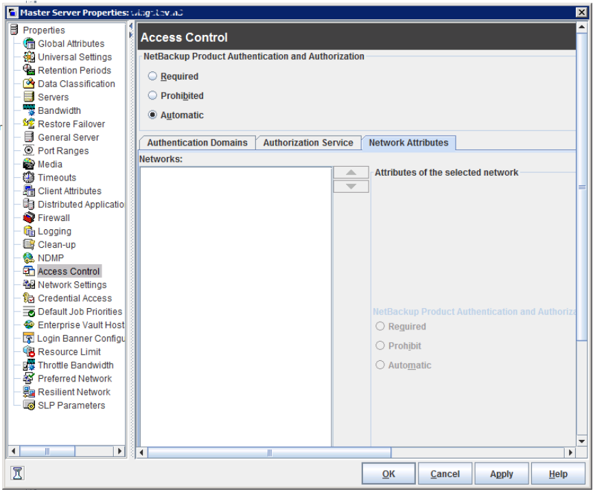
図 3-4 [ネットワーク属性 (Network Attributes)]タブ
