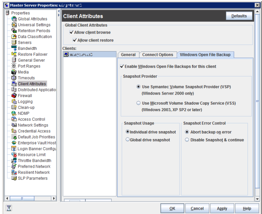
図 3-13 [クライアント属性 (Client Attributes)]ダイアログボックスの[Windows Open File Backup]タブ
