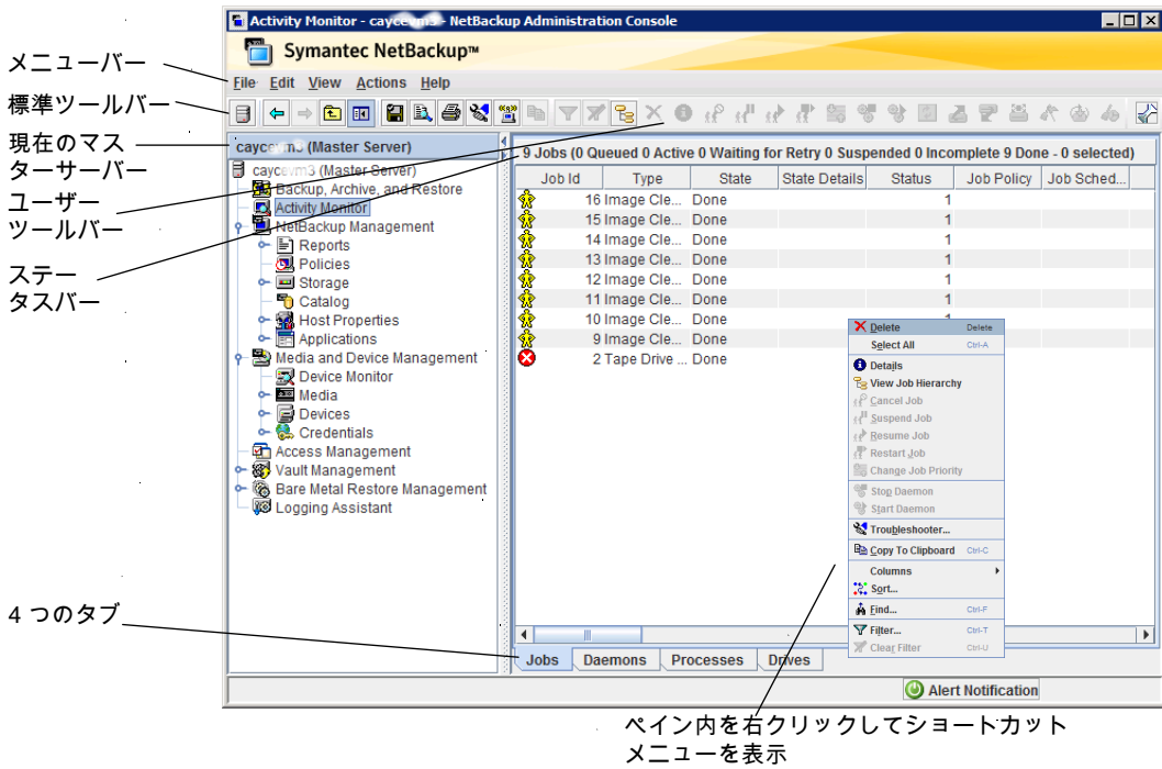
図 26-1 アクティビティモニター
