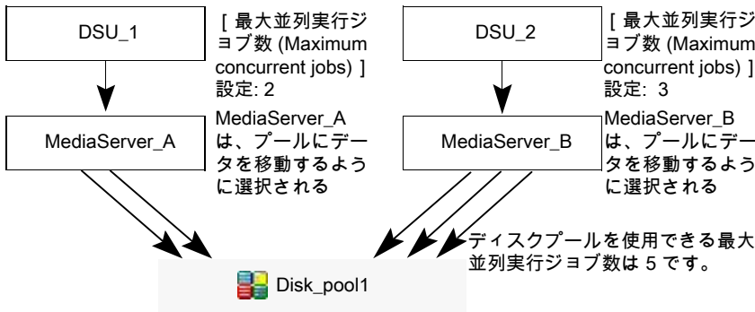
図 11-6 複数のディスクストレージユニットが1つのディスクプールと異なるメディアサーバーを使用する場合の影響
