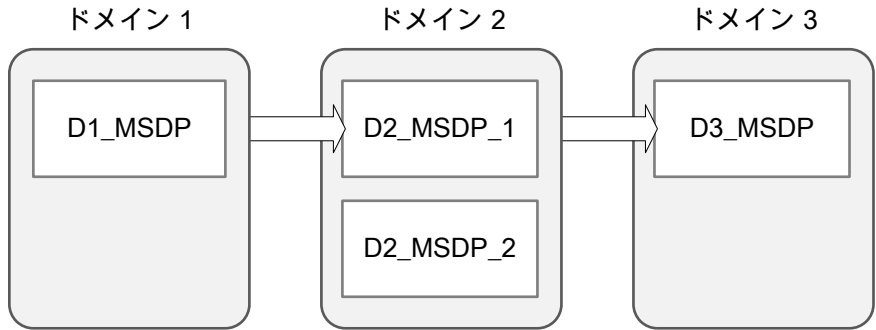
図 25-12 ストレージライフサイクルポリシーのトポロジーの例
