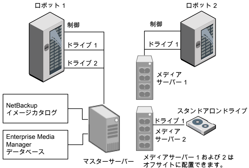
図 32-2 個別の非共有周辺機器を使用する NetBackup サーバー
