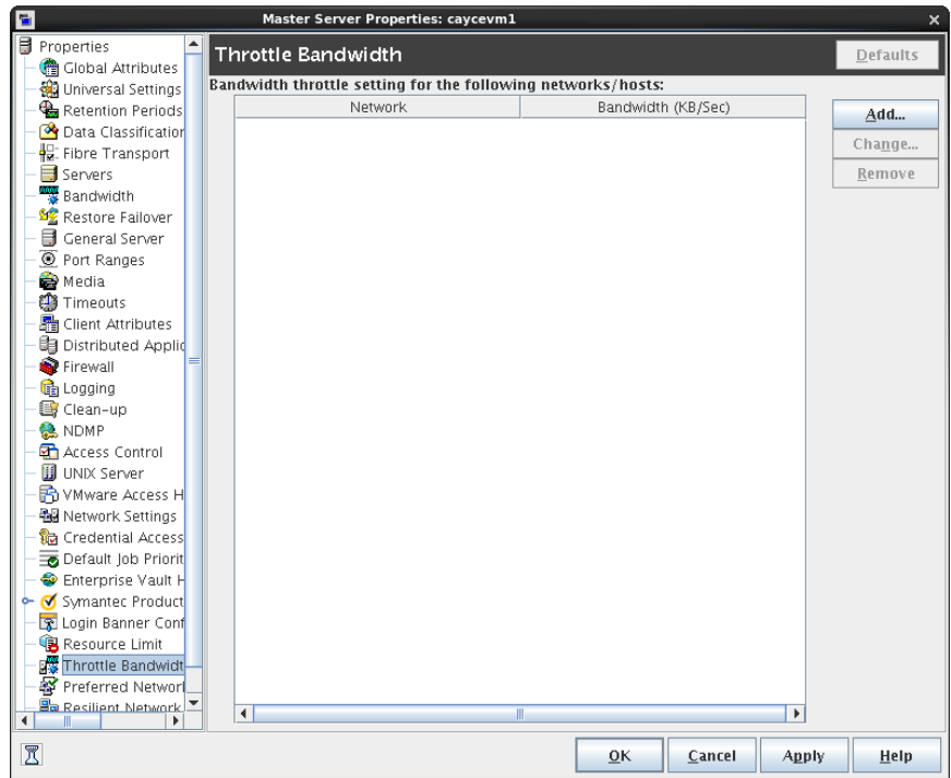
図 3-66 [帯域幅スロットル (Throttle Bandwidth)]ダイアログボックス
