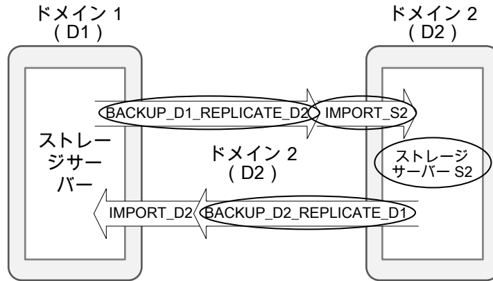
図 25-8 変更後のトポロジー
