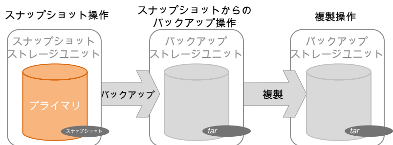
図 6-2 スナップショット操作、スナップショットからのバックアップ操作、および複製操作を含む SLP
