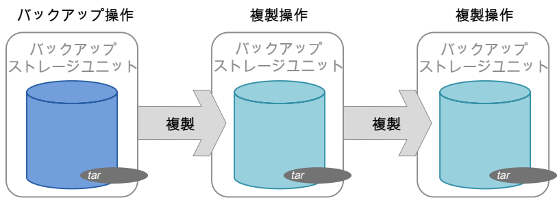
図 6-13 1 つのバックアップ操作と 2 つの複製操作を含む SLP
