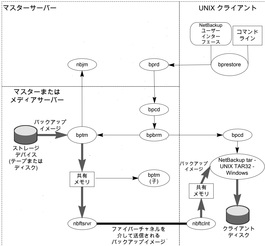
図 4-4 ファイバートランスポートを介した SAN クライアントのリストア
