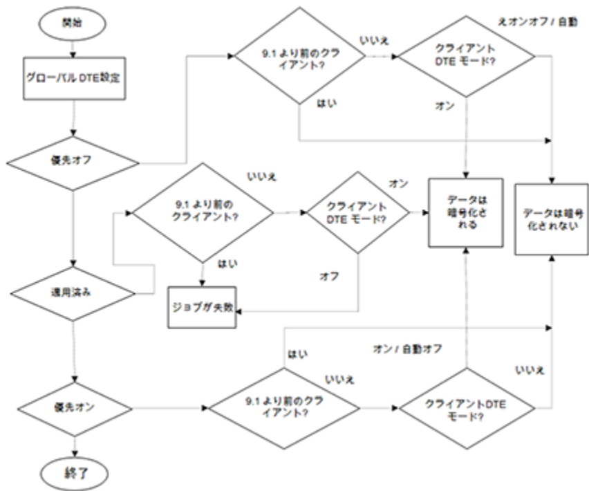
図 22-1 バックアップのワークフロー
