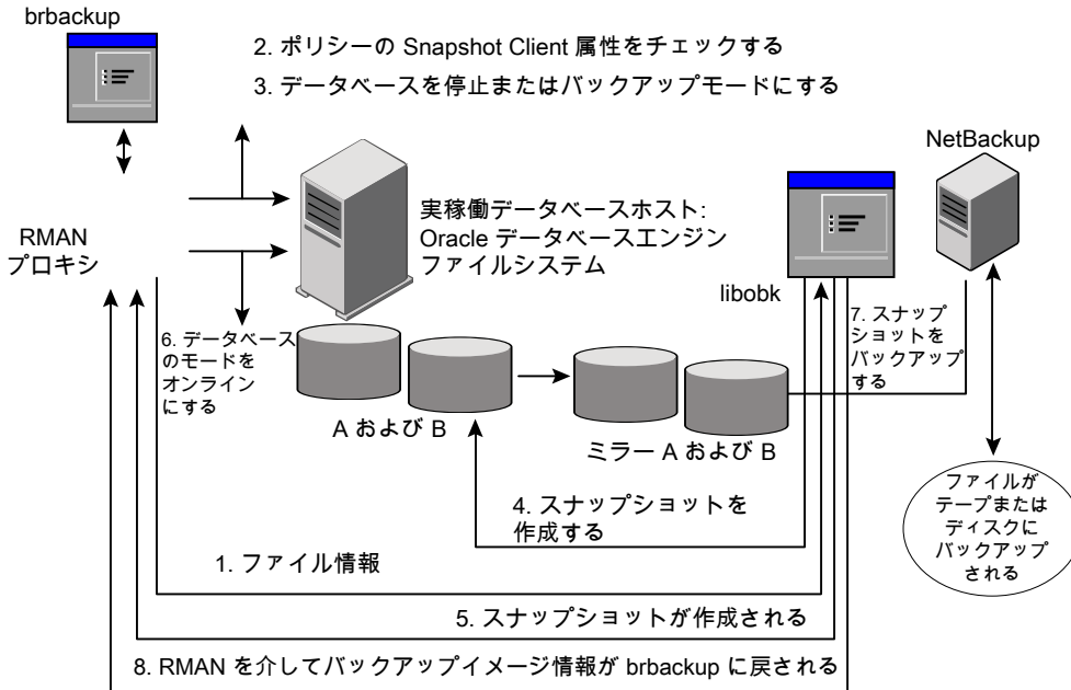
図 12-3 RMAN プロキシを使った SAP Oracle のオンラインバックアップおよびオフラインバックアップ
