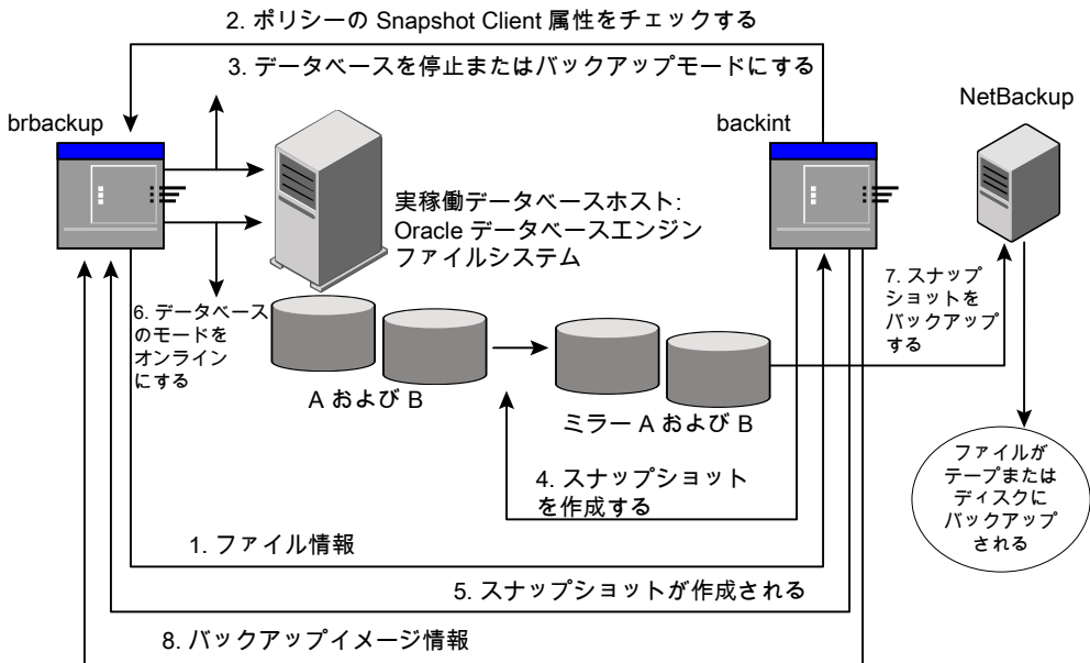
図 12-2 brbackup コマンドと backint コマンドを使った SAP Oracle のオンラインバックアップおよびオフラインバックアップ
